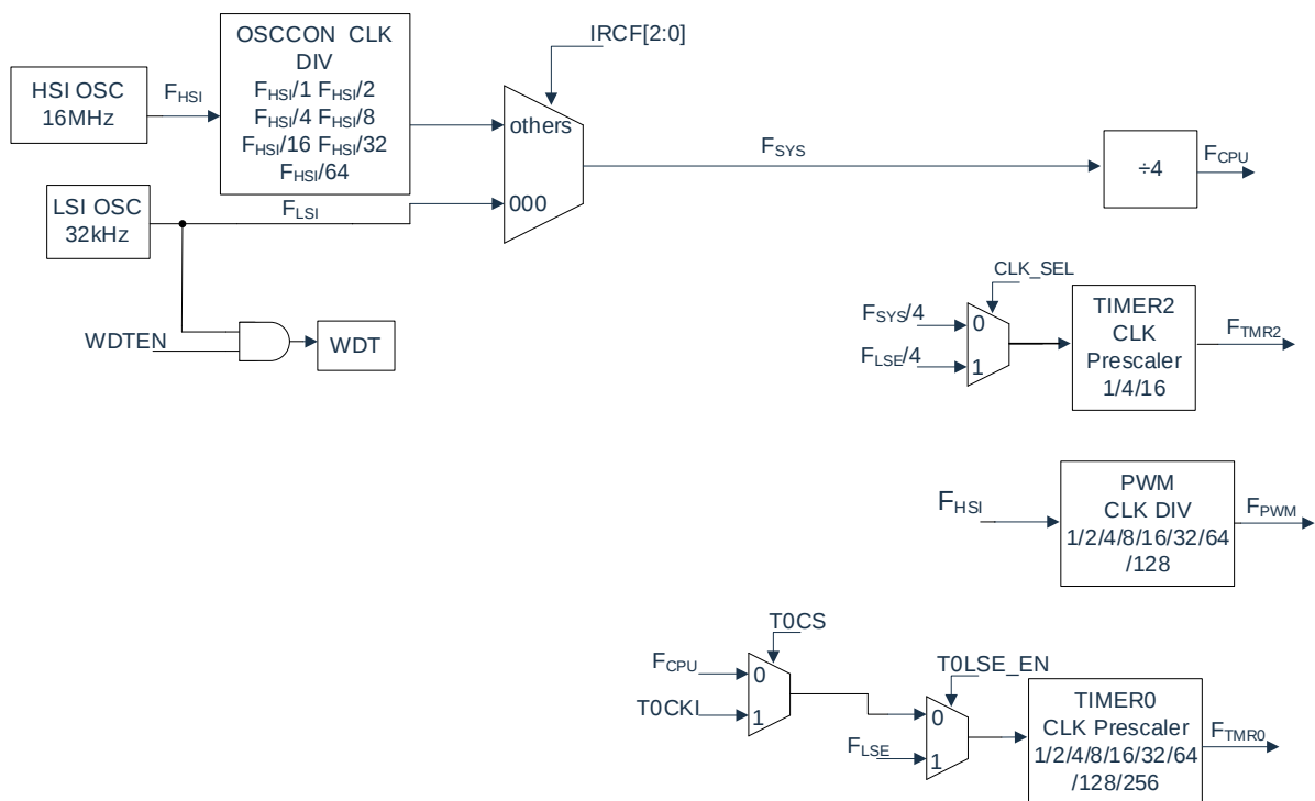
图 3-2: 时钟框图
