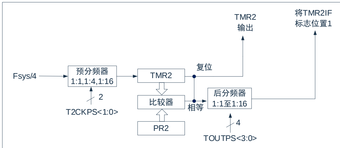
图 9-1: TIMER2 框图
