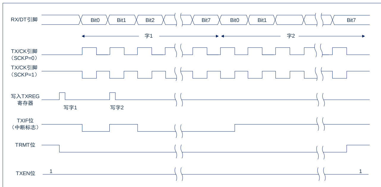
图 18-6：同步发送
