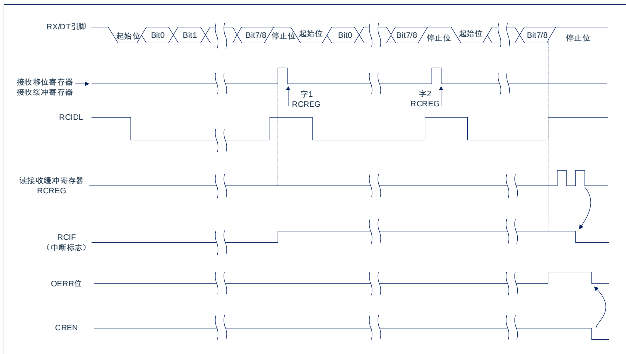
图 17-5: 异步接收
