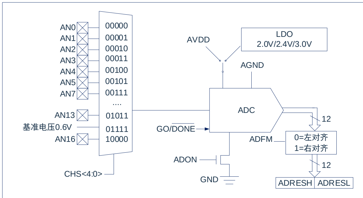
图 11-1：ADC 框图
