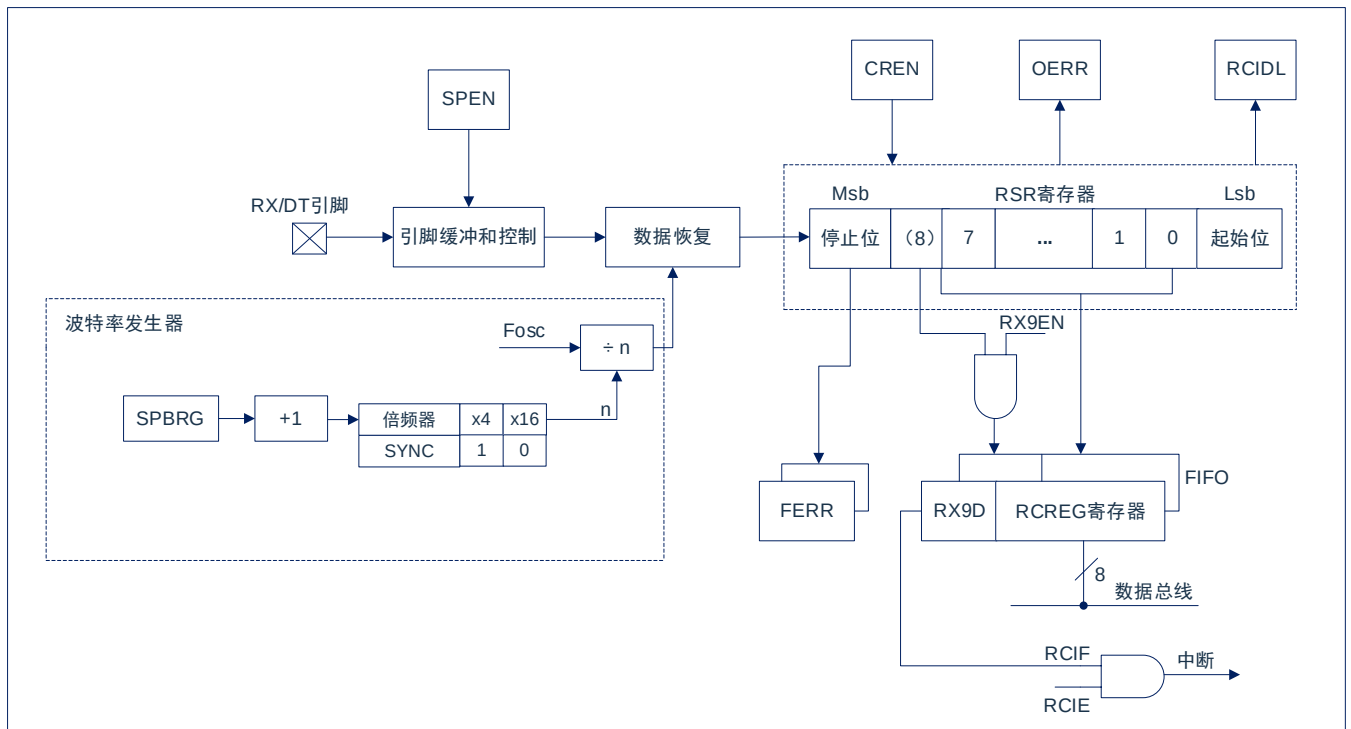
图17-2: USART接收框图
