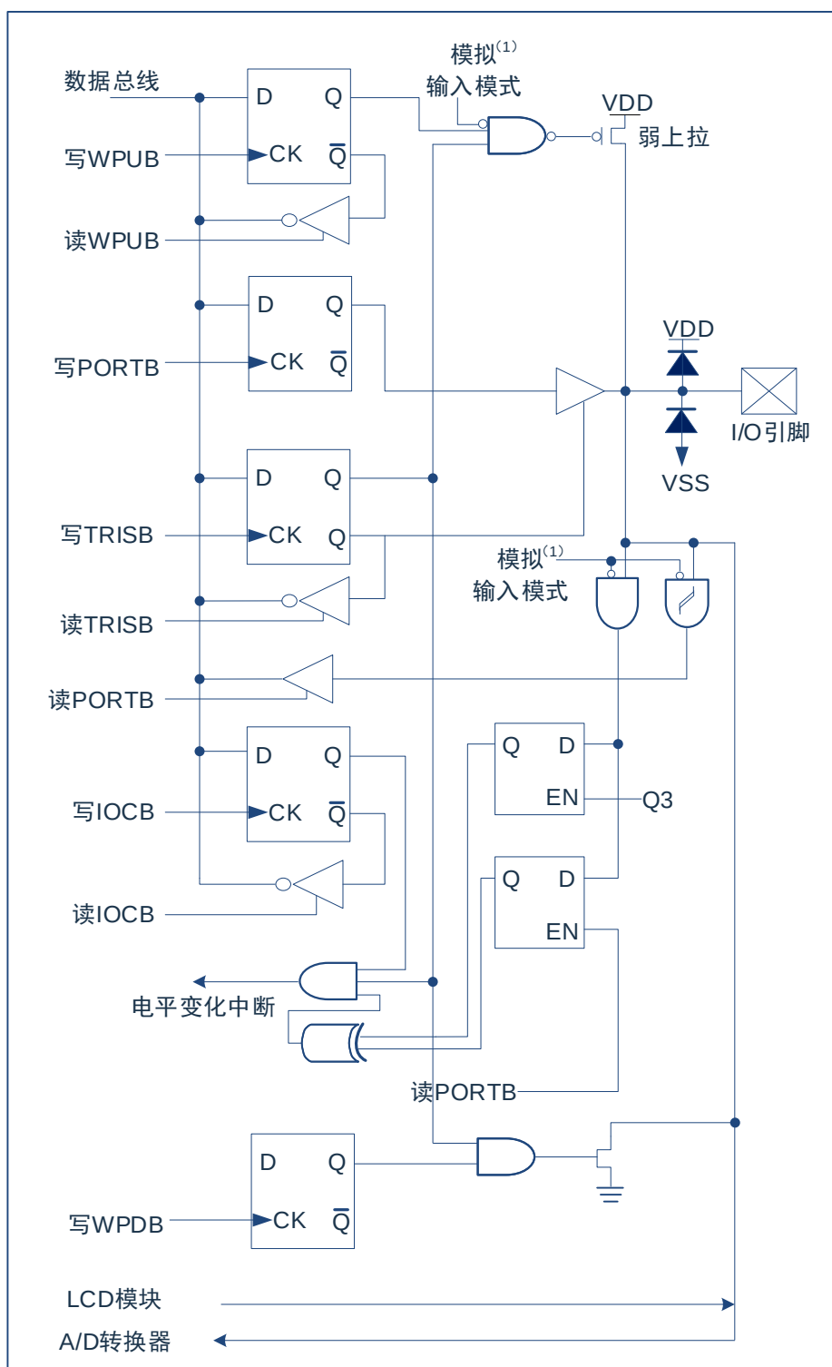
图 6-2: I/O 口结构图
