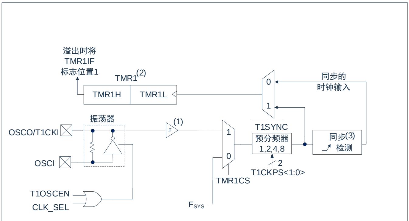
图9-1: TIMER1结构图
