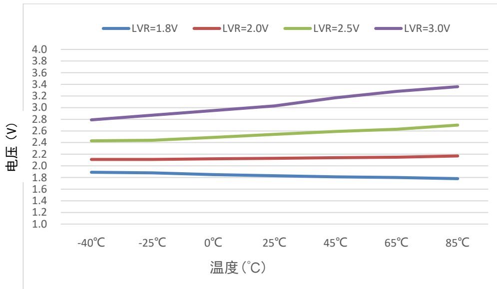
LVR 温度特性曲线
