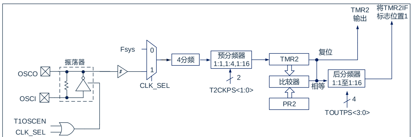
图 10-1: TIMER2 框图
