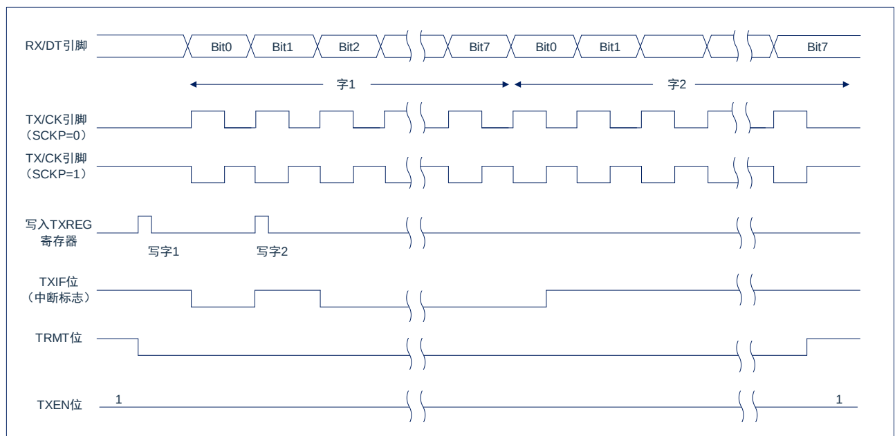
图 17-6：同步发送
