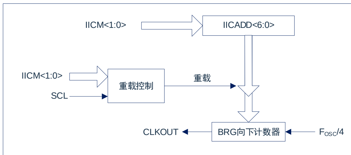
图19-3：波特率发生器框图
