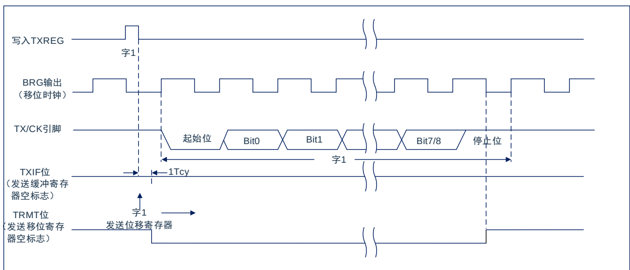
图 17-3: 异步发送
