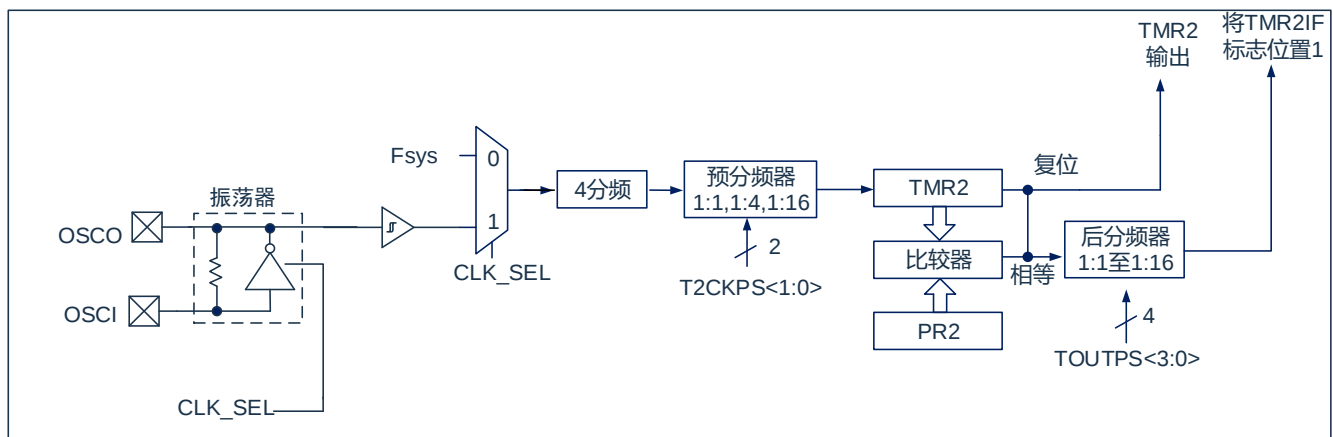
图 9-1：TIMER2 框图
