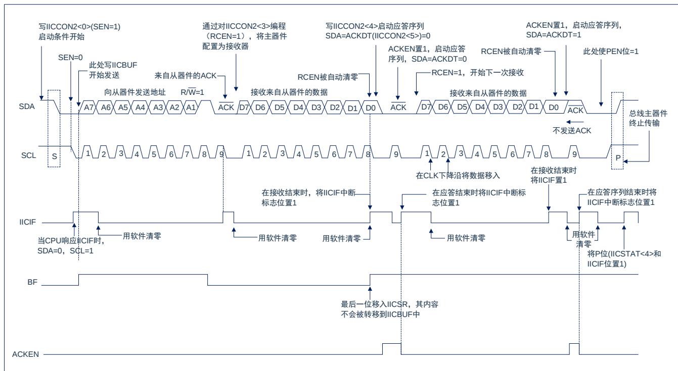
图17-6: I²C™主控模式接收时序
