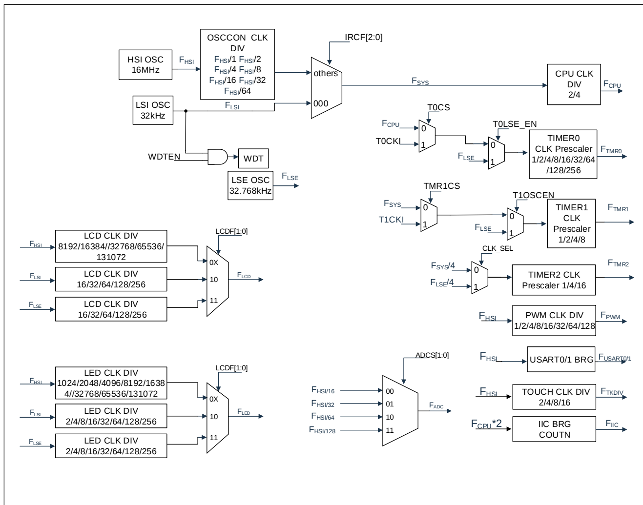
图 3-3: 时钟框图
