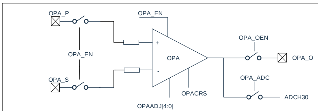
图 19-1: OPA 框图
