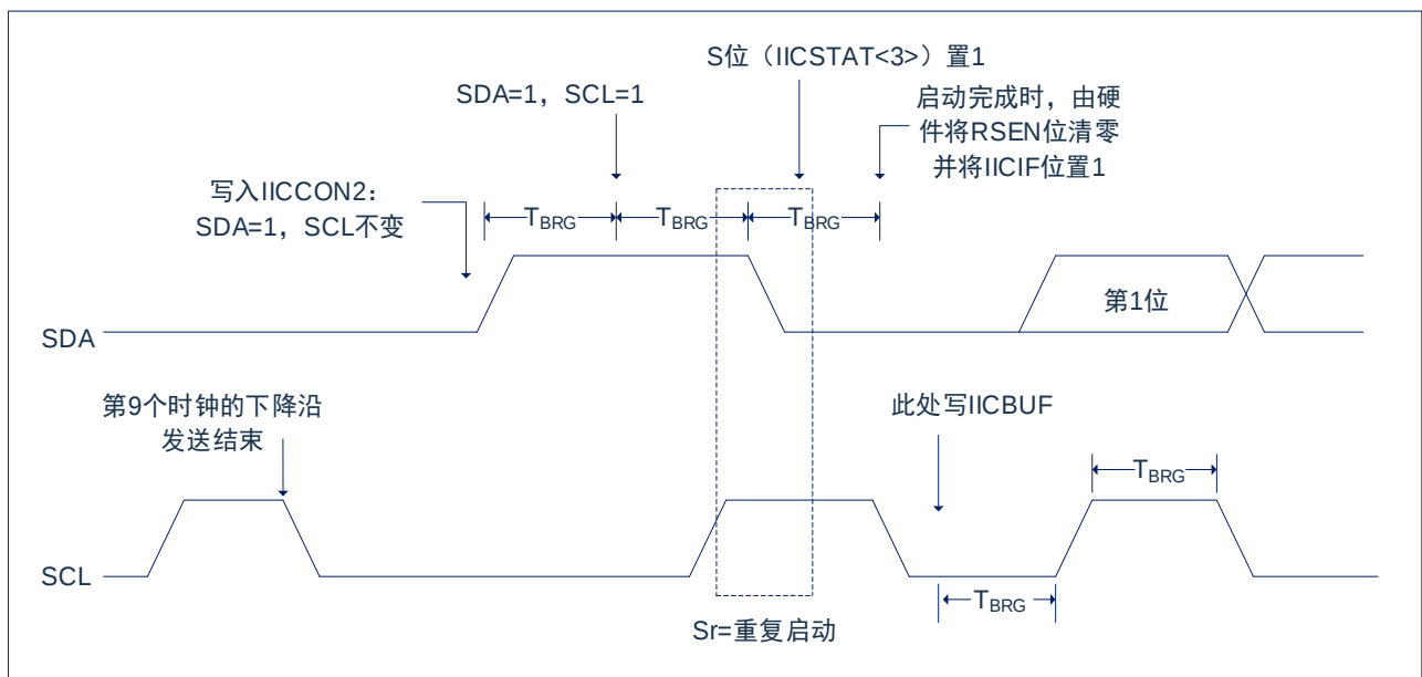
图20-8：重复启动条件时序波形
