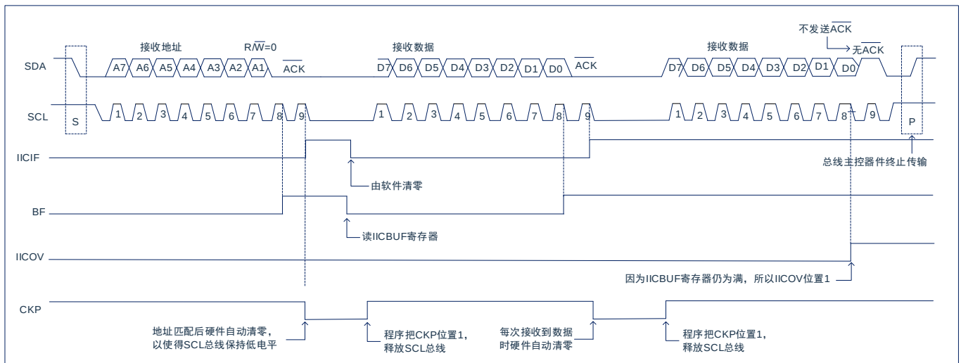
图 20-12: I²C™ 从动模式接收时序
