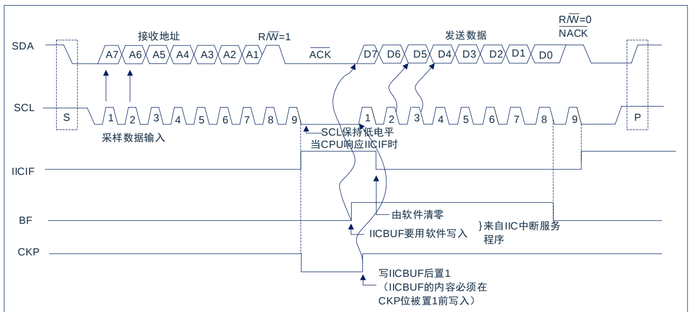
图 20-13: I²C™ 从动模式发送时序
