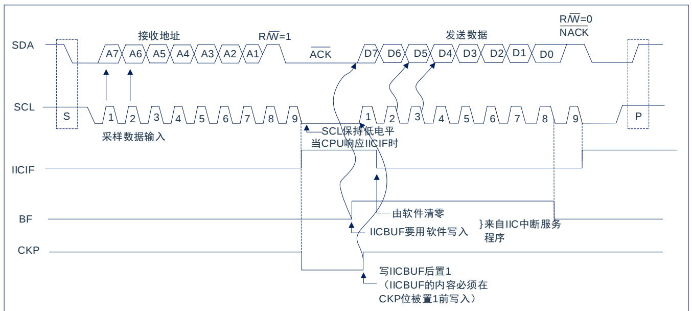
图 18-13: I²C™ 从动模式发送时序
