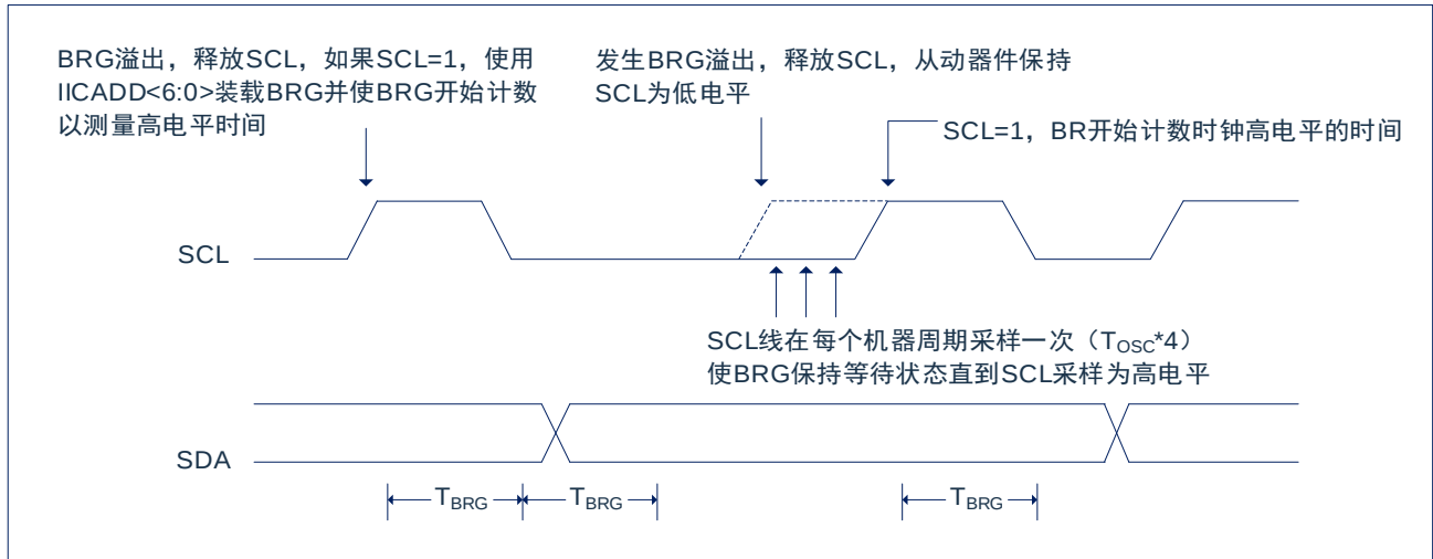
图 18-11：主控发送模式下的时钟仲裁时序
