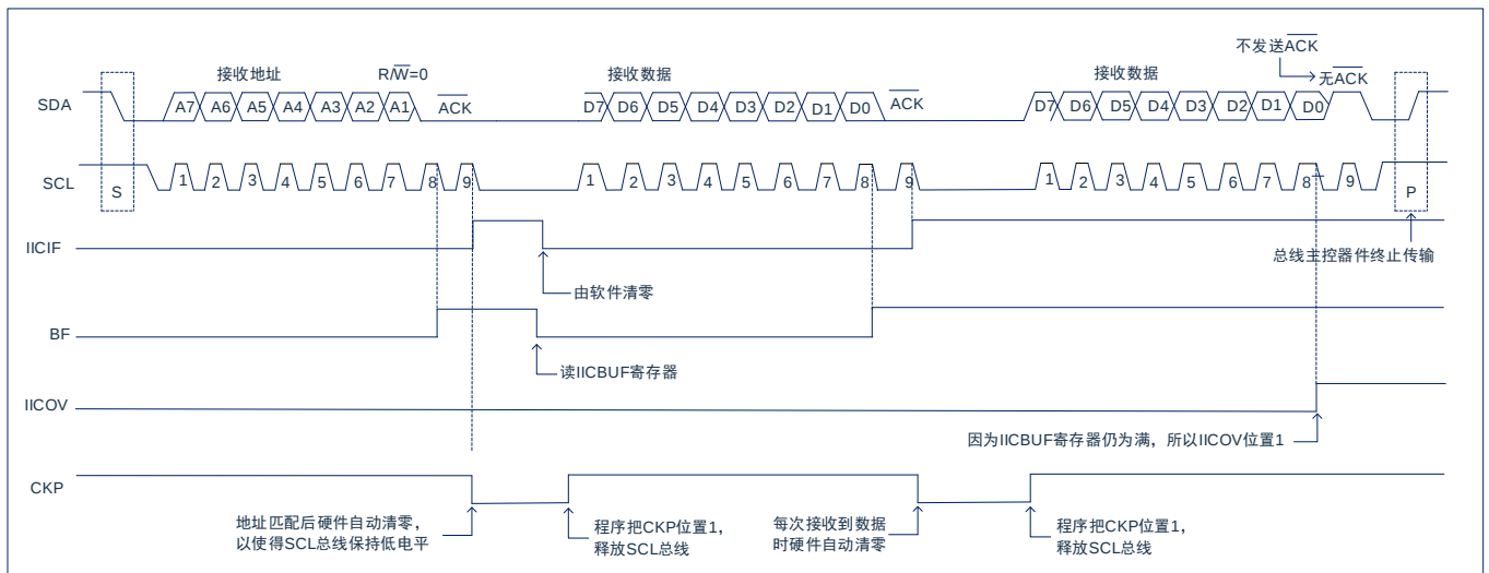
图 18-12: I²C™ 从动模式接收时序
