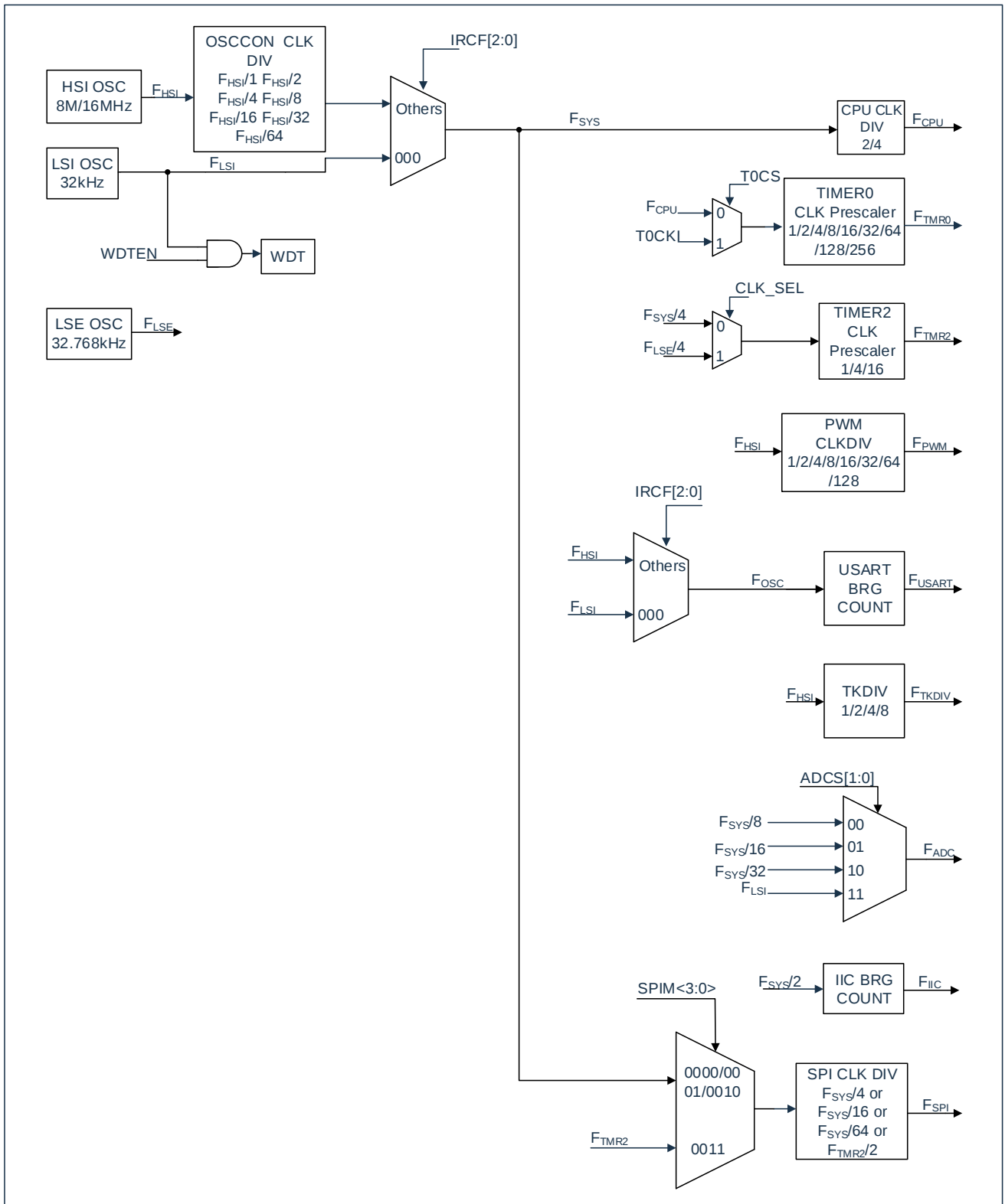
图 3-2: 时钟框图
