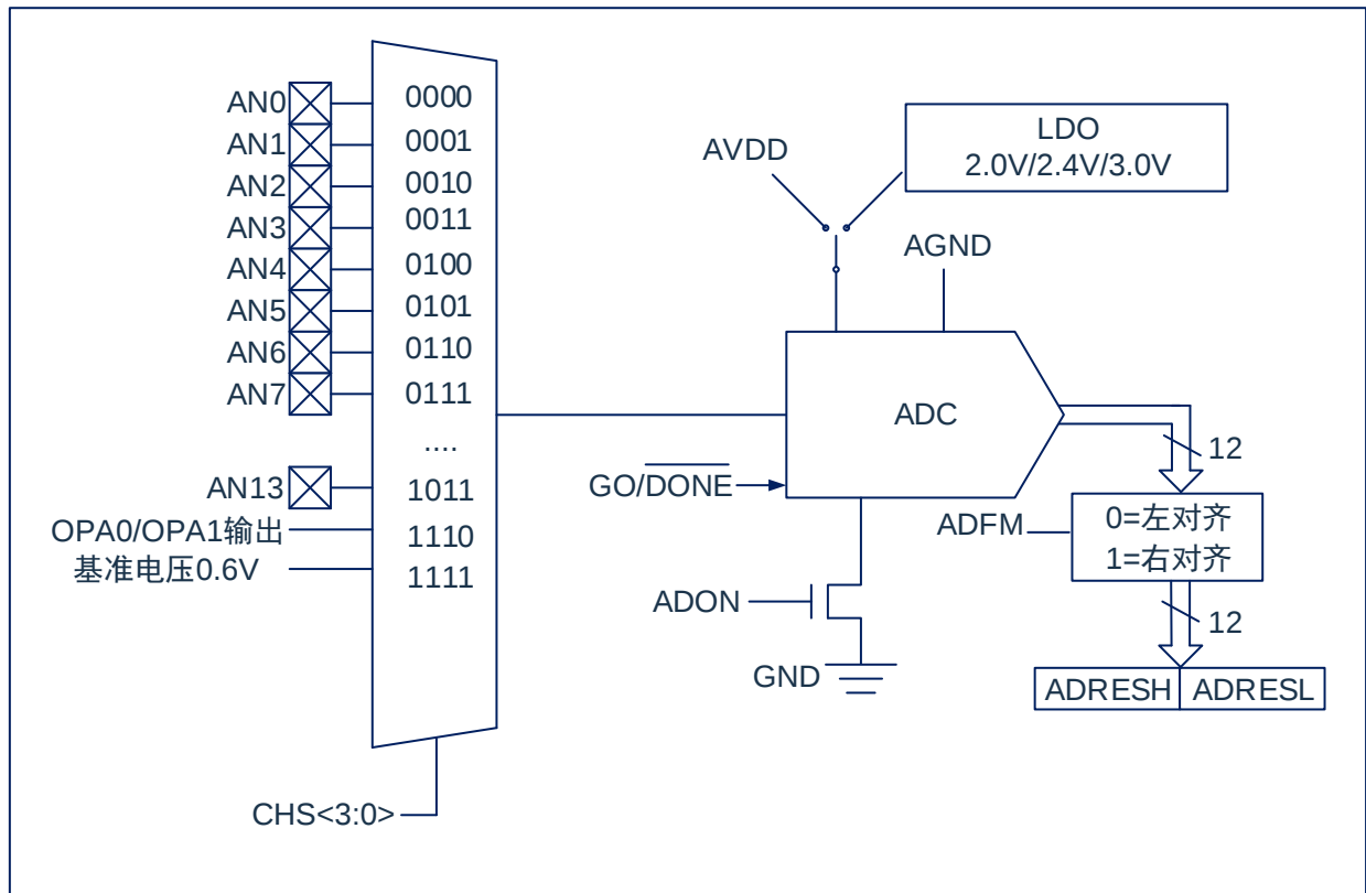
图 10-1: ADC 框图
