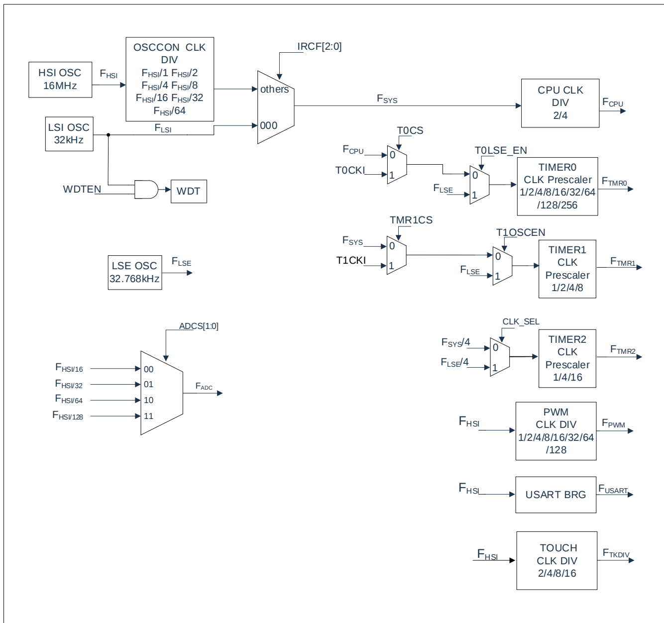
图 3-3: 时钟框图
