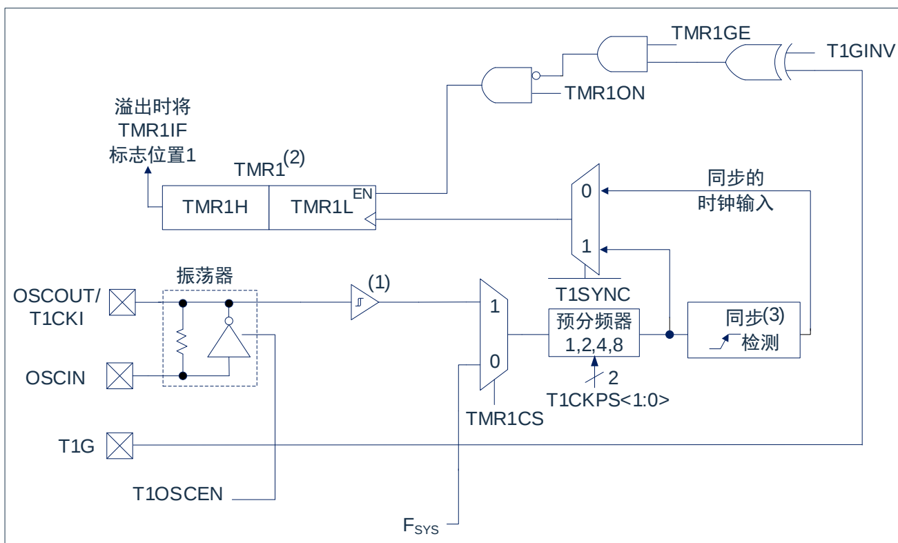
图9-1: TIMER1结构图
