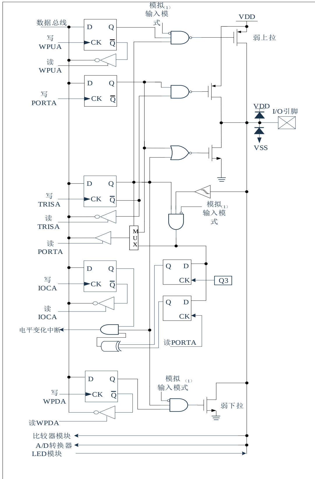
图 6-1: PORTA I/O 口结构图
