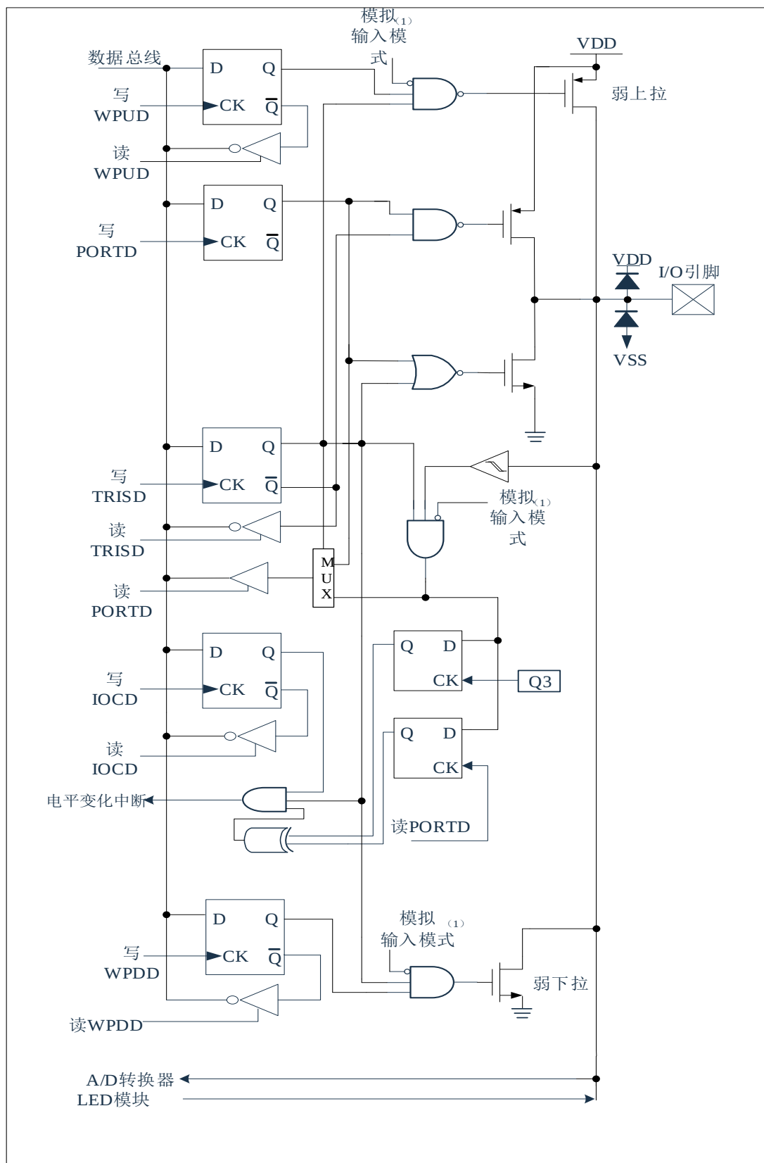
图 6-4: PORTD I/O 口结构图
