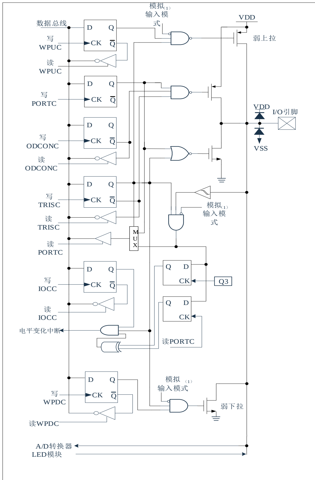
图 6-3: PORTC I/O 口结构图
