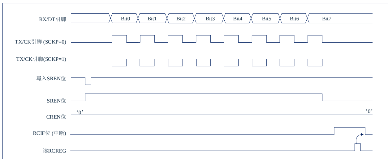
图 12-8：同步接收（主控模式，SREN）
