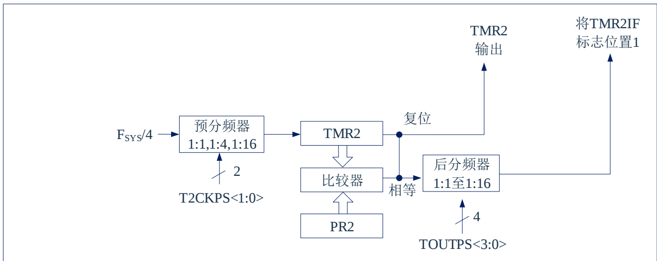
图 10-1: TIMER2 框图
