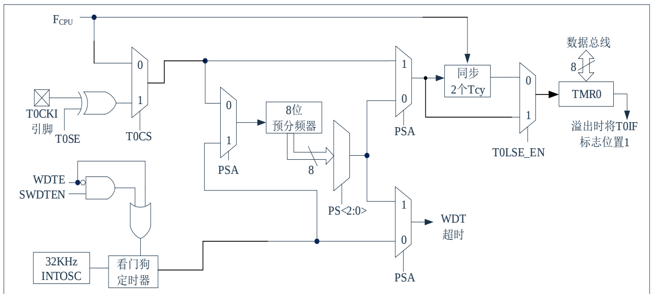
图 8-1: TIMER0/WDT 结构图
