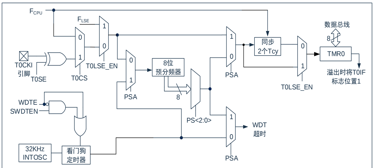
图 8-1: TIMER0/WDT 结构图
