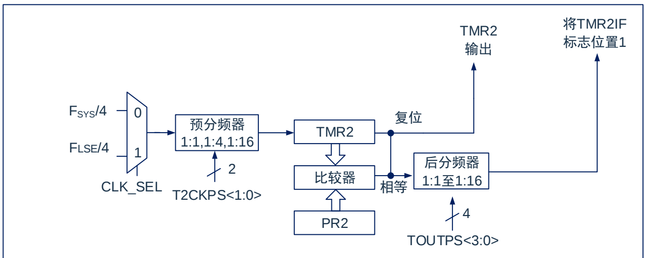
图 10-1: TIMER2 框图
