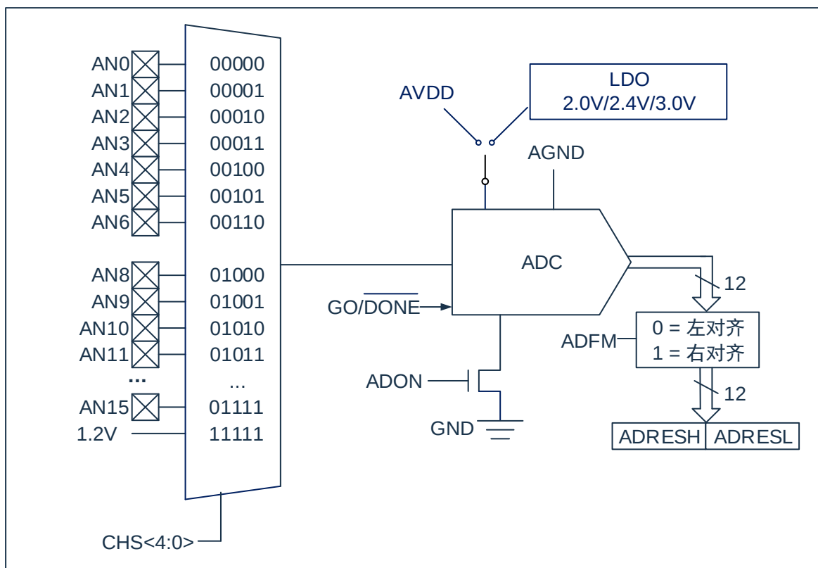
图 12-1: ADC 框图
