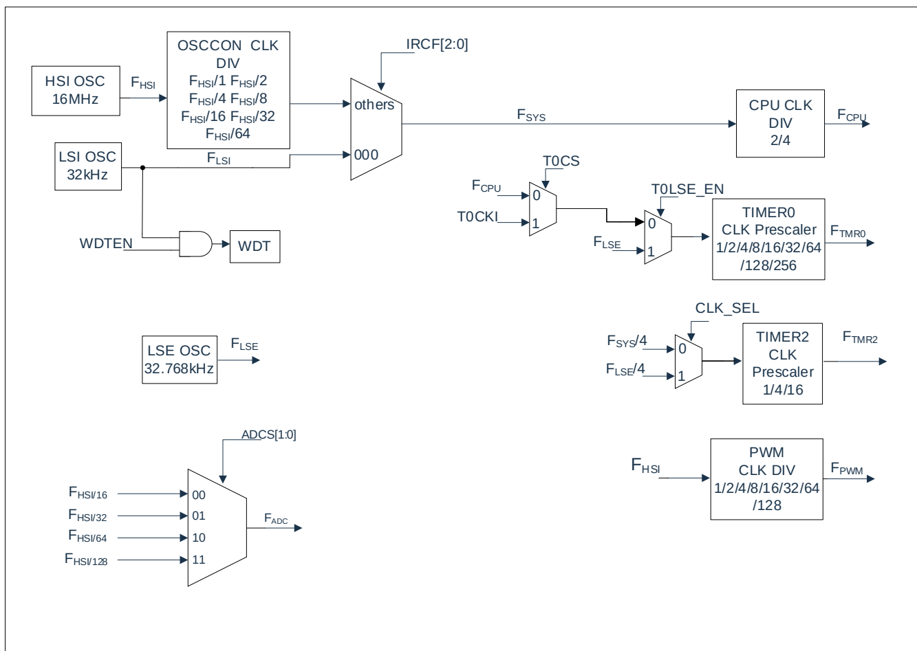
图 3-3: 时钟框图
