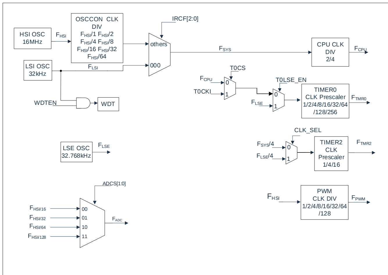
图 3-3: 时钟框图
