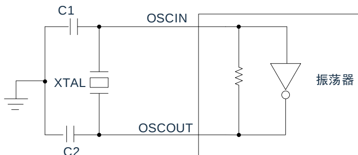
图 13-1： 典型应用电路
