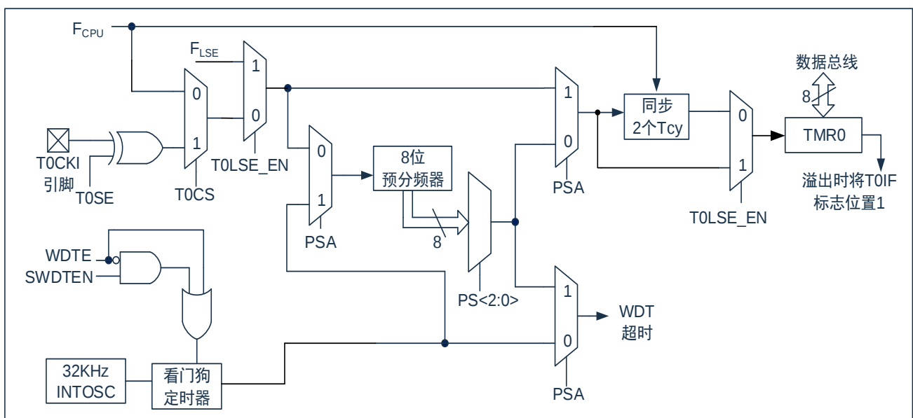
图 8-1: TIMER0/WDT 结构图
