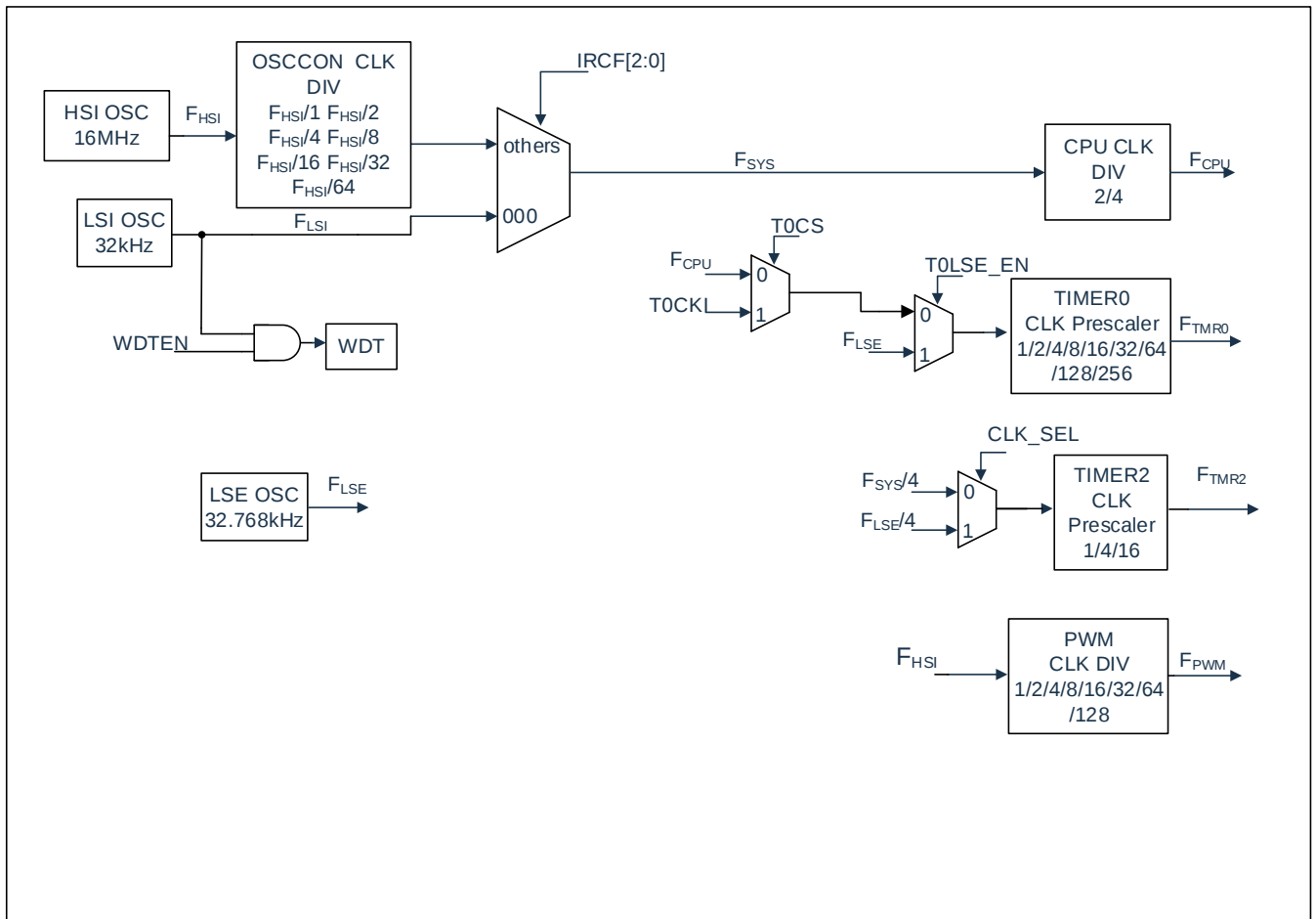
图 3-3: 时钟框图
