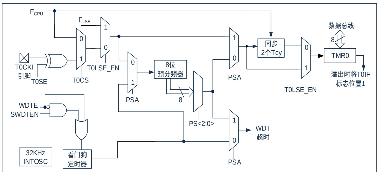
图 8-1: TIMER0/WDT 结构图
