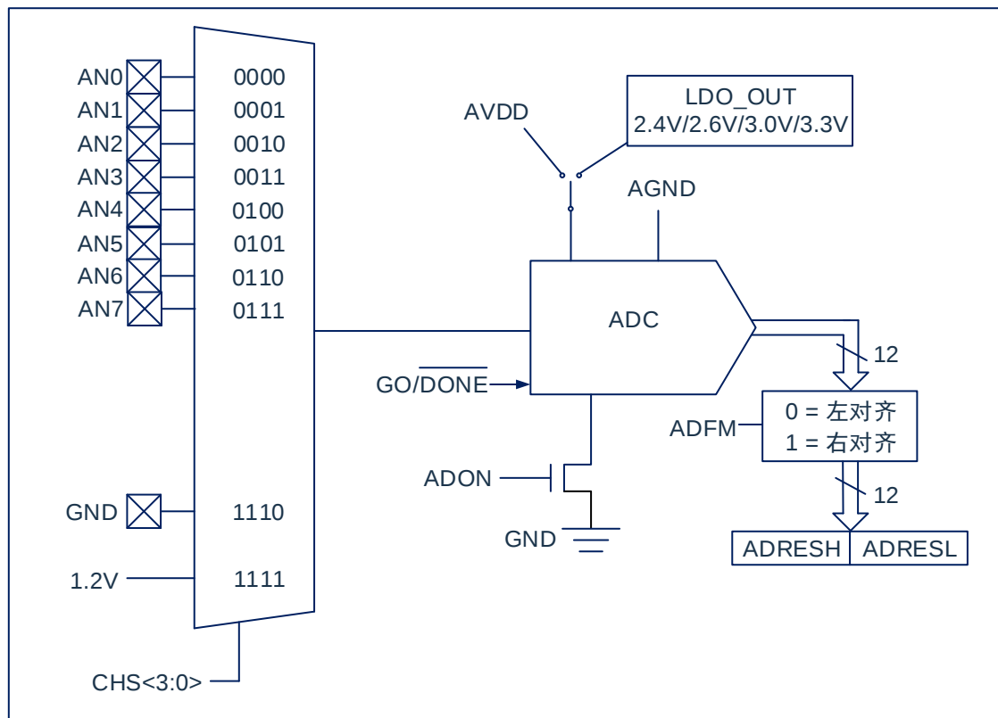
图 10-1：ADC 框图
