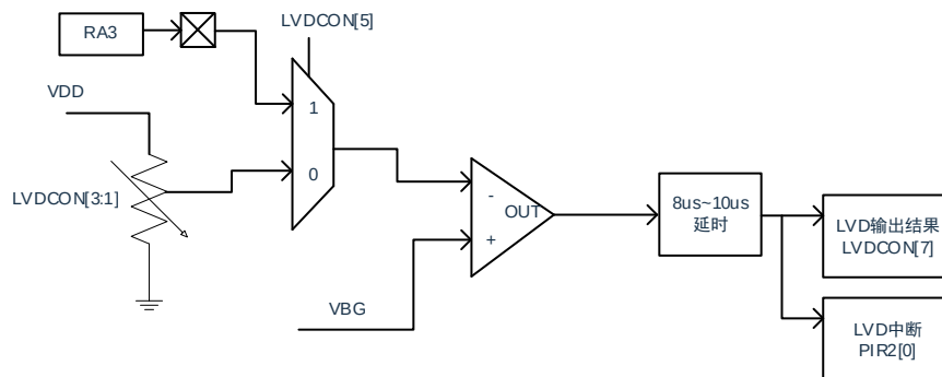
图 16-1: LVD 框图
