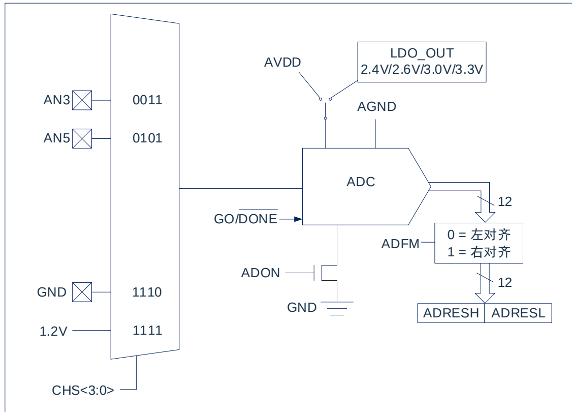
图 10-1: ADC 框图
