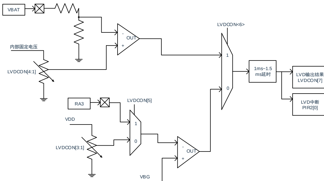
图 15.1: LVD 框图
