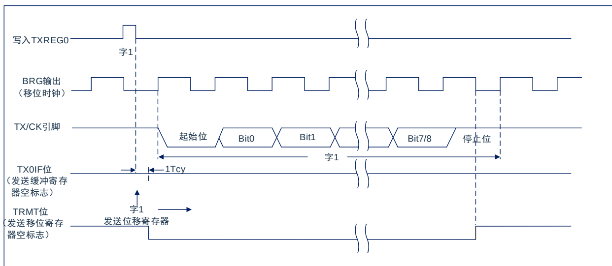
图 12-3: 异步发送
