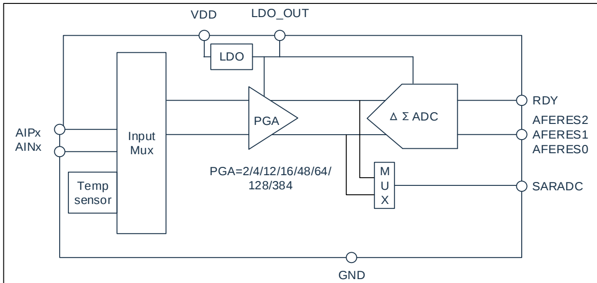
图 11-1: AFE 框图
