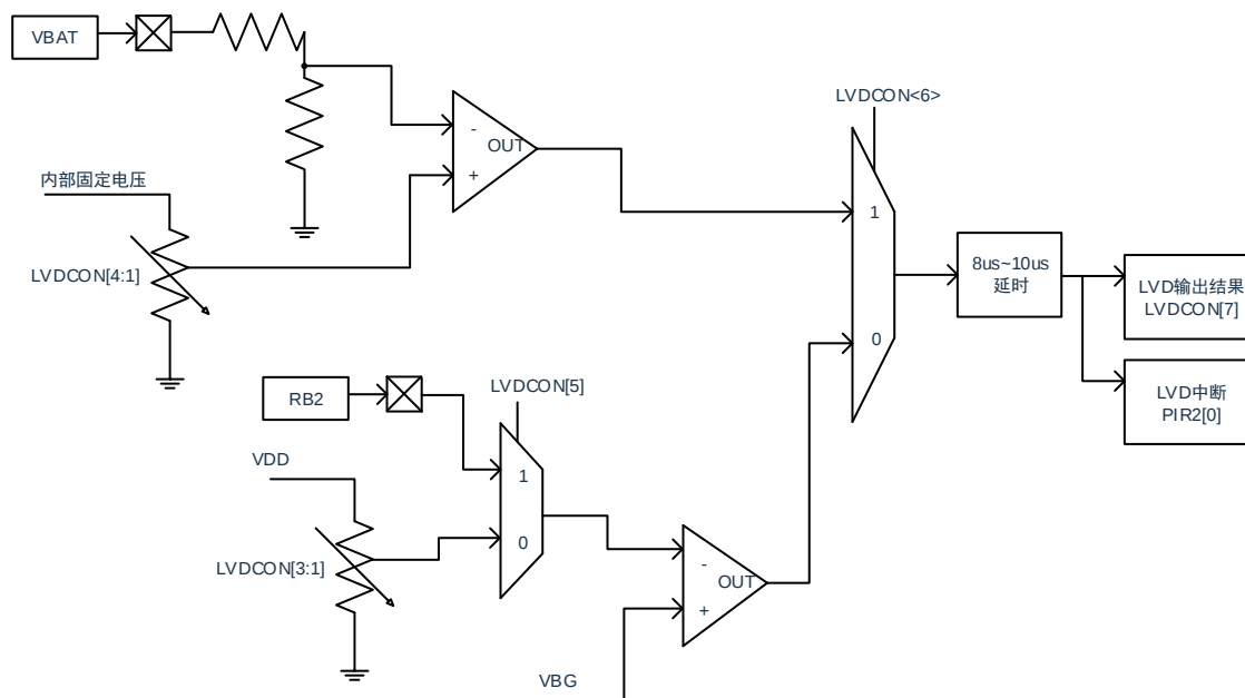
图 16.1: LVD 框图
