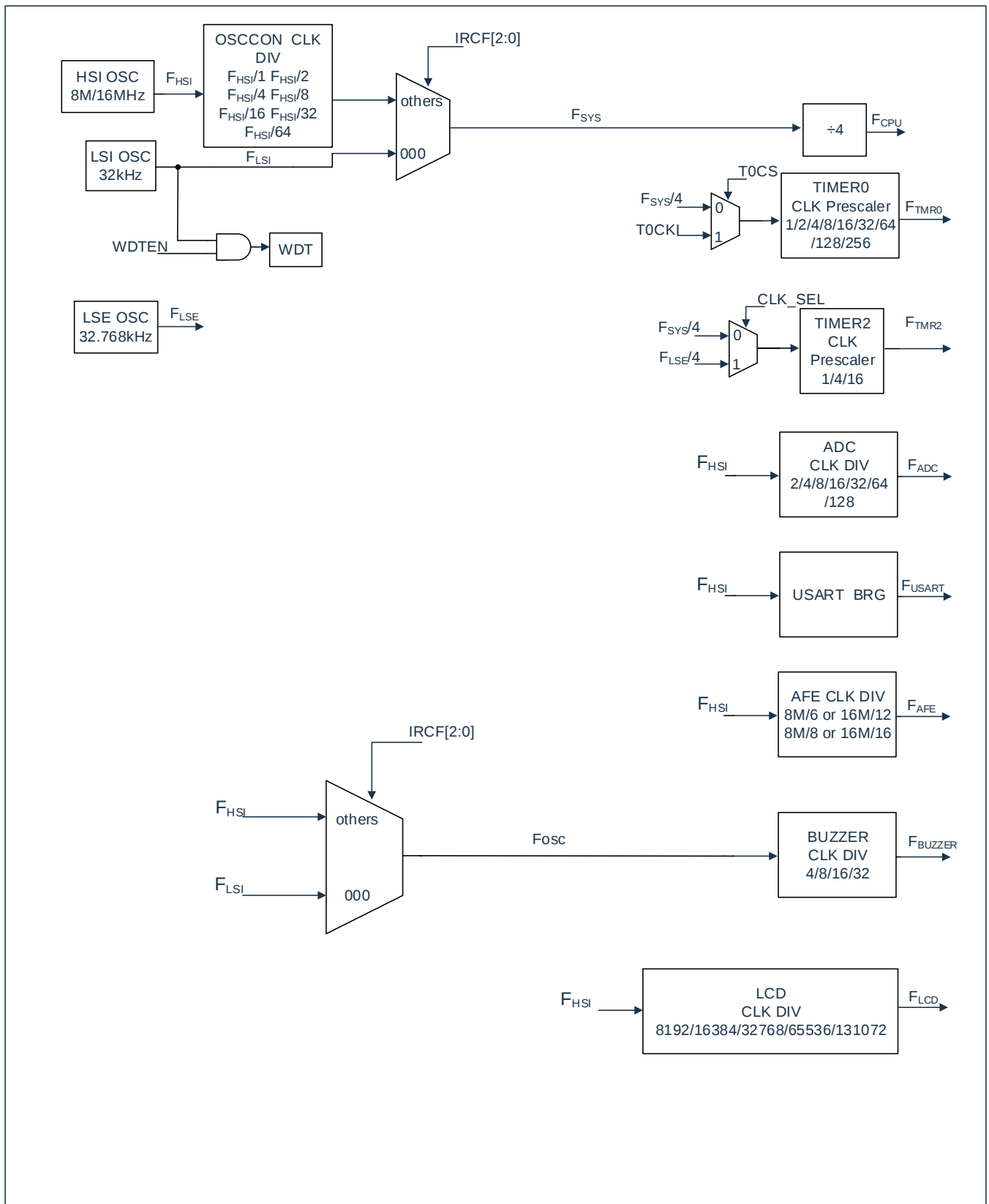
图 3-2: 时钟框图
