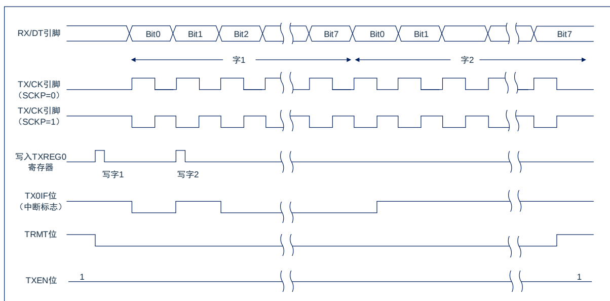
图 13-6：同步发送
