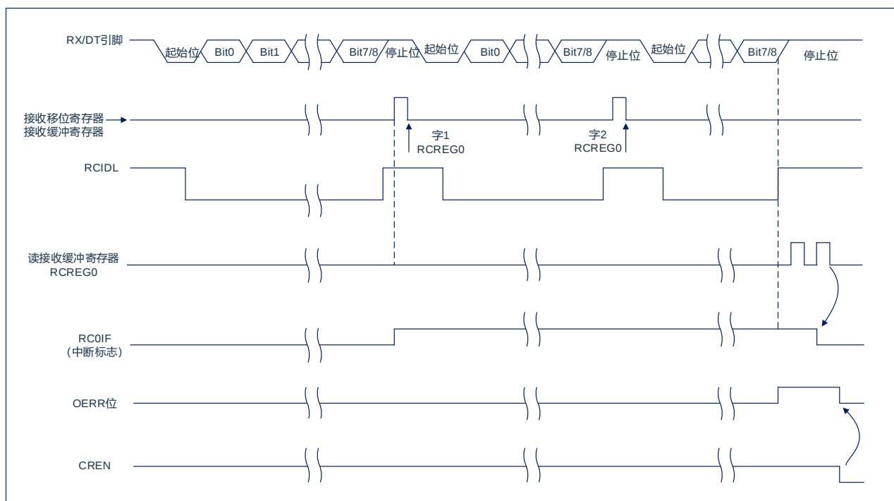
图 13-5: 异步接收
