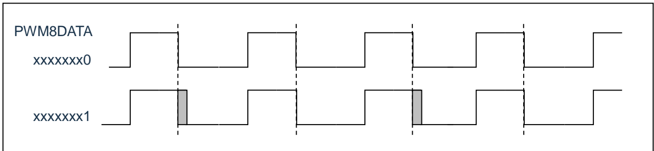
图 15-3: 7+1 模式 8 位 PWM 输出示意图
