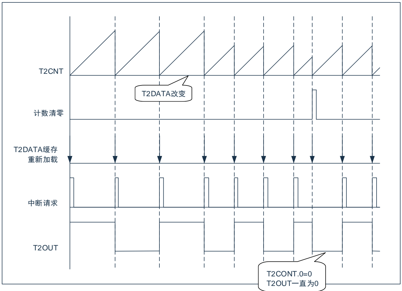
图 10-2: TMR2 时序图
