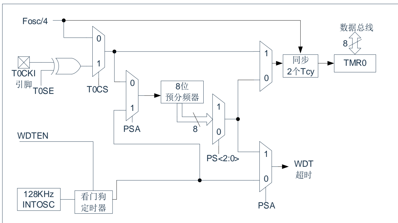
图 8-1: TMR0/WDT 结构图
