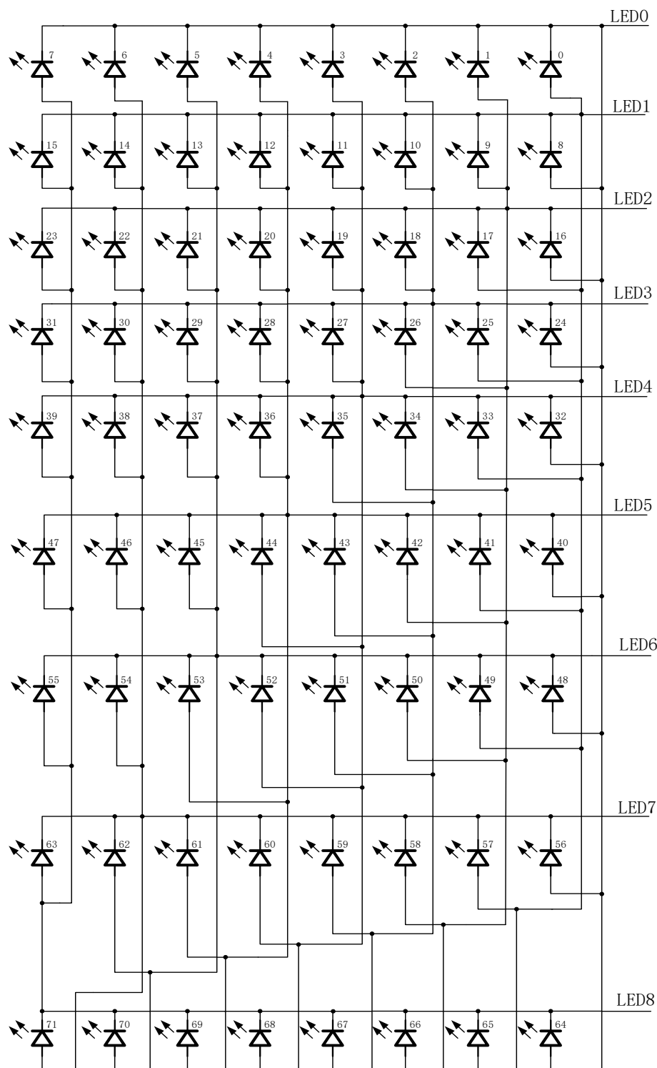
LED9*8点阵图
