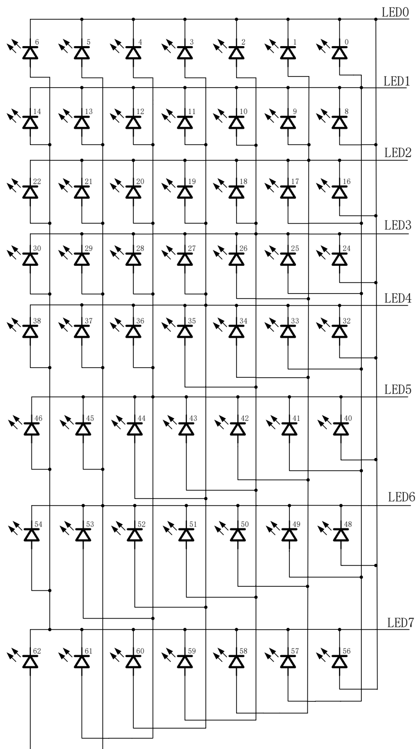
LED8*7点阵图
