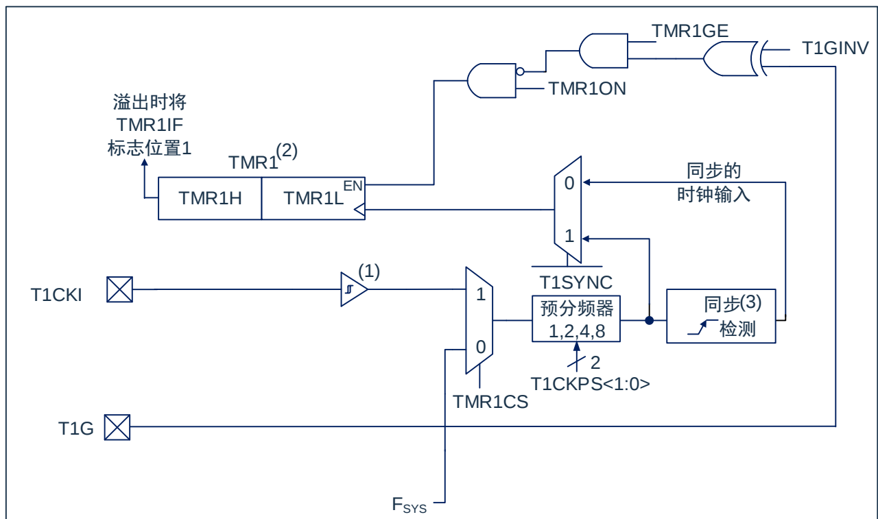
图9-1: TIMER1结构图
