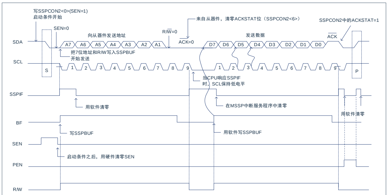
图16-9: I 2 C™主控模式发送时序
