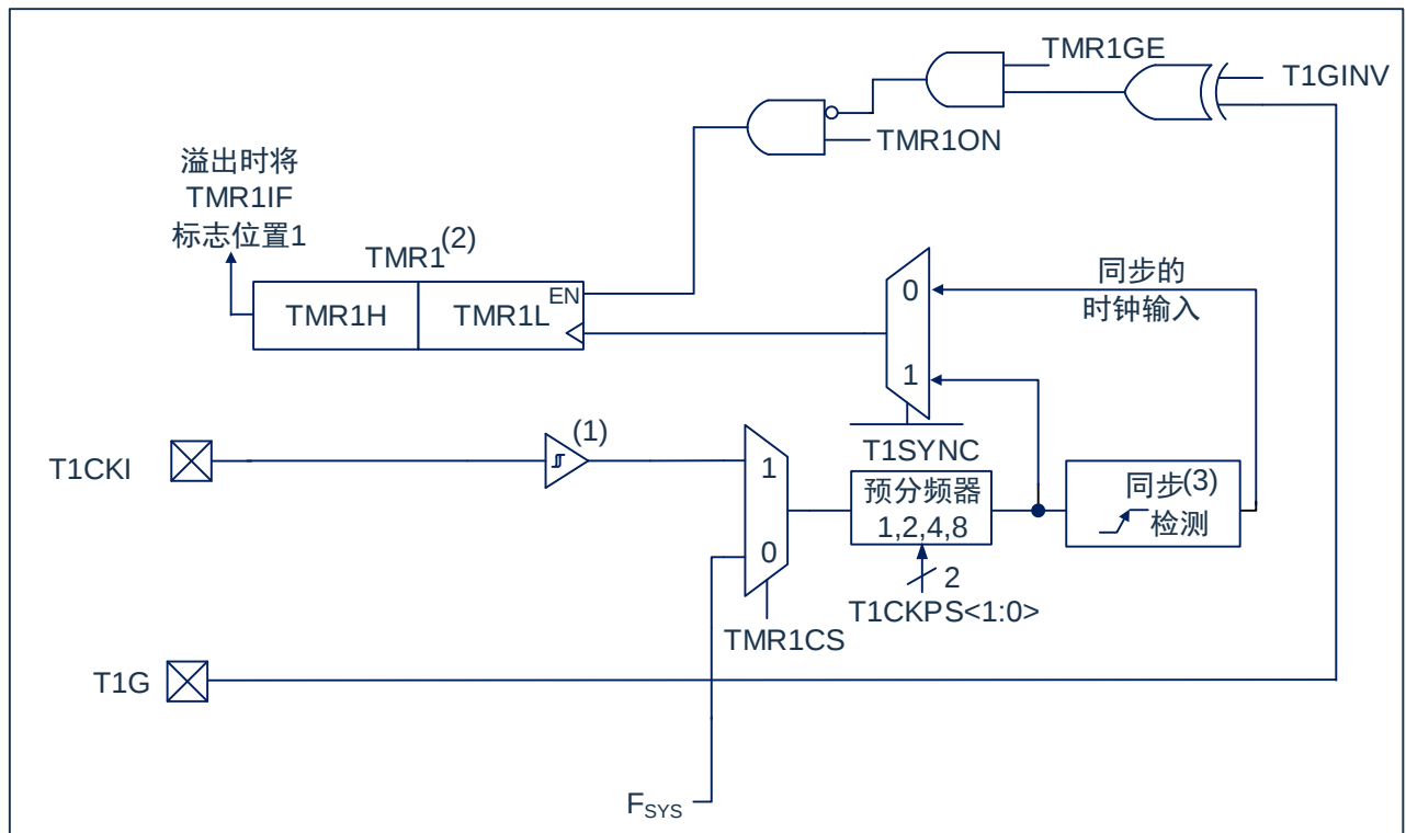
图9-1: TIMER1结构图
