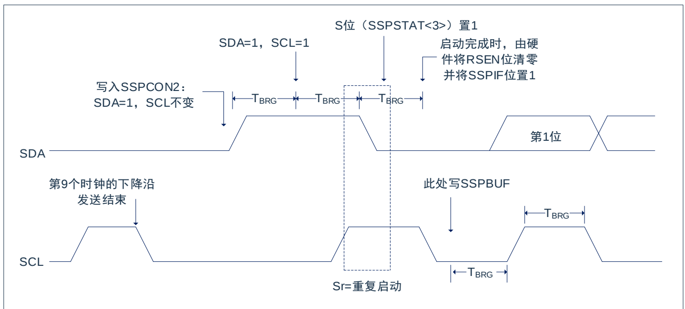
图16-12：重复启动条件时序波形
