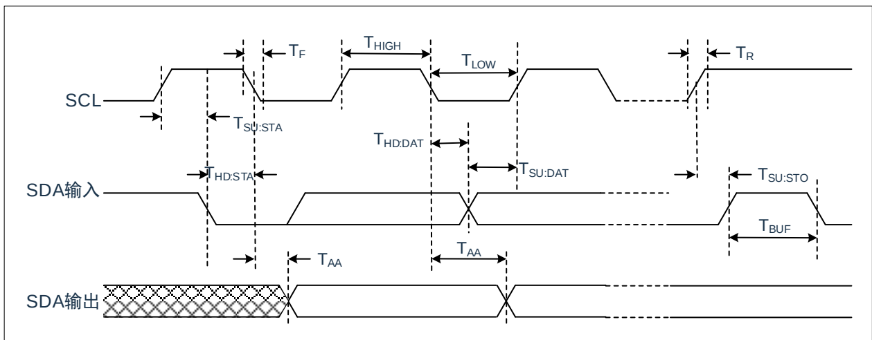
图 6-2: I²C™ 总线数据时序
