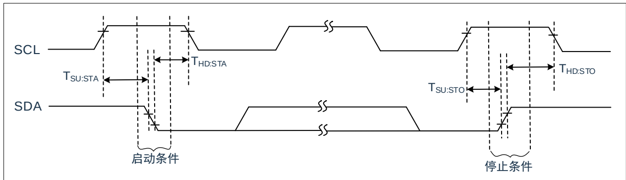
图 6-1: I²C™ 总线启动/停止位时序
