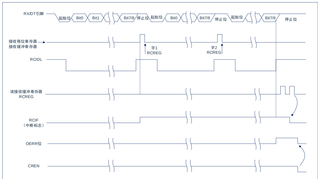
图 14-5: 异步接收
