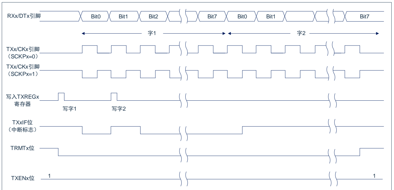
图 14-6: 同步发送
