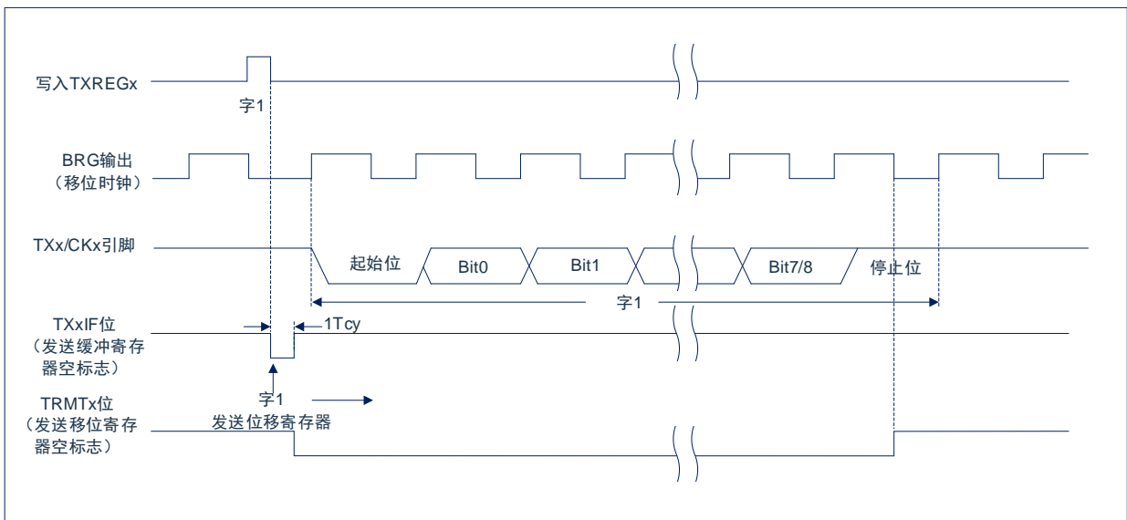
图 14-3: 异步发送
