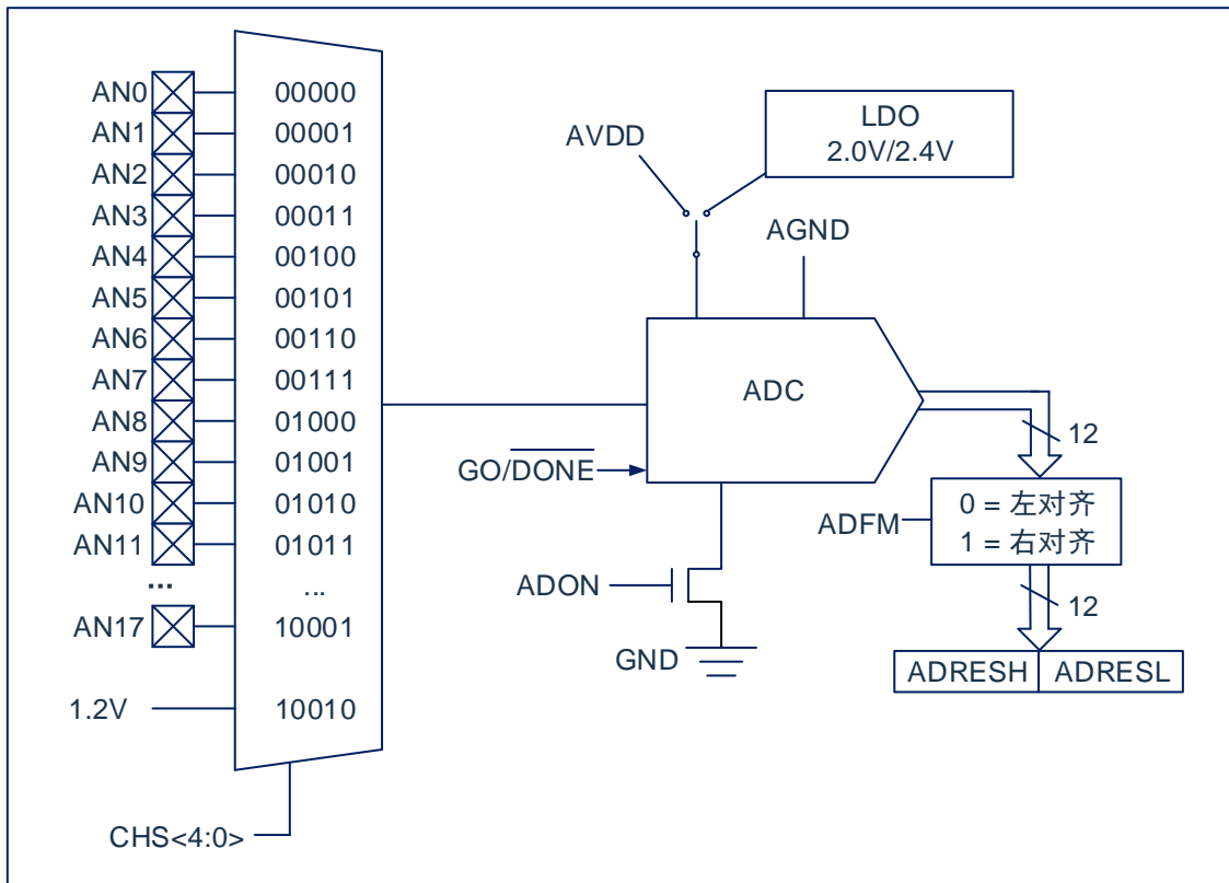
图 11-1: ADC 框图
