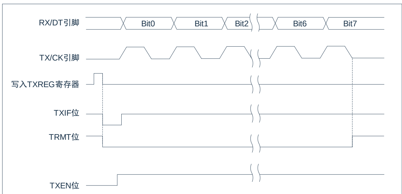
图 15-6: 同步发送
