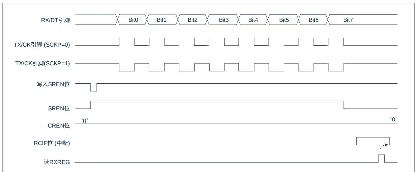
图 15-15 同步接收时序图（主控模式，SREN）
