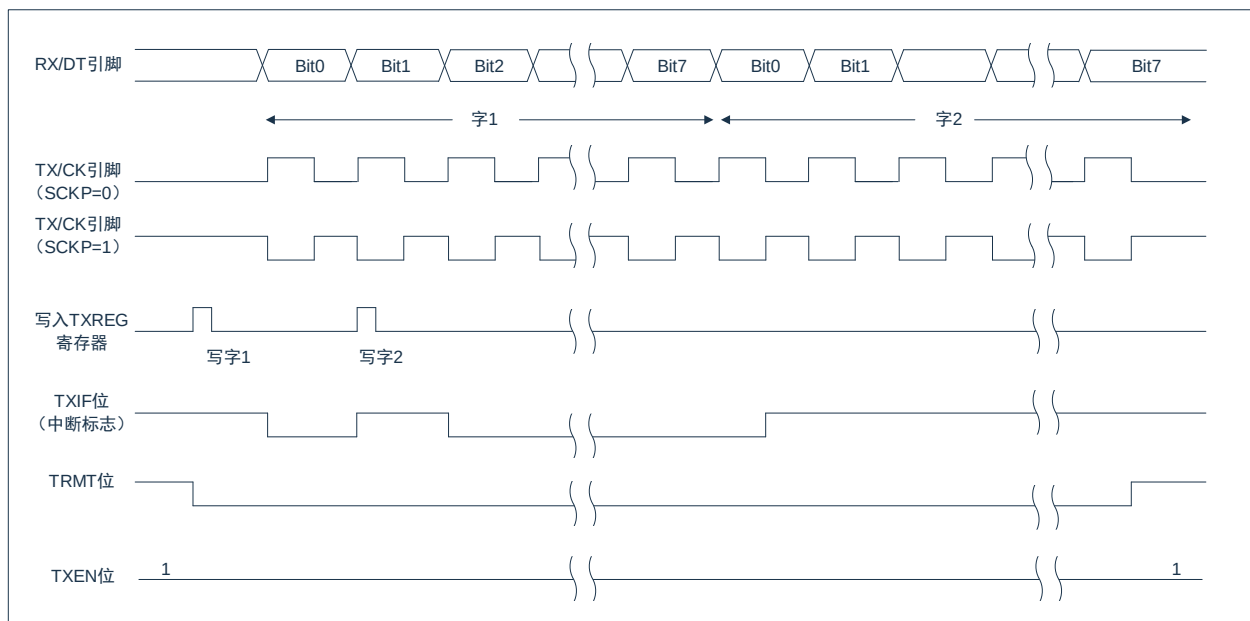
图 15-6: 同步发送
