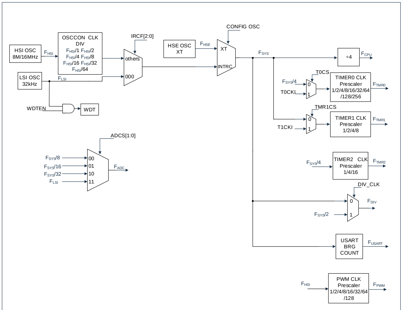
图 3-2: 时钟框图
