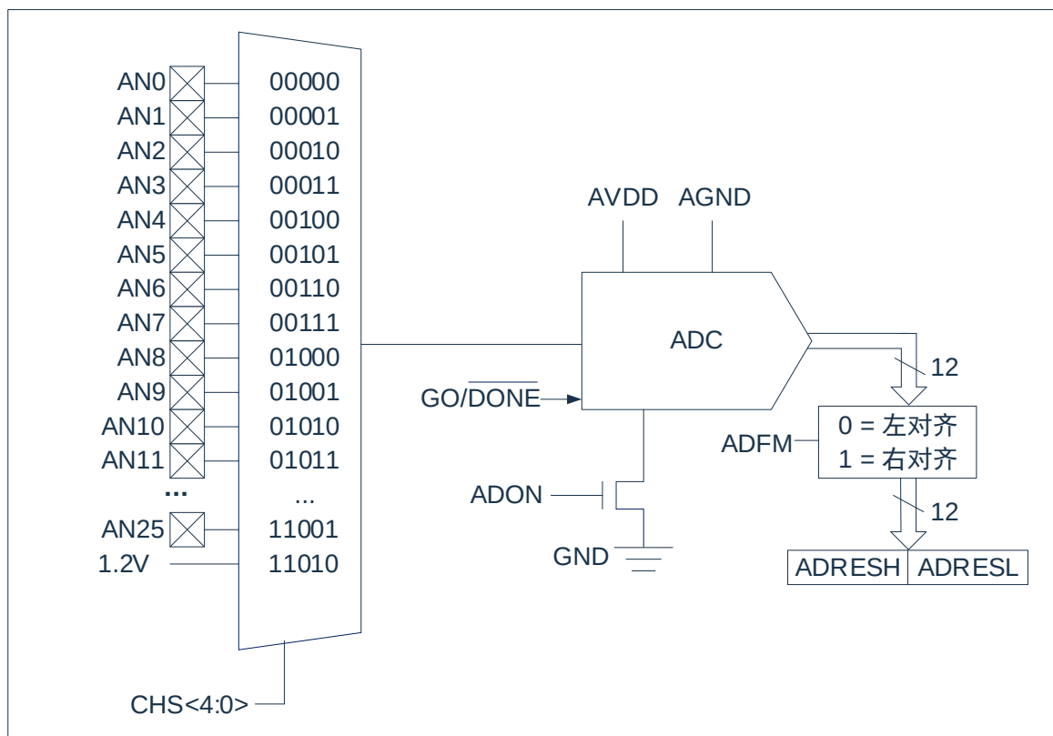
图 11-1: ADC 框图
