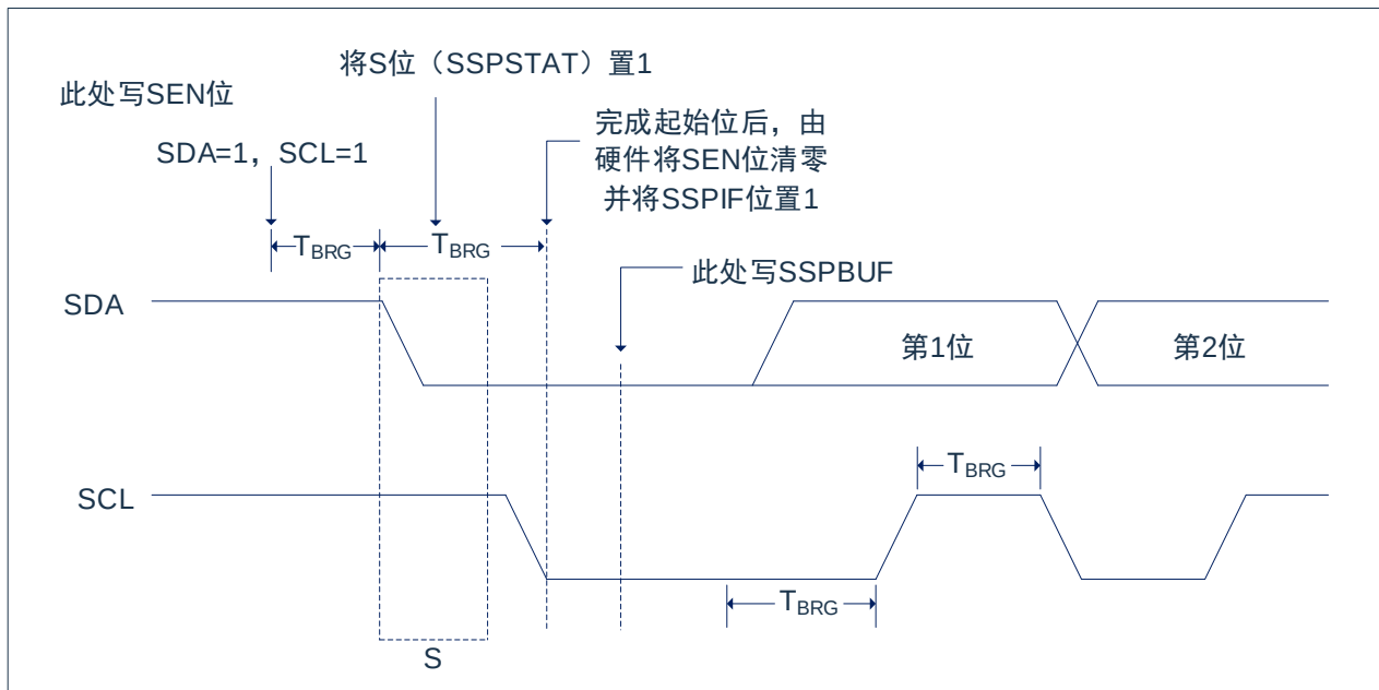
图15-11：第一个启动位时序
