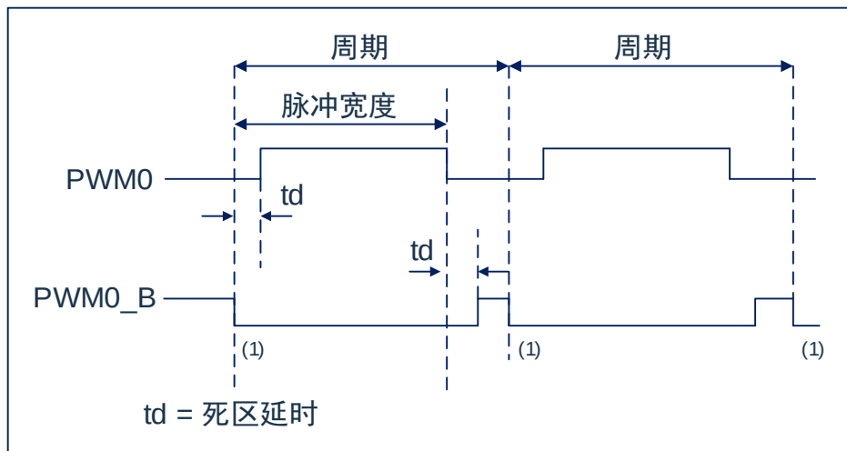
图18-1：PWM死区延时输出示例
