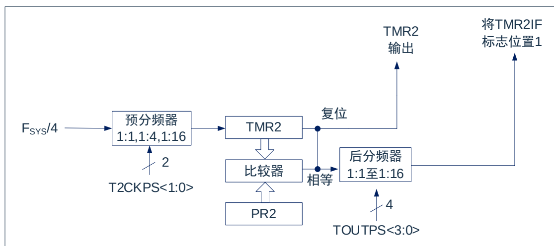
图 10-1: TIMER2 框图
