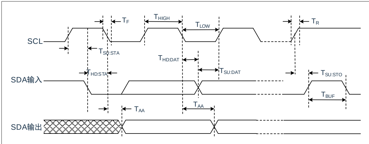
图 20-2: I 2 C™ 总线数据时序
