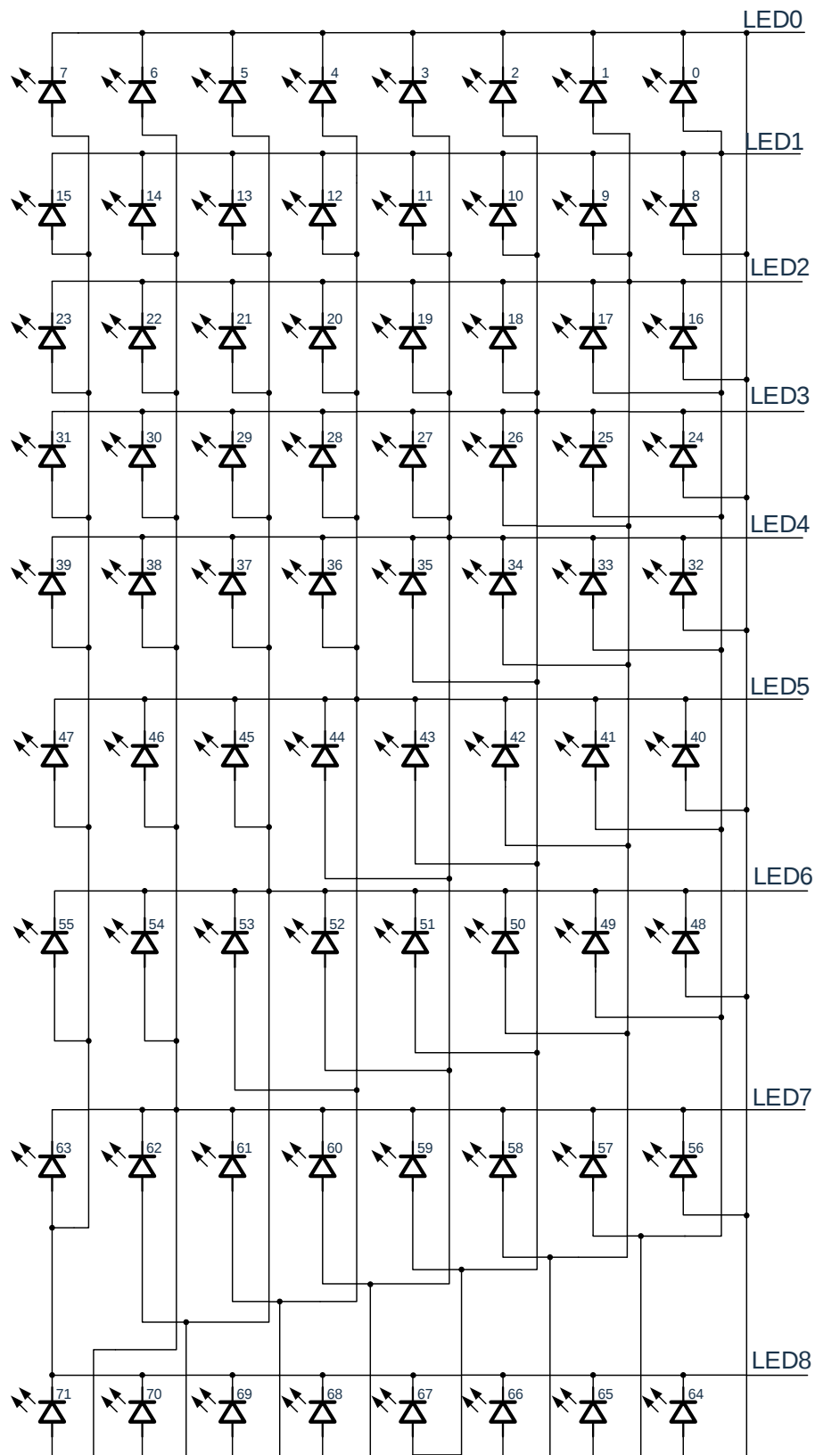
LED8*9点矩阵对应像素点
