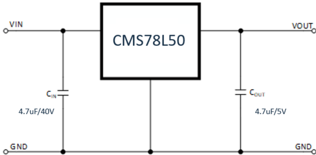
图 8-1: CMS78L50 典型应用
