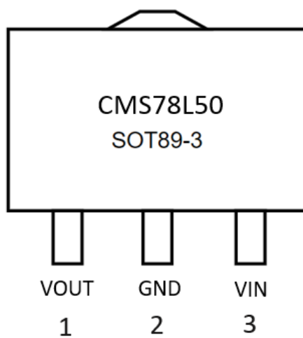
图 2-2: SOT89-3 引脚示意图
