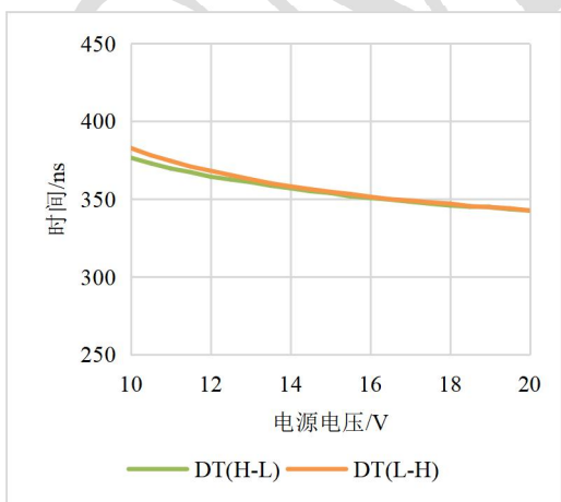
图 7-11：死区时间随电源电压变化曲线
