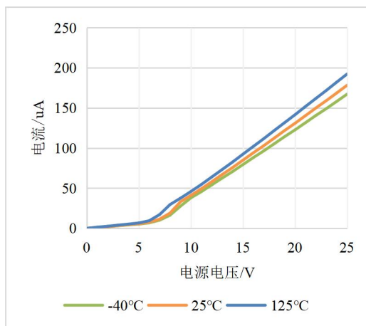
图 7-1: VCC 静态电流随电源电压变化曲线
