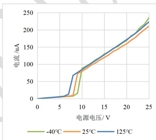
图 7-4: VBS 动态电流随电源电压变化曲线
