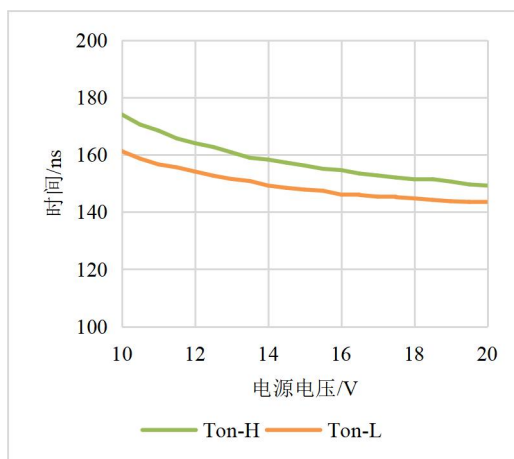
图 7-9：输出开启传输时间随电源电压变化曲线
