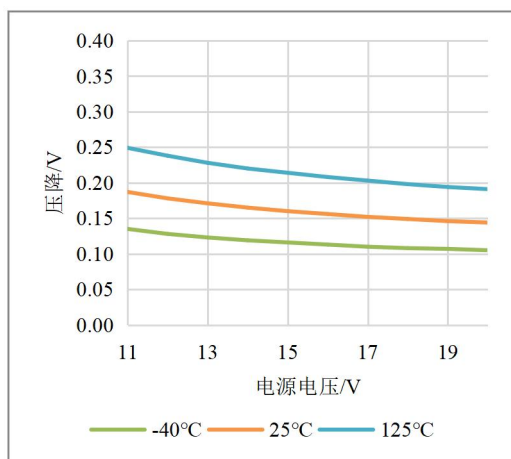
图 7-6: 低电平输出压降随电源电压变化曲线
