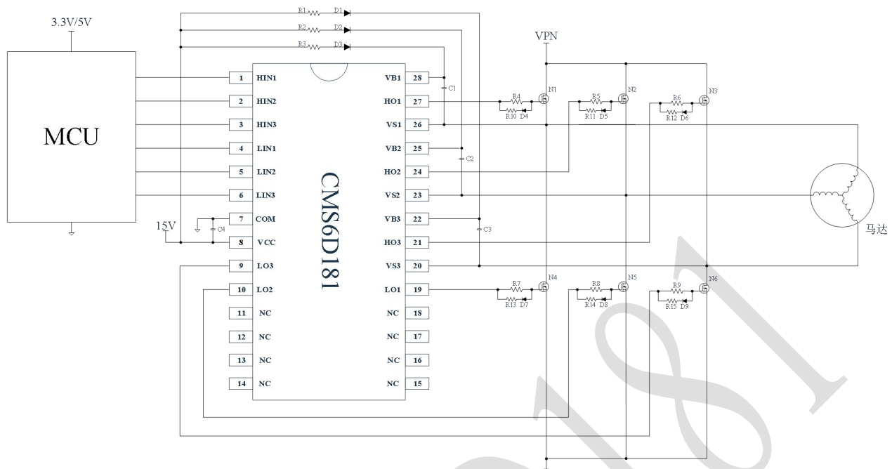
图 8-1: CMS6D181 典型半桥应用
