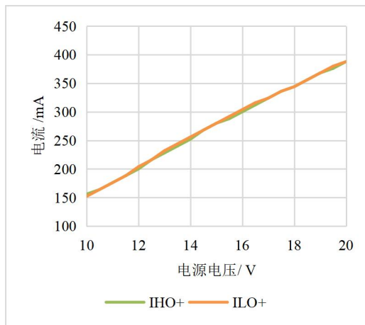
图 7-7：高电平短路脉冲电流随电源电压变化曲线
