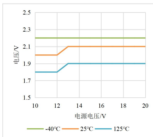
图 7-13: 输入正阈值随电源电压变化曲线
