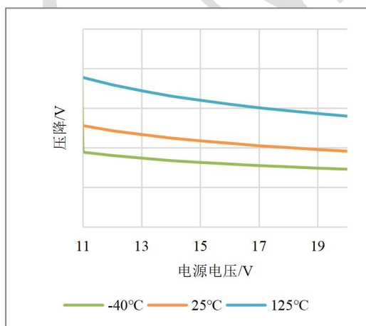
图 7-5: 高电平输出压降随电源电压变化曲线
