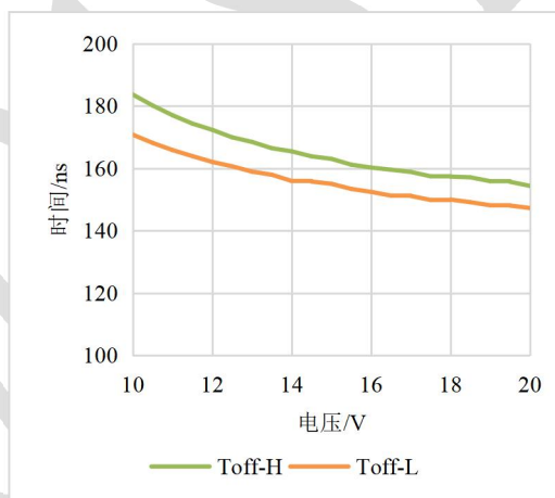
图 7-10：输出关闭传输时间随电源电压曲线
