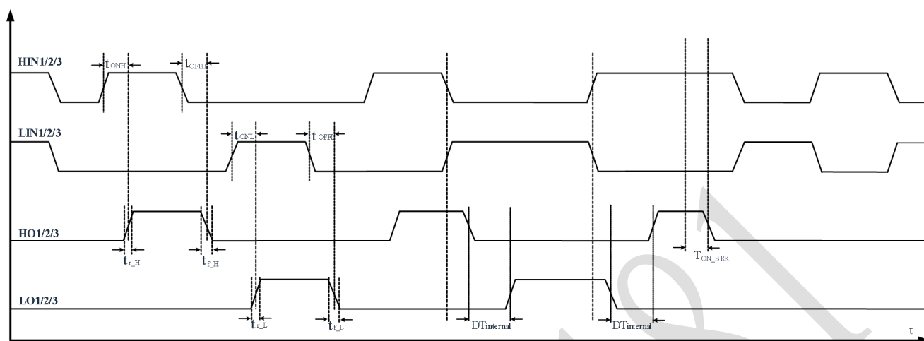
图 10-1：时间参数定义
