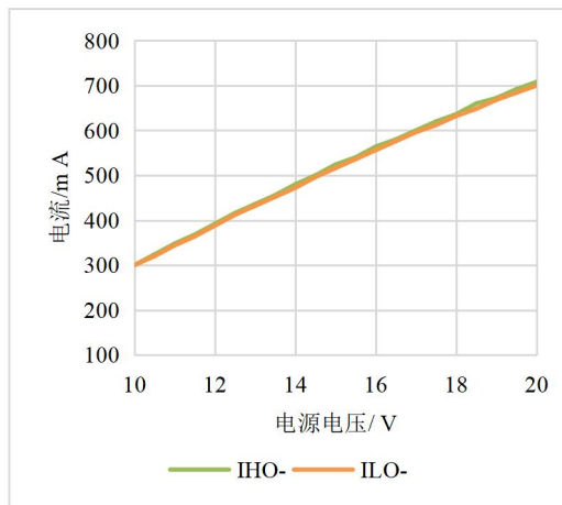
图 7-8：低电平短路脉冲电流随电源电压变化曲线
