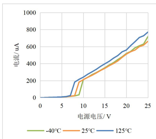
图 7-3: VCC 动态电流随电源电压变化曲线
