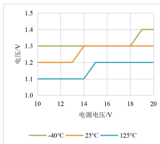
图 7-14: 输入负阈值随电源电压变化曲线
