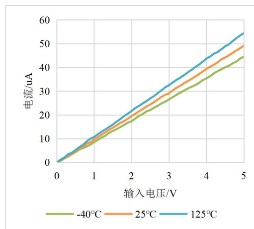
图 7-12：输入电流随输入电压变化曲线
