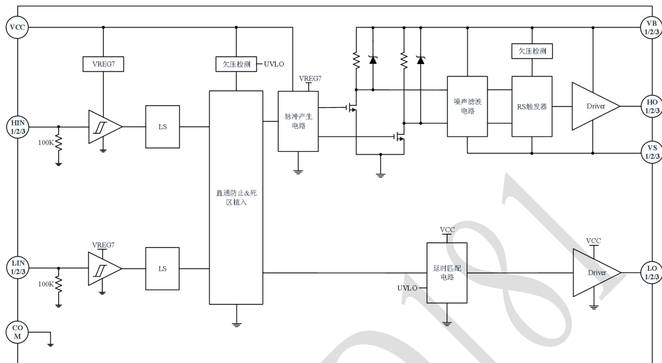
图 3-1: CMS6D181 内部框图
