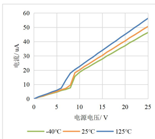
图 7-2: VBS 静态电流随电源电压变化曲线
