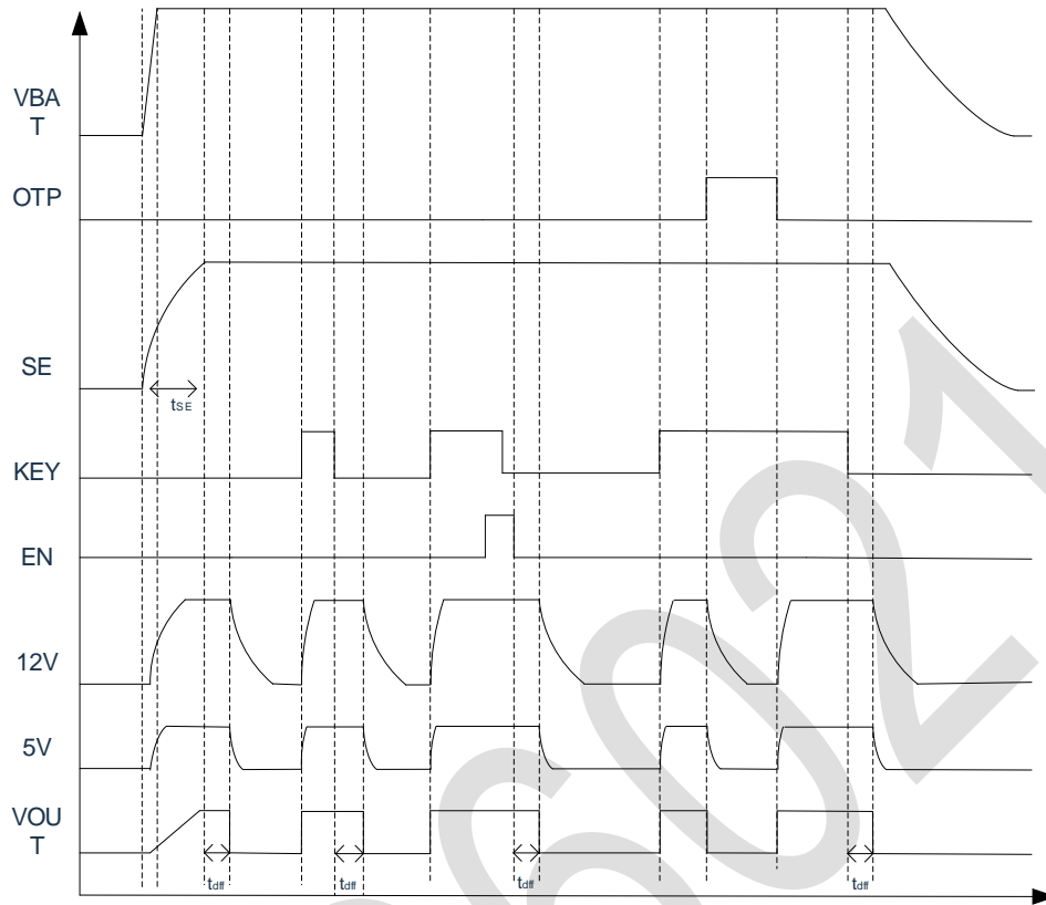
图 3-2: 逻辑时序图
