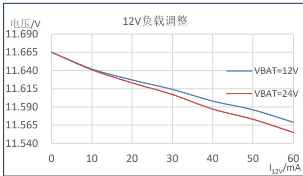
图 9-9: 12V 负载调整
