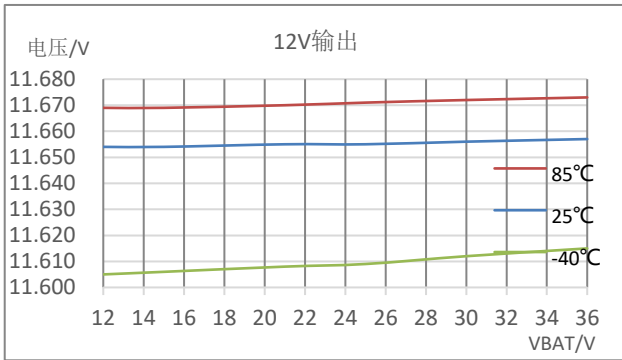
图 9-7: 12V 线性调整 vs VBAT
