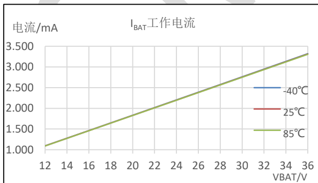
图 9-11: I_{BAT} 工作电流 vs VBAT
