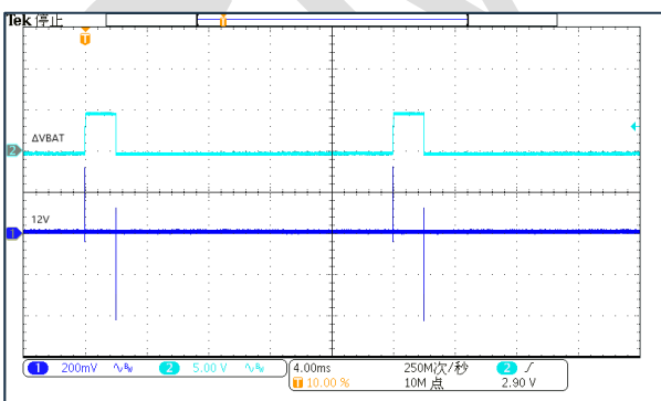
图 9-23: 12V 线性调整
