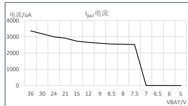
图 9-12: VBAT=VKEY 掉电 I_{BAT} 工作电流
