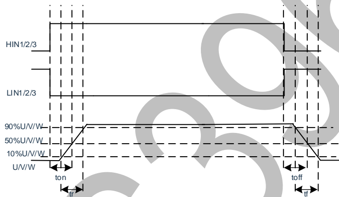
图 8-1 开关参数定义
