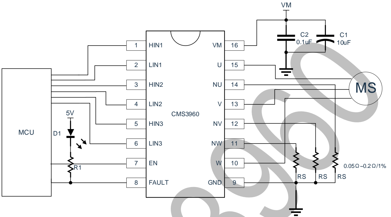
图 10-1: CMS3960 无位置传感器应用电路
