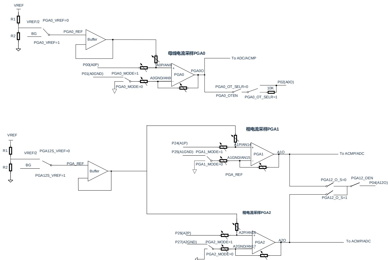
图 18-1: PGA 结构图
