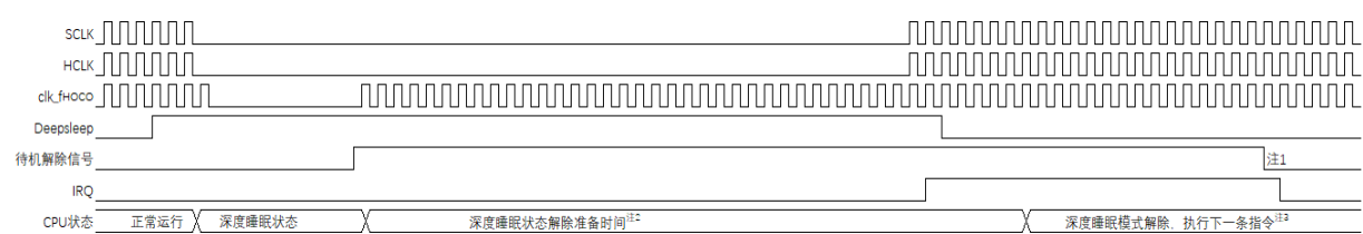
图23-6：通过中断请求解除深度睡眠模式
