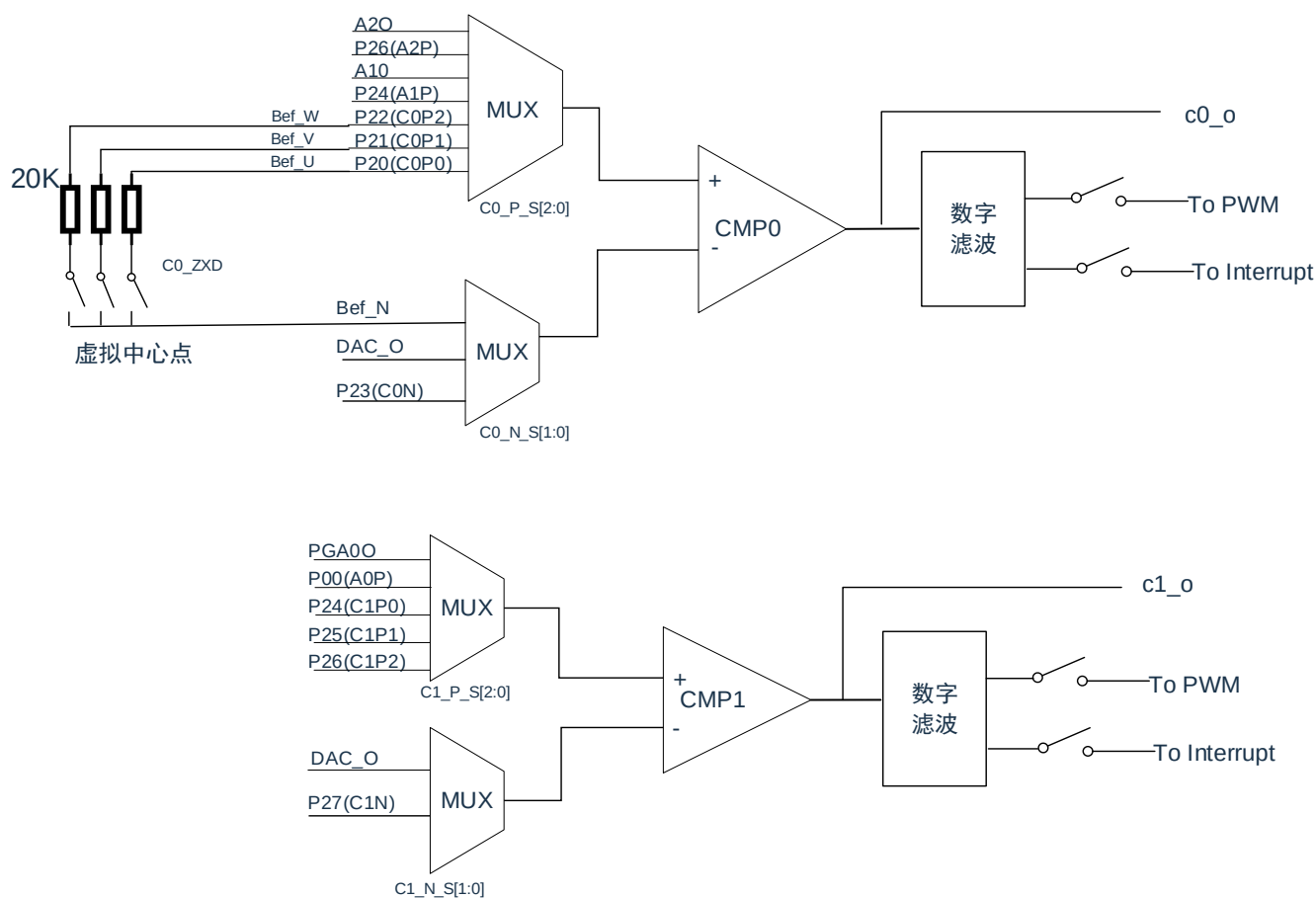
图19-1：比较器结构框图
