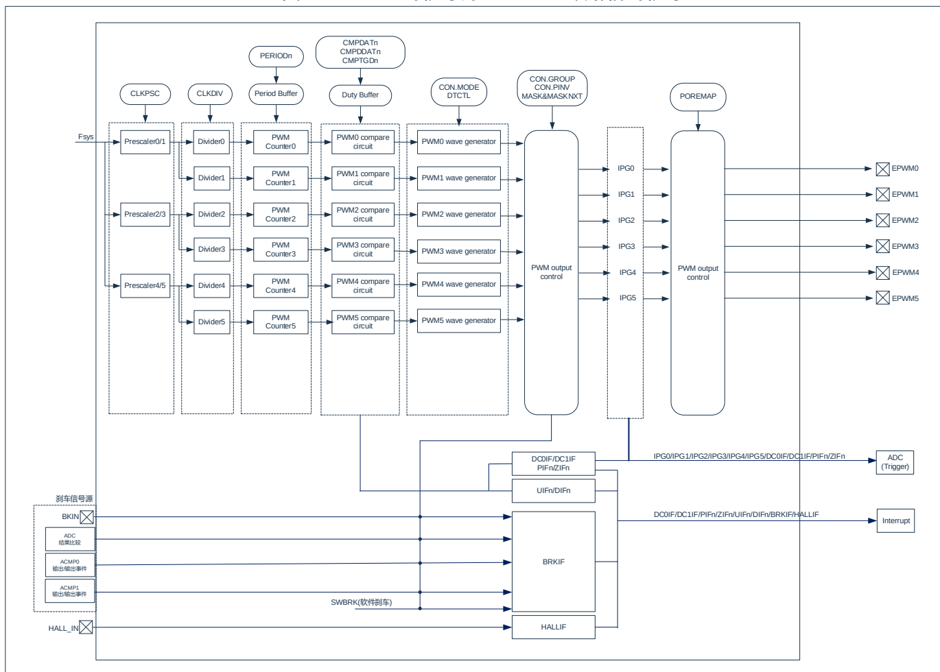
图13-1: IPGn的信号为EPWMn重映射前的信号。
