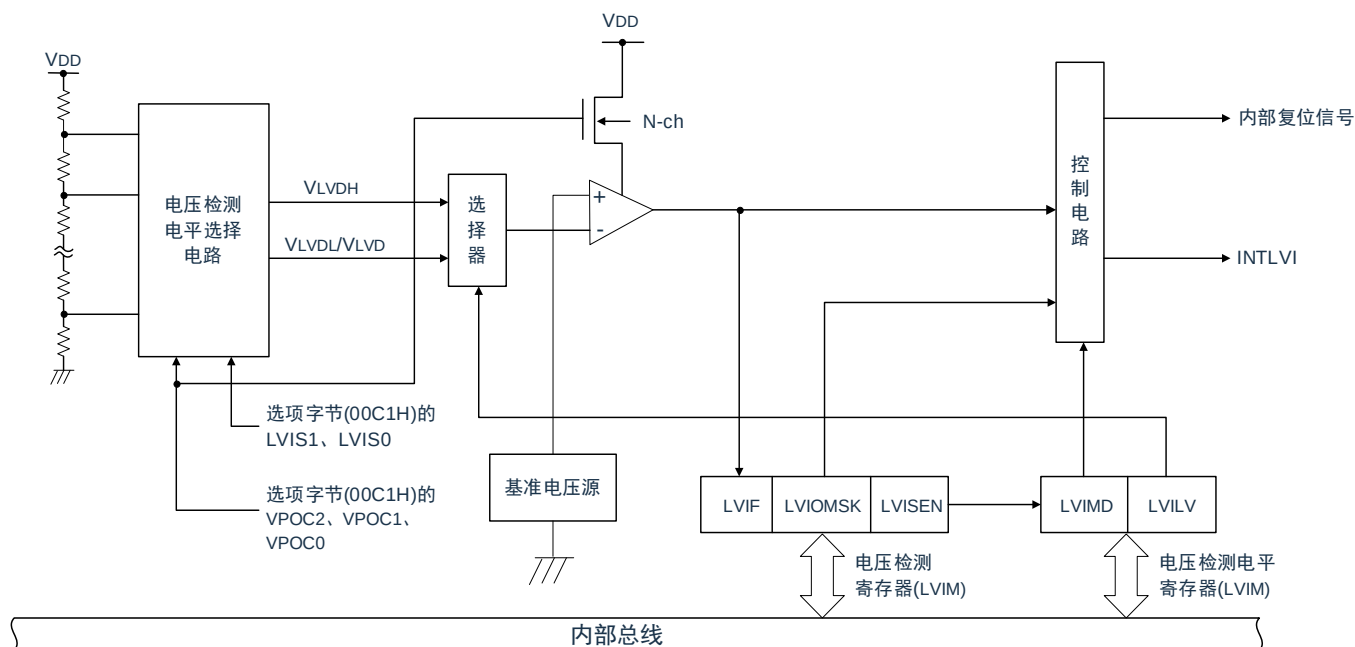
图26-1：电压检测电路的框图
