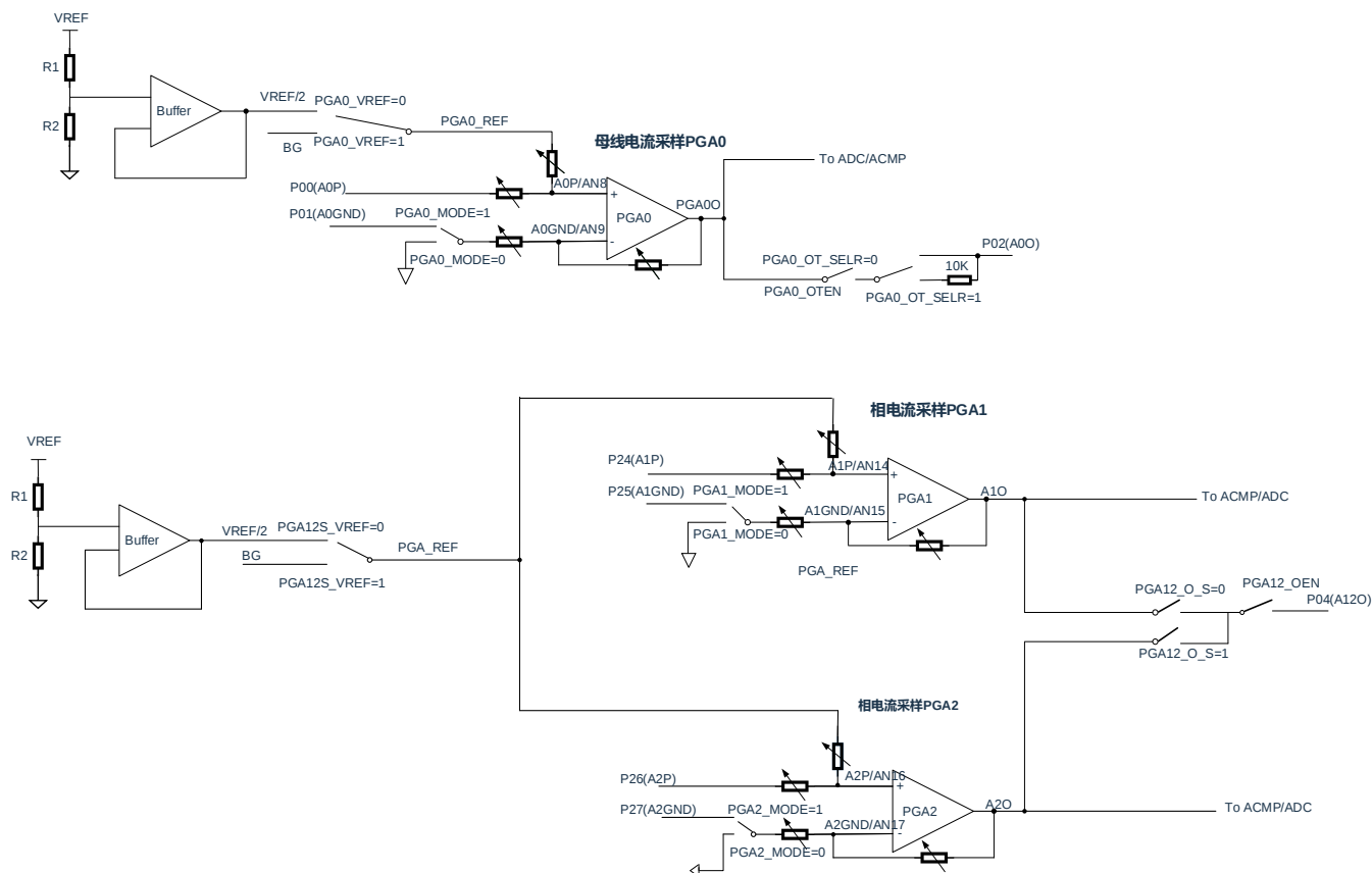
图 18-1: PGA 结构图
