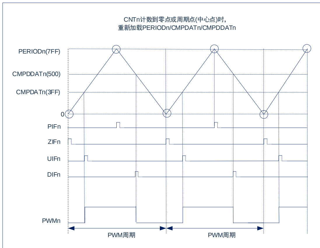
图13-6：中心对齐模式非对称计数波形图
