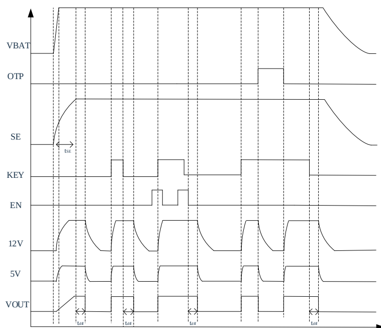
逻辑时序图
