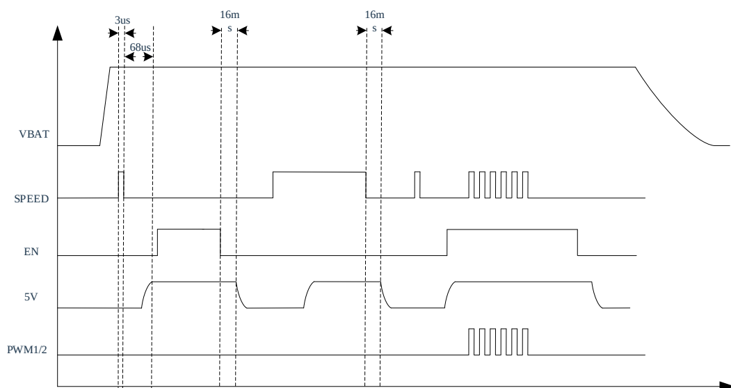
逻辑时序图
