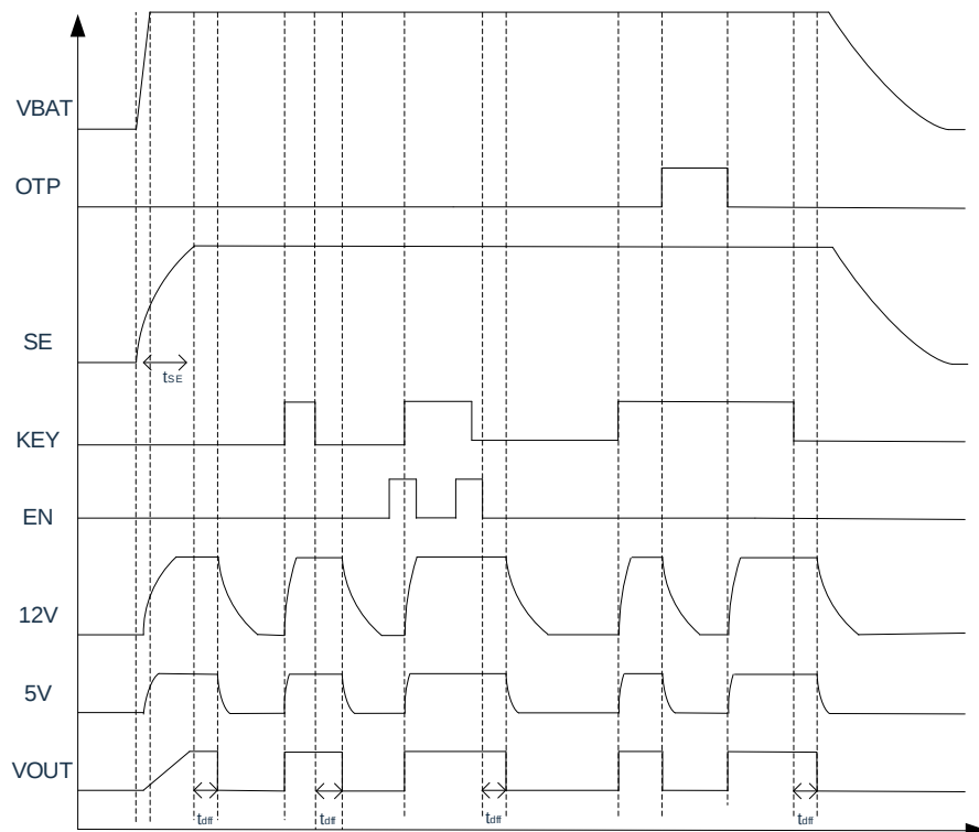
逻辑时序图
