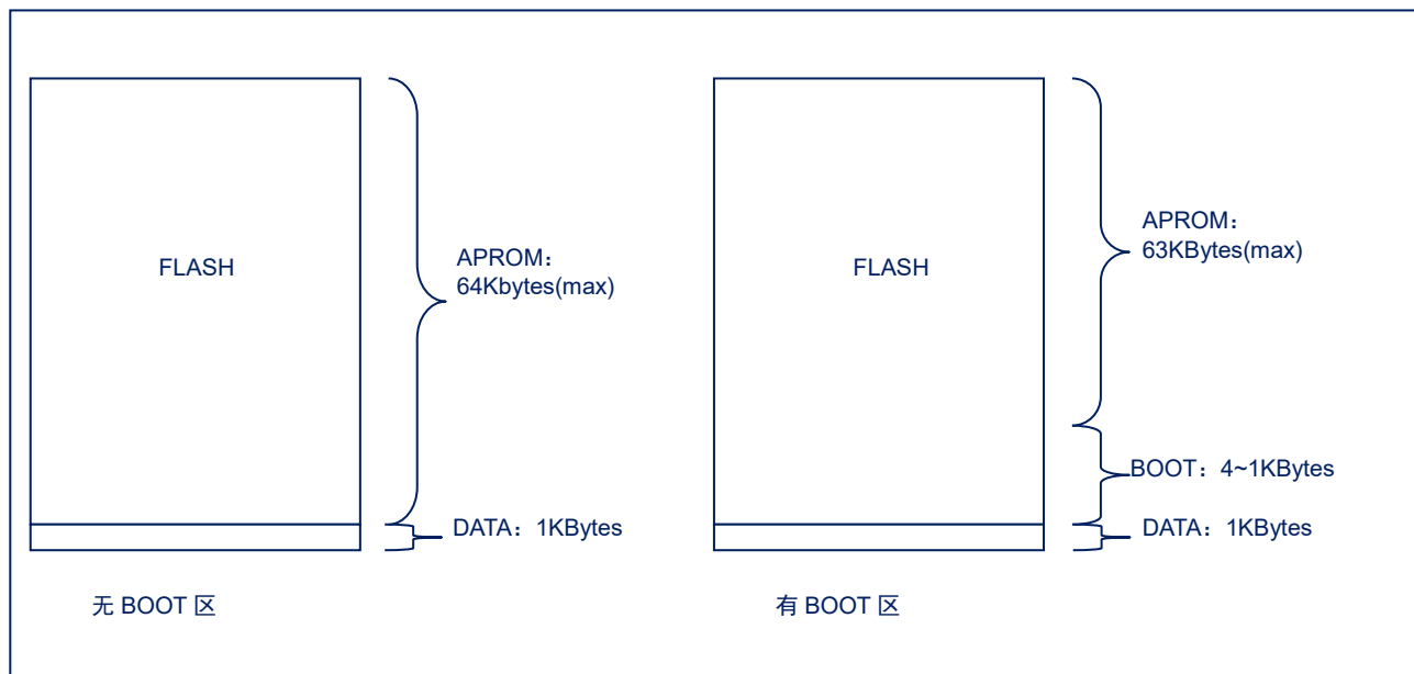
图 25-1：存储结构图
