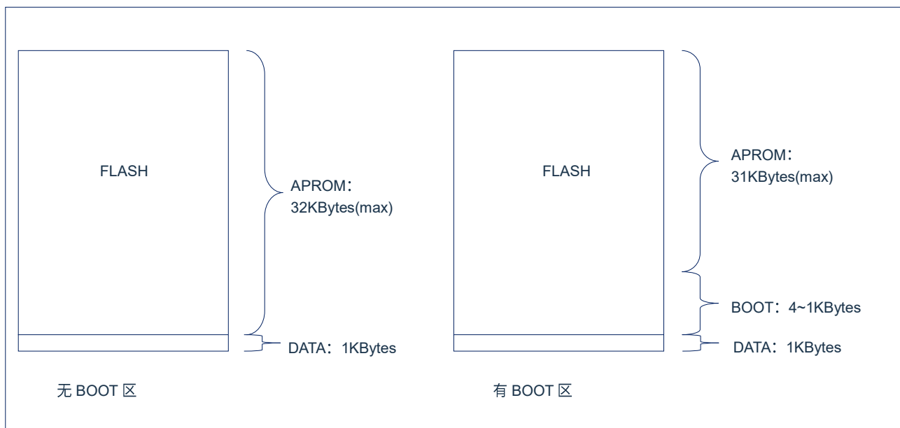
图 24-1: 存储器结构图
