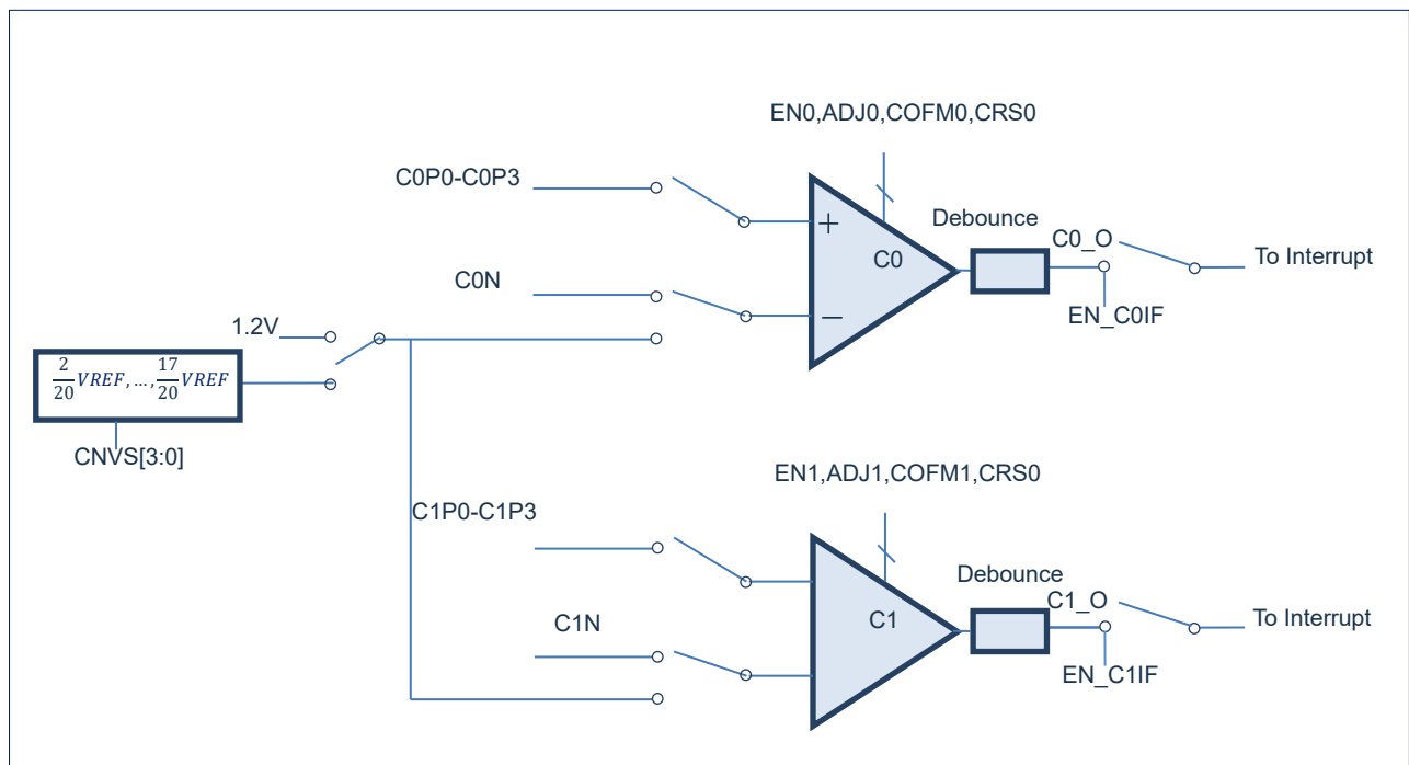
图 23-1：比较器结构图
