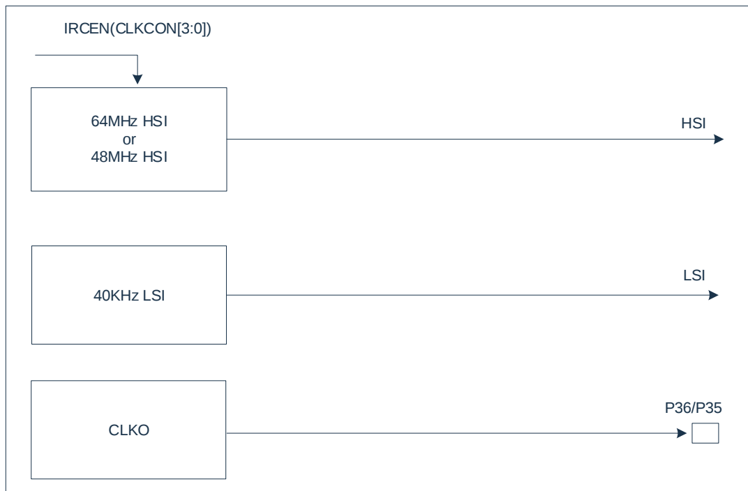
图 3-1：时钟结构框图
