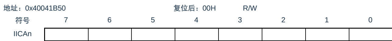
图16-3 IICAn移位寄存器n (IICAn) 的格式
