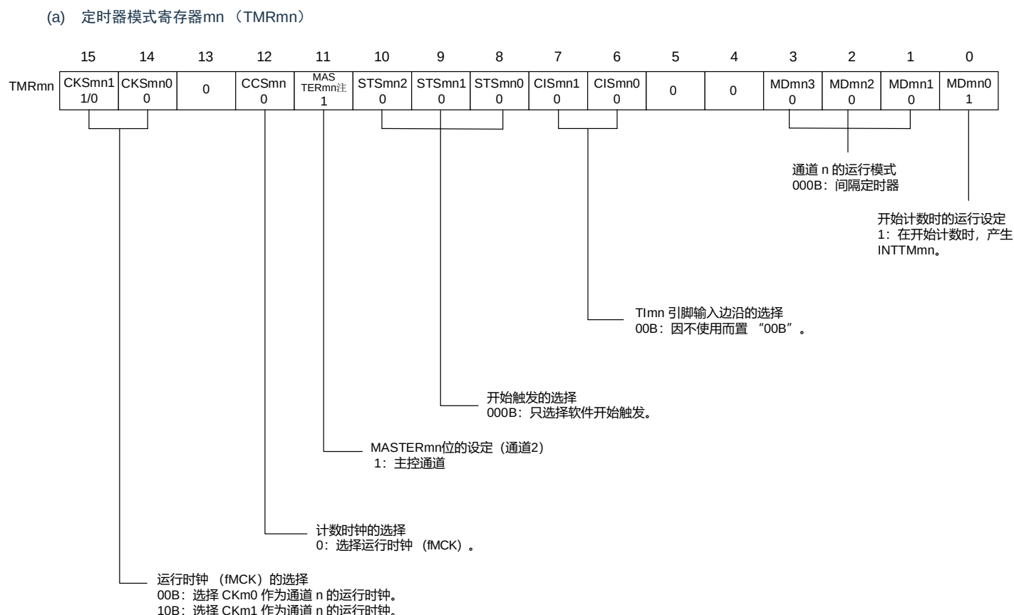
图5-75 多重PWM 输出功能时（主控通道）的寄存器设定内容例子
