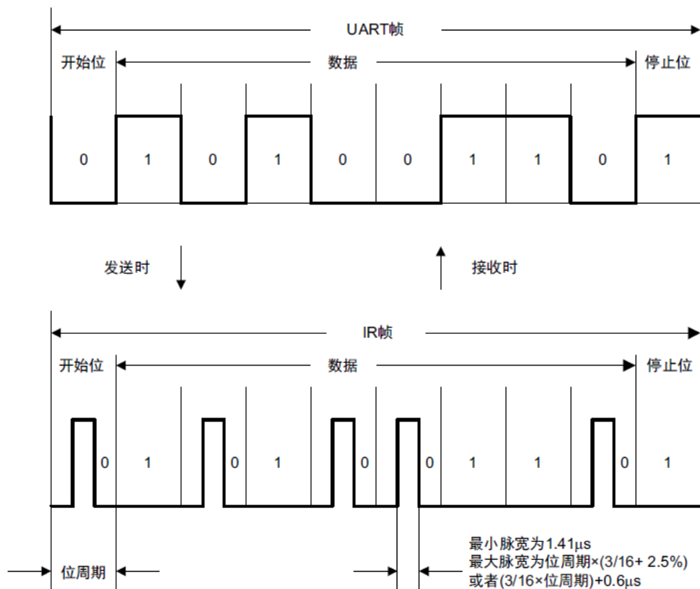
图17-4 IrDA的发送/接收运行图
