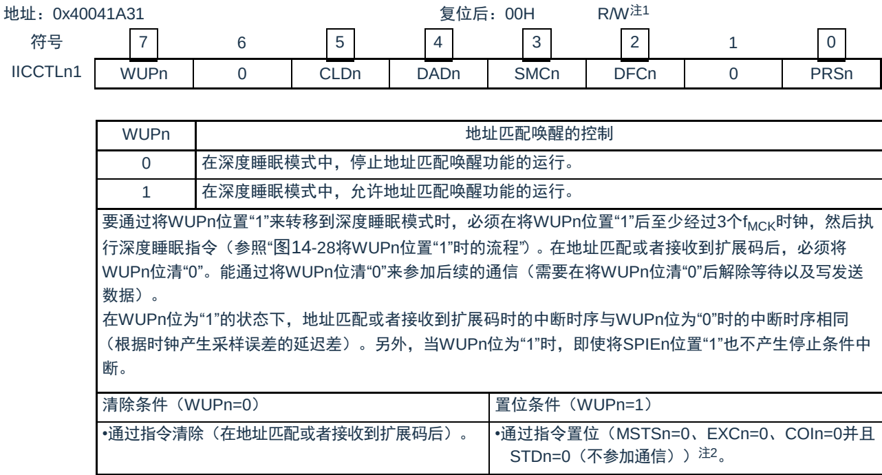
图16-9 IICA控制寄存器n1 (IICCTLn1) 的格式(1/2)
