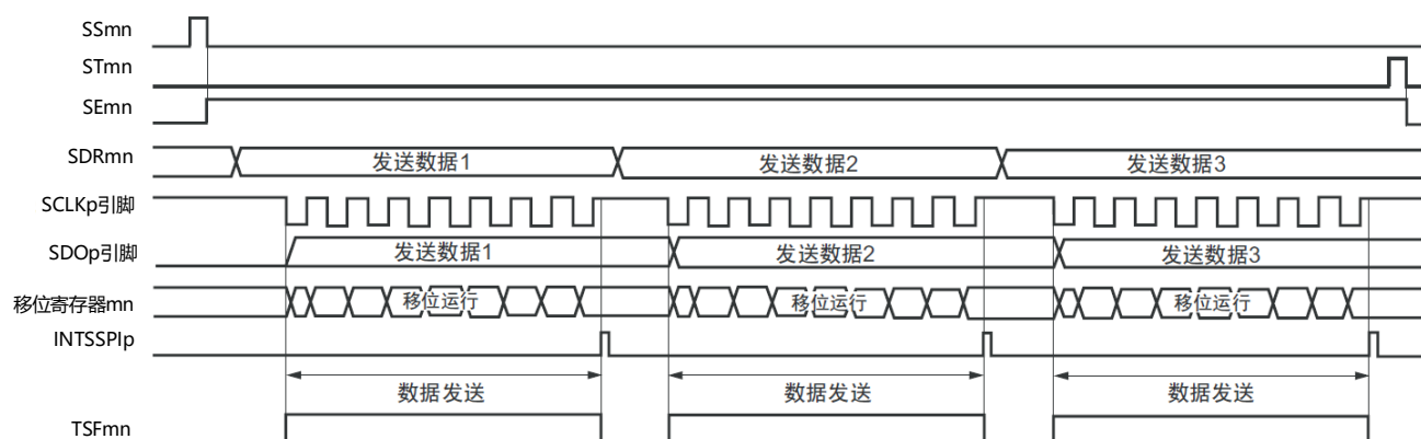
图14-51从属发送（单次发送模式）的时序图（类型1：DAPmn=0、CKPmn=0）
