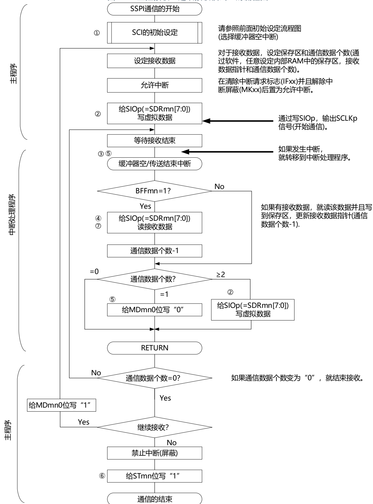
图14-38主控接收（连续接收模式）的流程图
