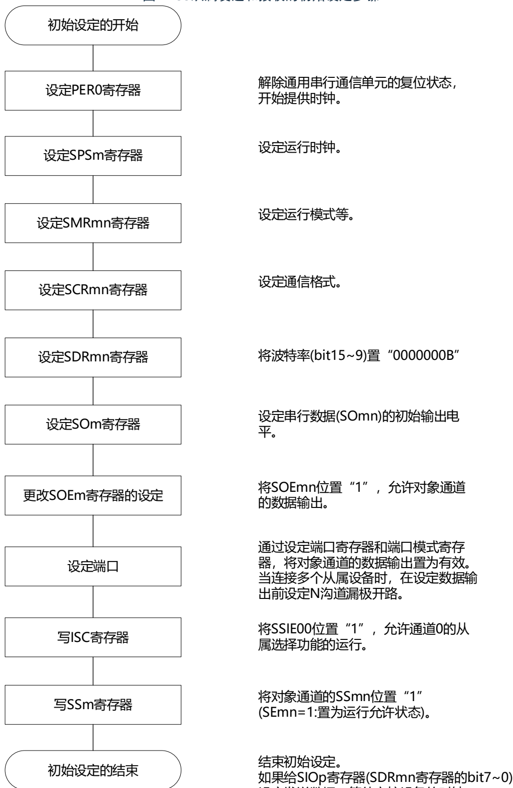
图14-88从属发送和接收的初始设定步骤
