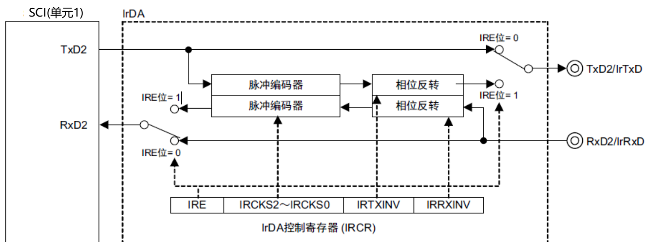
图17-1 IrDA与SCI的合作示意框图
