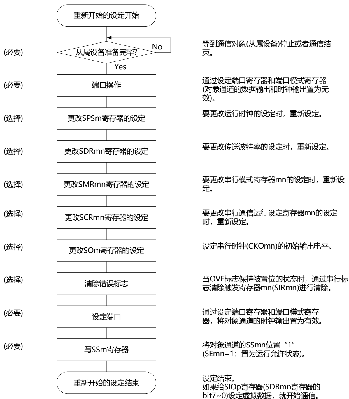
图14-34重新开始主控接收的设定步骤
