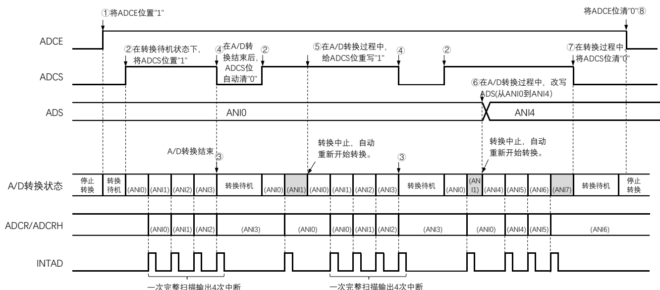
图 11-23 软件触发模式（扫描模式、单次转换模式）的运行时序例子
