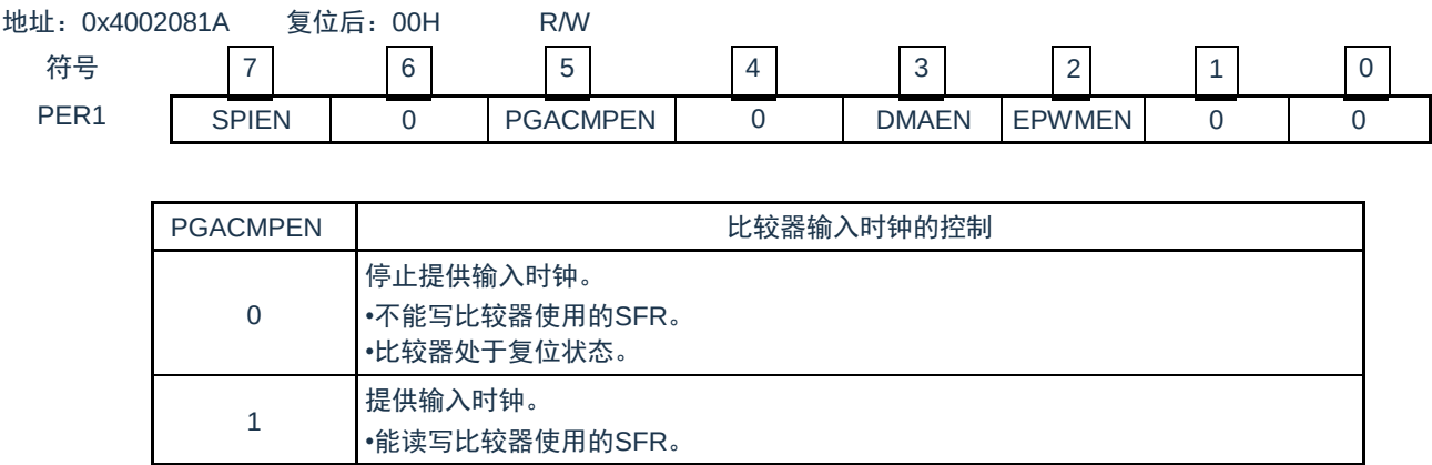
图12-1 外围允许寄存器1（PER1）的格式
