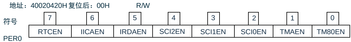
图19-2：外围允许寄存器0（PER0）的格式
