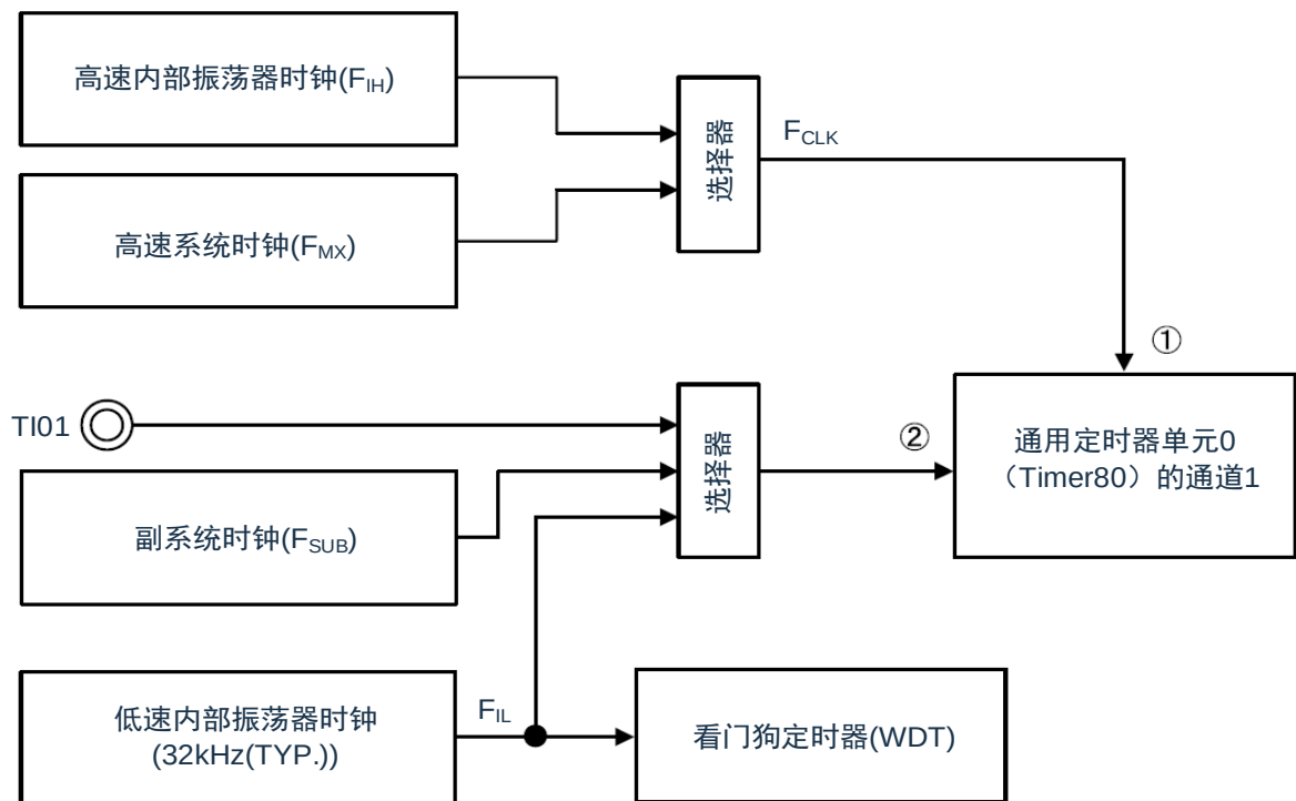
图30-10: 频率检测功能的结构
