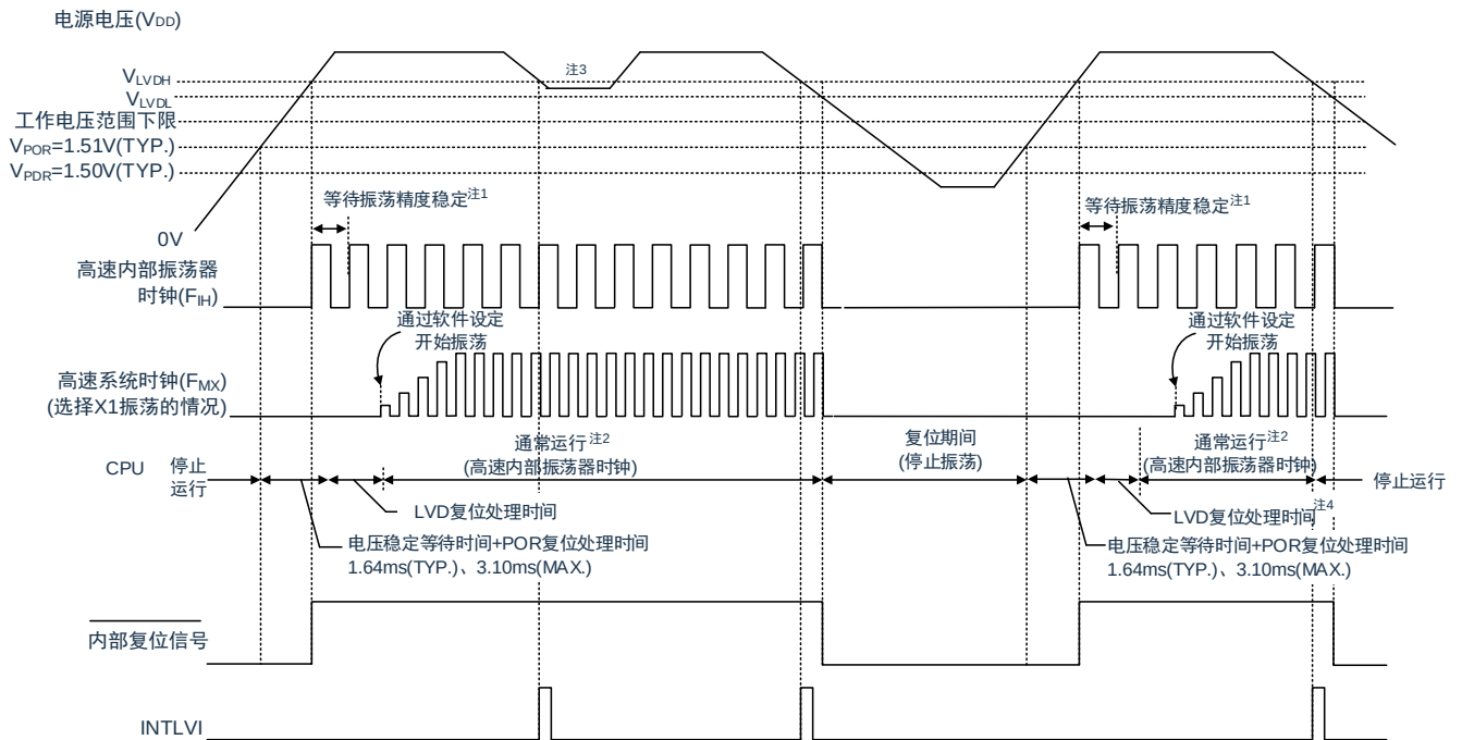
图 28-3：上电复位电路和电压检测电路的内部复位信号的产生时序(2/3)
