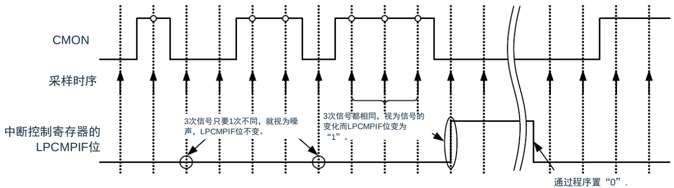
图14-11：低功耗比较器的数字滤波器和中断运行示例
