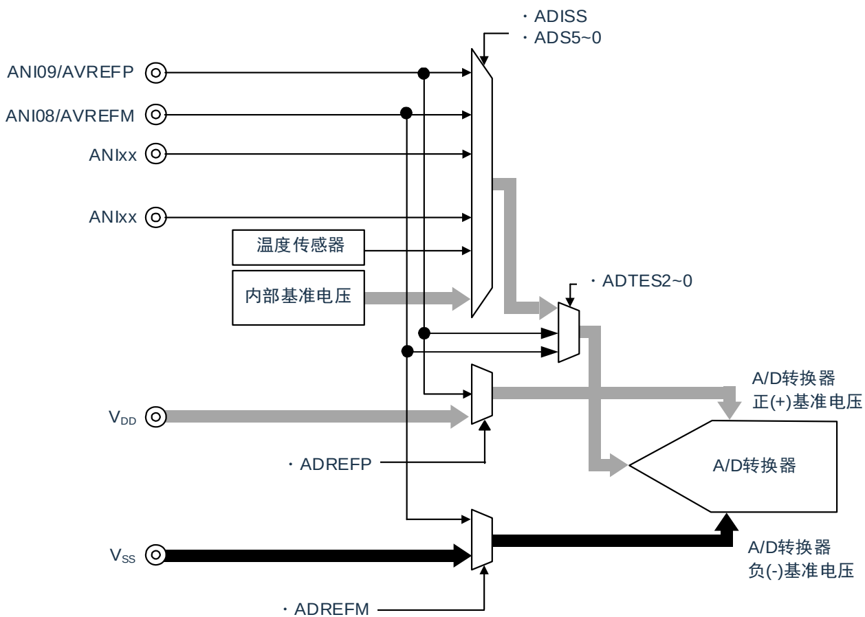
图30-11: A/D测试功能的结构
