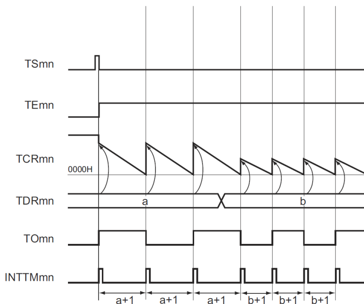
图5-41：作为间隔定时器/方波输出运行的基本时序例子（MDmn0=1）
