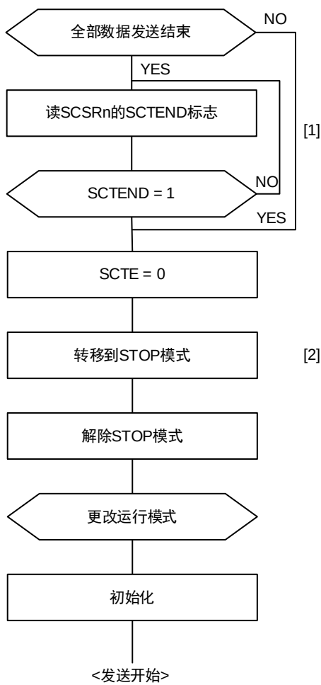
图 20-30发送时的模式转移流程图例子
