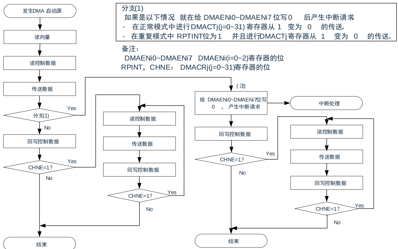
图22-15：DMA的内部运行流程图
