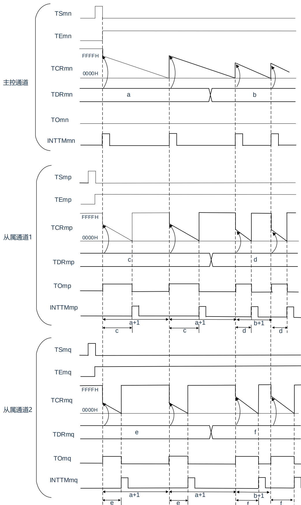
图5-72：作为多重PWM输出功能的运行基本时序例子（输出2种PWM的情况）
