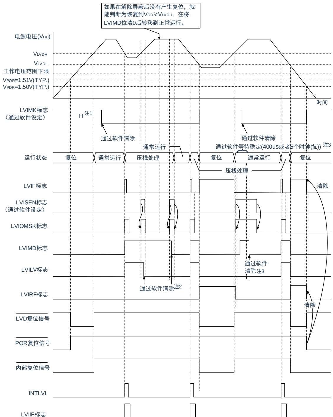
图 29-6：复位&中断信号的产生时序（选项字节的LVIMDS1、LVIMDS0=1、0）(1/2)
