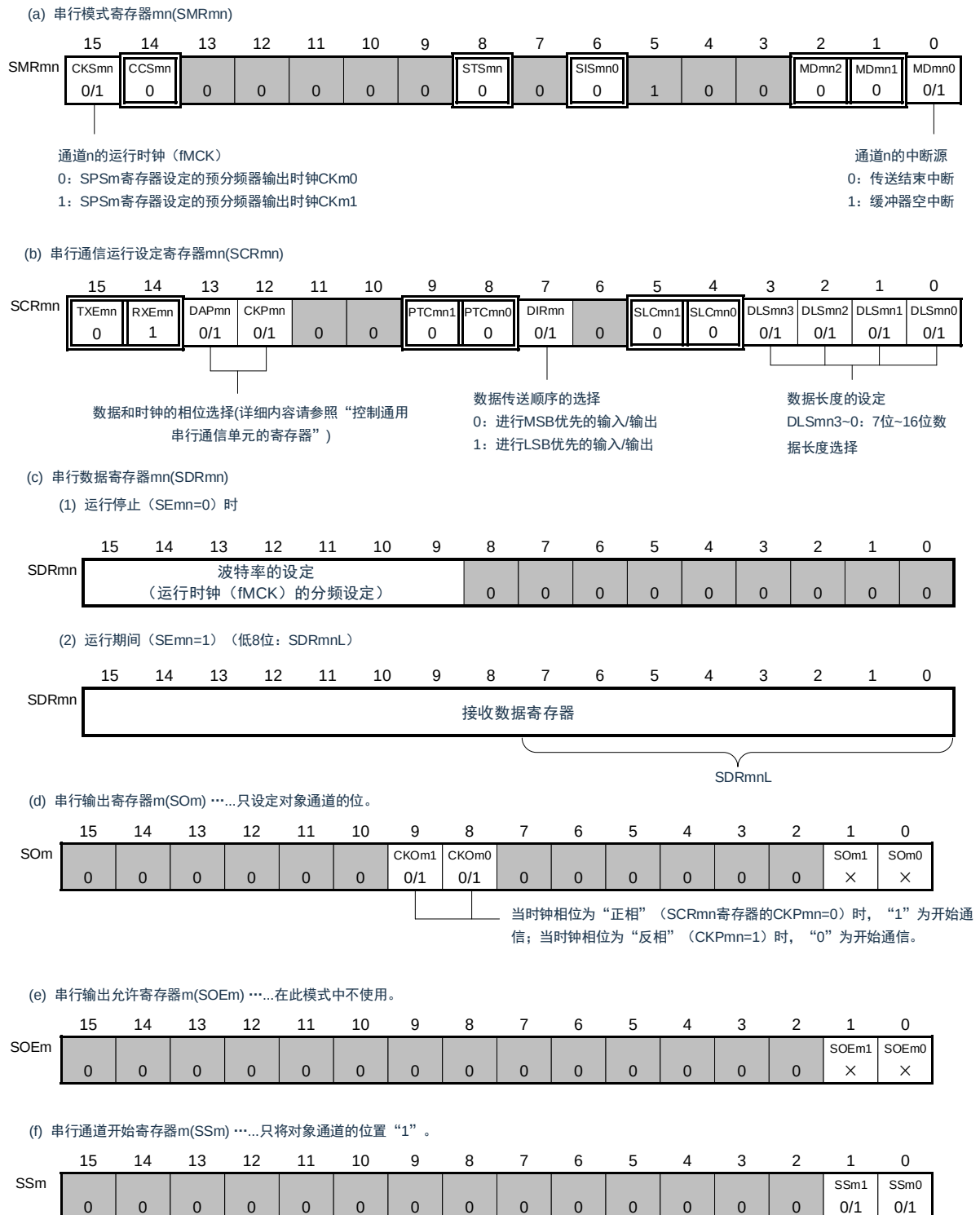
图16-31：3线串行I/O（SSPlmn）
