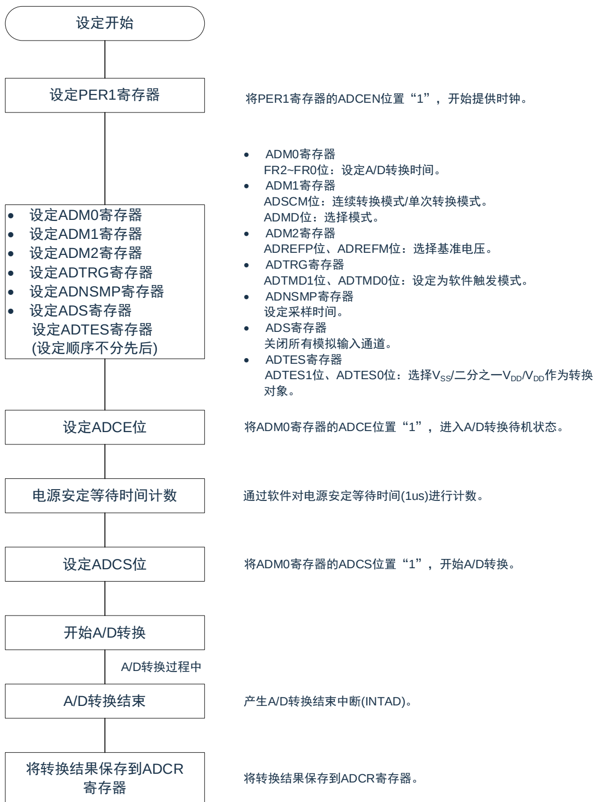
图11-35：测试模式的设定( V_{SS}/half\_V_{DD}/V_{DD} 作为转换对象)
