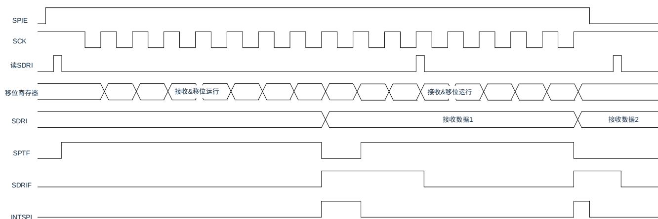
图17-20: 接收时序的时序图 (CPHA=1、CPOL=1)
