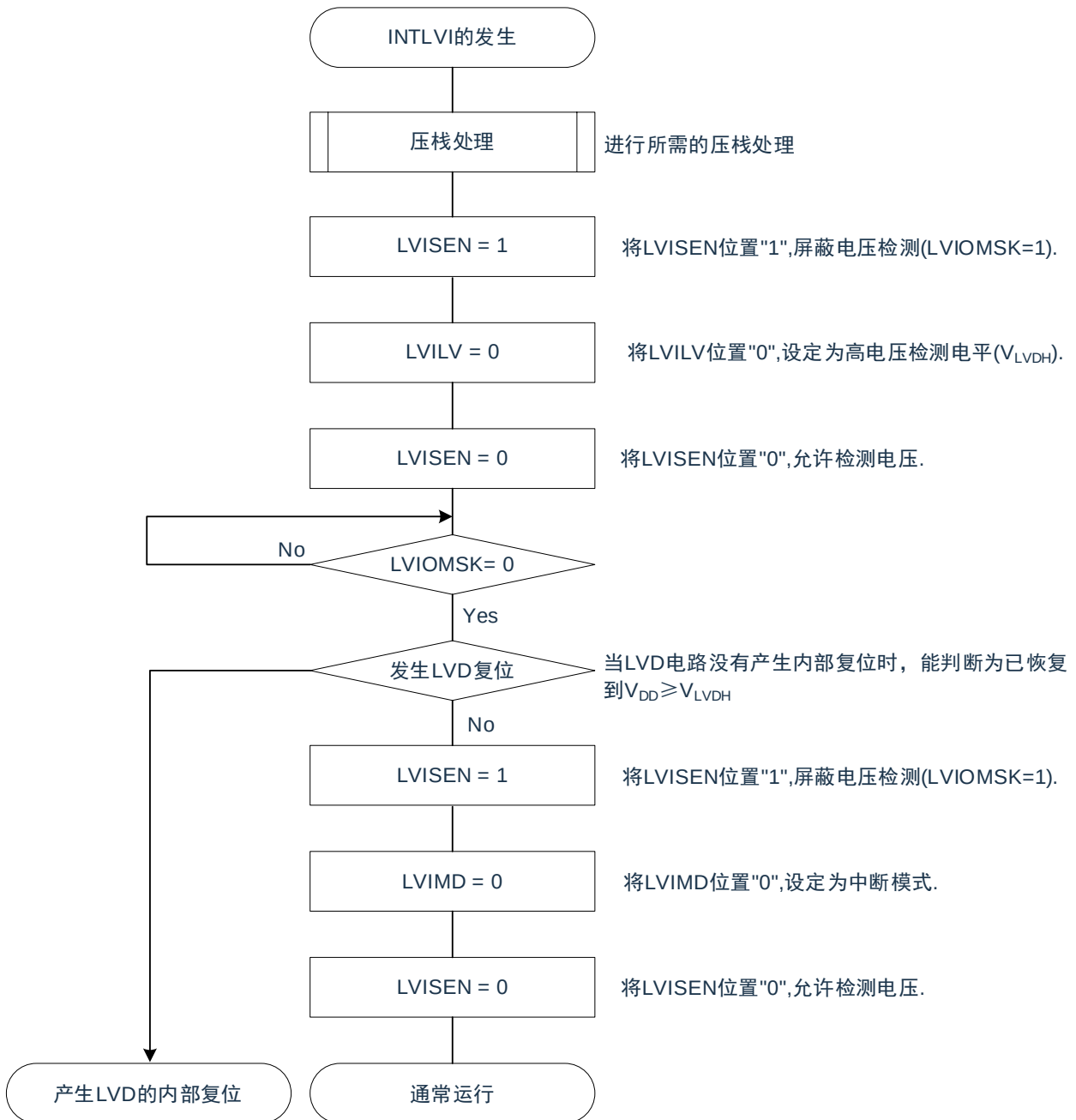
图 29-7：工作电压的确认/复位的设置步骤
