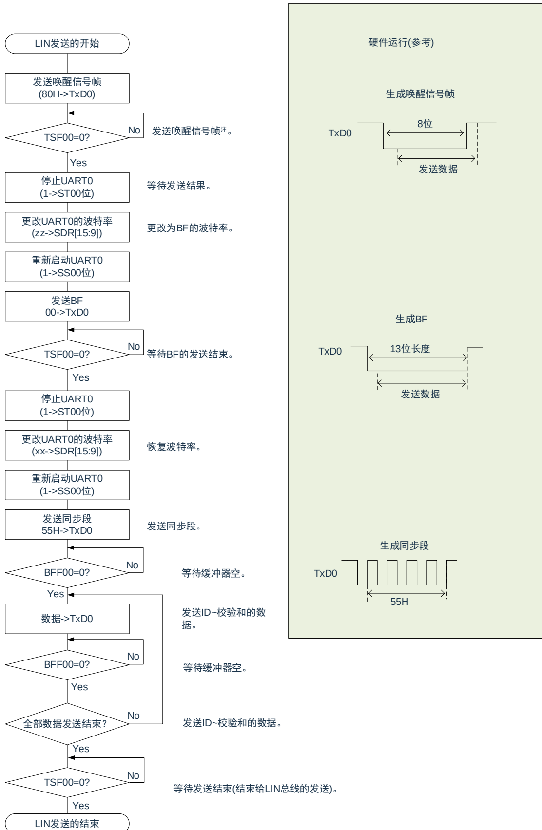
图16-118: LIN发送的流程图
