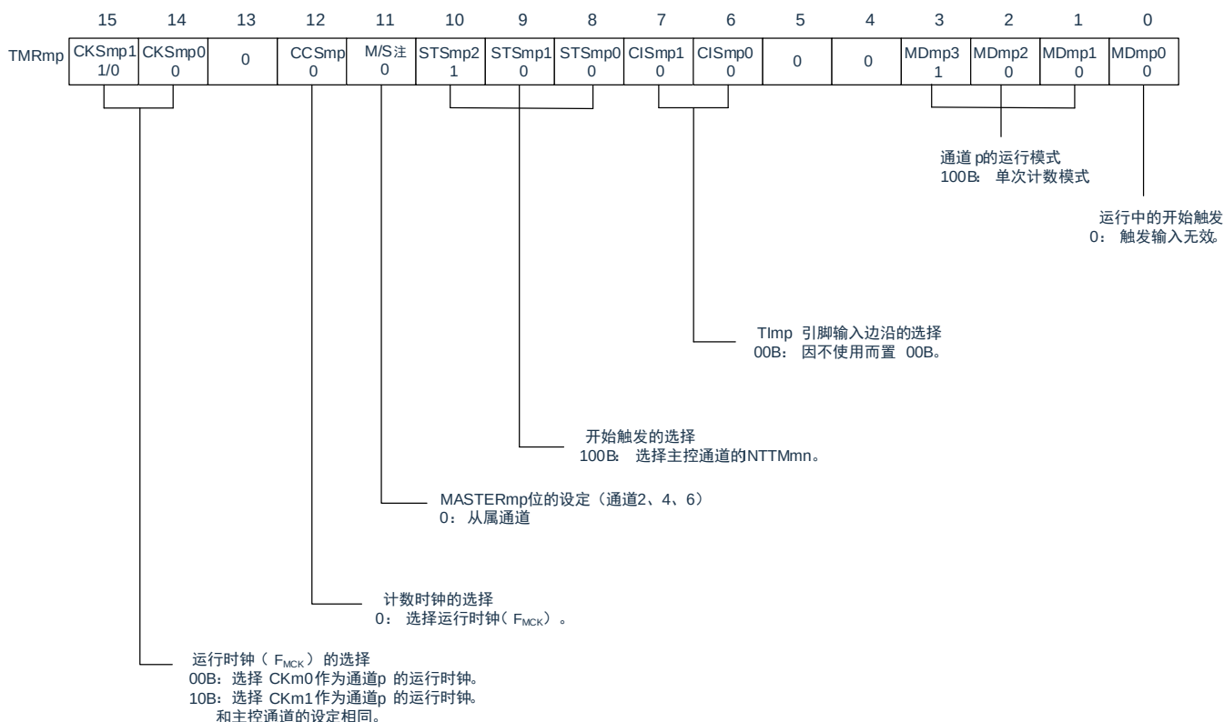
图5-62：单触发脉冲输出功能时（从属通道）的寄存器设定内容例子
