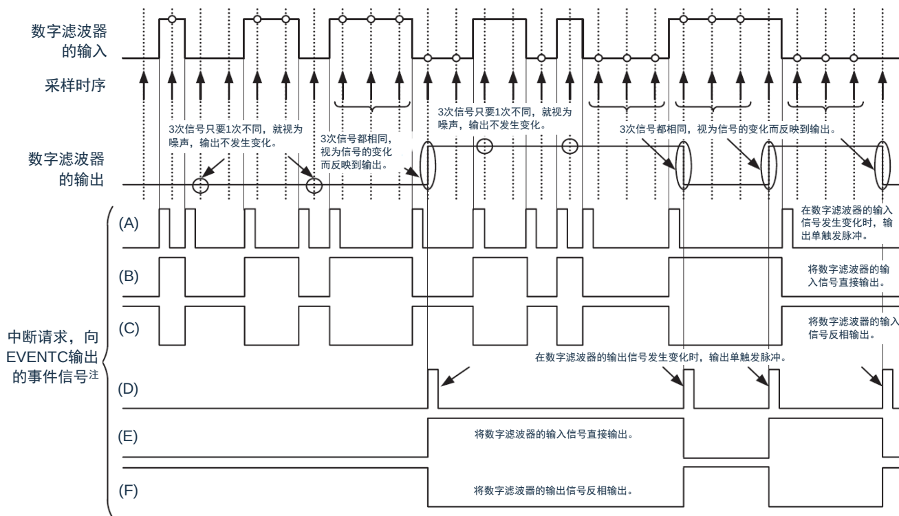
图13-13：数字滤波器、中断请求和向EVENTC输出事件信号的运行
