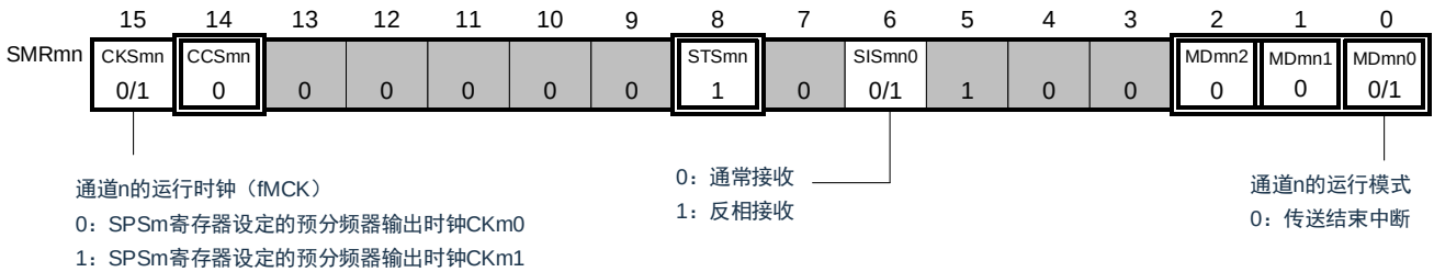
图16-104: UART (UARTm) 的UART接收时的寄存器设定内容例子(1/2)
