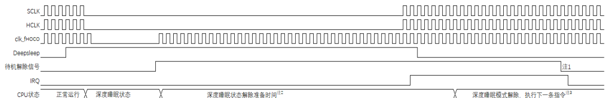
图26-3：通过中断请求解除深度睡眠模式
