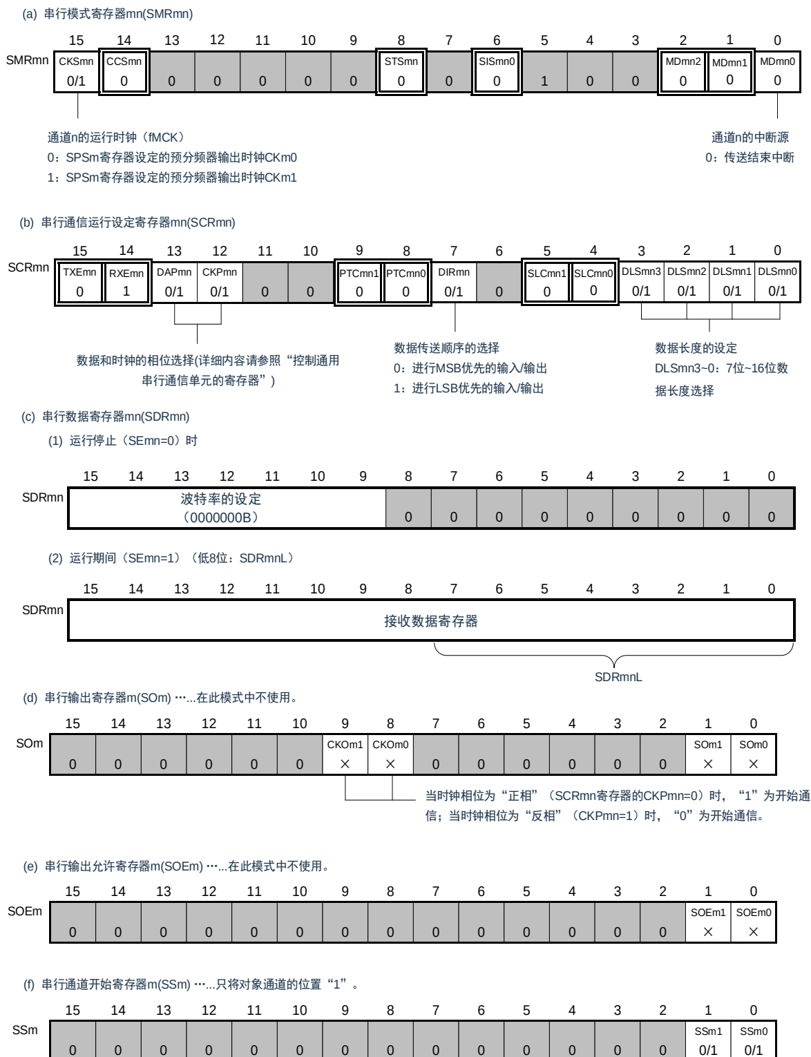
图16-55：3线串行I/O（SSPImn）
