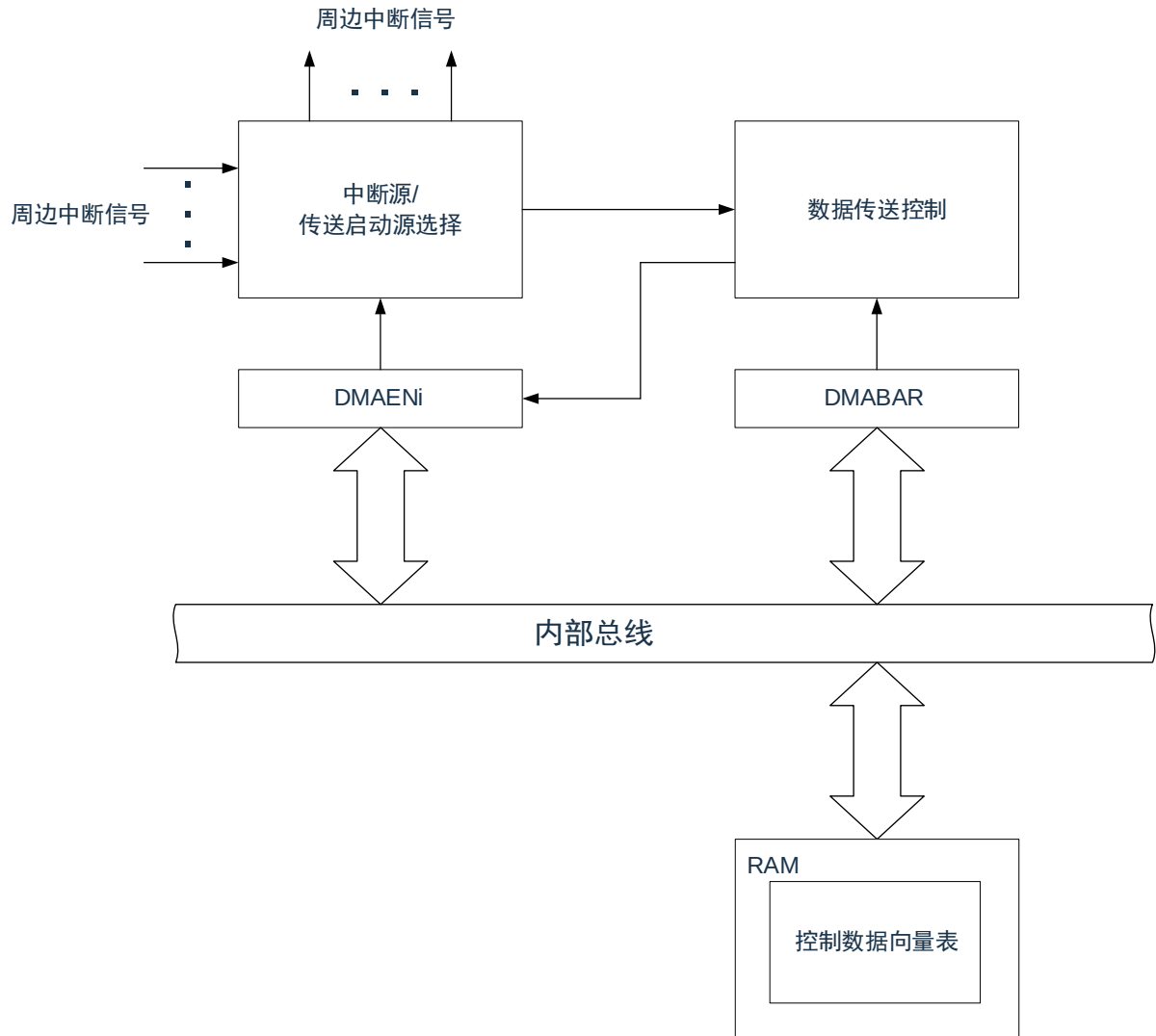
图22-1：DMA的框图
