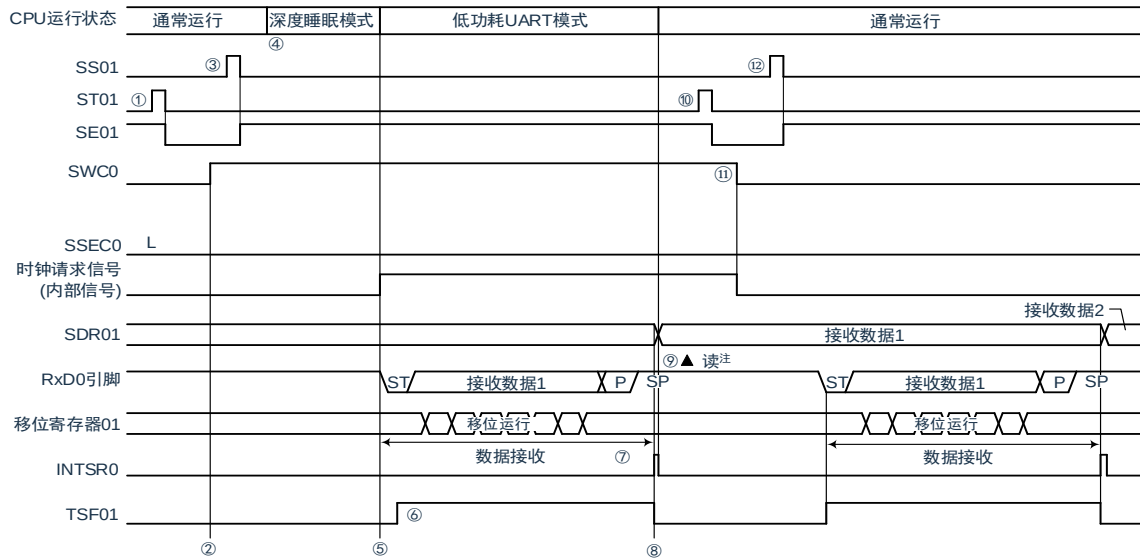
图 16-110：低功耗UART模式运行 (SSECm=0/1) 时序图
