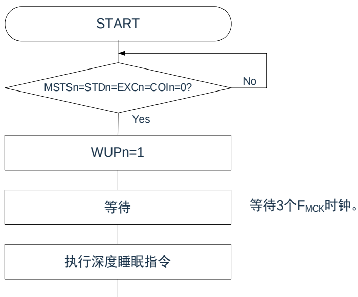
图18-21：将WUPn位置“1”时的流程
