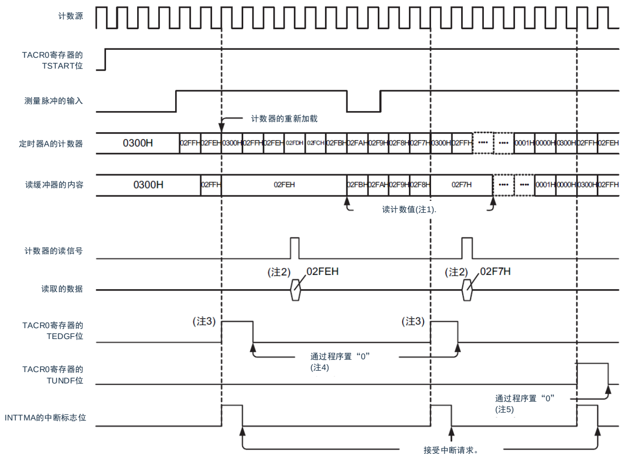
图 6-15：脉冲周期测量模式的运行例子
