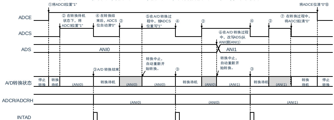
图 11-20：软件触发模式（选择模式、单次转换模式）的运行时序例子
