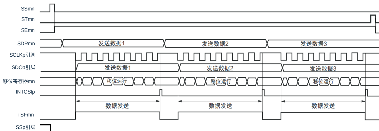
图16-76：从属发送（单次发送模式）的时序图（类型1：DAPmn=0、CKPmn=0）
