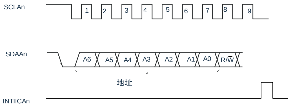
图18-15: 地址
