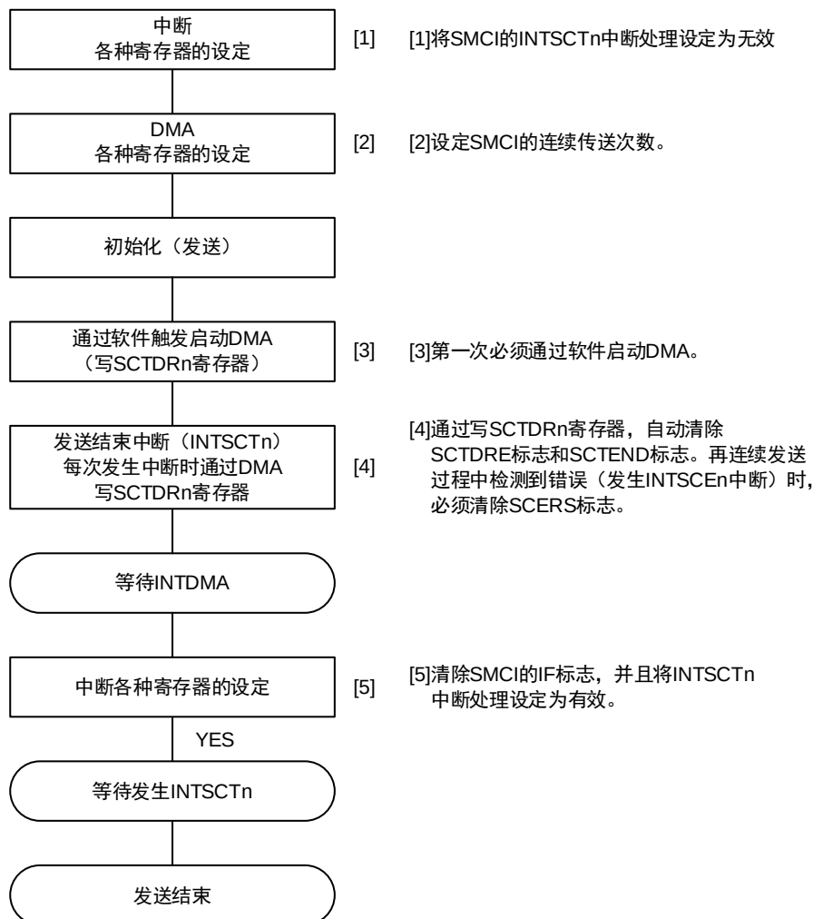
图 20-26 使用DMA进行连续数据发送的流程
