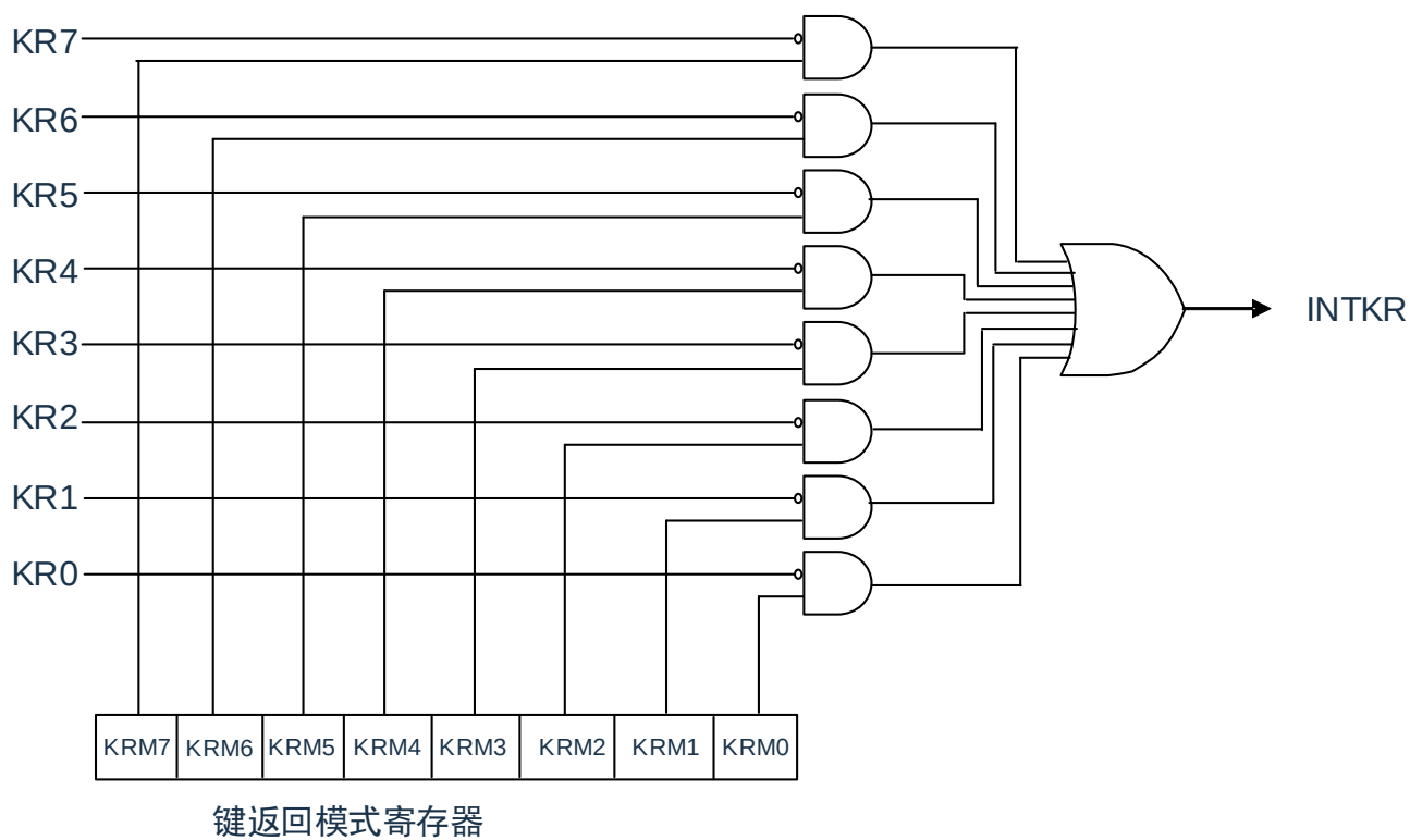
图25-1：键中断的框图
