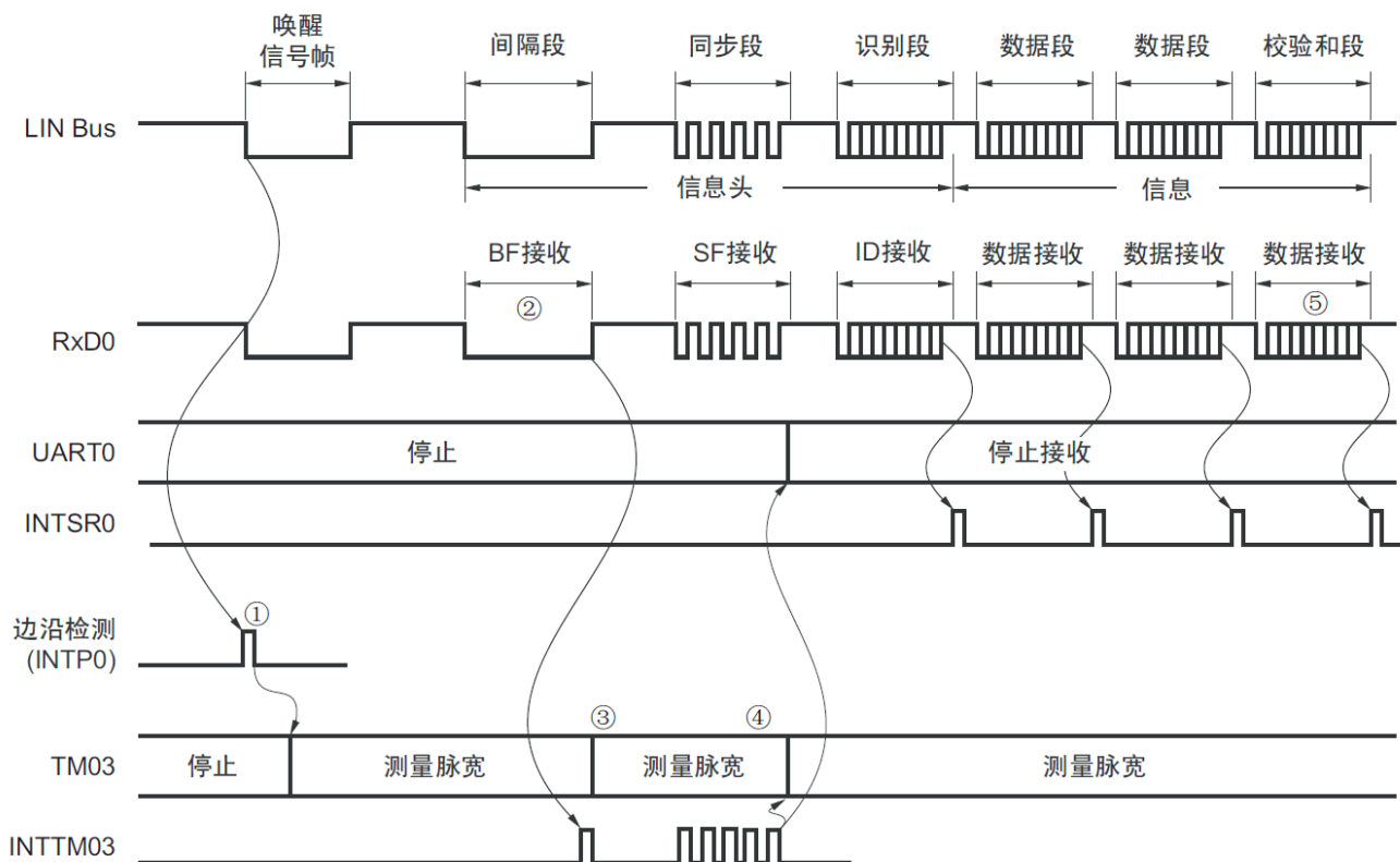
图16-119：LIN的接收操作
