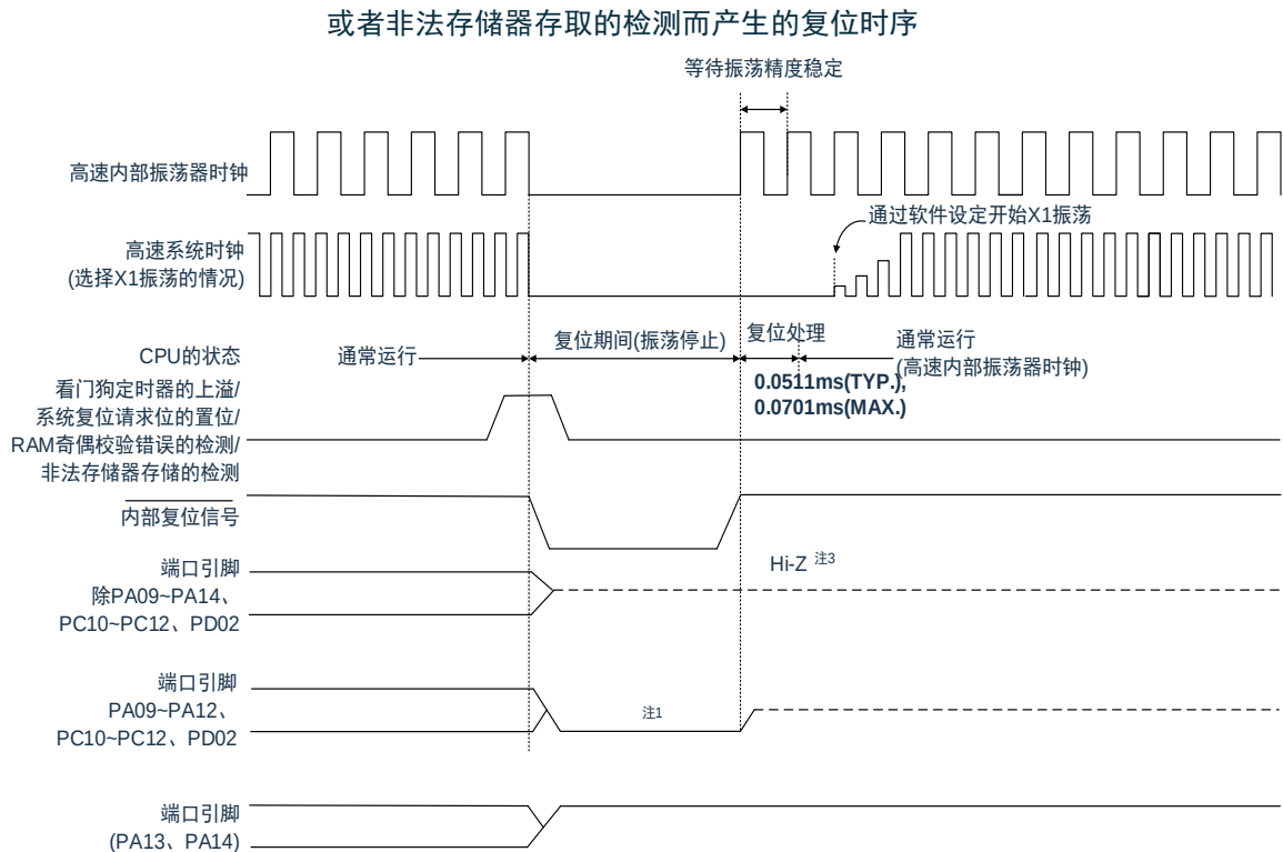
图27-3：因看门狗定时器的上溢、系统复位请求位的置位、RAM奇偶校验错误的检测
