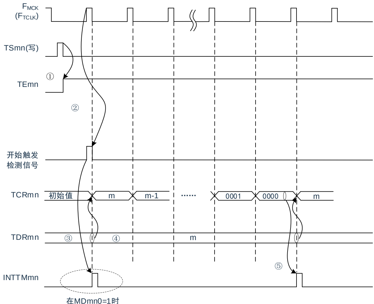
图5-24：运行时序（间隔定时器模式）
