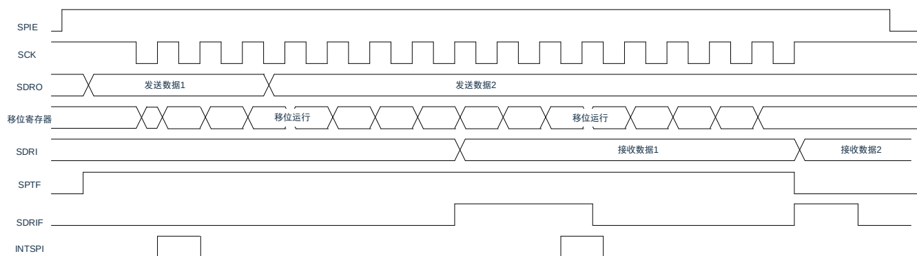
图17-17: 发送/接收时序(连续发送模式)的时序图 (INTMD=1, CPHA=1、CPOL=1)
