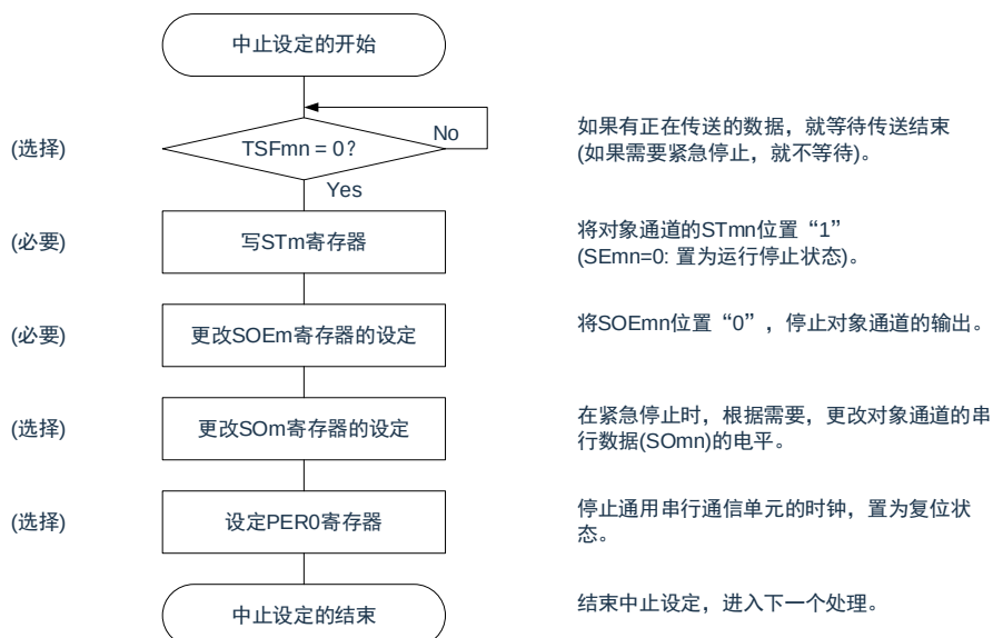
图16-49：从属发送的中止步骤
