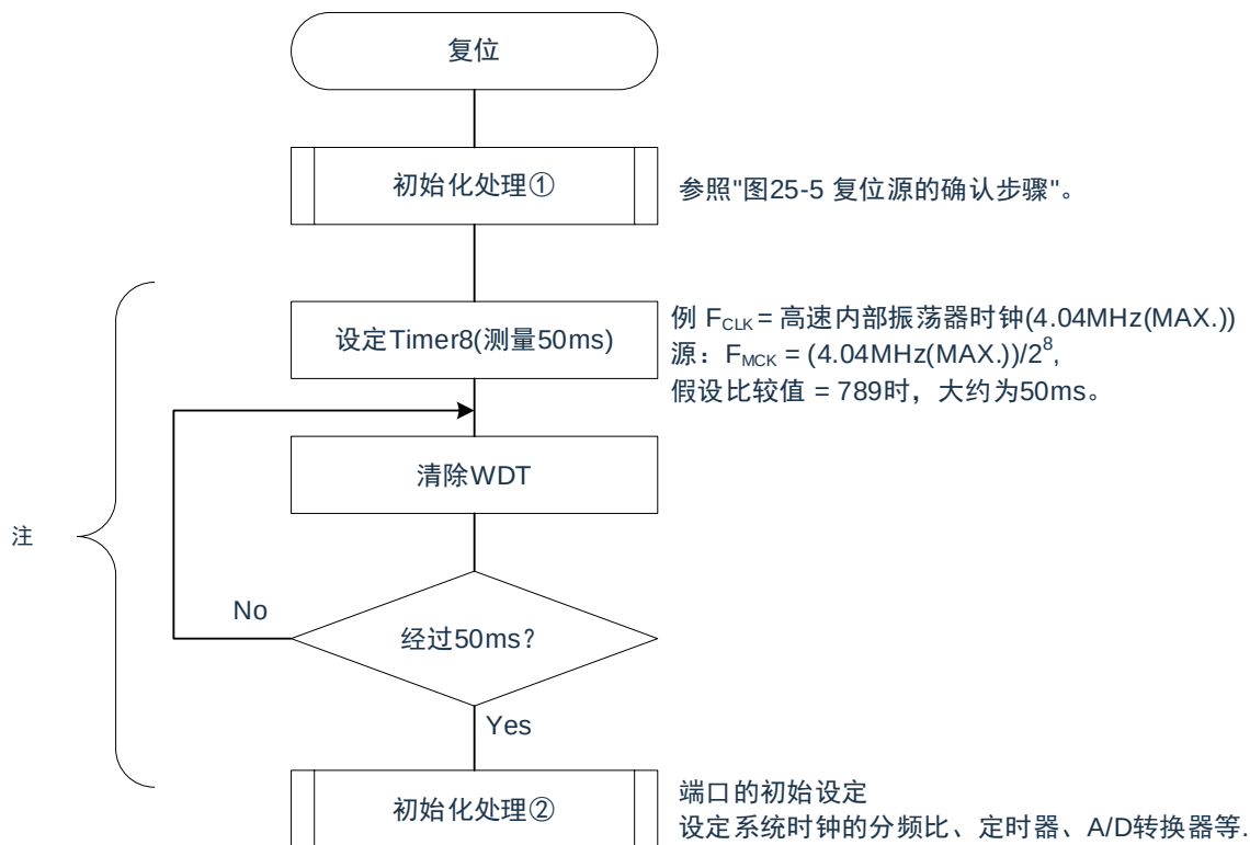
图 29-9：LVD检测电压附近的电源电压波动不超过50ms时的软件处理例子
