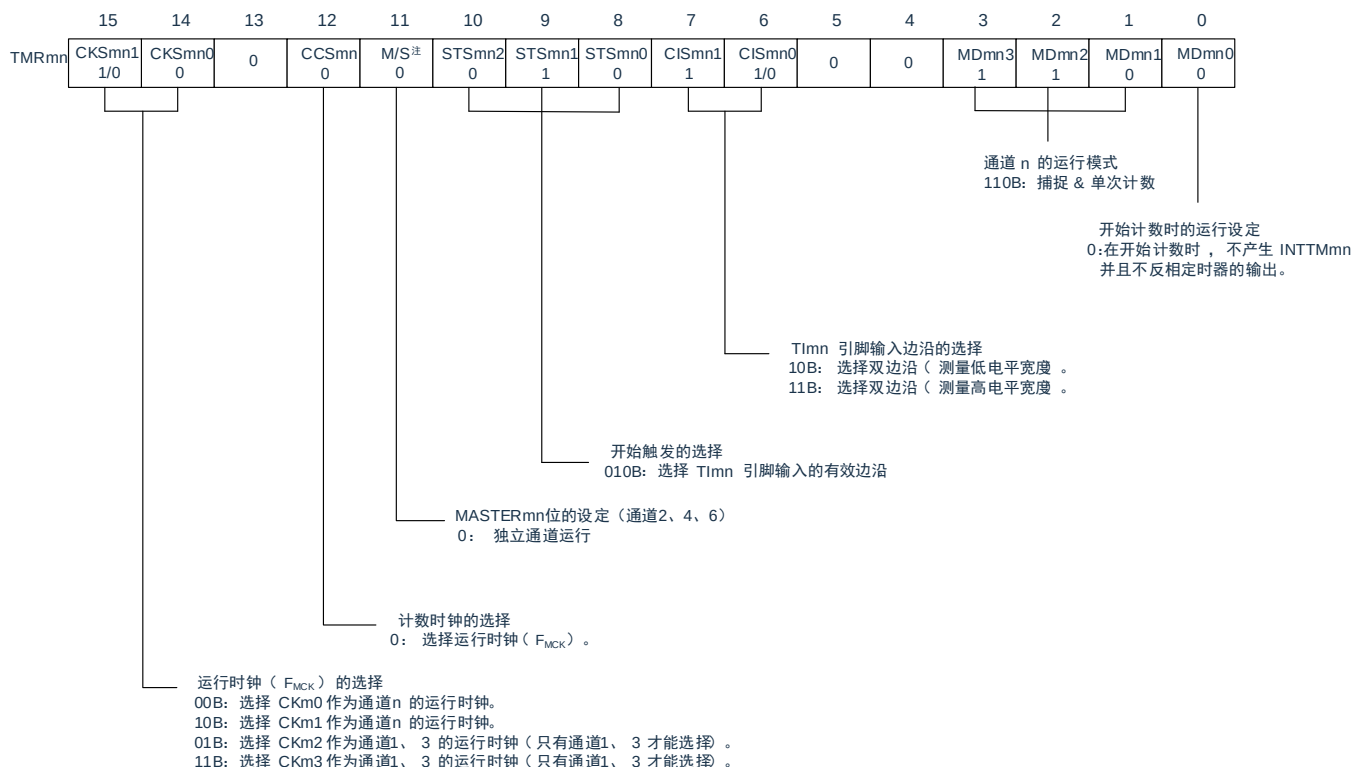
图5-54：测量输入信号的高低电平宽度时的寄存器设定内容例子
