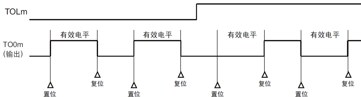
图5-33: 在定时器运行中更改TOLm寄存器的内容时的运行
