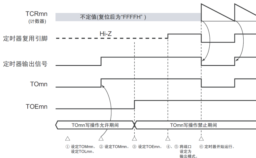
图5-30：从设定定时器的输出到开始运行的状态变化
