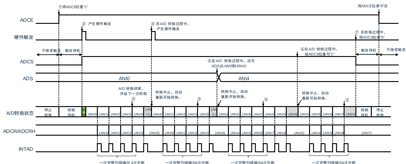
图11-29：硬件触发等待模式（扫描模式、连续转换模式）的运行时序例子
