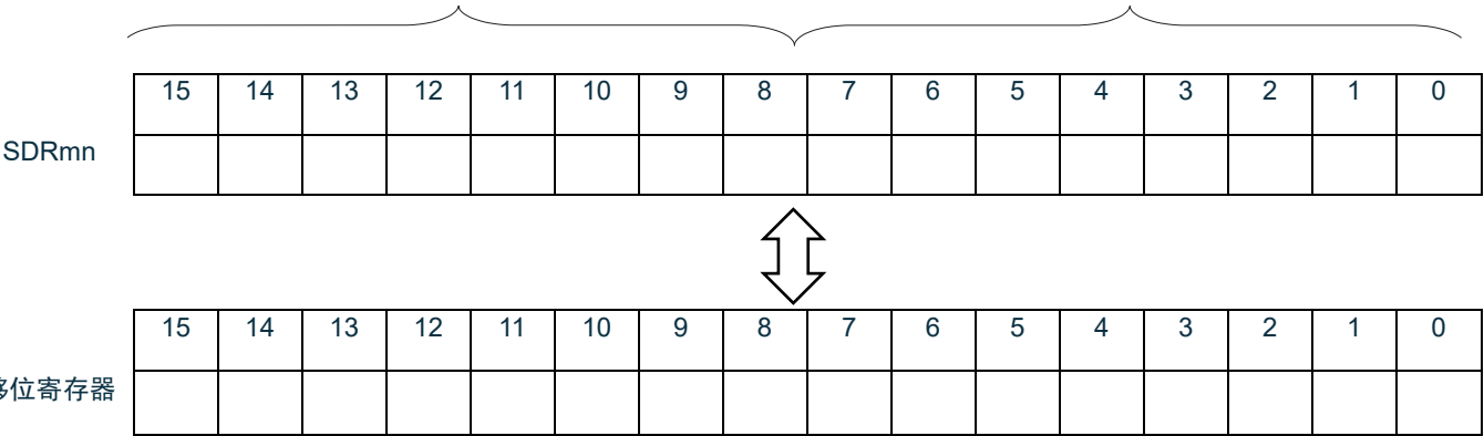
图16-2：串行数据寄存器mn（SDRmn）的格式
