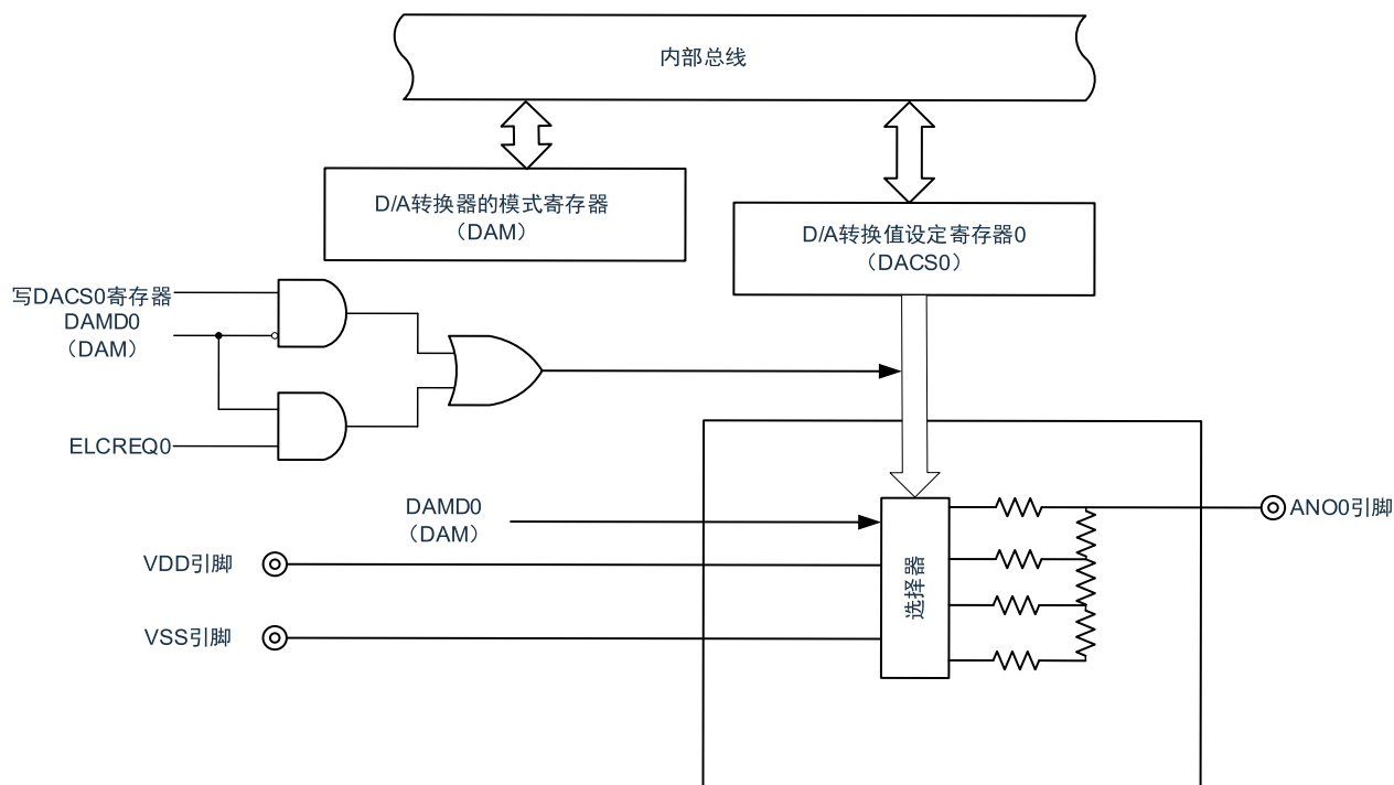
图12-1：D/A转换器的框图
