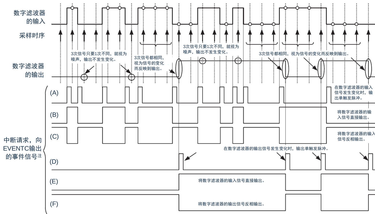
图14-12：数字滤波器、中断请求和向EVENTC输出事件信号的运行
