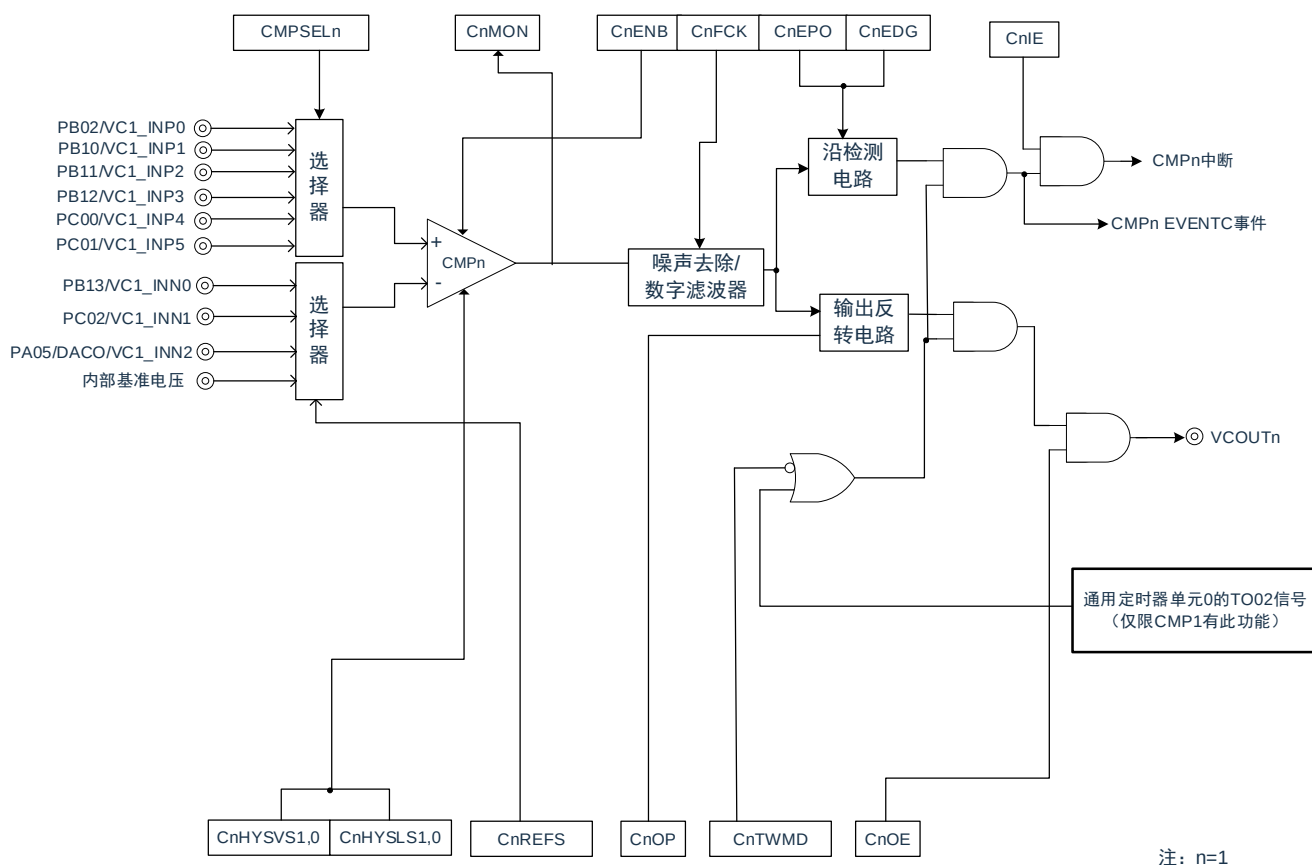
图13-2：比较器1的框图
