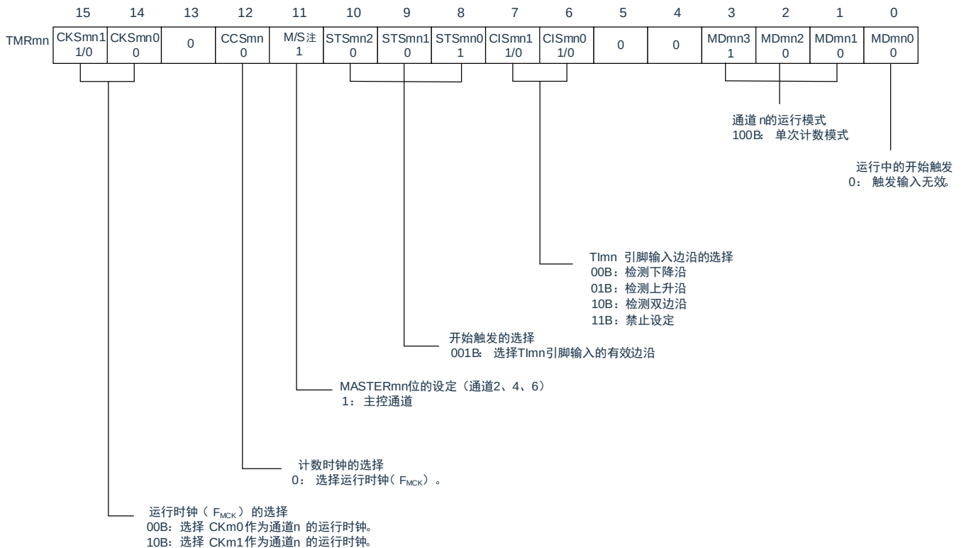
图5-61：单触发脉冲输出功能时（主控通道）的寄存器设定内容例子
