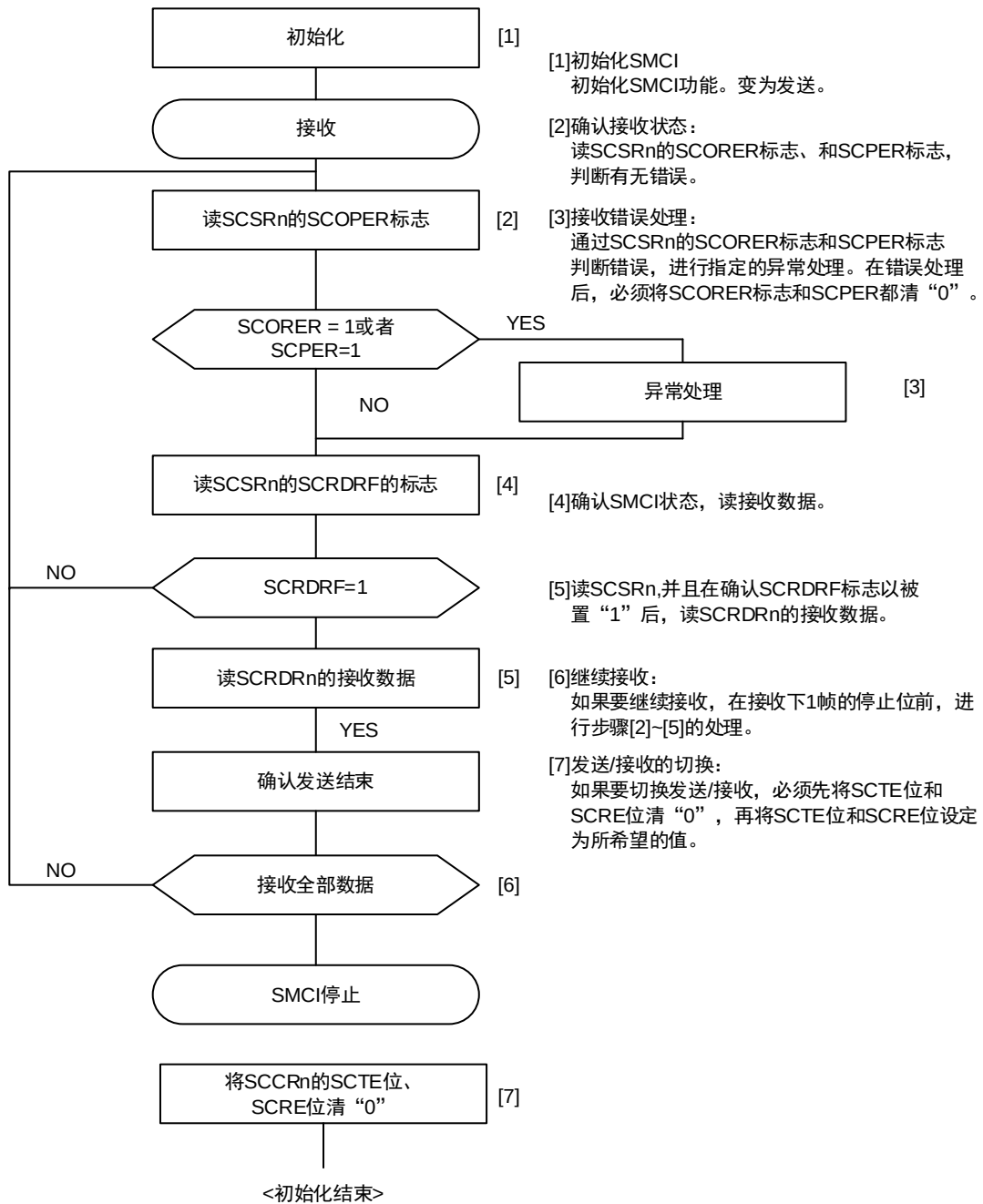
图 20-22 SMCI接收流程图的例子
