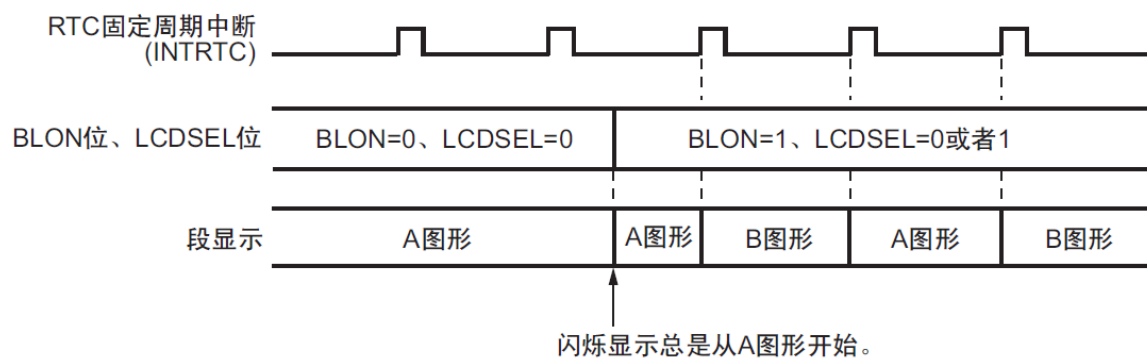
图 21-9：从A 图形显示到闪烁显示的切换运行
