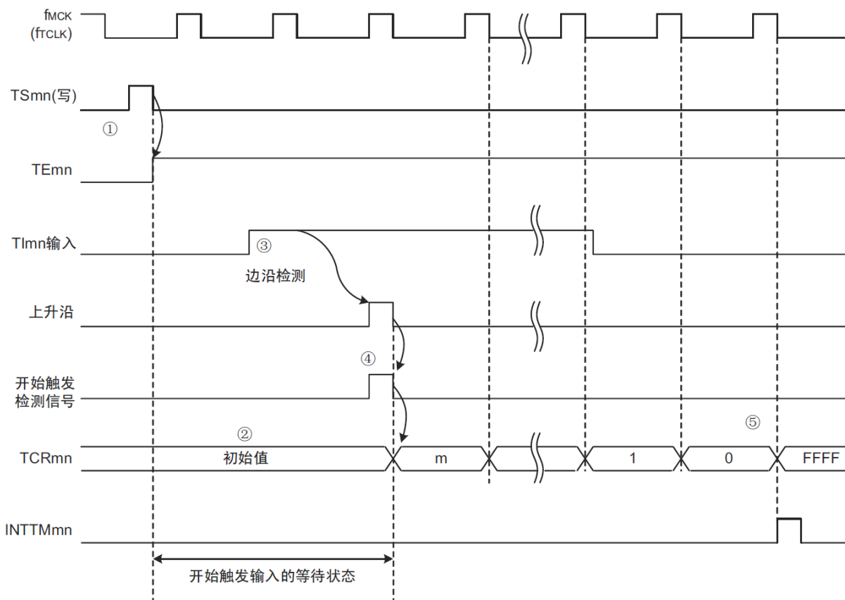
图5-27：运行时序（单次计数模式）
