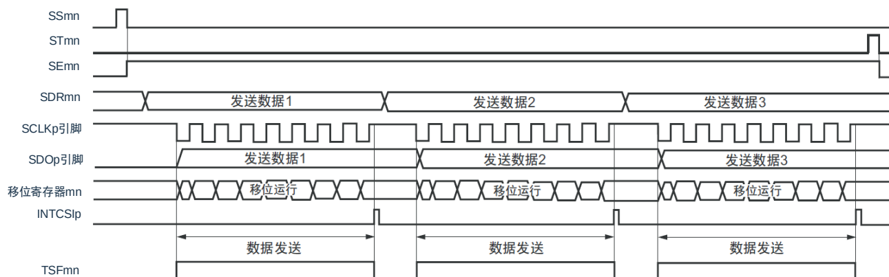
图16-51：从属发送（单次发送模式）的时序图（类型1：DAPmn=0、CKPmn=0）
