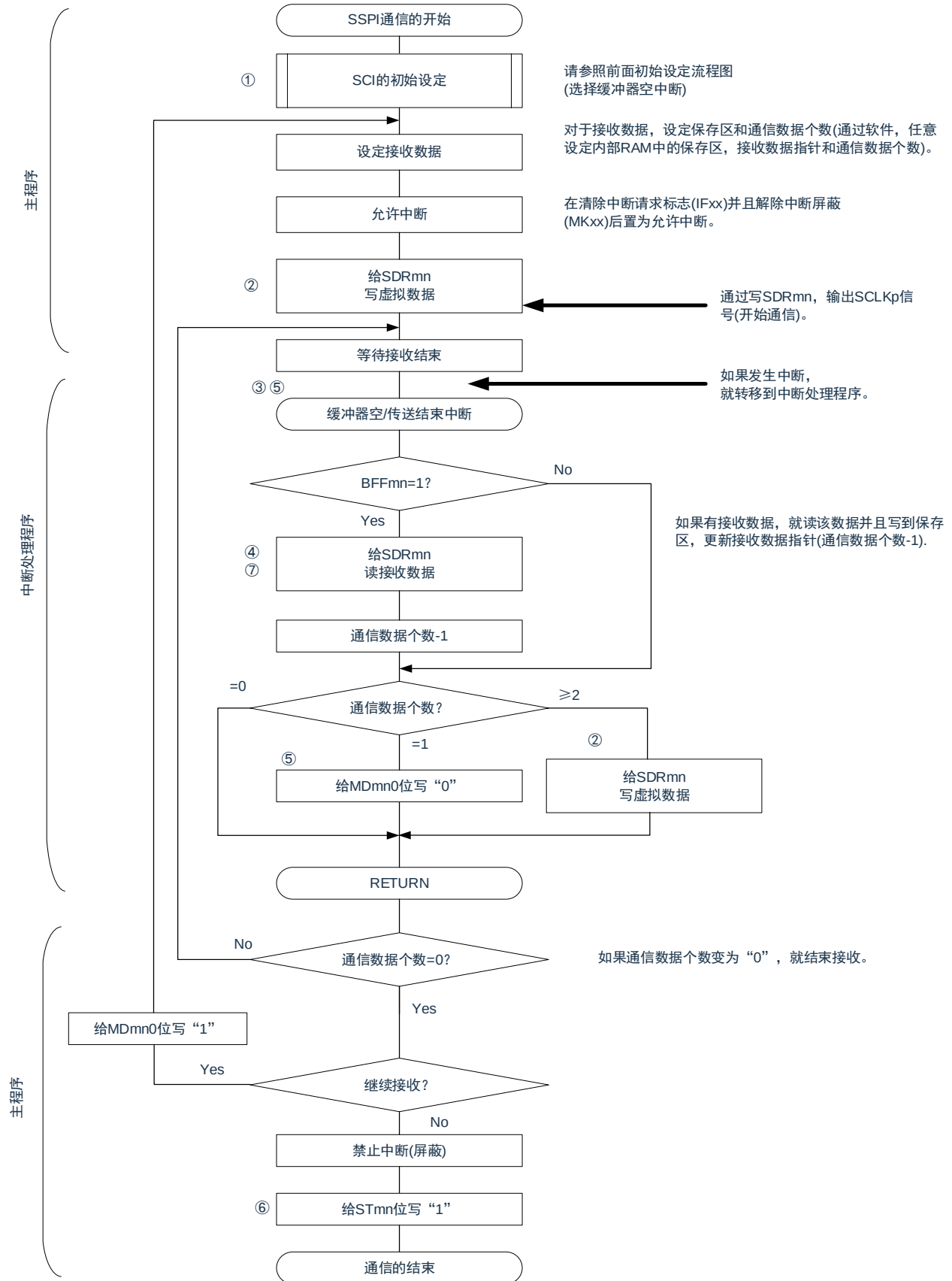
图16-38: 主控接收（连续接收模式）的流程图
