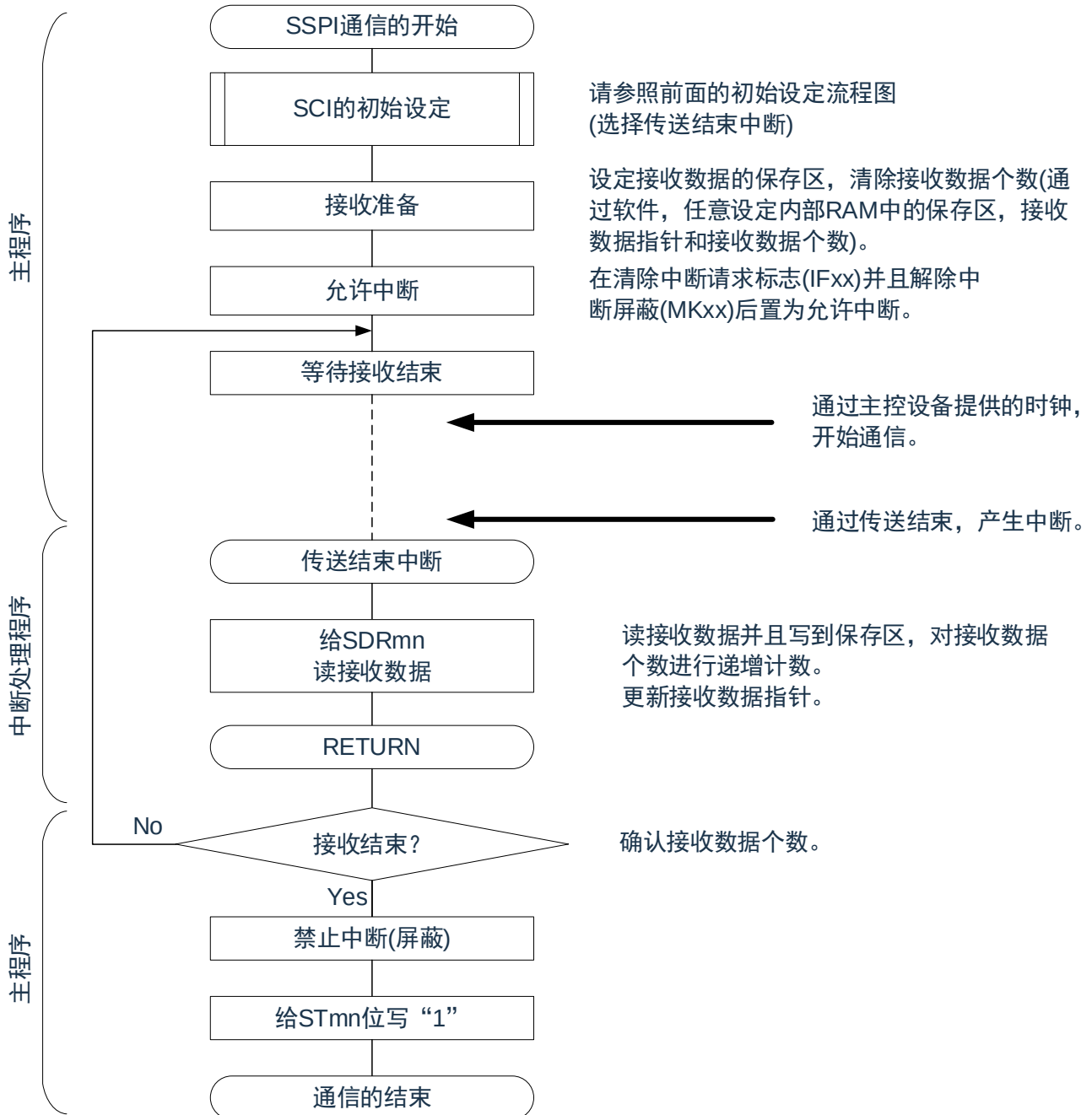
图16-60：从属接收（单次接收模式）的流程图
