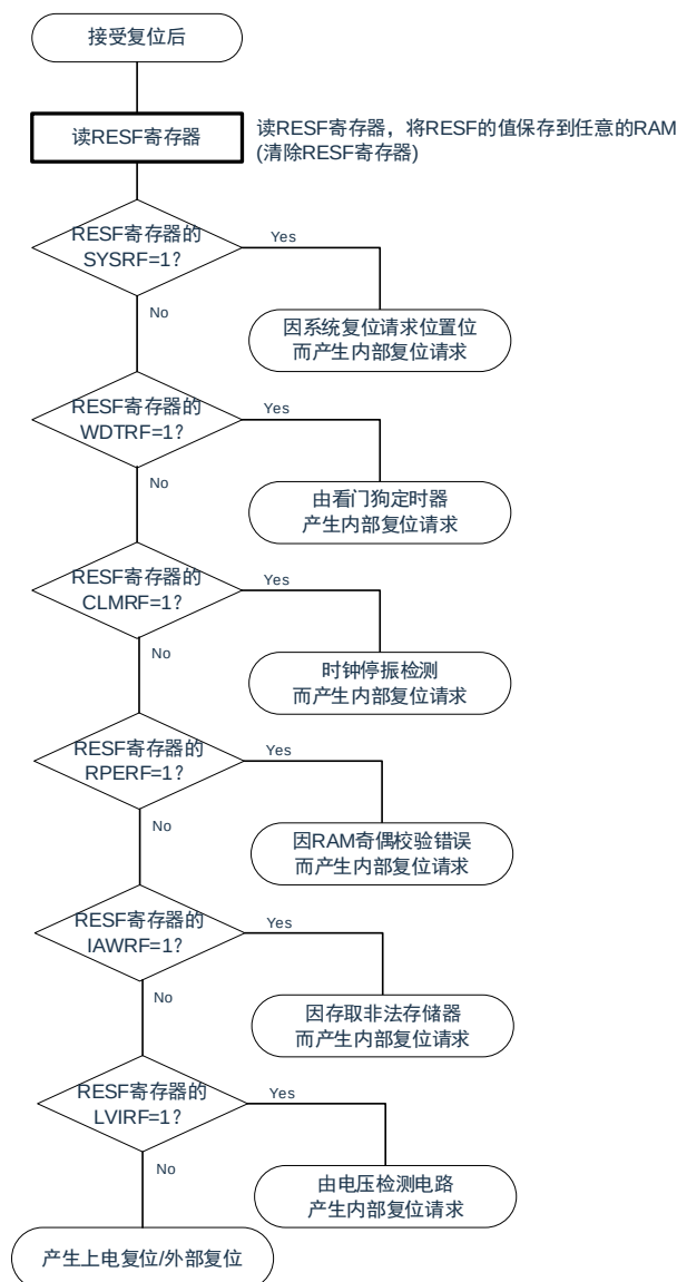
图 27-5：复位源的确认步骤
