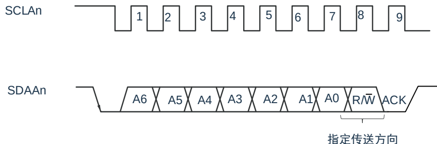
图18-17：应答
