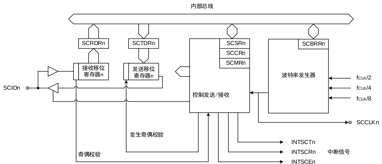
图 20-1 SMCI的框图
