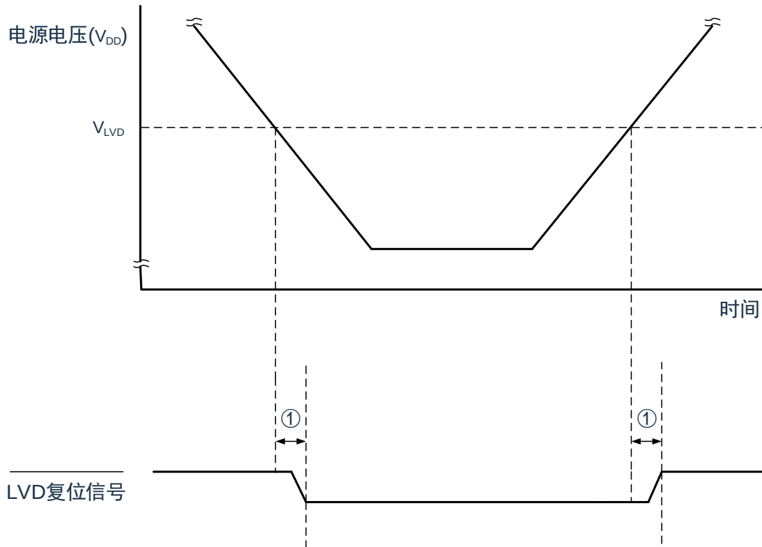
图 29-10: 从产生LVD复位源到产生或者解除LVD复位的延迟
