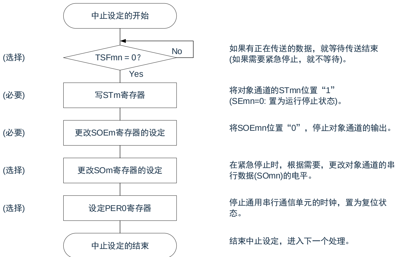
图16-74：从属发送的中止步骤
