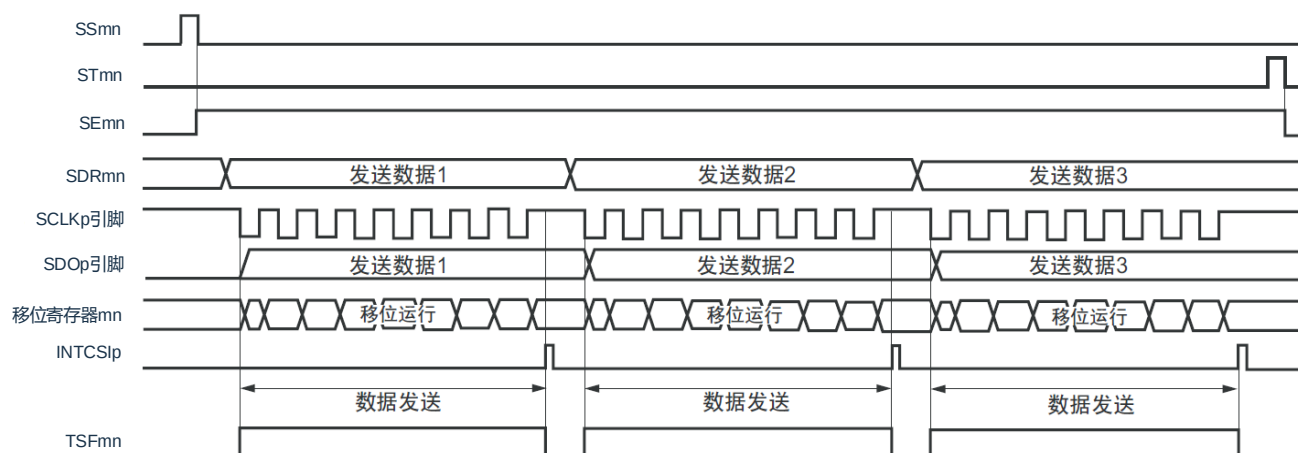
图16-27：主控发送（单次发送模式）的时序图（类型1：DAPmn=0、CKPmn=0）
