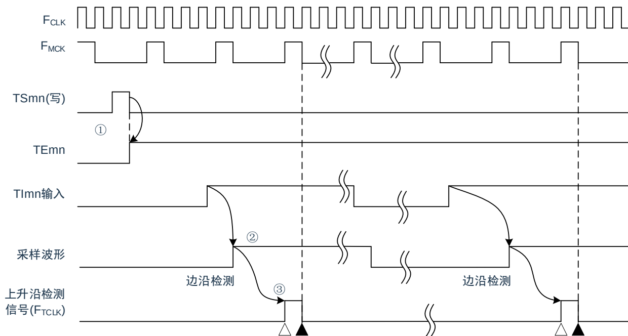
图5-23: 计数时钟 ( F_{TCLK} ) 的时序 (CCSmn=1, 未使用噪声滤波器的情况)
