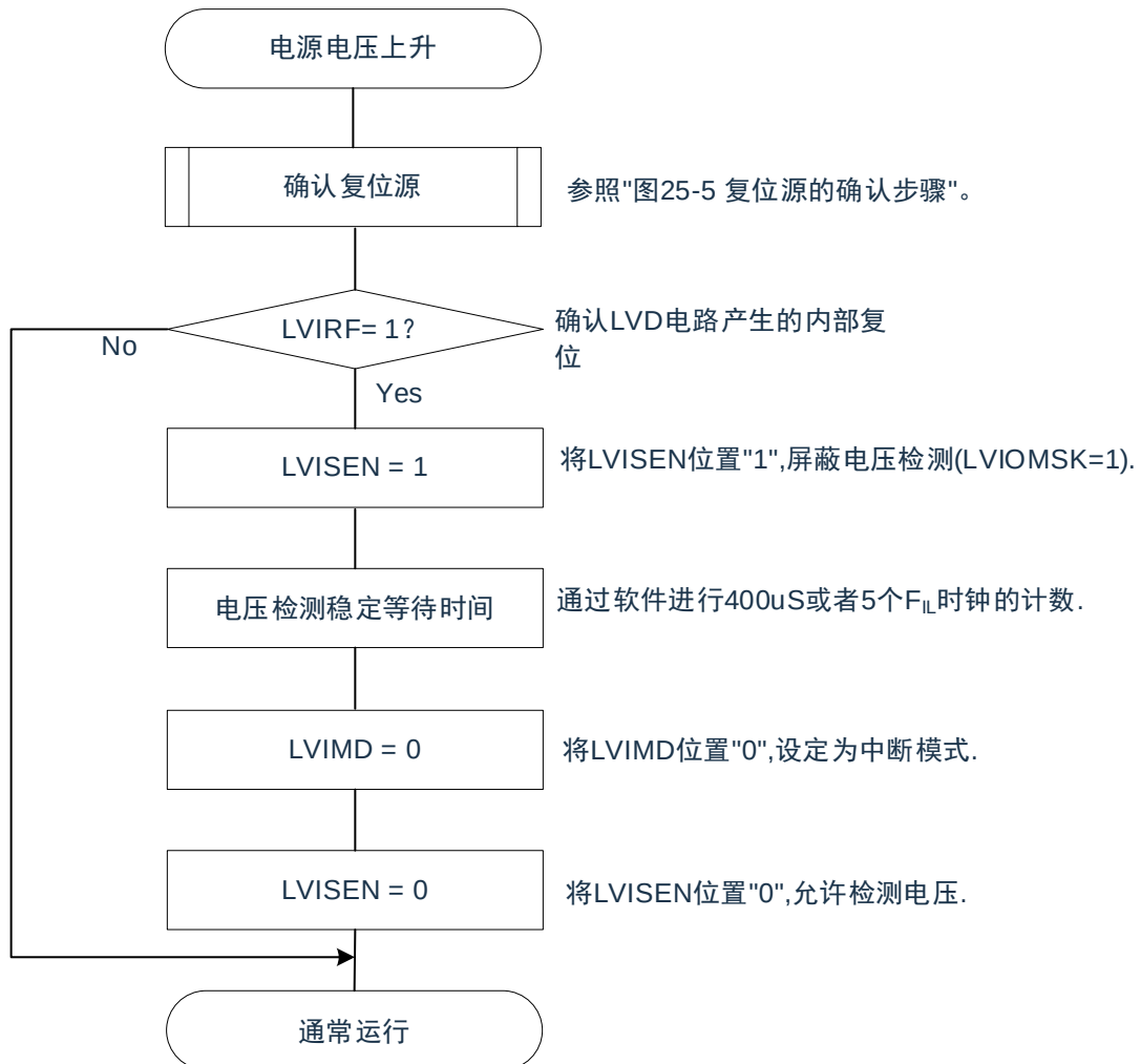
图 29-8：中断&复位模式的初始设置步骤
