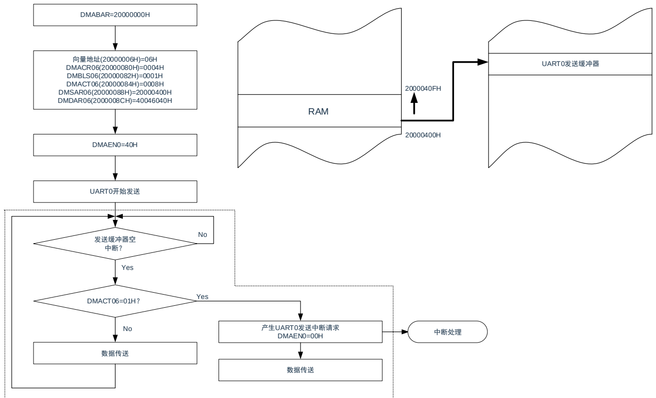
图22-18：正常模式的使用例子2：UART0连续发送
