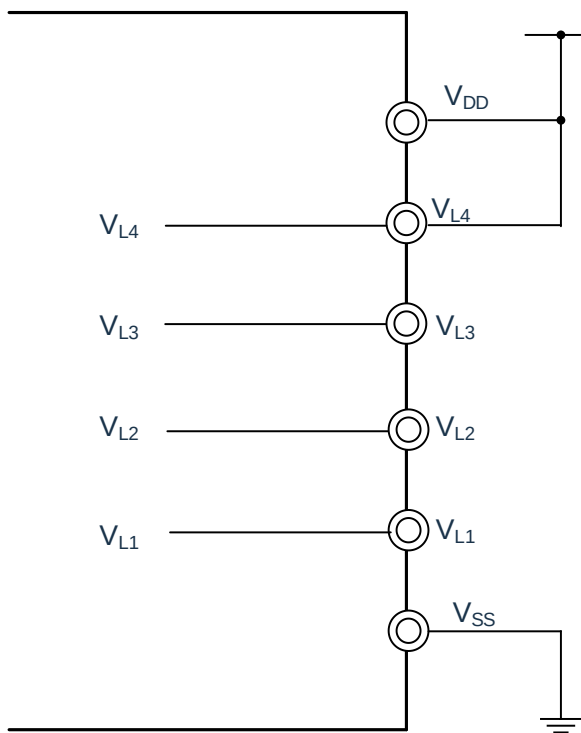
图 21-11：LCD驱动电源的连接例子（内部电阻分割方式）
