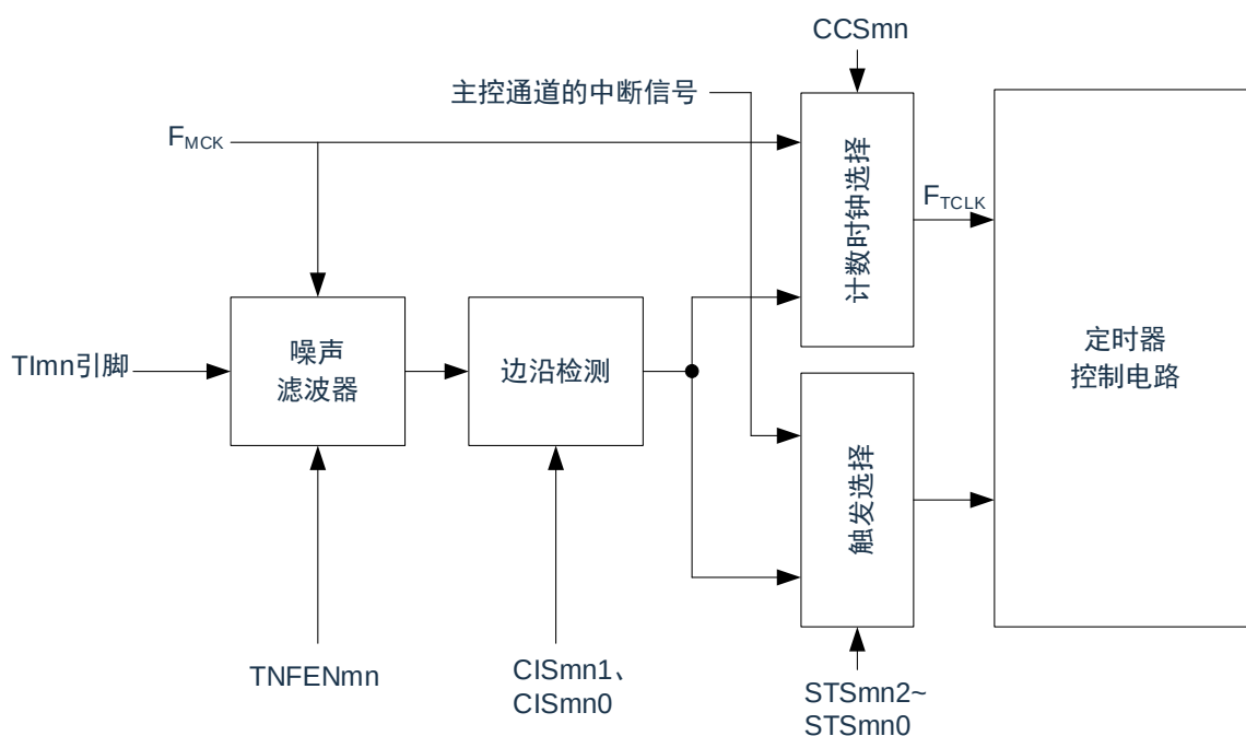
图5-38：输入电路的结构
