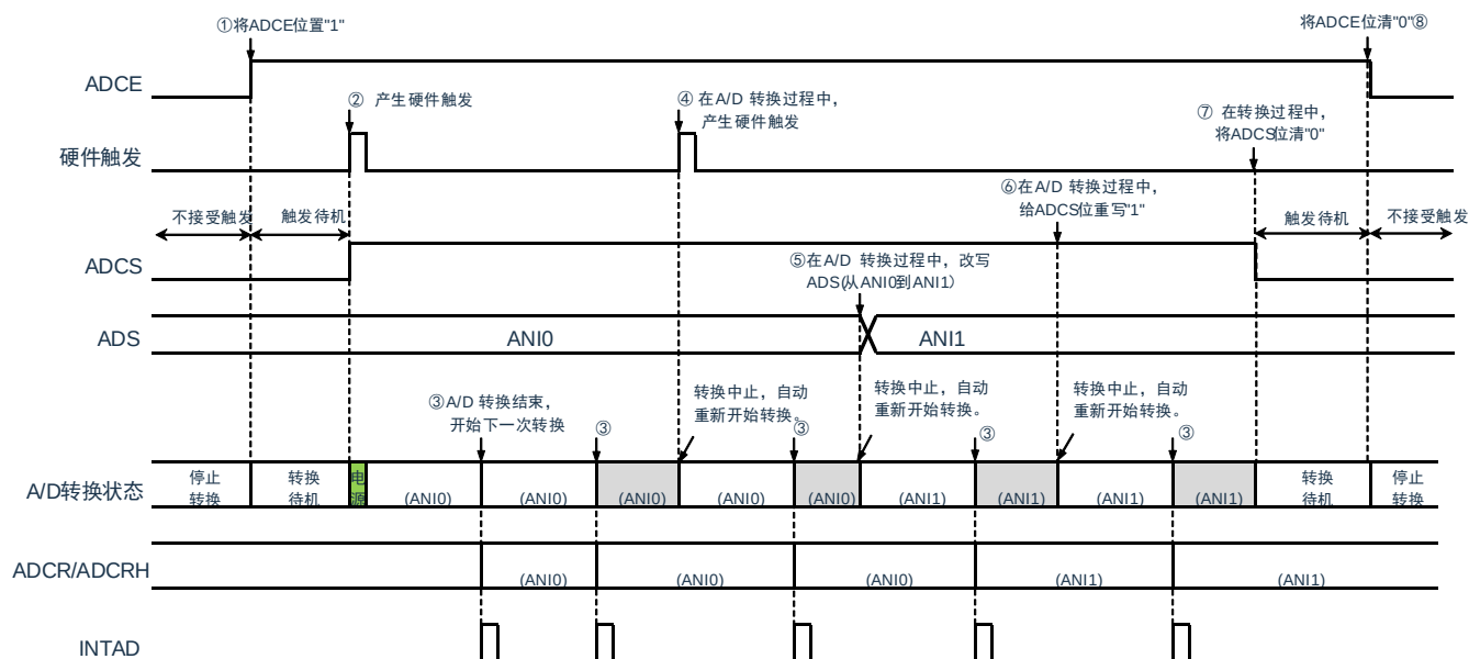
图11-27：硬件触发等待模式（选择模式、连续转换模式）的运行时序例子
