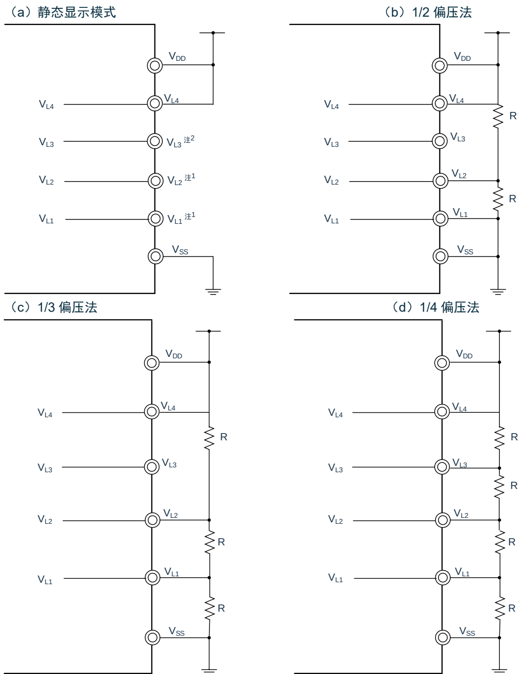
图 21-12: LCD驱动电源的连接例子（外部电阻分割方式）
