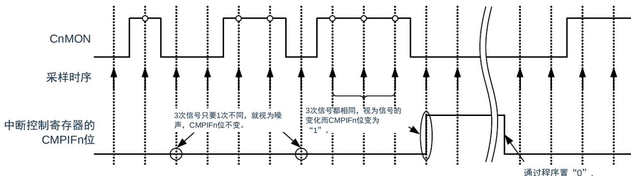
图13-12：比较器n（n=0、1）的数字滤波器和中断运行示例
