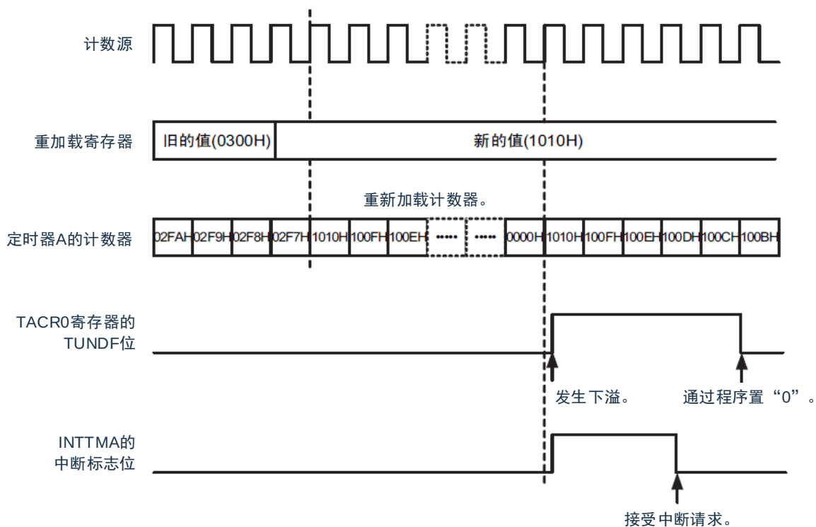
图 6-10：定时器模式的运行例子
