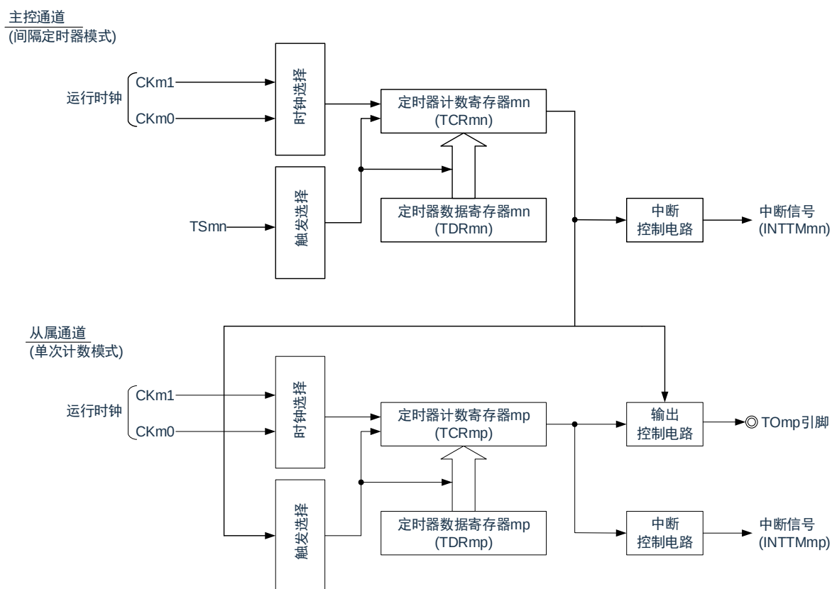
图5-65：作为PWM功能运行的框图
