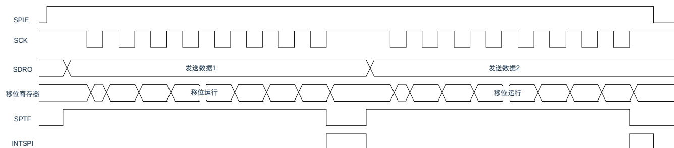
图17-16: 发送/接收时序(单次发送模式)的时序图 (INTMD=0,CPHA=1、CPOL=1)
