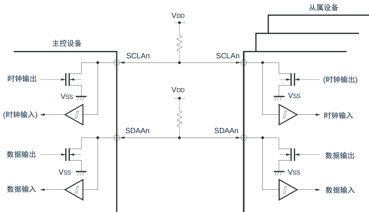
图18-12：引脚结构图
