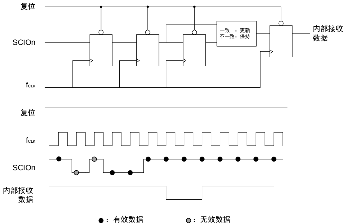
图 20-15 噪声滤波器电路和时序图
