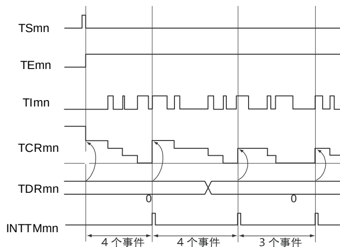
图5-44：作为外部事件计数器运行的基本时序例子
