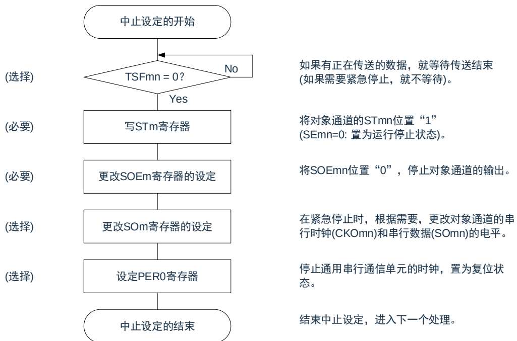
图16-33: 主控接收的中止步骤
