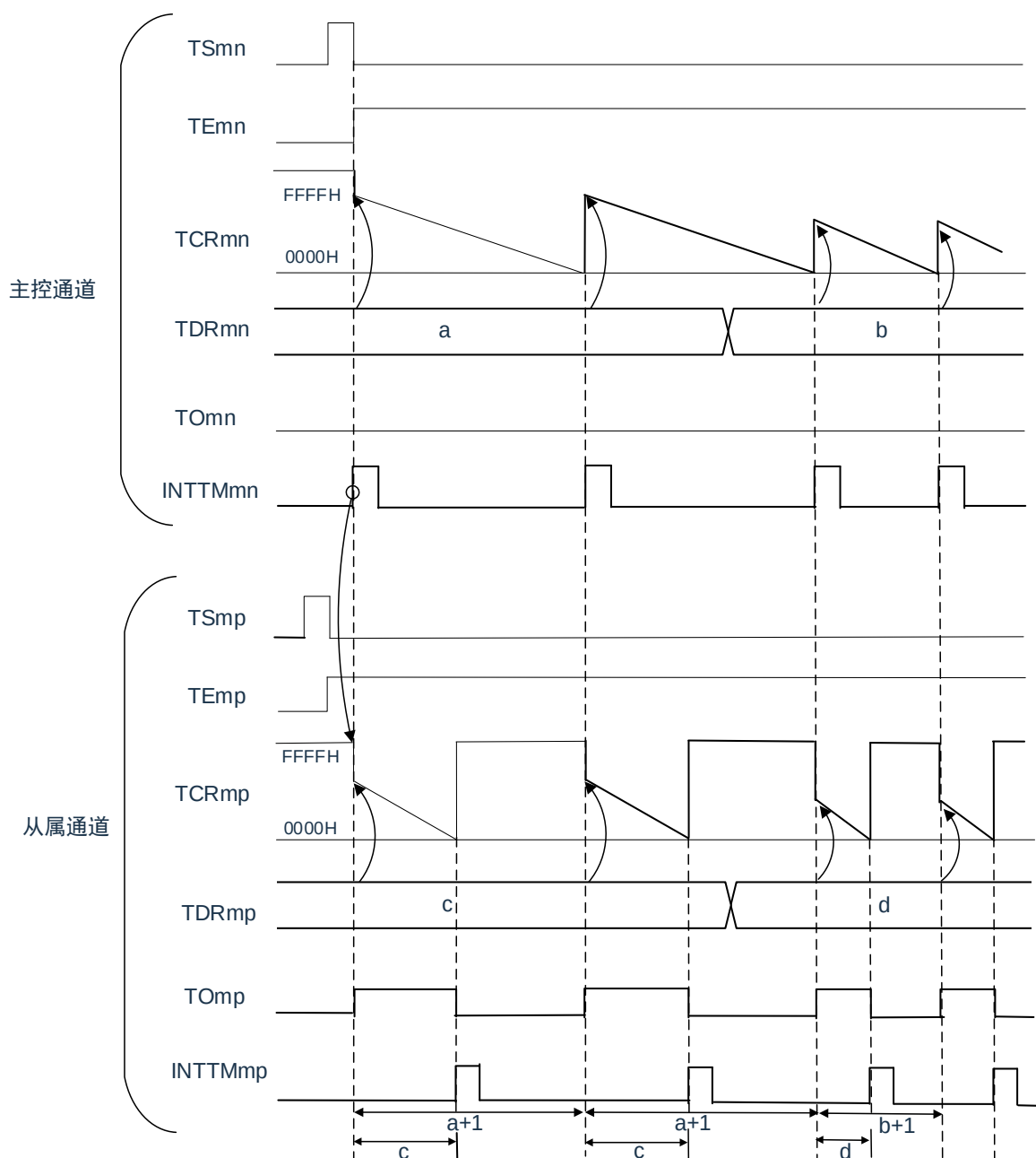
图5-66：作为PWM功能的运行基本时序例子
