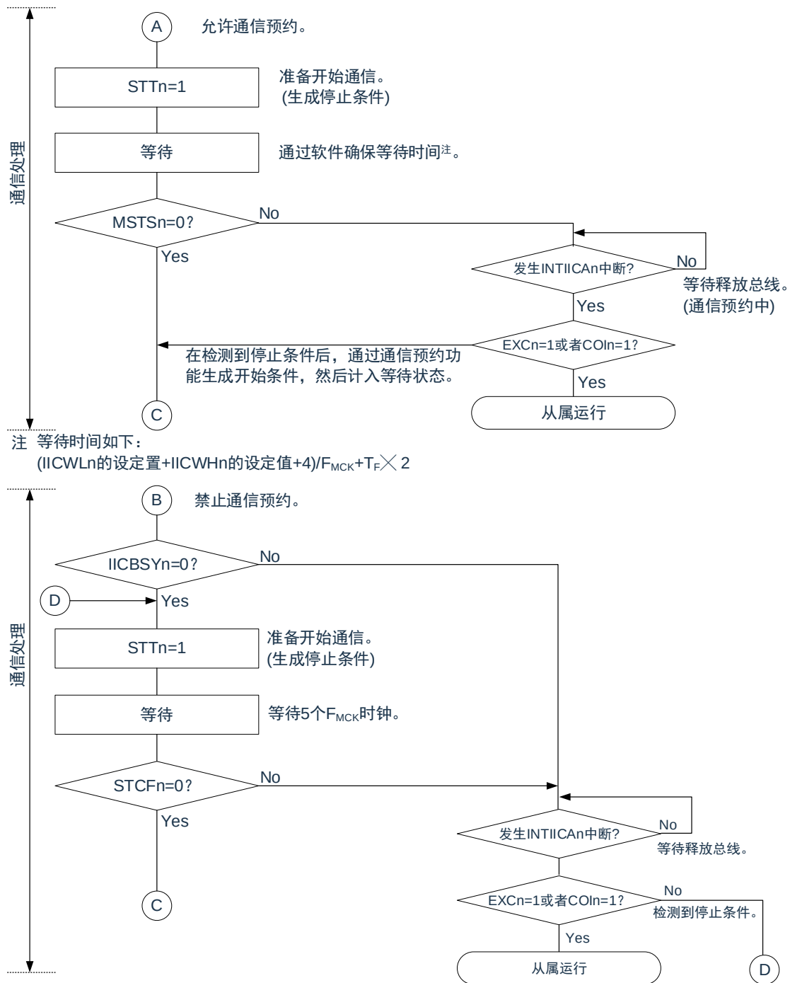
图18-28：多主控系统的主控运行(2/3)
