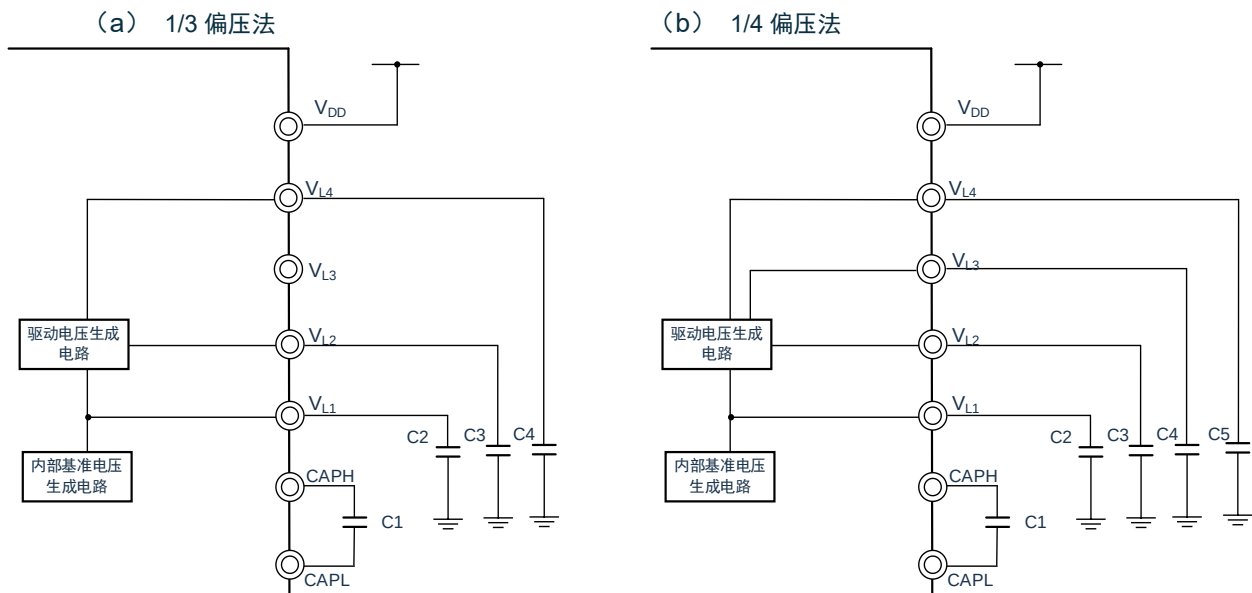
图 21-13: LCD 驱动电源的连接例子（内部升压方式）
