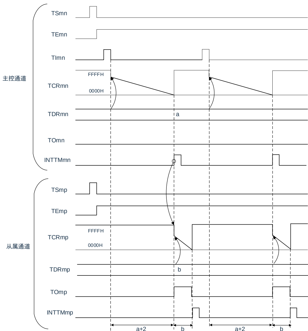
图5-60：作为单触发脉冲输出功能的运行基本时序例子
