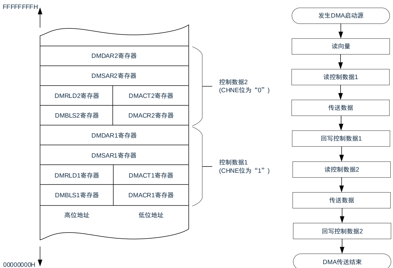
图22-21：链传送的流程图
