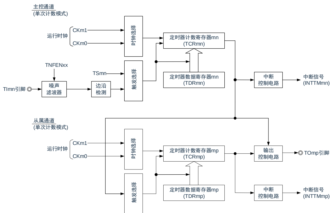
图5-59：作为单触发脉冲输出功能运行的框图
