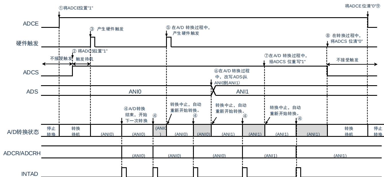
图11-23：硬件触发无等待模式（选择模式、连续转换模式）的运行时序例子
