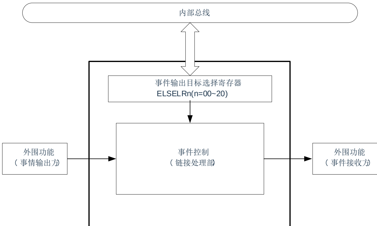
图21-1：EVENTC的框图
