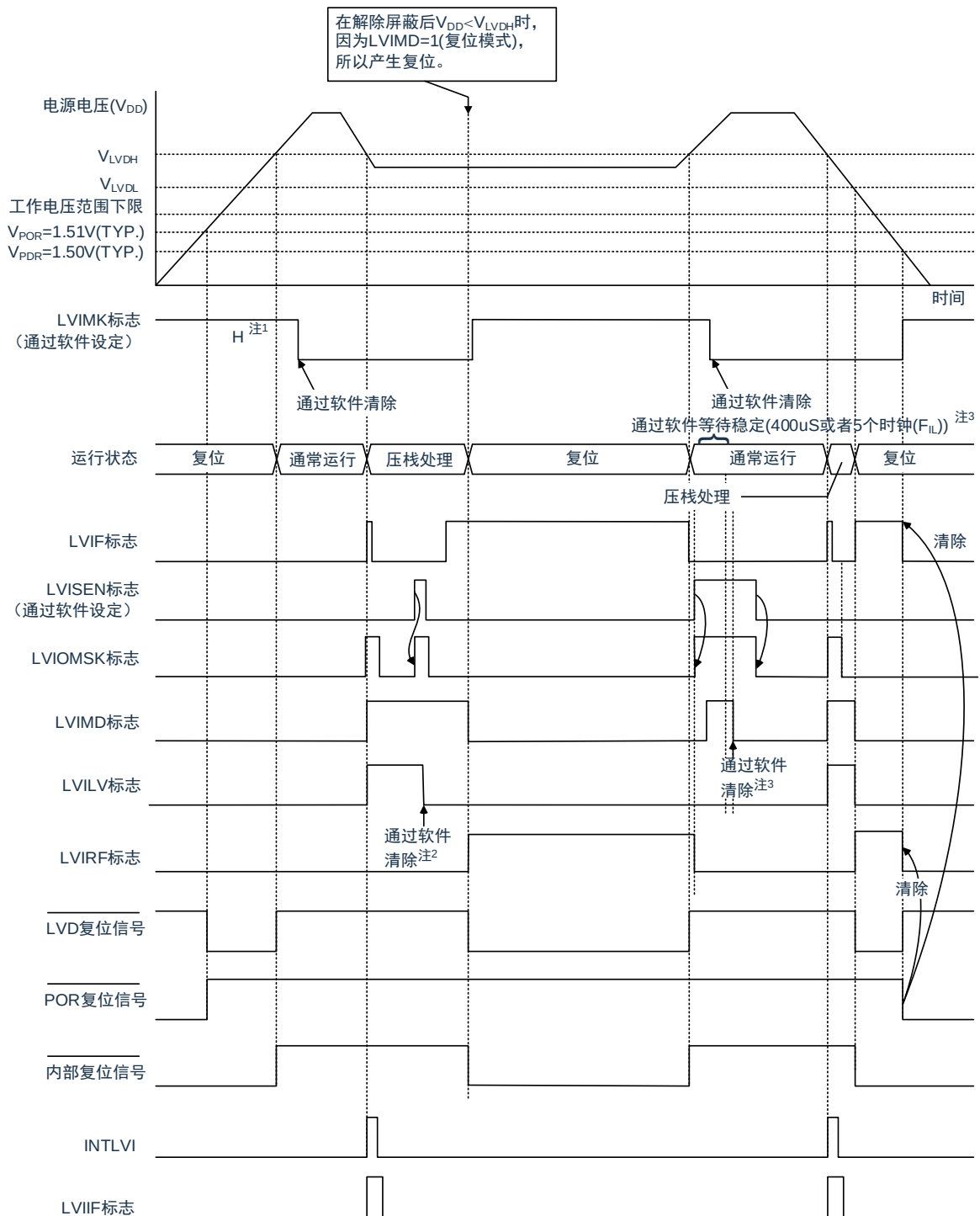
图29-6：中断&复位信号的产生时序（选项字节的LVIMDS1、LVIMDS0=1、0）(2/2)
