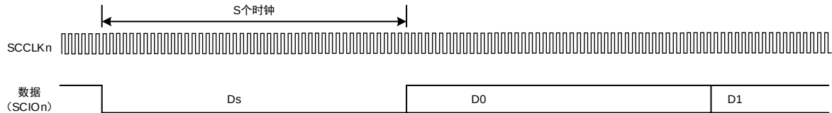
图 20-23 输出时钟和发送数据的相位关系 (SCBCP2 ~ SCBCP0=100B、 S=32 的例子)
