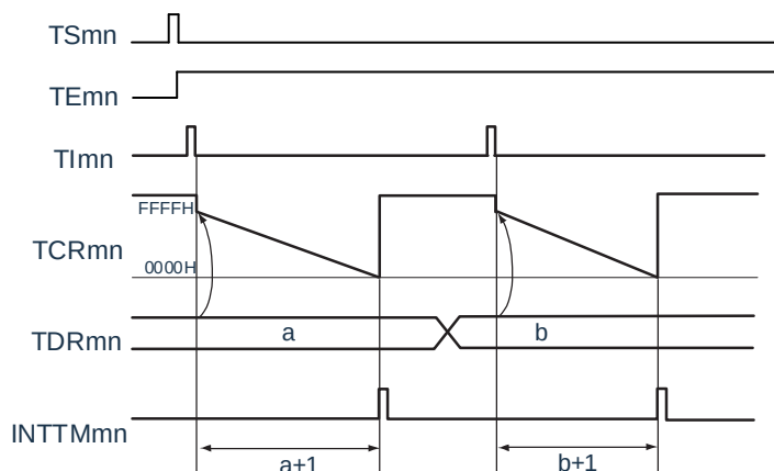
图5-56：作为延迟计数器的运行基本时序例子
