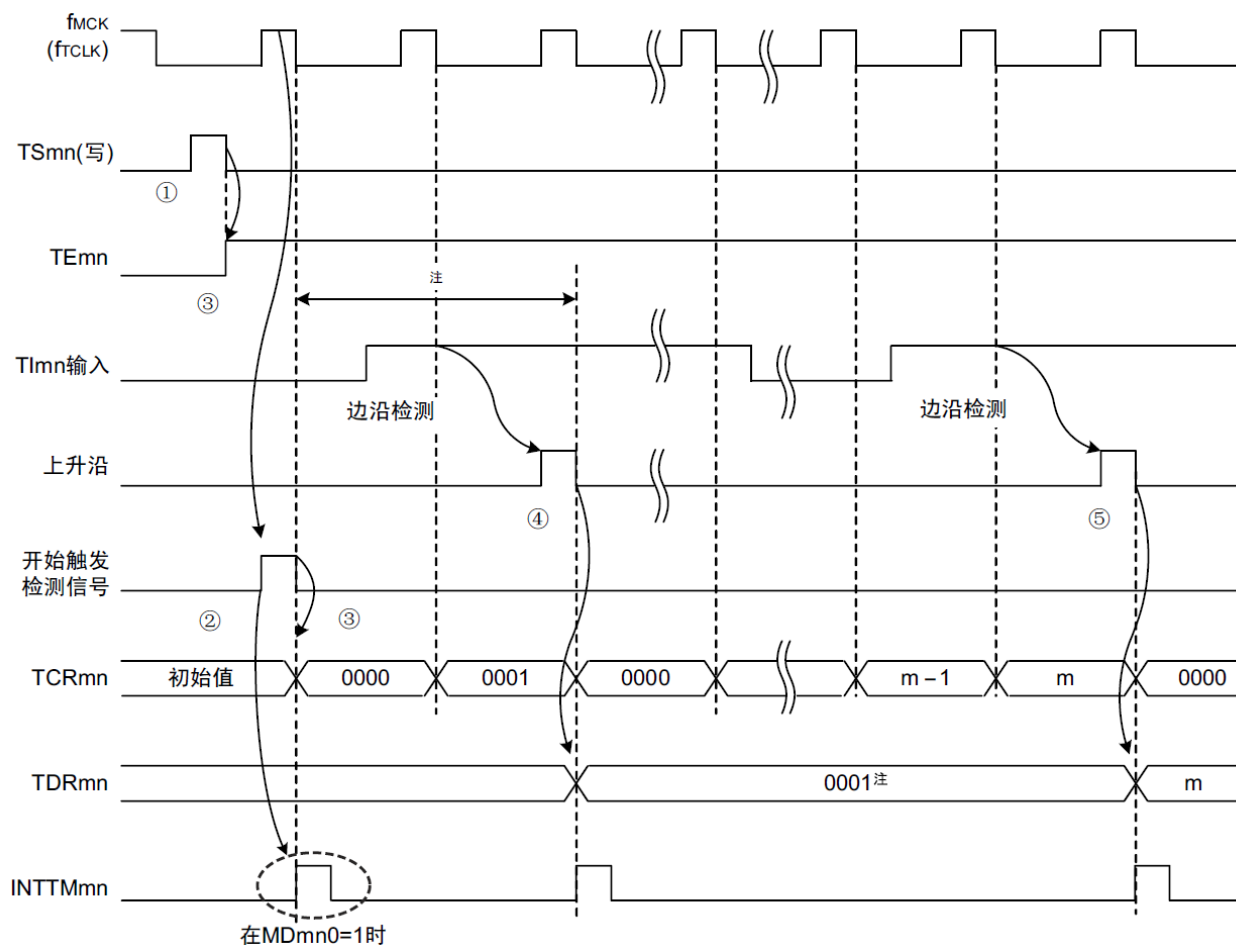
图5-26：运行时序（捕捉模式：输入脉冲的间隔测量）
