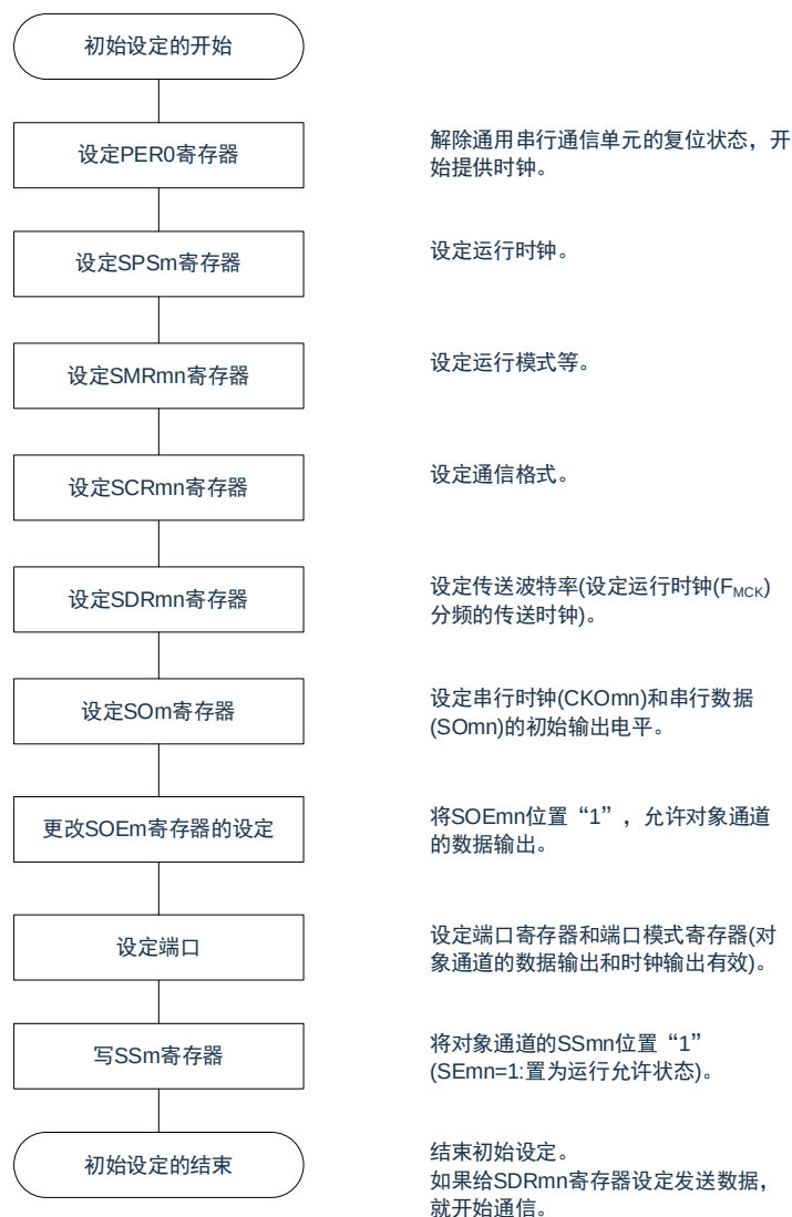
图16-40：主控发送和接收的初始设定步骤
