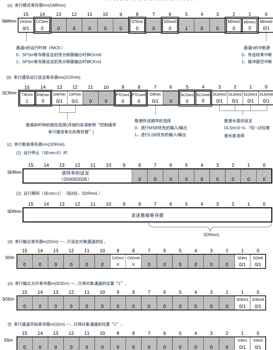
图16-47：3线串行I/O（SSPlmn）
