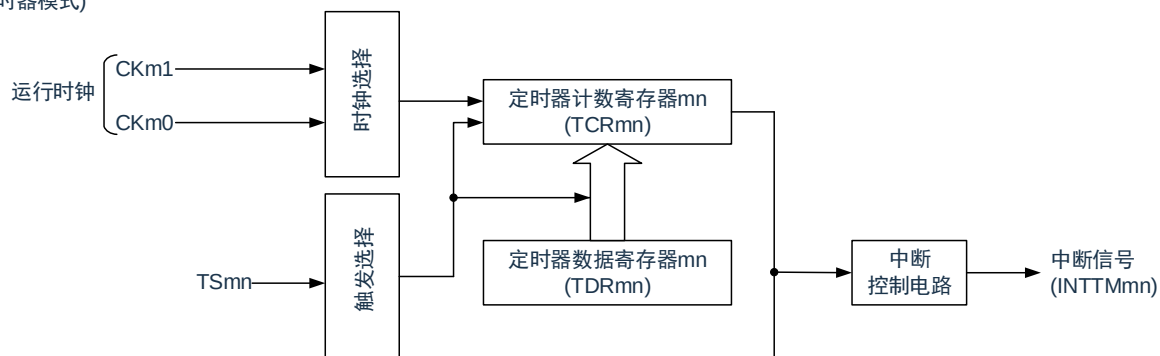
图5-71：作为多重PWM输出功能运行的框图（输出2种PWM的情况）
