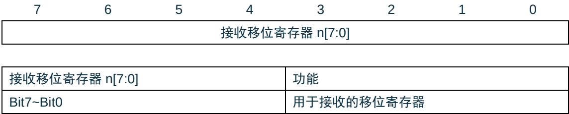
图 20-2 接收移位寄存器的格式
