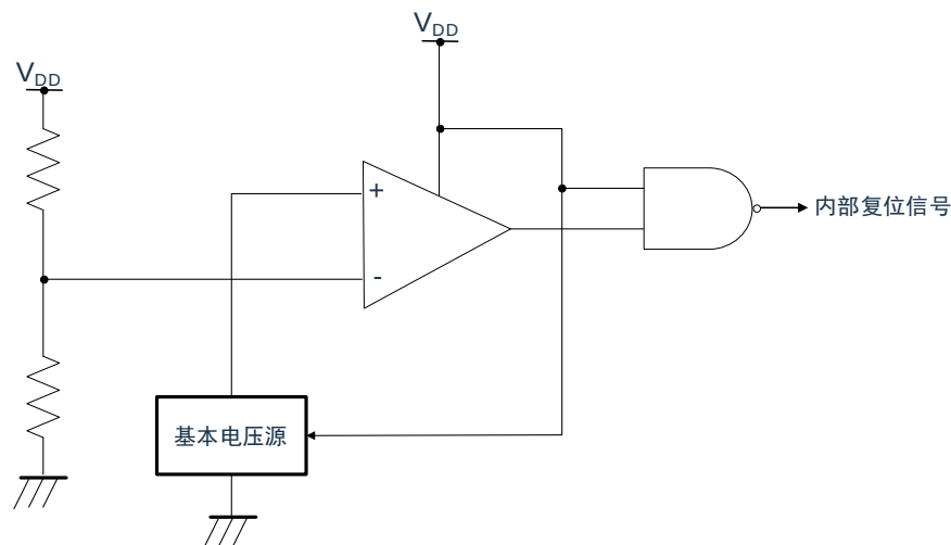
图 28-1：上电复位电路的框图
