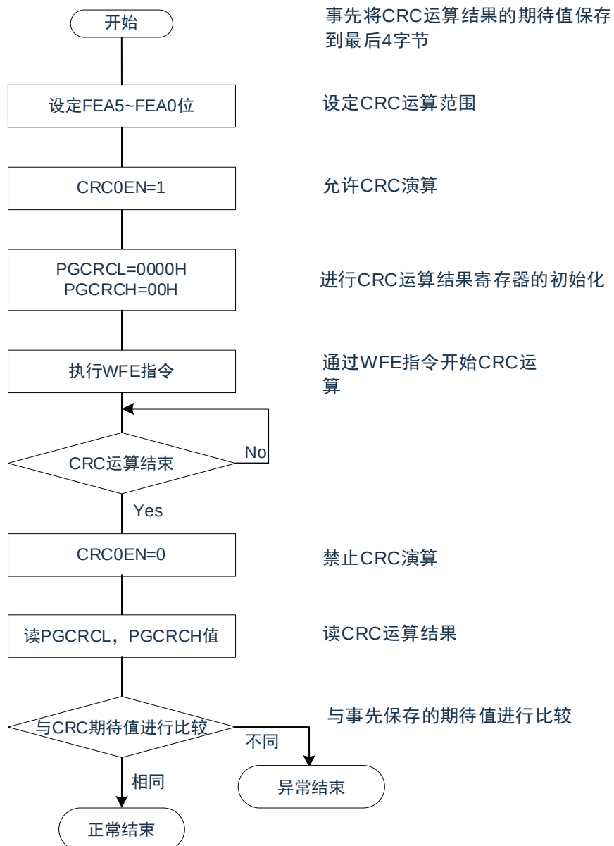
图30-3：闪存CRC运算功能（高速CRC）的流程图
