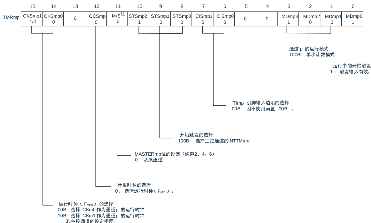
图5-68: PWM功能时（从属通道）的寄存器设定内容例子
