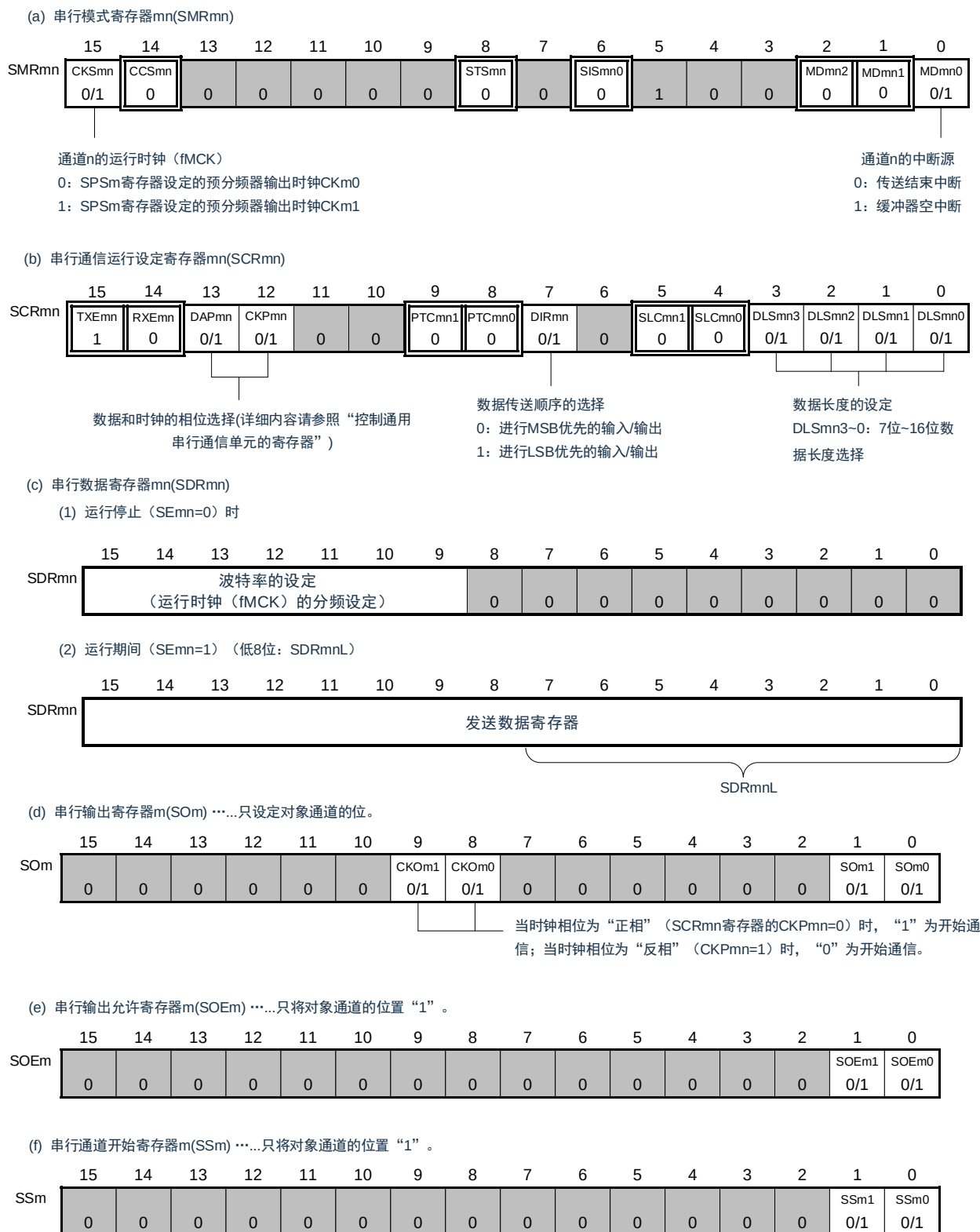
图16-23: 3线串行I/O (SSPlmn)
