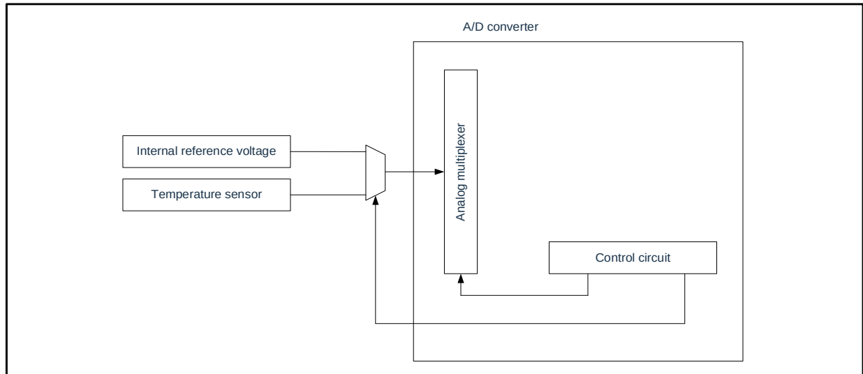
图 31-1：温度传感器框图
