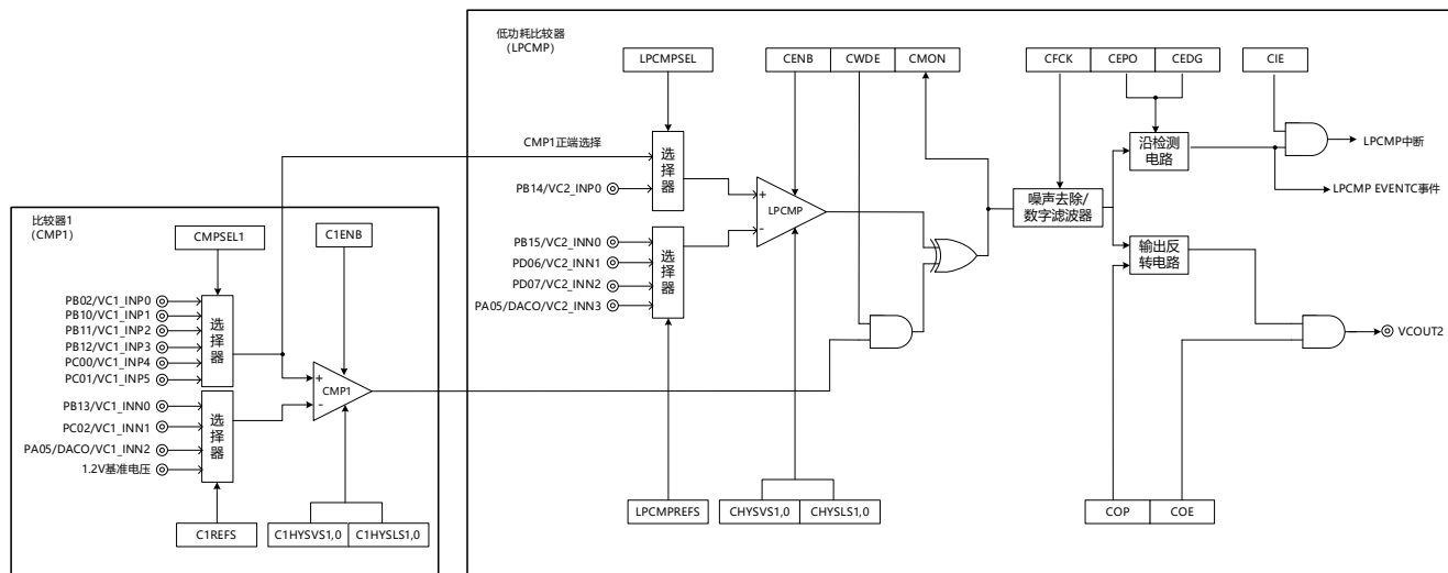
图 14-1：低功耗比较器的框图
