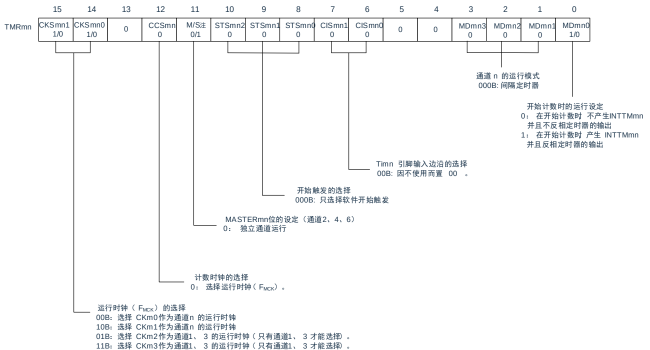
图5-42：间隔定时器/方波输出时的寄存器设定内容例子
