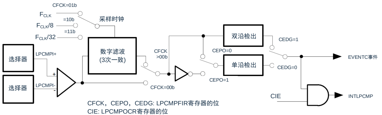
图14-10：低功耗比较器的数字滤波器和沿检出结构
