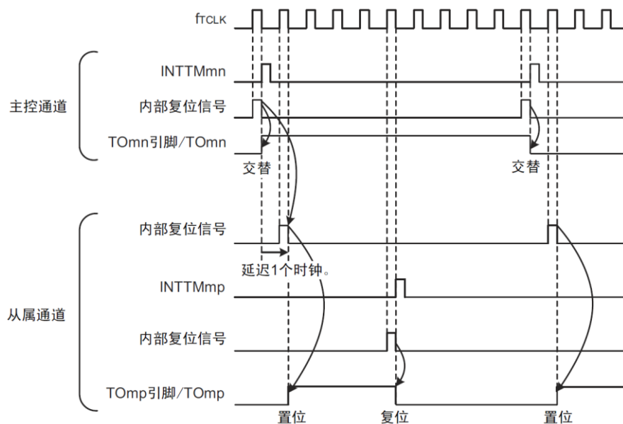
图5-34：置位/复位时序运行状态
