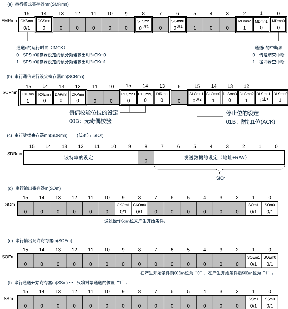
图16-122：简易I 2 C（IICmn）地址段发送时的寄存器设定内容例子
