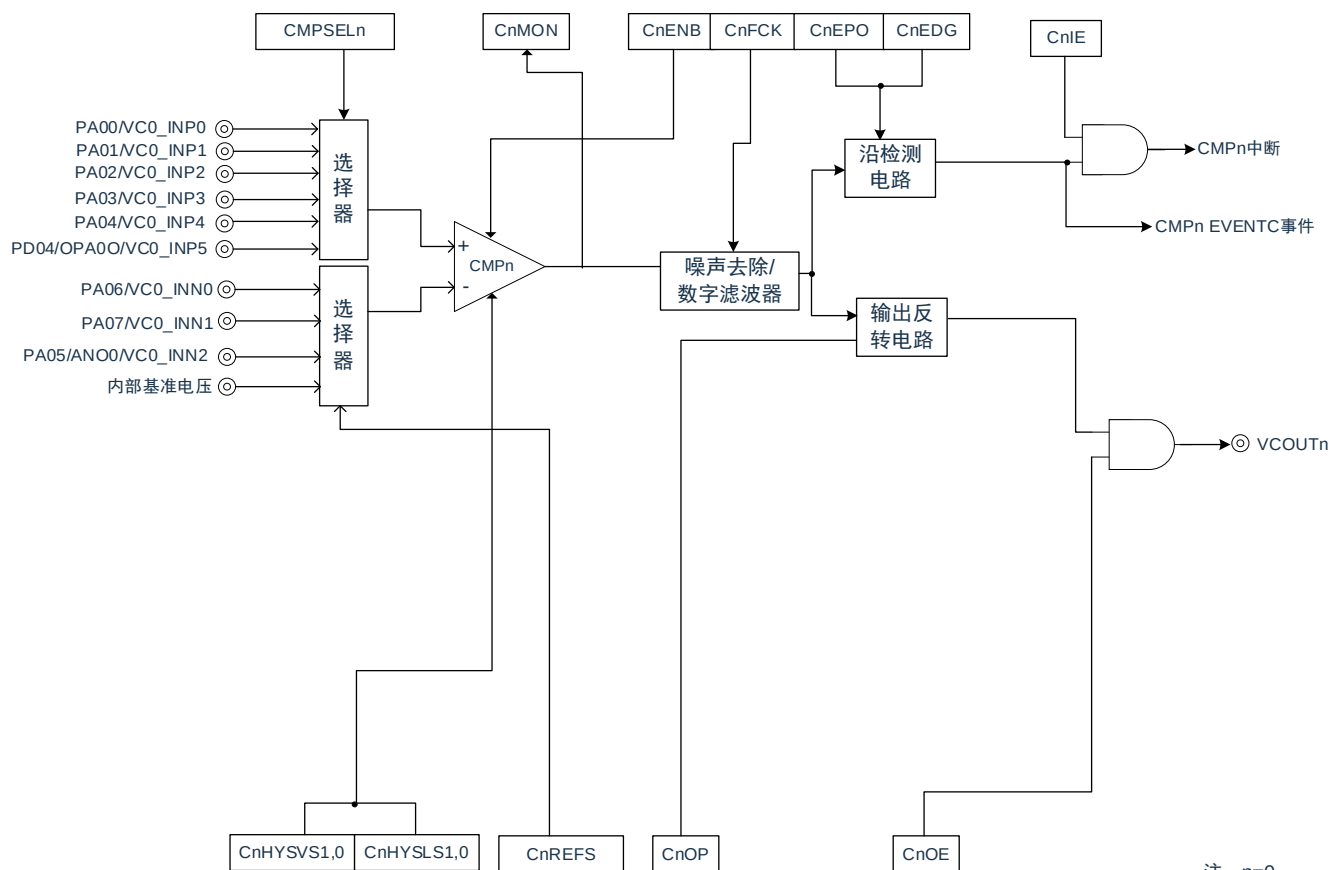
图13-1：比较器0的框图
