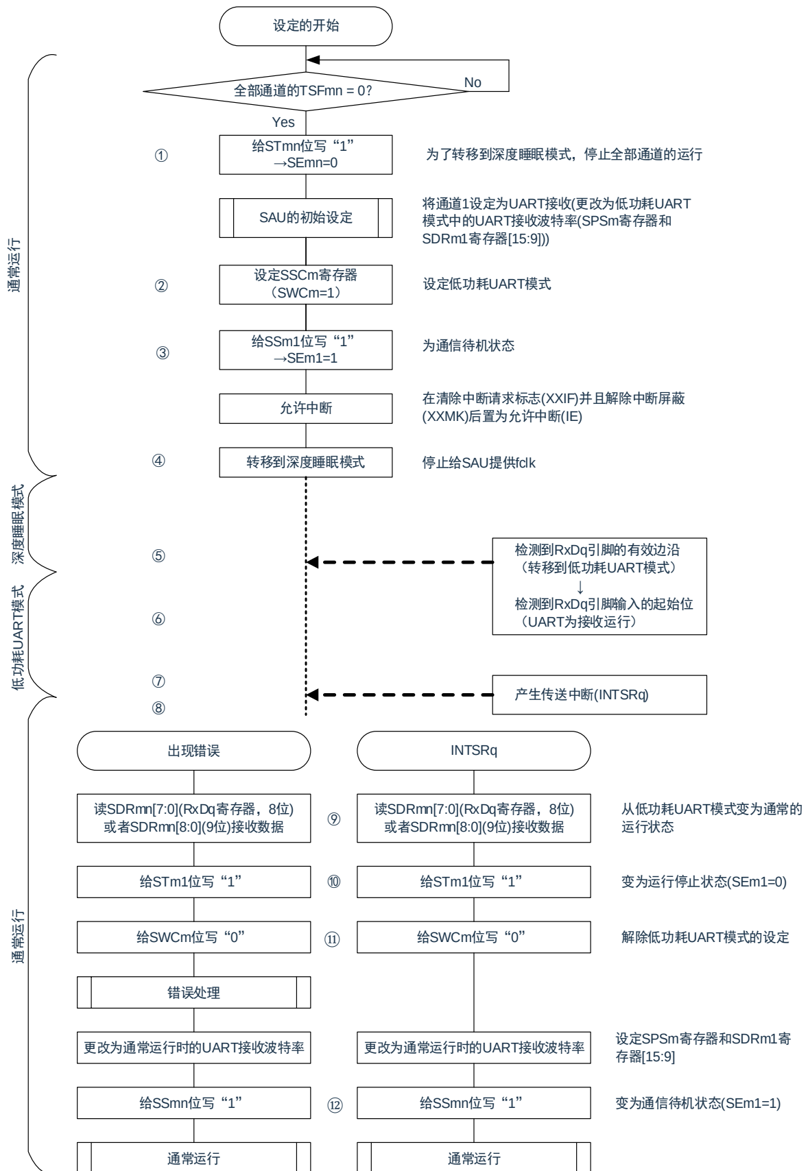
图 16-111: 低功耗UART模式运行 (SSECm=0/1) 的流程图
