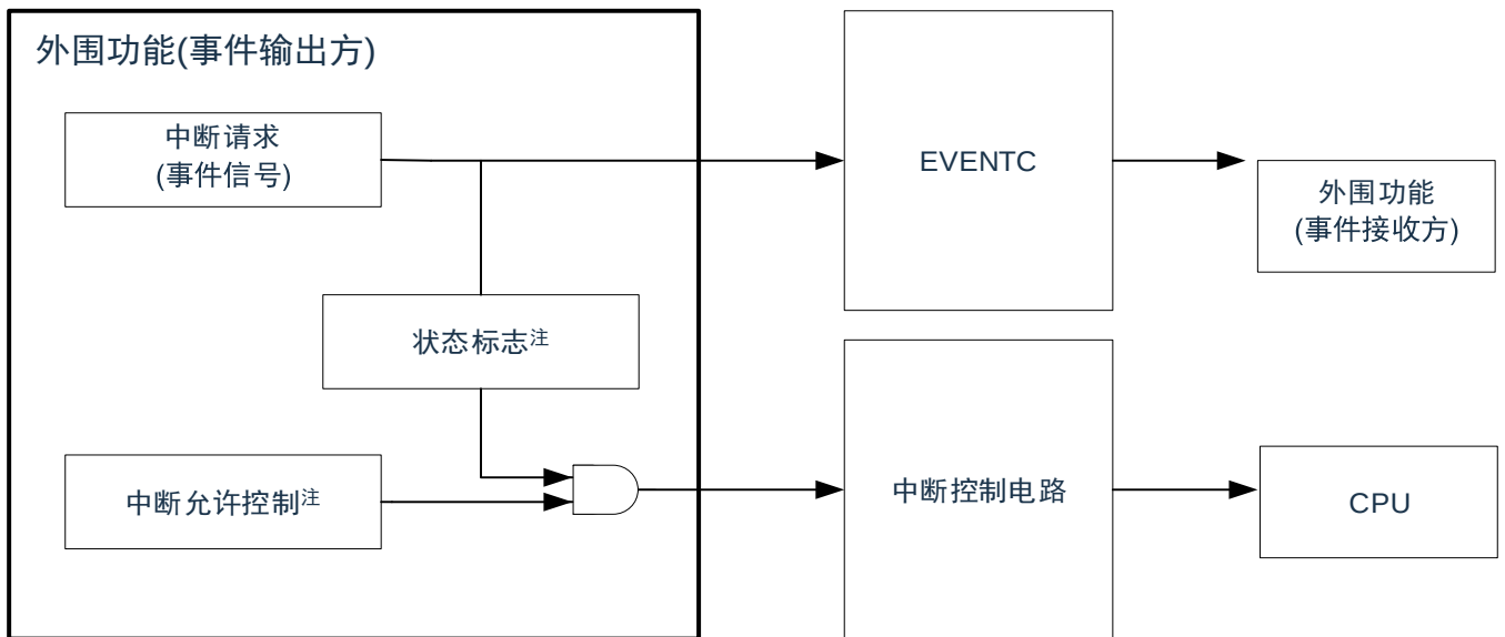
图23-3：中断处理和EVENTC的关系
