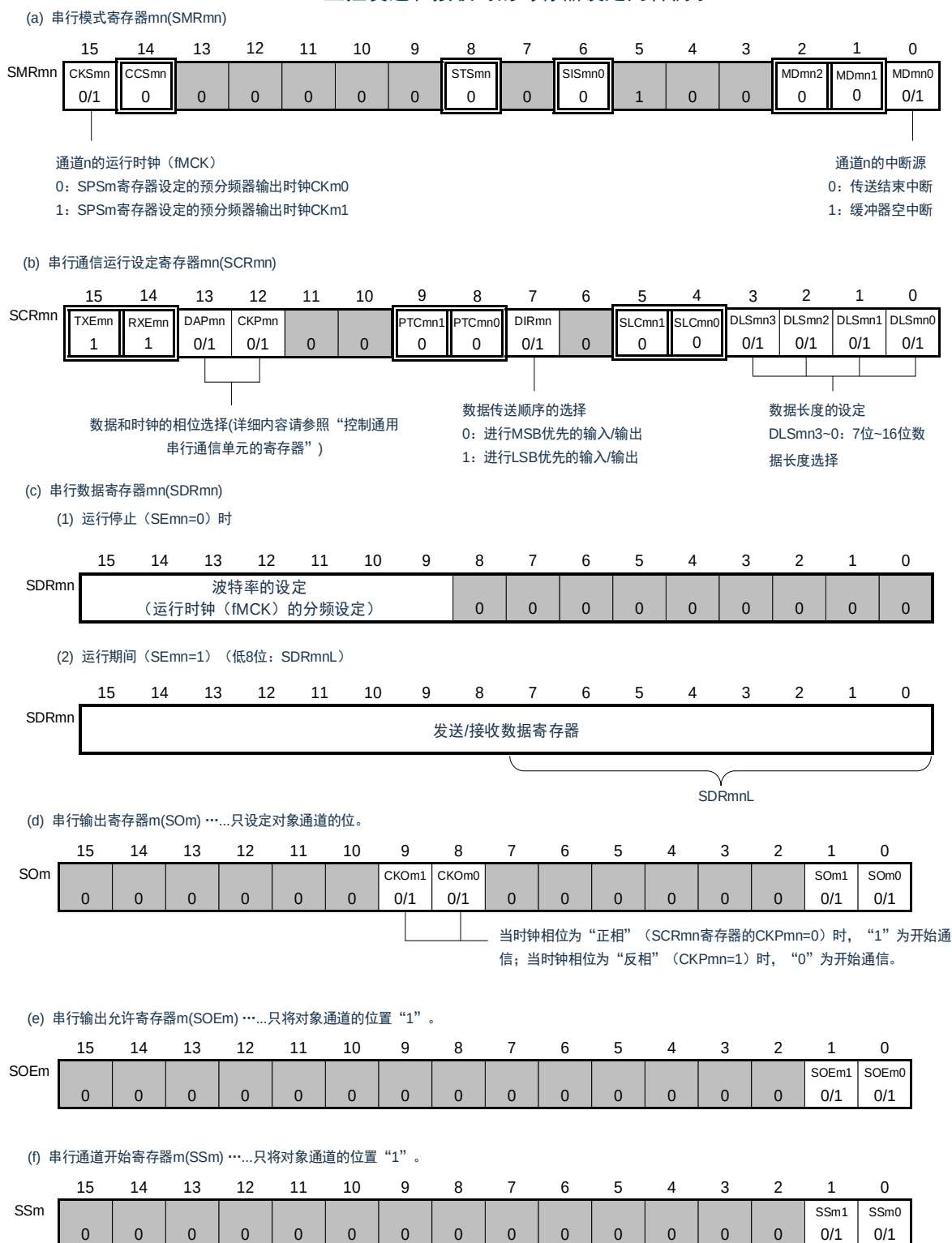
图16-39：3线串行I/O（SSPlmn）
