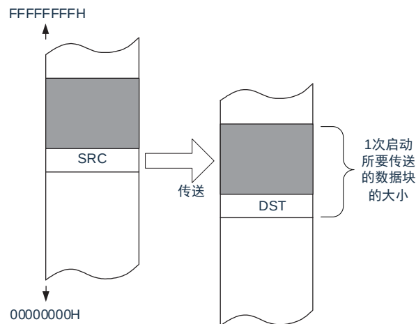
图22-19：重复模式的数据传送
