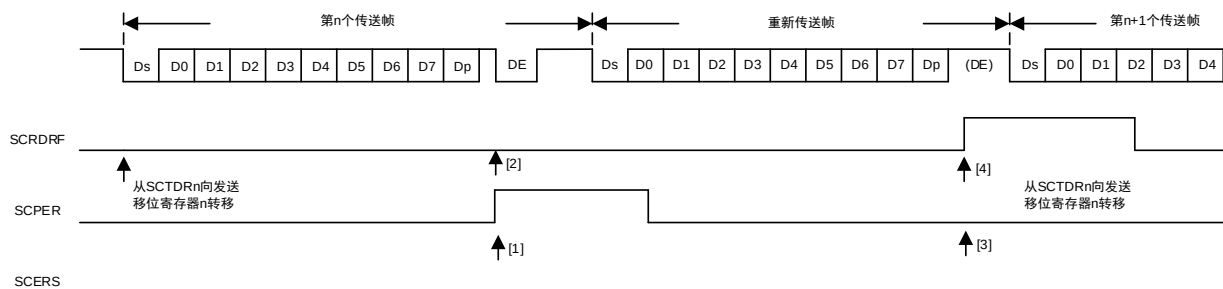
图 20-21 SMCI 接收模式中的重新传送运行
