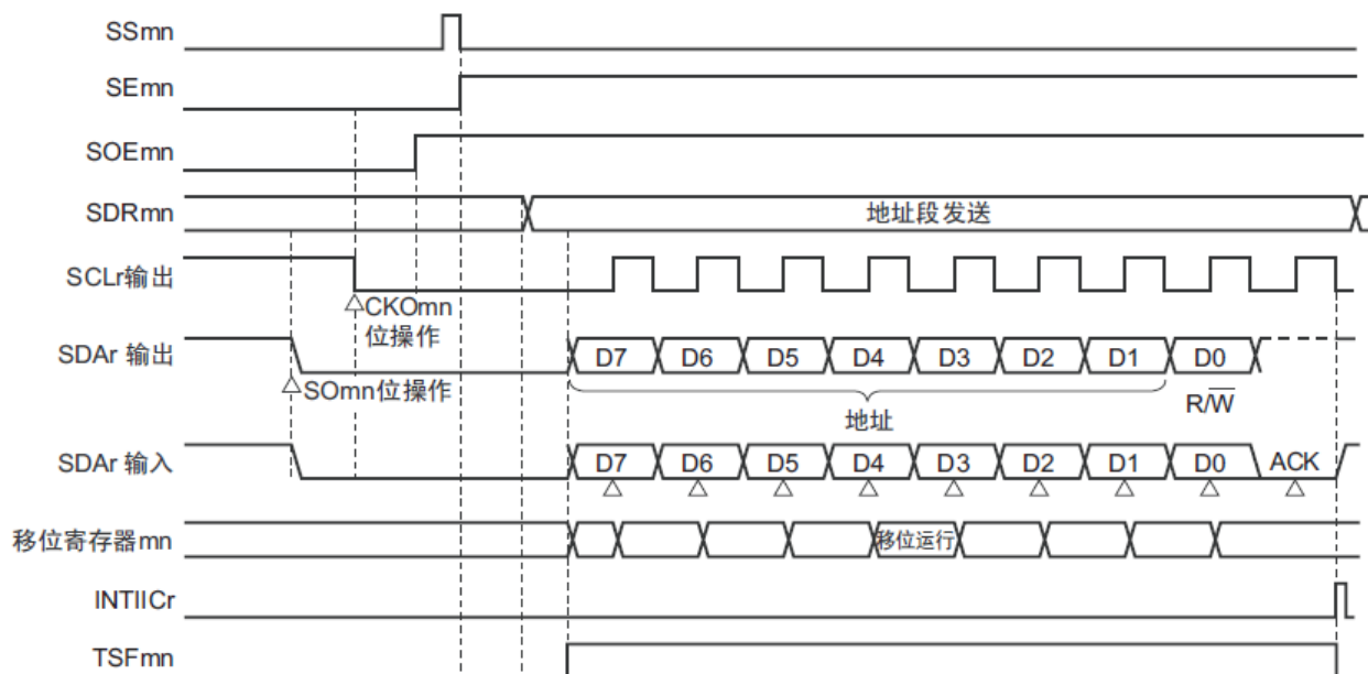
图16-124：地址段发送的时序图
