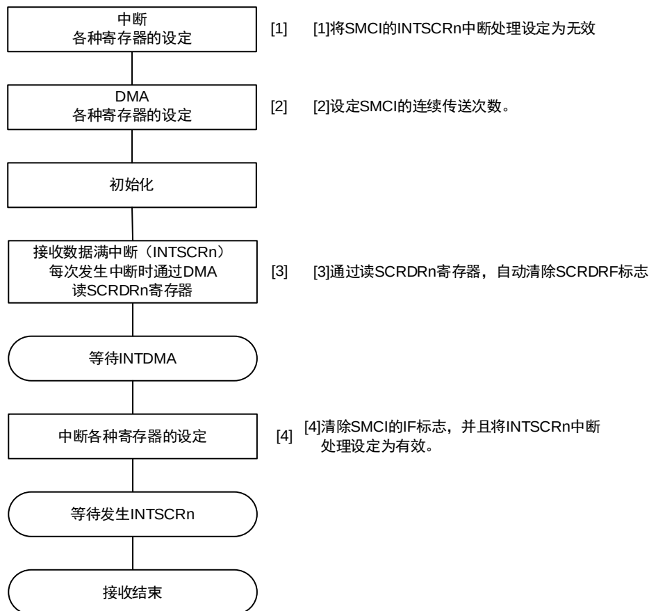
图 20-28使用DMA进行连续数据接收的流程
