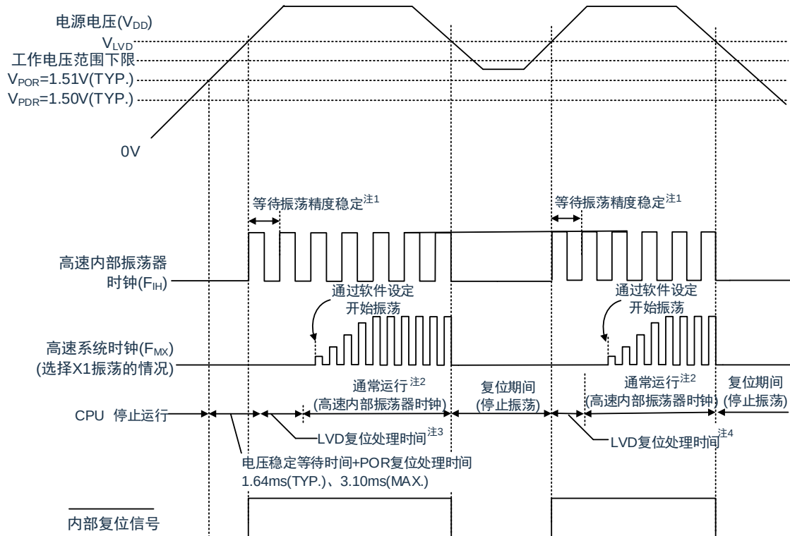
图 28-4：上电复位电路和电压检测电路的内部复位信号的产生时序(3/3)
