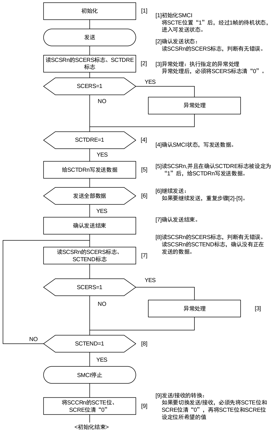
图 20-20 发送流程图的例子
