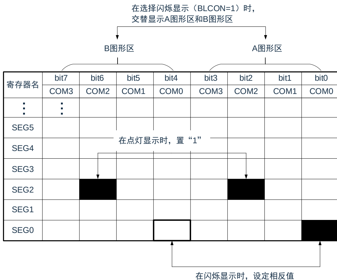
图 21-8：图形切换显示时的 LCD显示寄存器的设定例子
