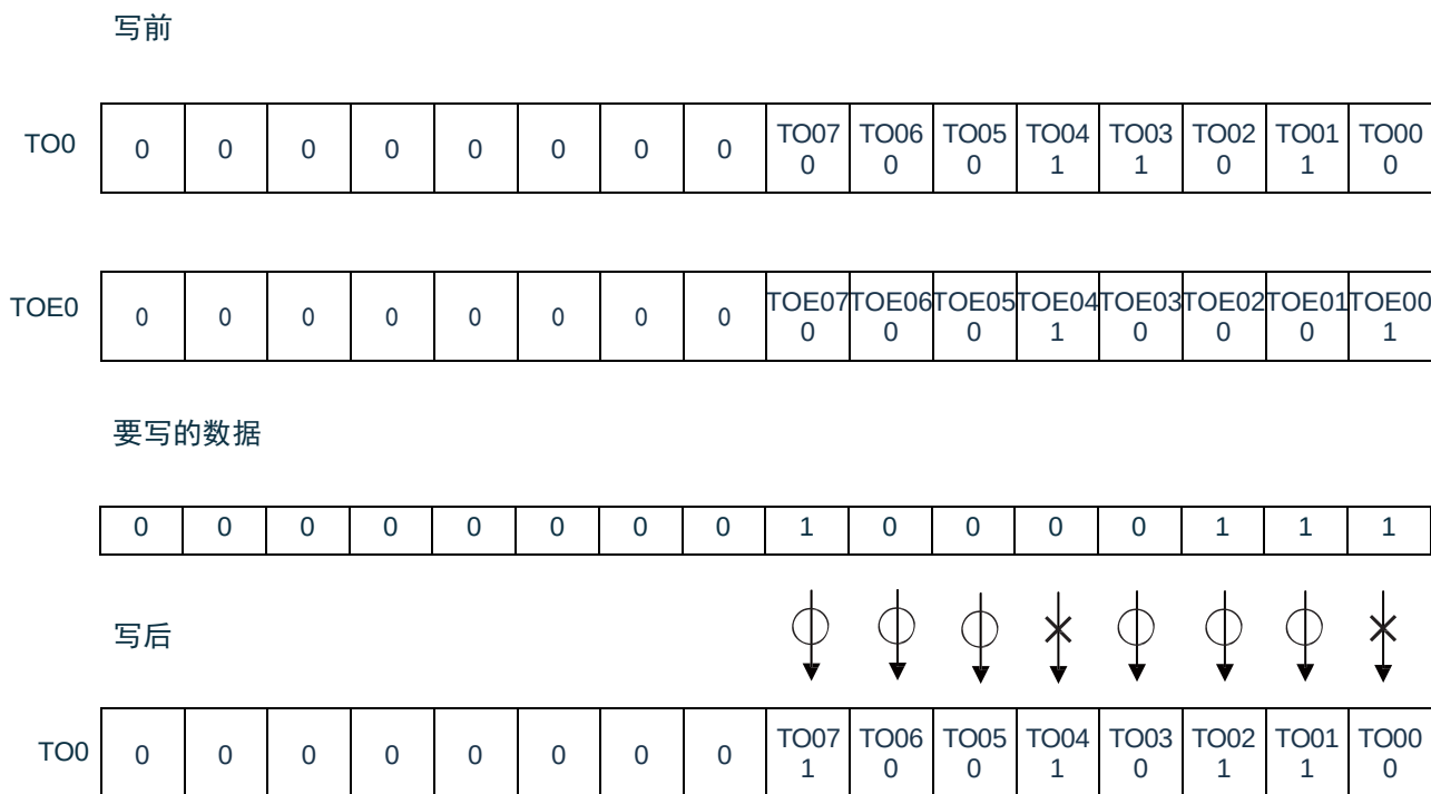
图5-35: TO0n位的一次性操作例子
