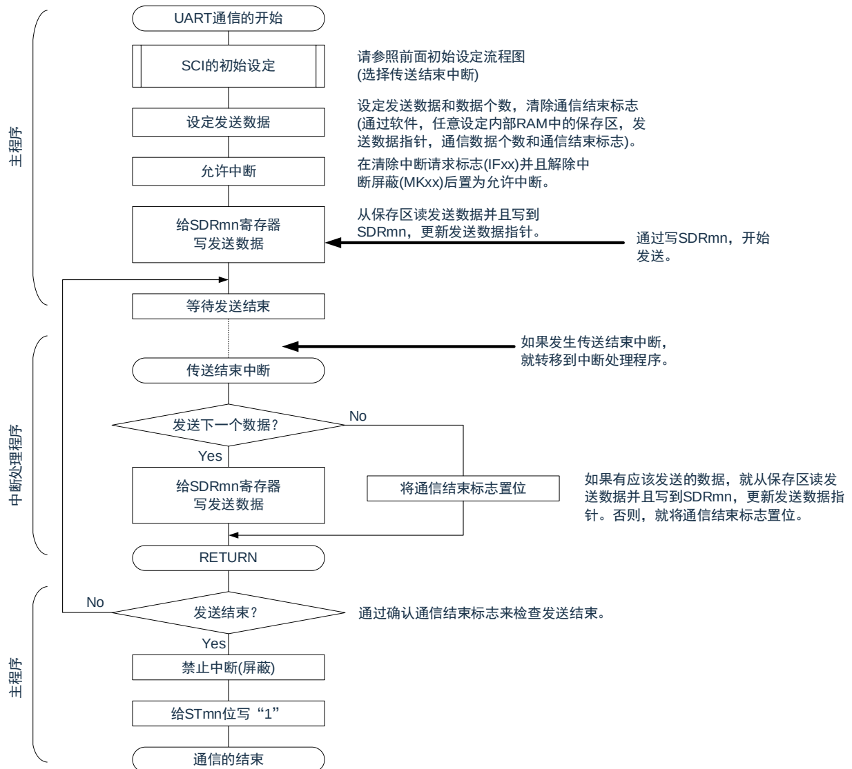
图16-101: UART发送（单次发送模式）的流程图
