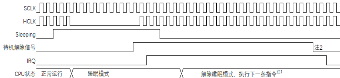
图26-1：通过中断请求解除睡眠模式
