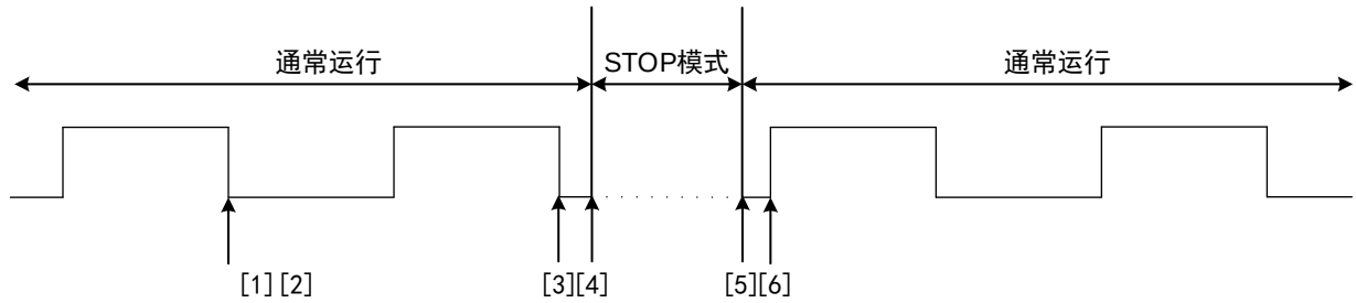
图 20-25 时钟停止和重新启动的步骤
