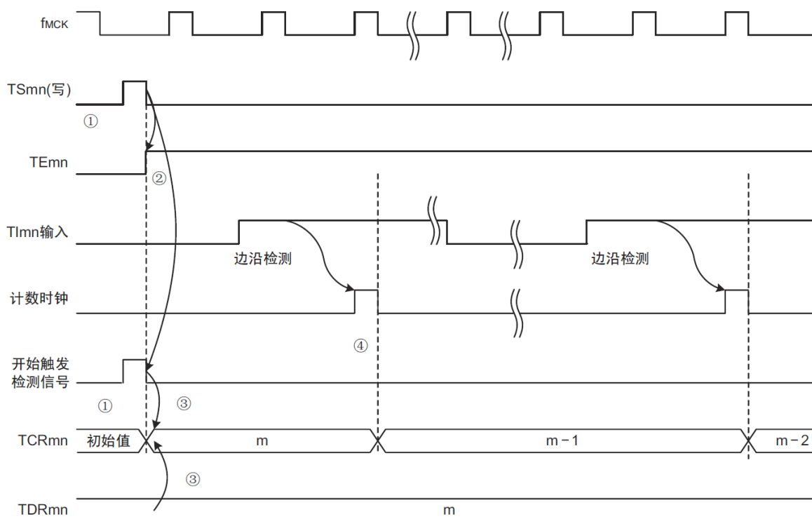
图5-25: 运行时序 (事件计数器模式)
