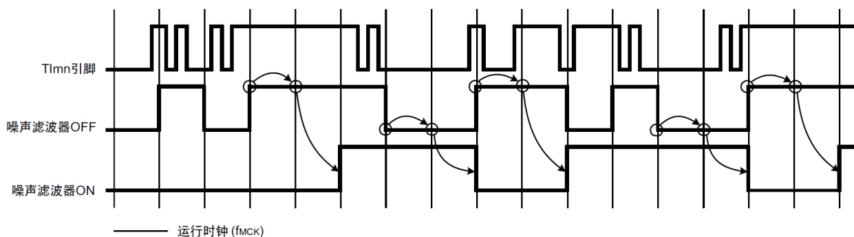
图5-39：TImn输入引脚在噪声滤波器ON或者OFF情况下的采样波形
