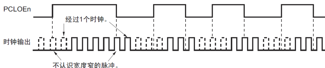
图9-3：CLKBUZn引脚的时钟输出时序
