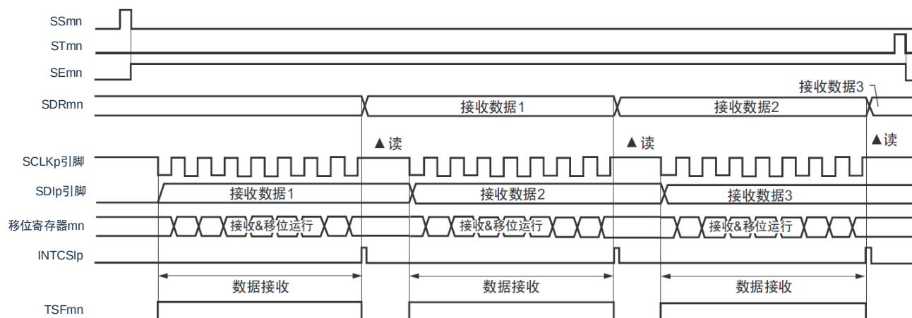
图16-59：从属接收（单次接收模式）的时序图（类型1：DAPmn=0、CKPmn=0）
