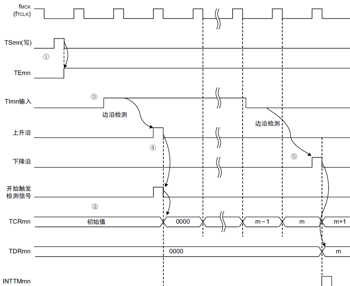
图5-28：运行时序（捕捉&单次计数模式：高电平宽度的测量）
