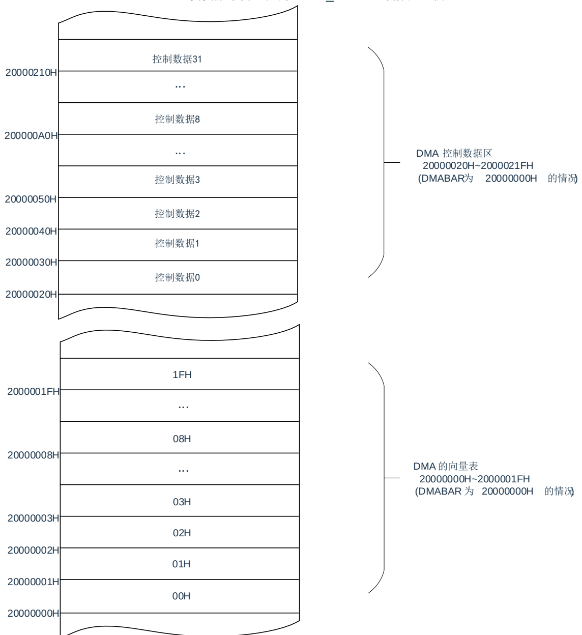
图22-4：控制数据的起始地址和向量表
