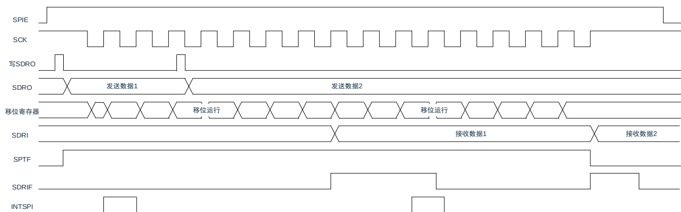
图17-10：发送/接收时序(连续发送模式)的时序图 (INTMD=1,CPHA=1、CPOL=1)
