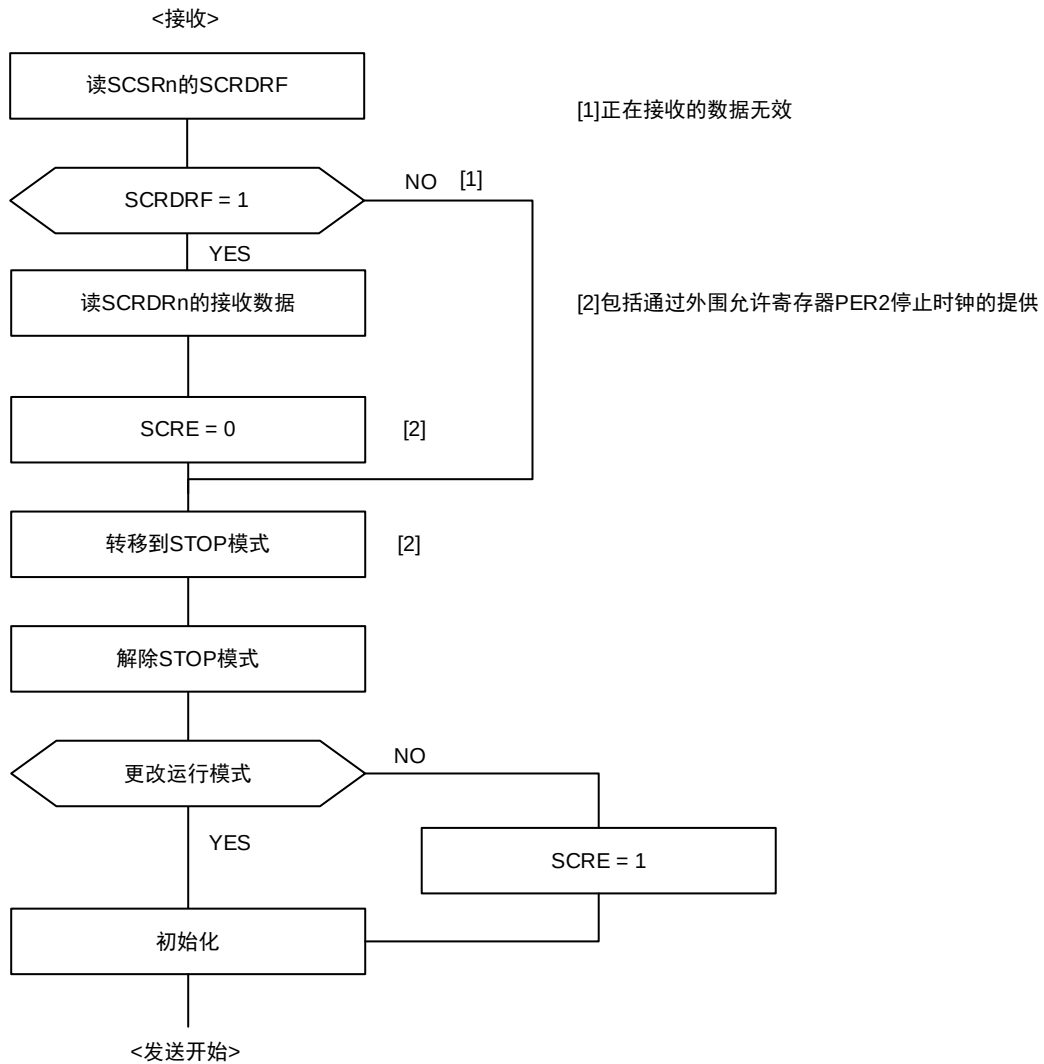
图 20-32接收时的模式转移流程图例子
