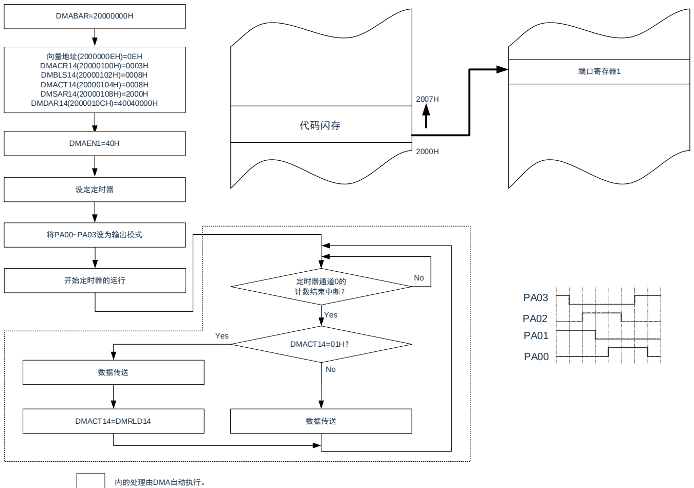
图22-20：重复模式的使用例子1：使用端口的步进马达控制脉冲输出
