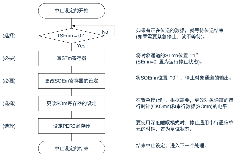
图16-25：主控发送的中止步骤
