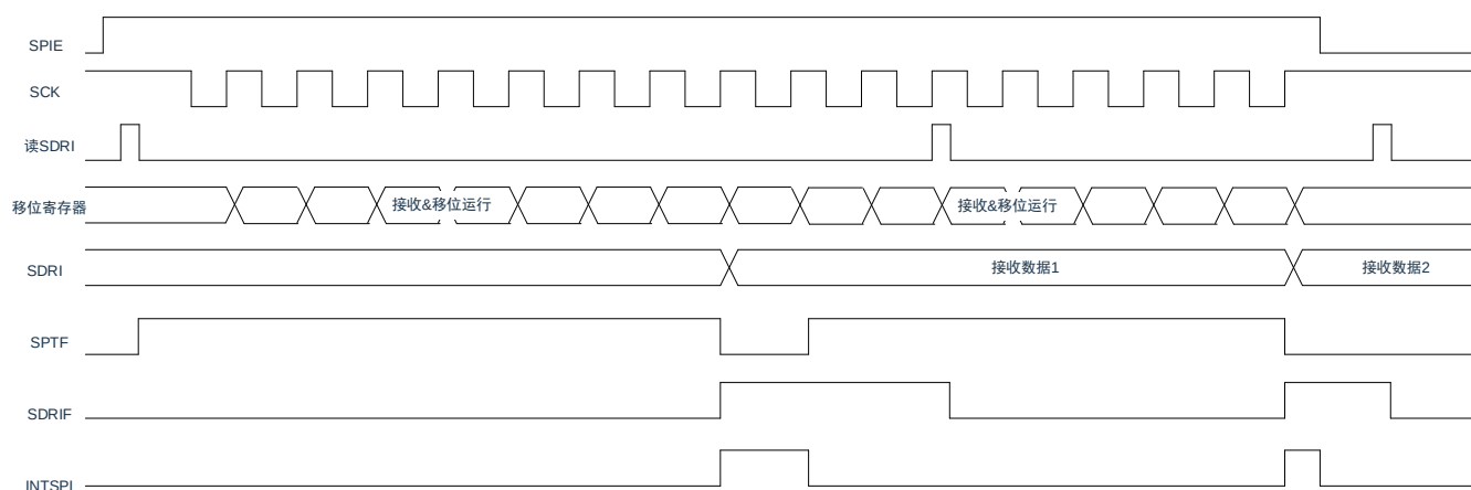
图17-13: 接收时序的时序图 (CPHA=1、CPOL=1)
