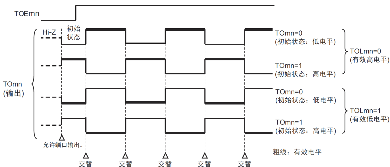
图5-31：交替输出时 ( TOMmn=0 ) 的 TOmn 引脚输出状态
