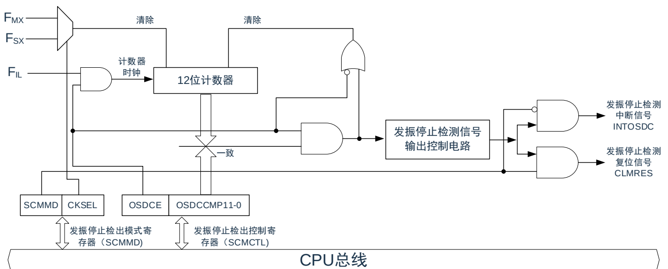
图4-18：发振停止检测电路的框图（例）
