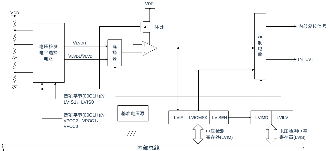
图 29-1：电压检测电路的框图
