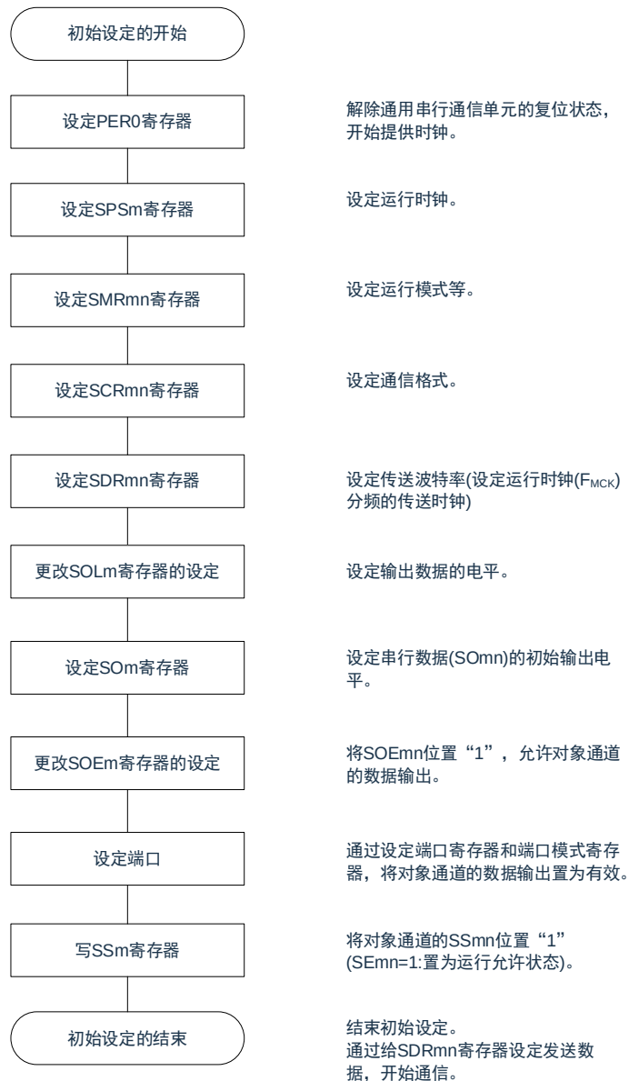
图16-97: UART发送的初始设定步骤
