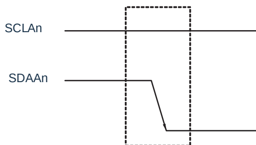
图18-14：开始条件
