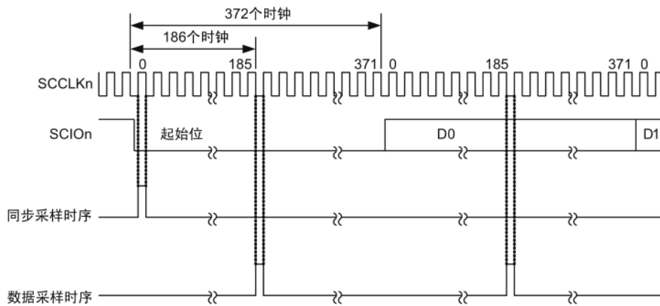
图 20-16 智能卡接口的接受数据采样时序(使用372倍的时钟时)
