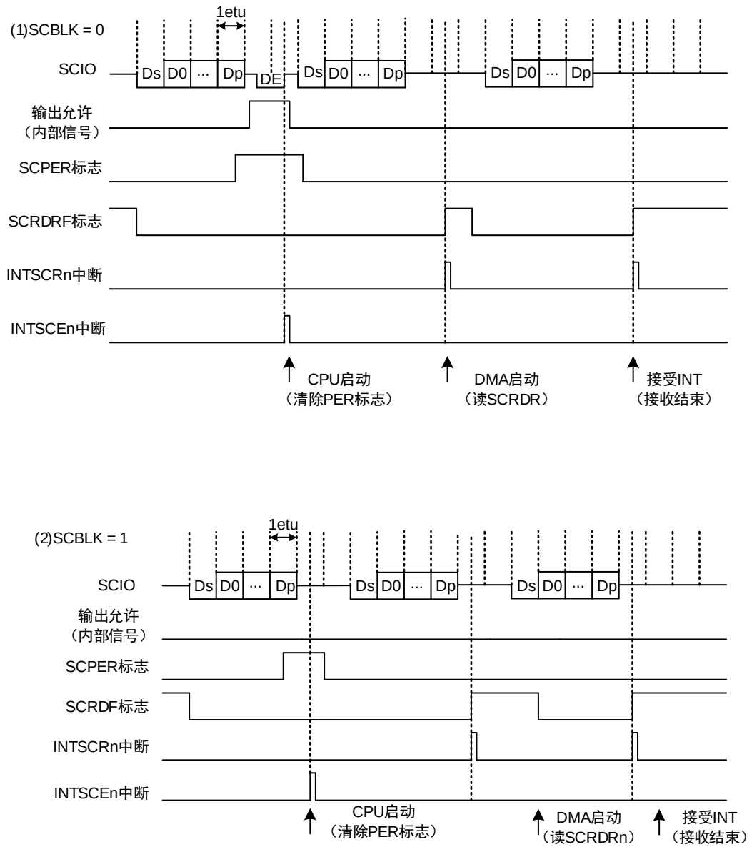
图 20-29使用DMA进行连续数据接收的时序图
