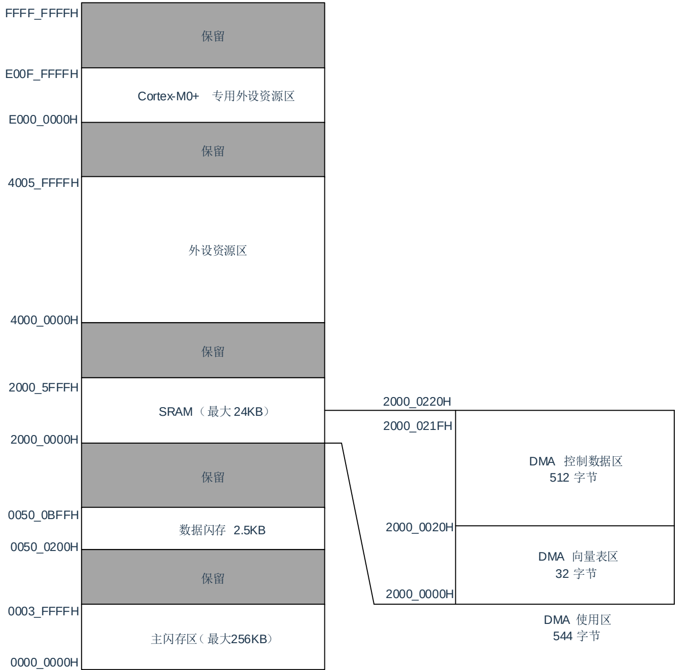
图22-2：DMABAR寄存器的设置值为“2000_0000H”时的存储器映像例子
