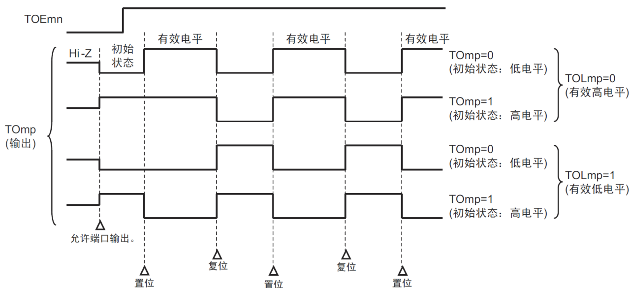
图5-32: PWM输出时 (TOMmn=1) 的TOMn引脚输出状态
