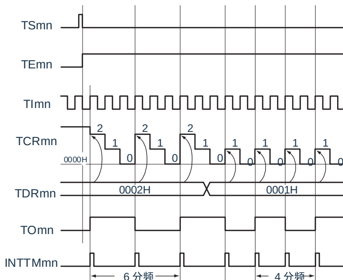
图5-47：作为分频器运行的基本时序例子（MDmn0=1）
