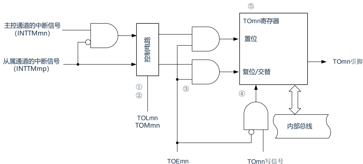
图5-29：输出电路的结构
