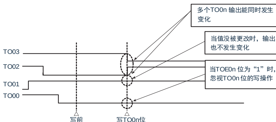
图5-36: 一次性操作TO0n位时的TO0n引脚状态
