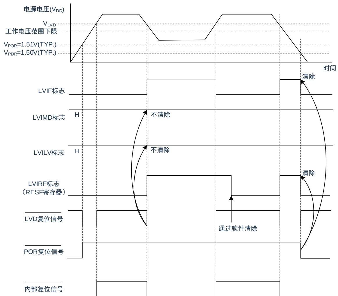
图 29-4：内部复位信号的产生时序（选项字节的 LVIMDS1、LVIMDS0=1、1）
