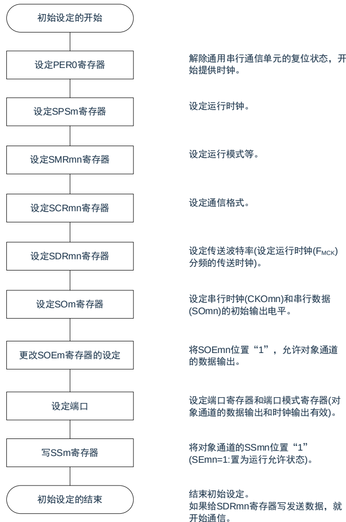
图16-24：主控发送的初始设置步骤
