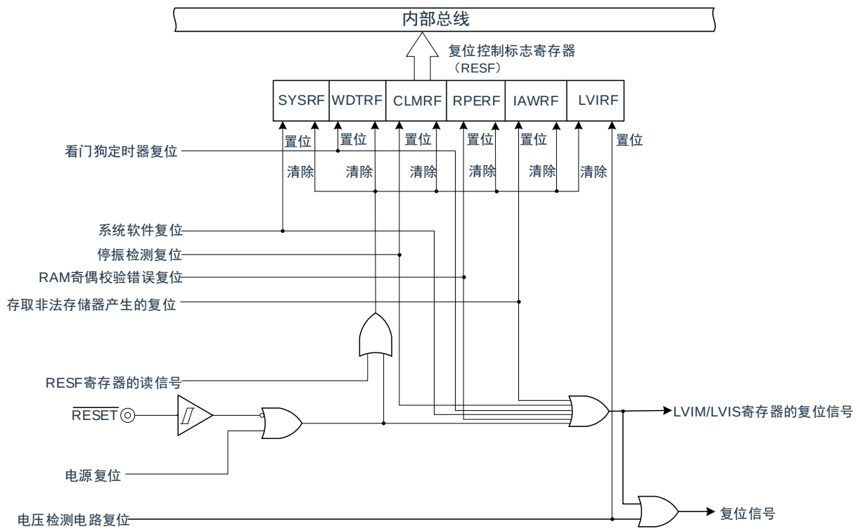
图27-1：复位功能的框图
