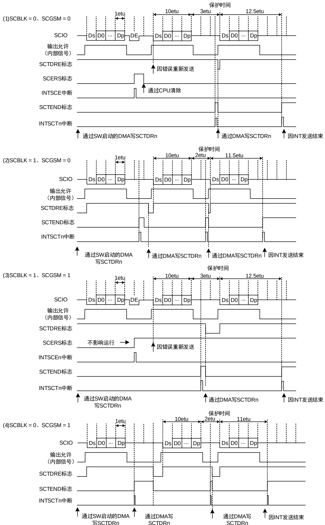
图 20-27 使用DMA进行连续数据发送的时序图
