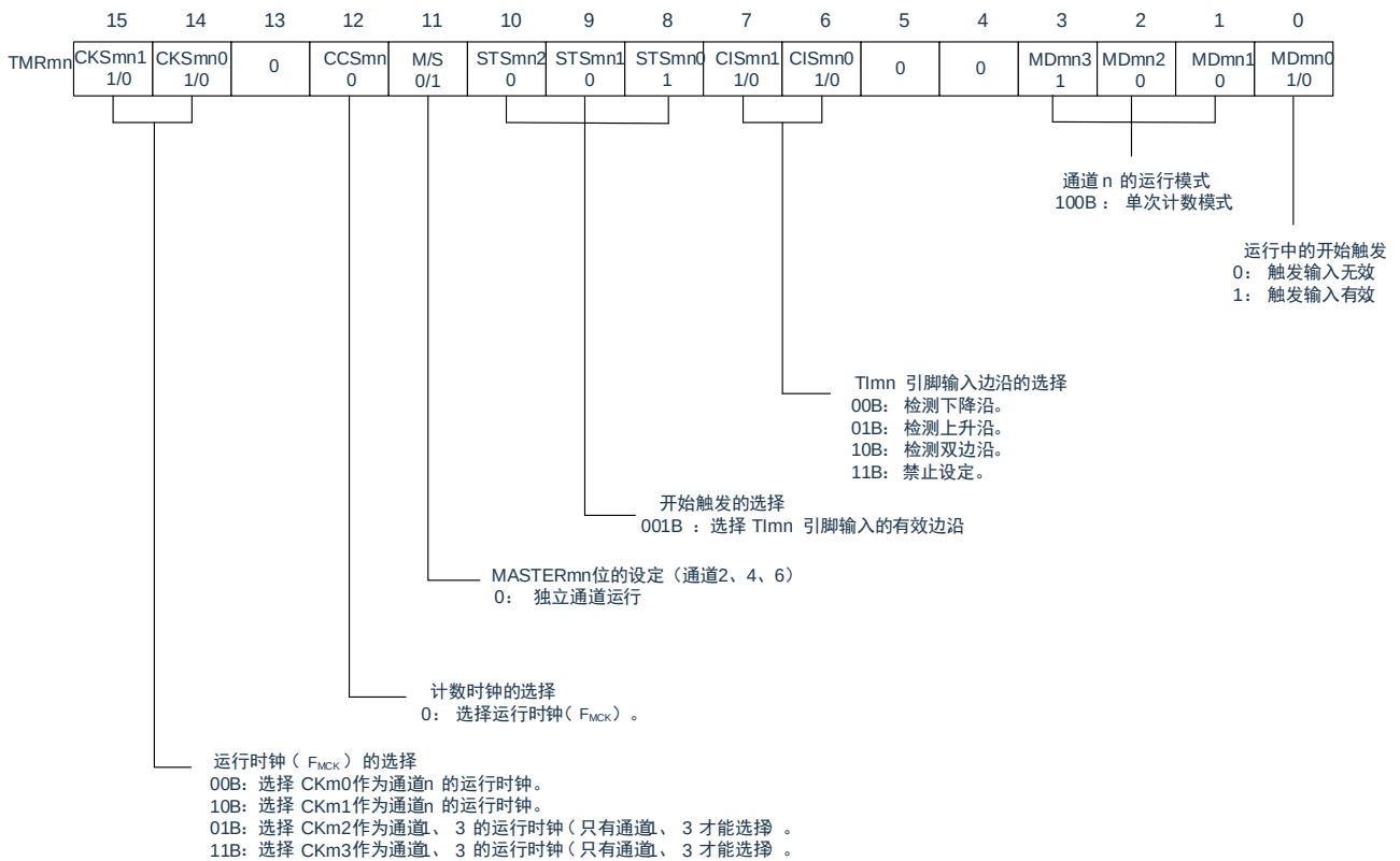
图5-57：延迟计数器功能时的寄存器设定内容例子
