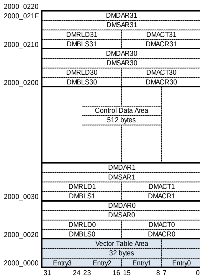
图22-3：控制数据的分配(DMABAR设置为2000_0000H)
