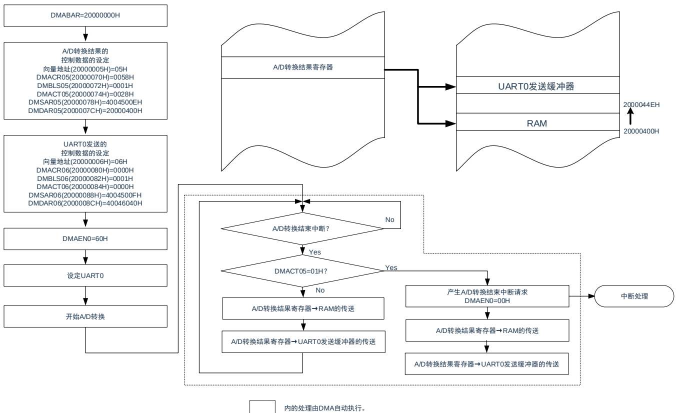
图22-22：链传送的使用例子：连续取A/D转换结果进行UART0发送
