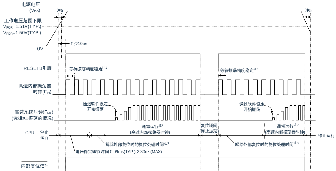
图 28-2：上电复位电路和电压检测电路的内部复位信号的产生时序(1/3)
