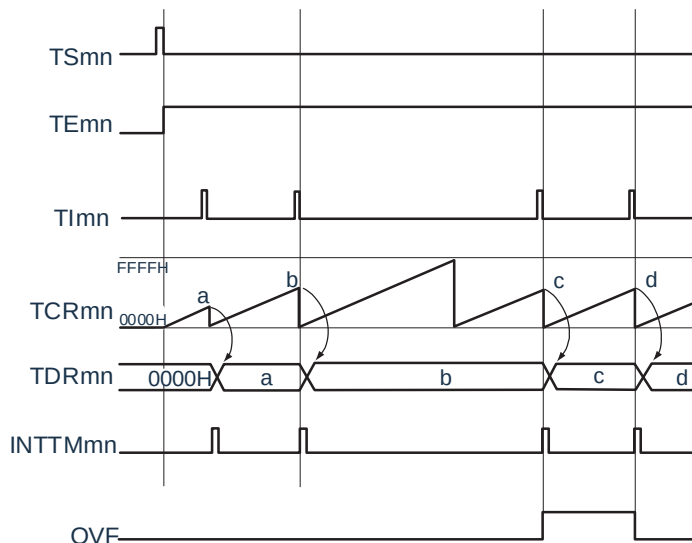
图5-50：作为输入脉冲间隔测量的运行基本时序例子 (MDmn0=0)
