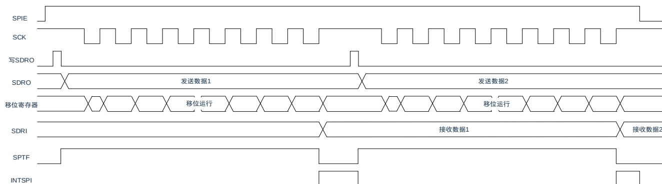
图17-10：发送/接收时序(连续发送模式)的时序图 (INTMD=1,CPHA=1、CPOL=1)
