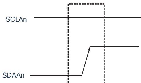
图18-18: 停止条件
