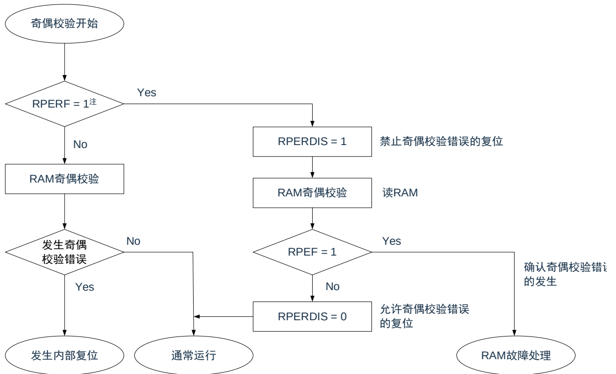
图30-8: RAM奇偶校验的流程
