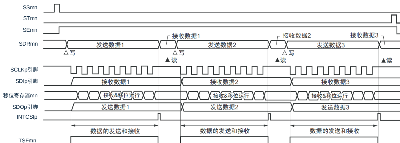
图16-43：主控发送和接收（单次发送和接收模式）的时序图（类型1：DAPmn=0、CKPmn=0）
