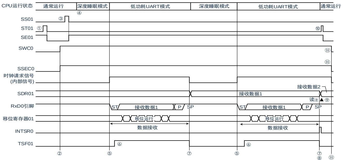
图 16-112: 低功耗UART模式运行 (SSECm=1) 的时序图
