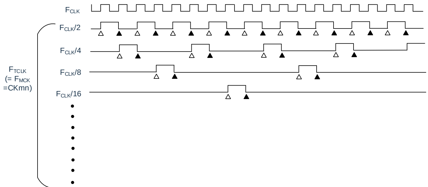
图5-22: F_{CLK} 和计数时钟 ( F_{TCLK} ) 的时序 ( CCSmn=0 的情况)
