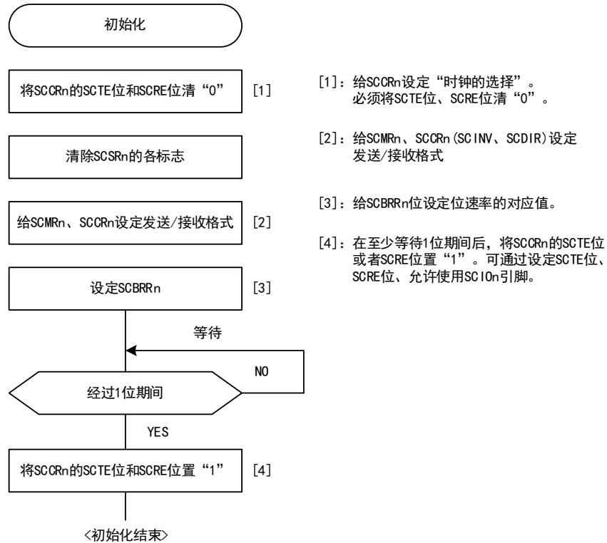
图 20-17 SCMI初始化的采样流程图
