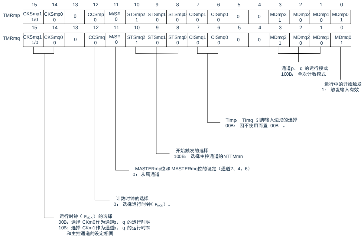
图5-74：多重PWM输出功能时（从属通道）的寄存器设定内容例子（输出2种PWM的情况）
