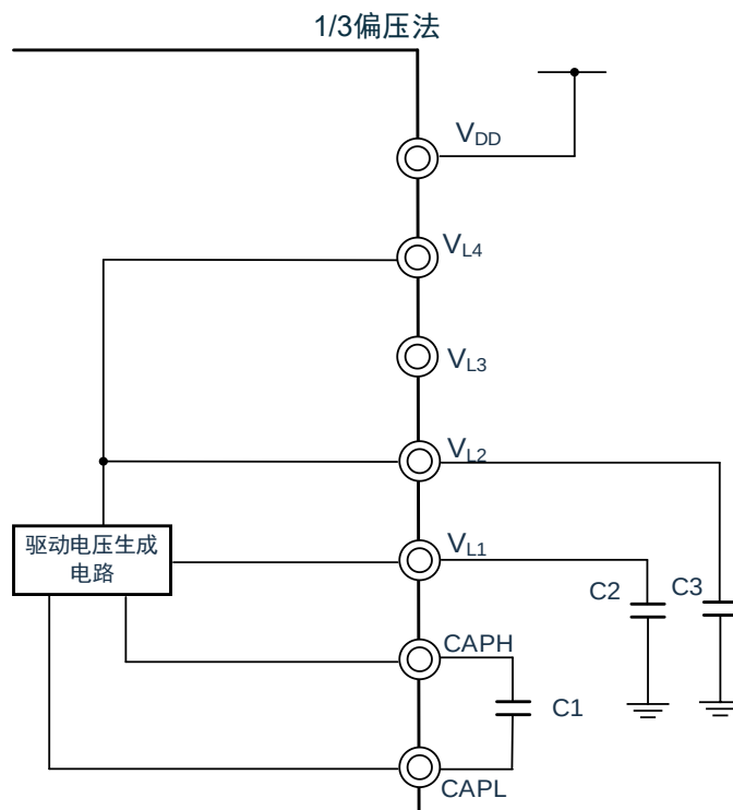
图 21-14：LCD驱动电源的连接例子（电容分割方式）
