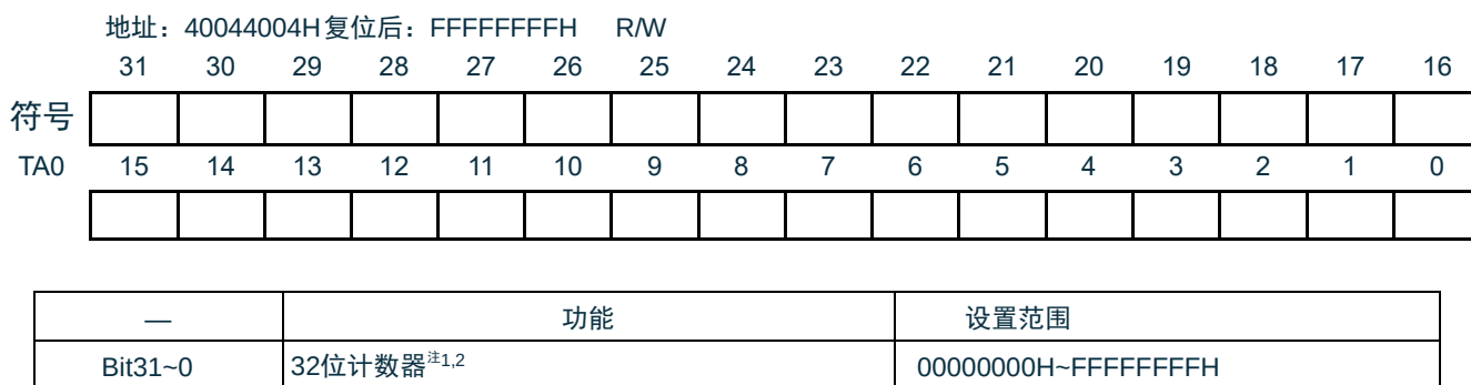
图 6-4：定时器A计数寄存器0（TA0）的格式
