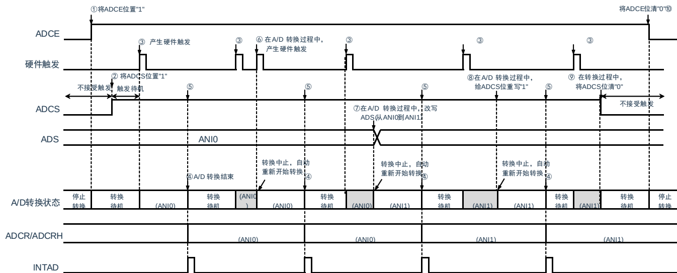
图11-24：硬件触发无等待模式（选择模式、单次转换模式）的运行时序例子
