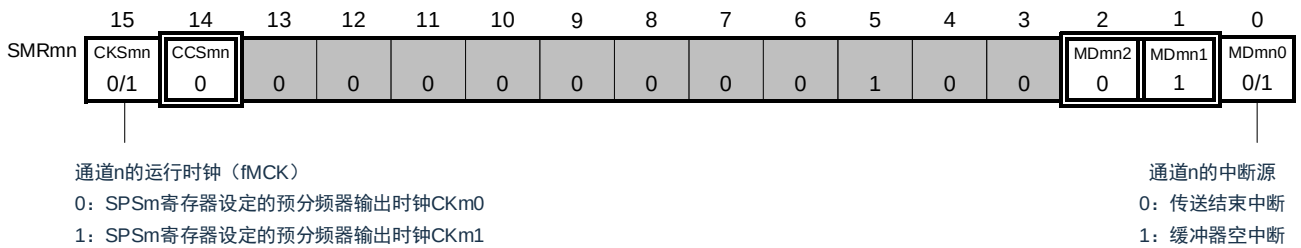
图16-96: UART (UARTm) 的UART发送时的寄存器设定内容例子(1/2)
