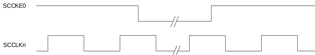
图 20-24 时钟输出的固定时序
