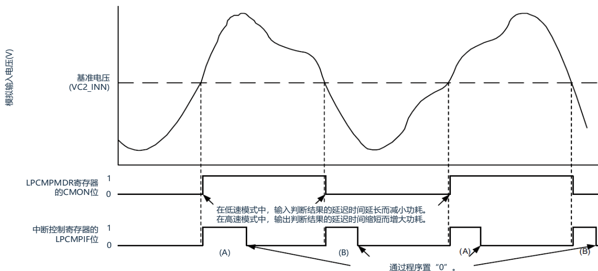
图14-9：低功耗比较器的运行例子（窗口模式）
