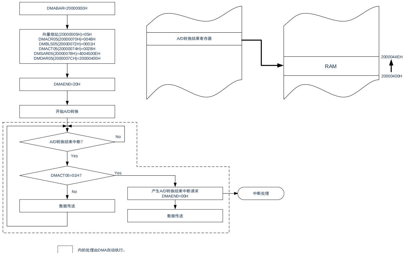
图22-17：正常模式的使用例子1：连续取A/D转换结果
