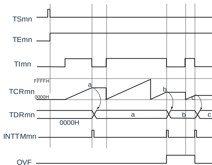
图5-53：作为输入信号高低电平宽度测量的运行基本时序例子
