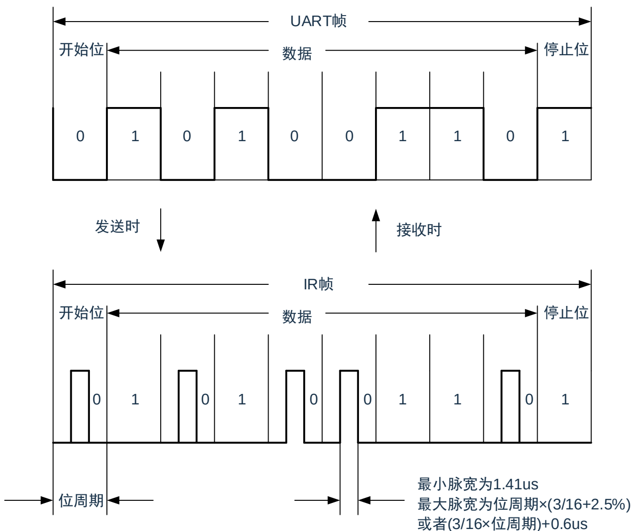
图19-4：IrDA的发送/接收运行图
