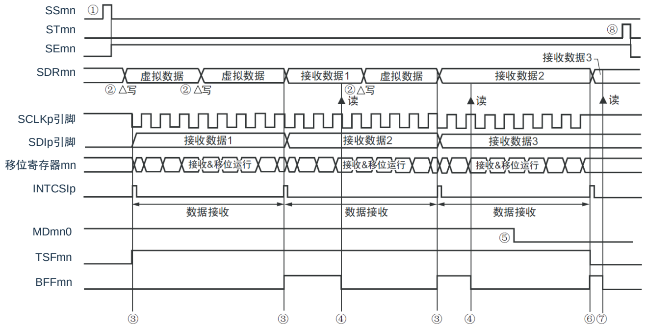
图16-37：主控接收（连续接收模式）的时序图（类型1：DAPmn=0、CKPmn=0）
