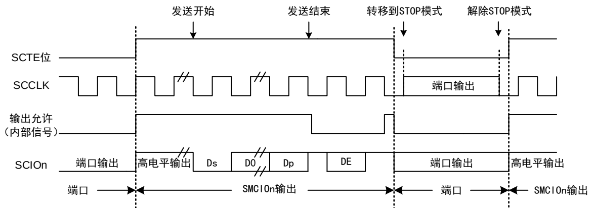
图 20-31 模式转移时的端口引脚状态
