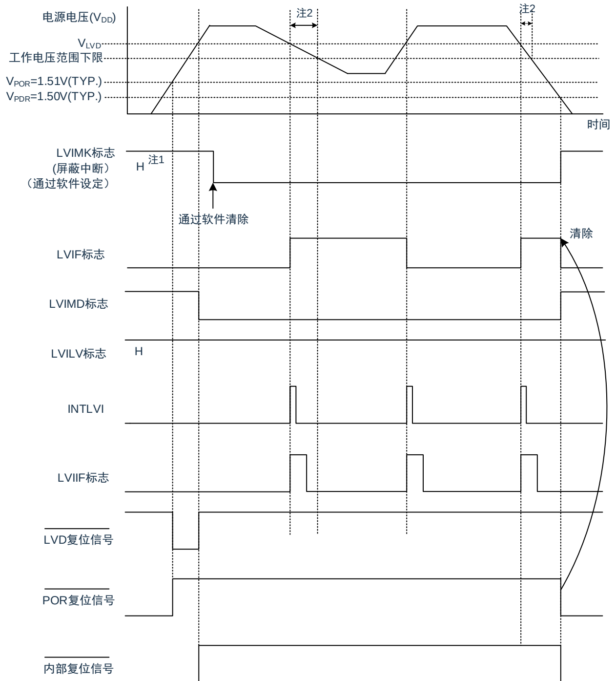
图 29-5：中断信号的产生时序（选项字节的LVIMDS1、LVIMDS0=0、1）
