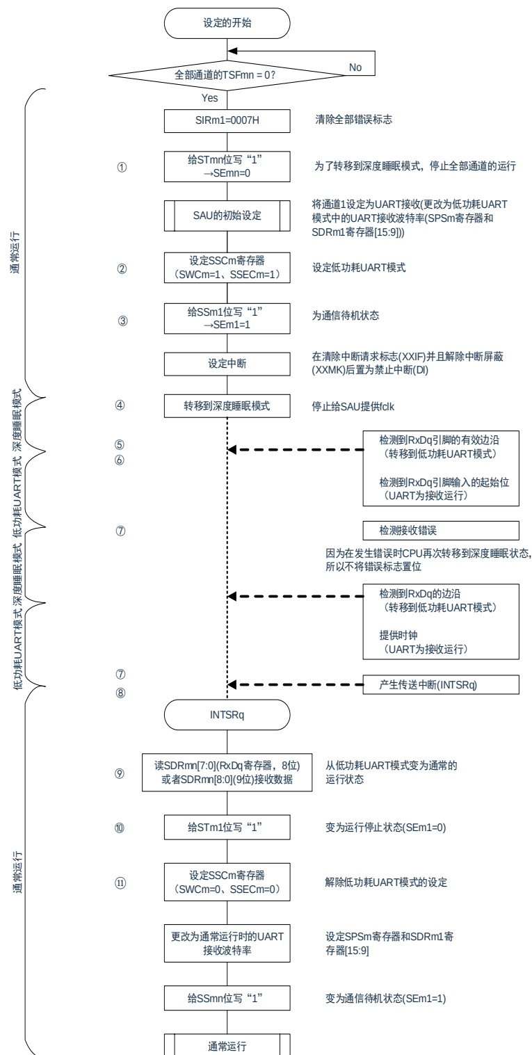
图 16-113: 低功耗UART模式运行 (SSECm=1) 的流程图
