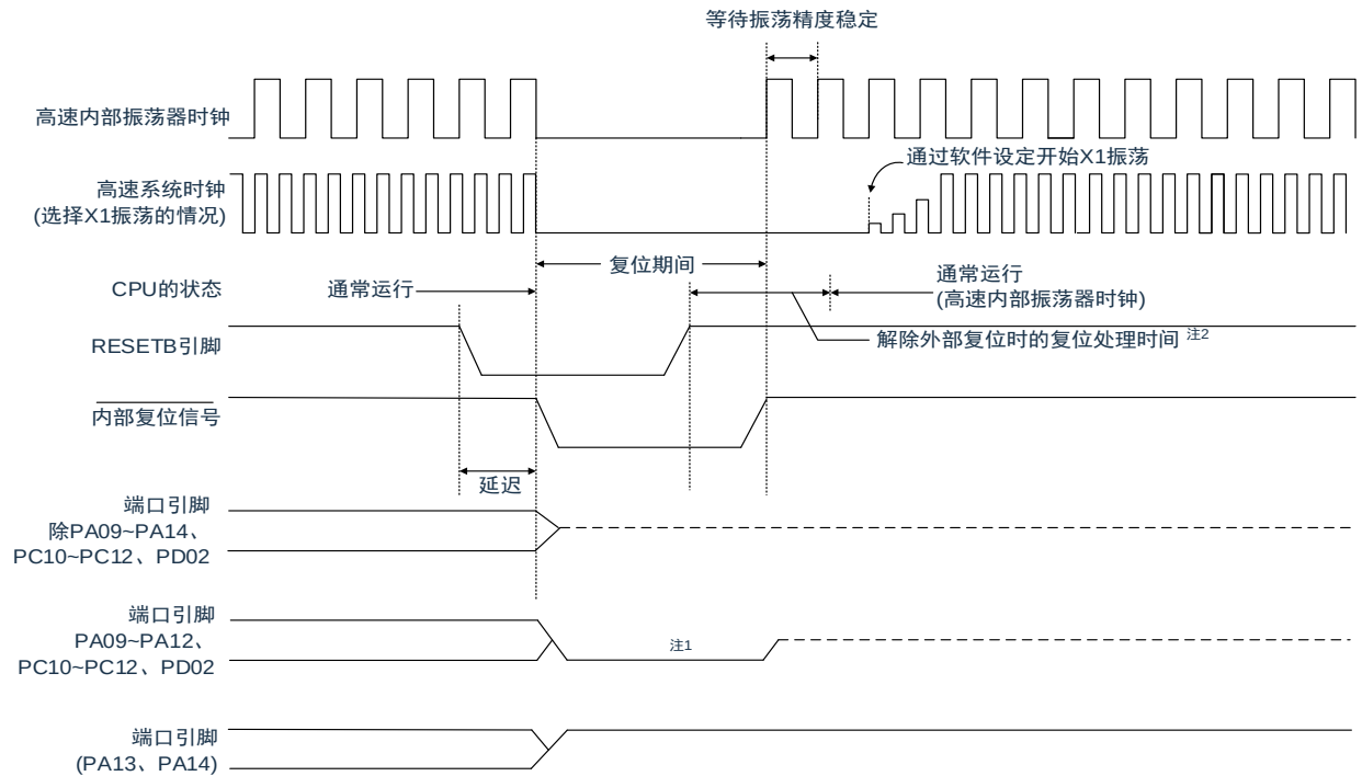
图27-2：RESETB输入的复位时序
