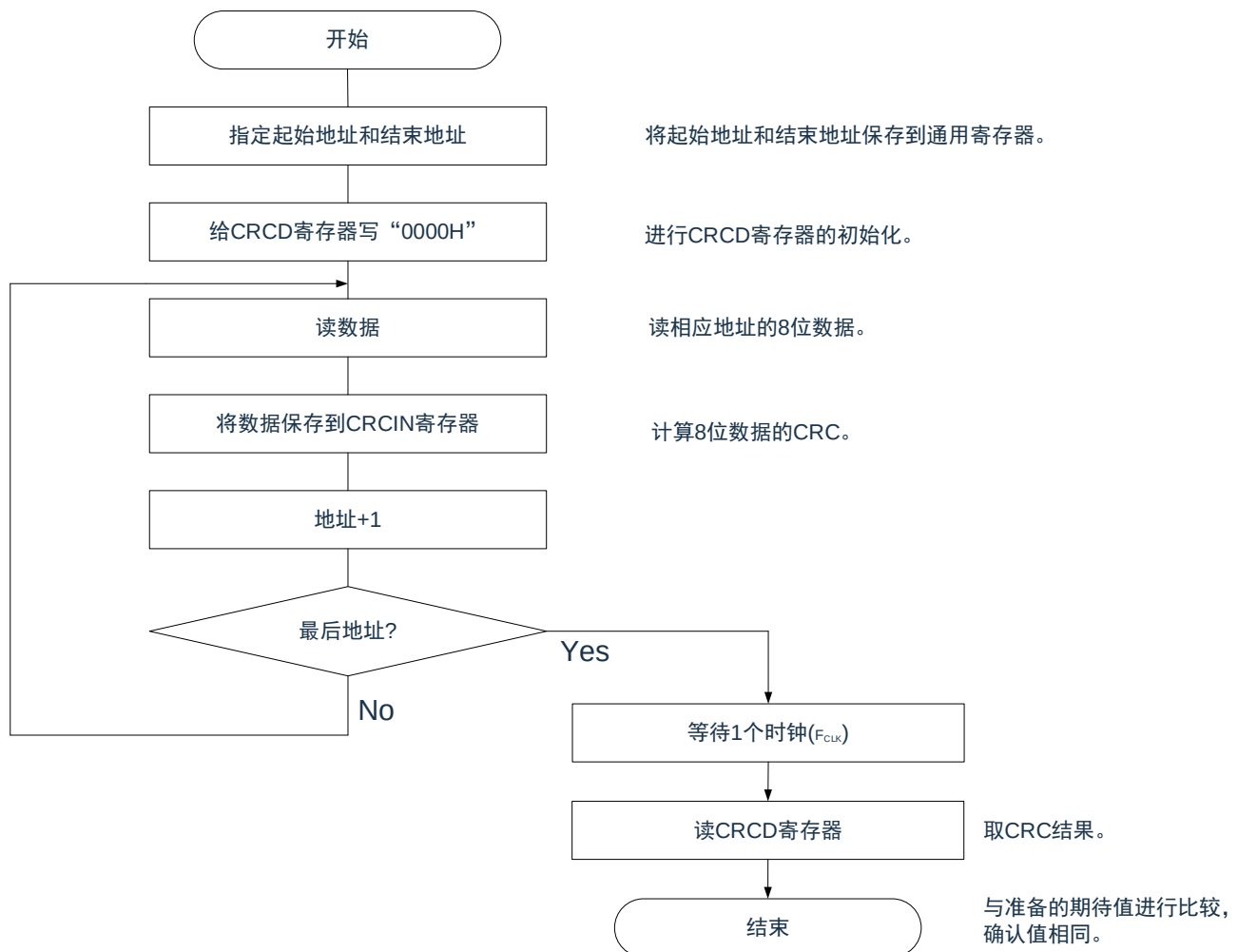
图30-6：CRC运算功能（通用CRC）的流程图
