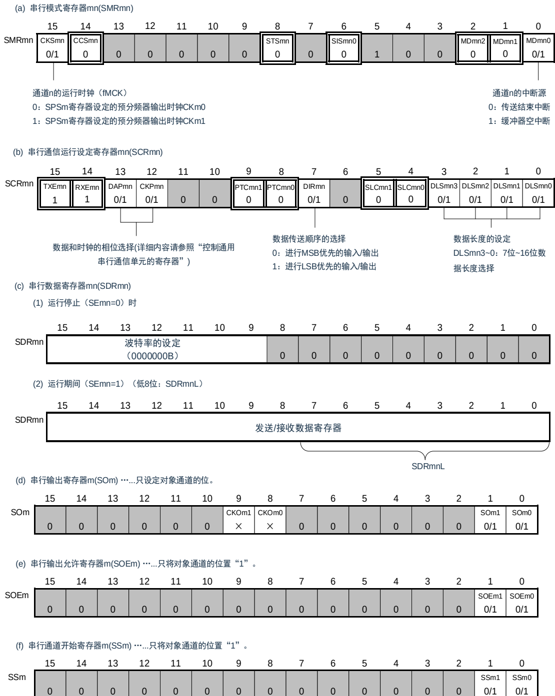
图16-61：3线串行I/O（SSPImn）
