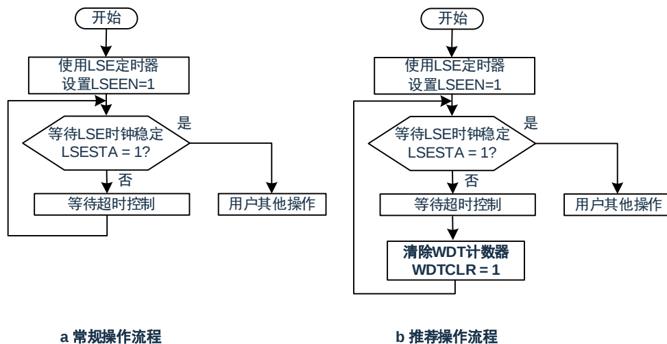
图 21-2：等待 LSE 稳定过程中的 WDT 操作
