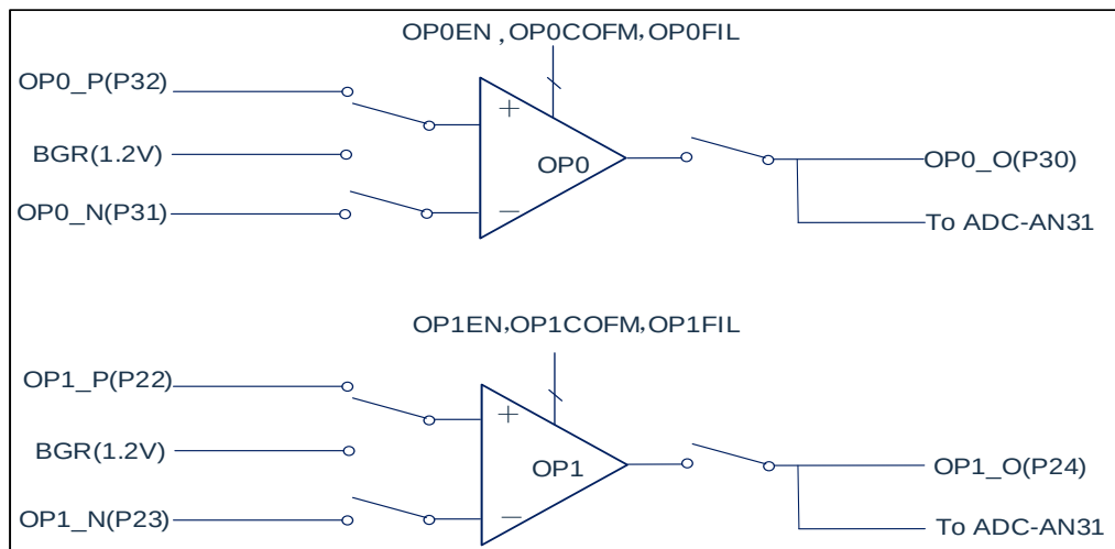
OP0/OP1 结构框图
