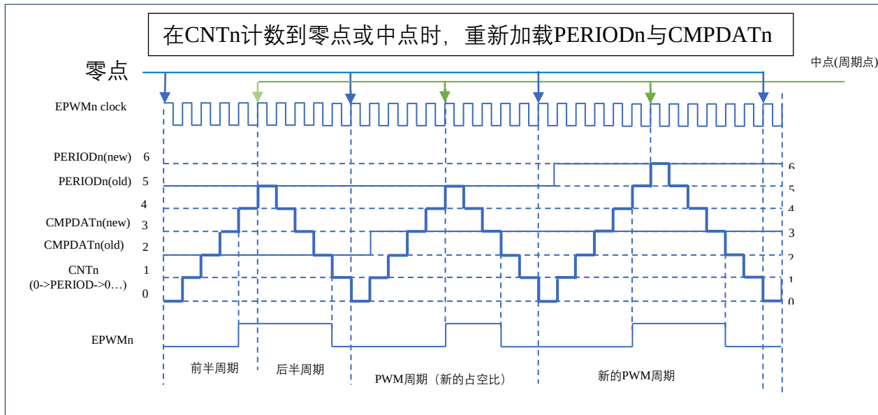
图12-5: 中心对齐计数器波形 (对称计数)
