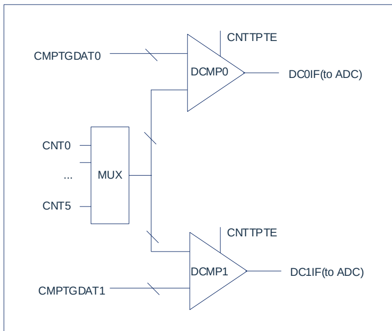
图12-7：独立计数器比较功能
