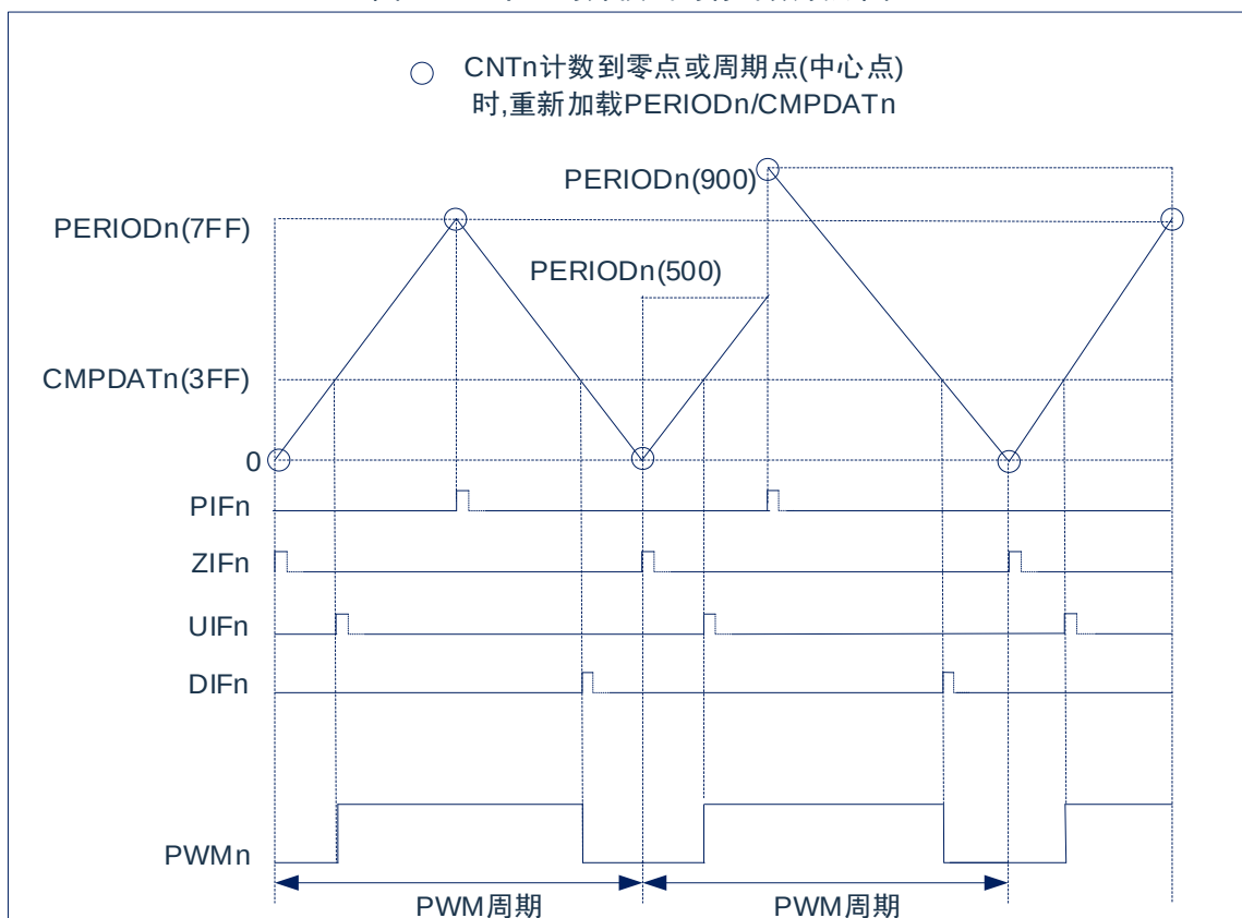
图12-4：中心对齐模式对称计数波形图
