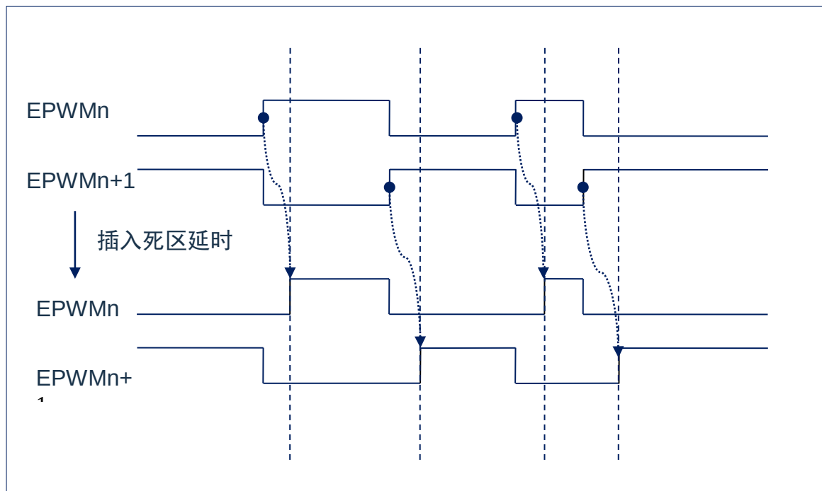
图12-10：中心对齐与边沿对齐均支持互补输出模式
