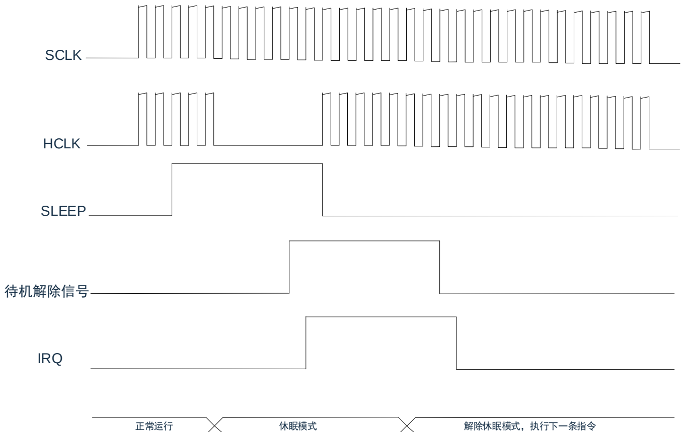
图21-1：通过中断请求解除睡眠模式
