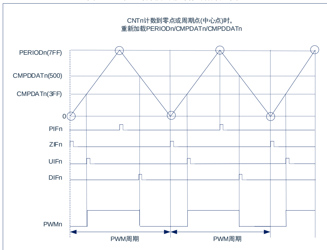
图12-6：中心对齐模式非对称计数波形图
