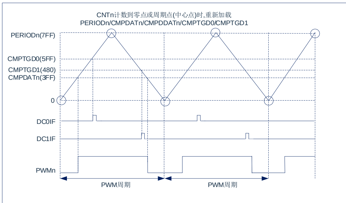
图12-9：中心对齐模式，数字比较器的工作方式
