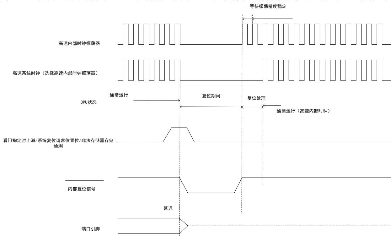
图 22-3: 因看门狗定时器的上溢、系统复位请求位的置位或者非法存储器存取的检测而产生的复位时序。
