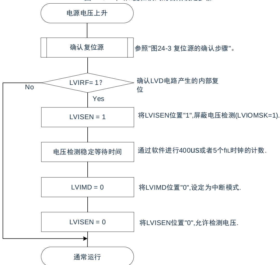
图24-6：中断&复位模式的初始设定步骤
