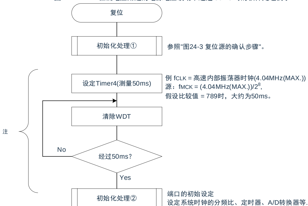
图 24-7：LVD 检测电压附近的电源电压波动不超过 50ms 时的软件处理例子
