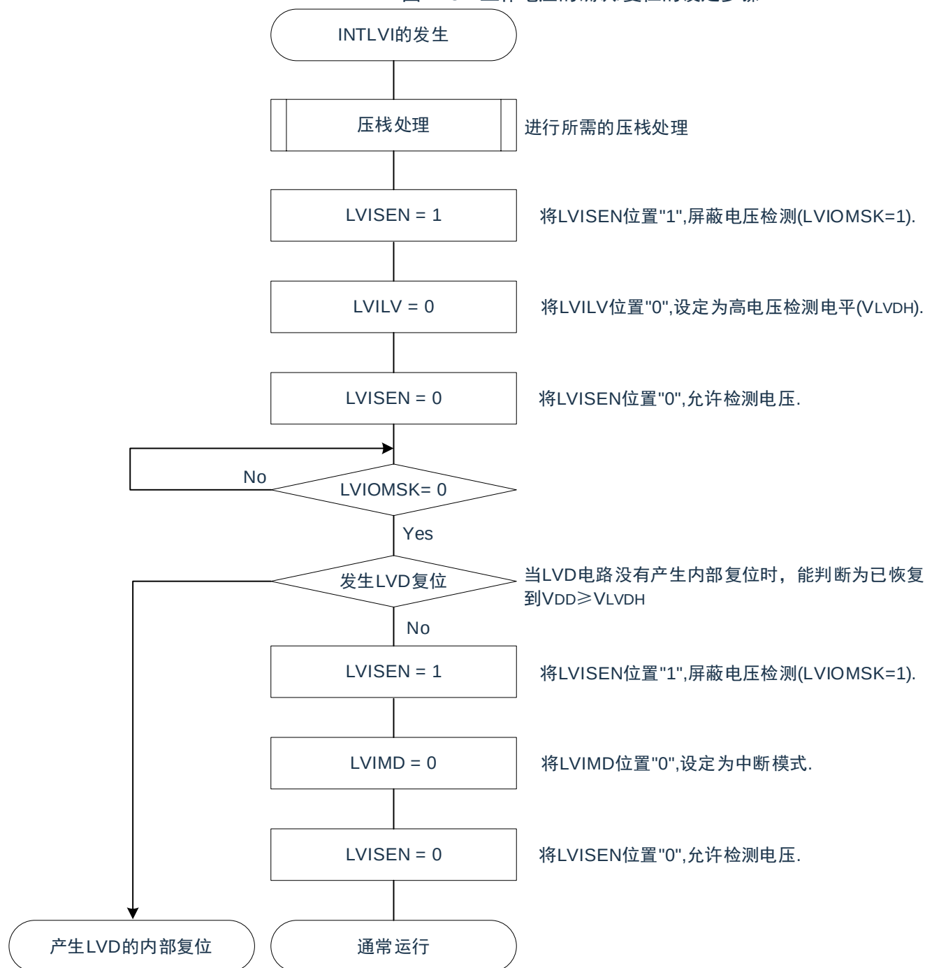
图24-5：工作电压的确认/复位的设定步骤
