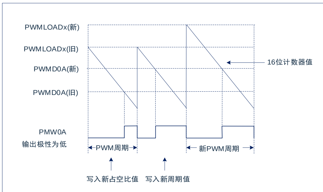
图 11-1: PWM 时序图
