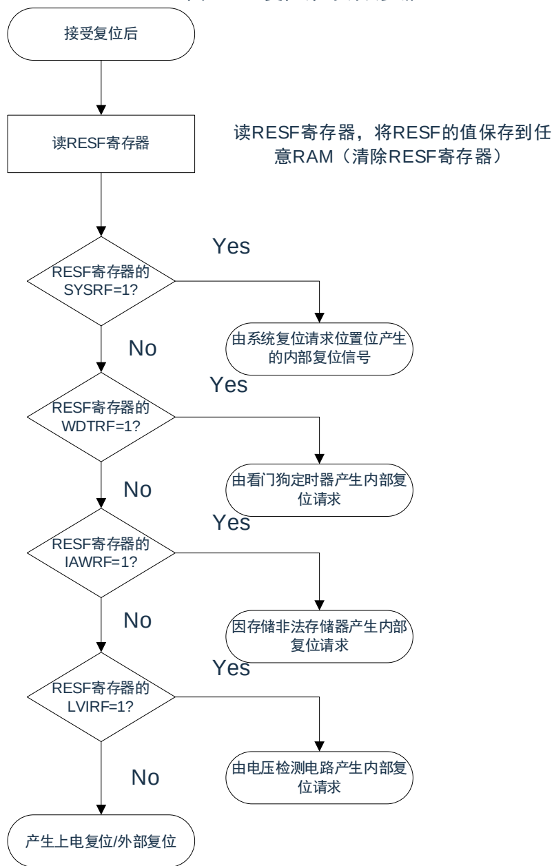
图22-4：复位源的确认步骤
