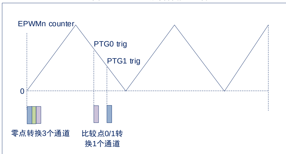
图16-2：EPWM触发启动ADC设置
