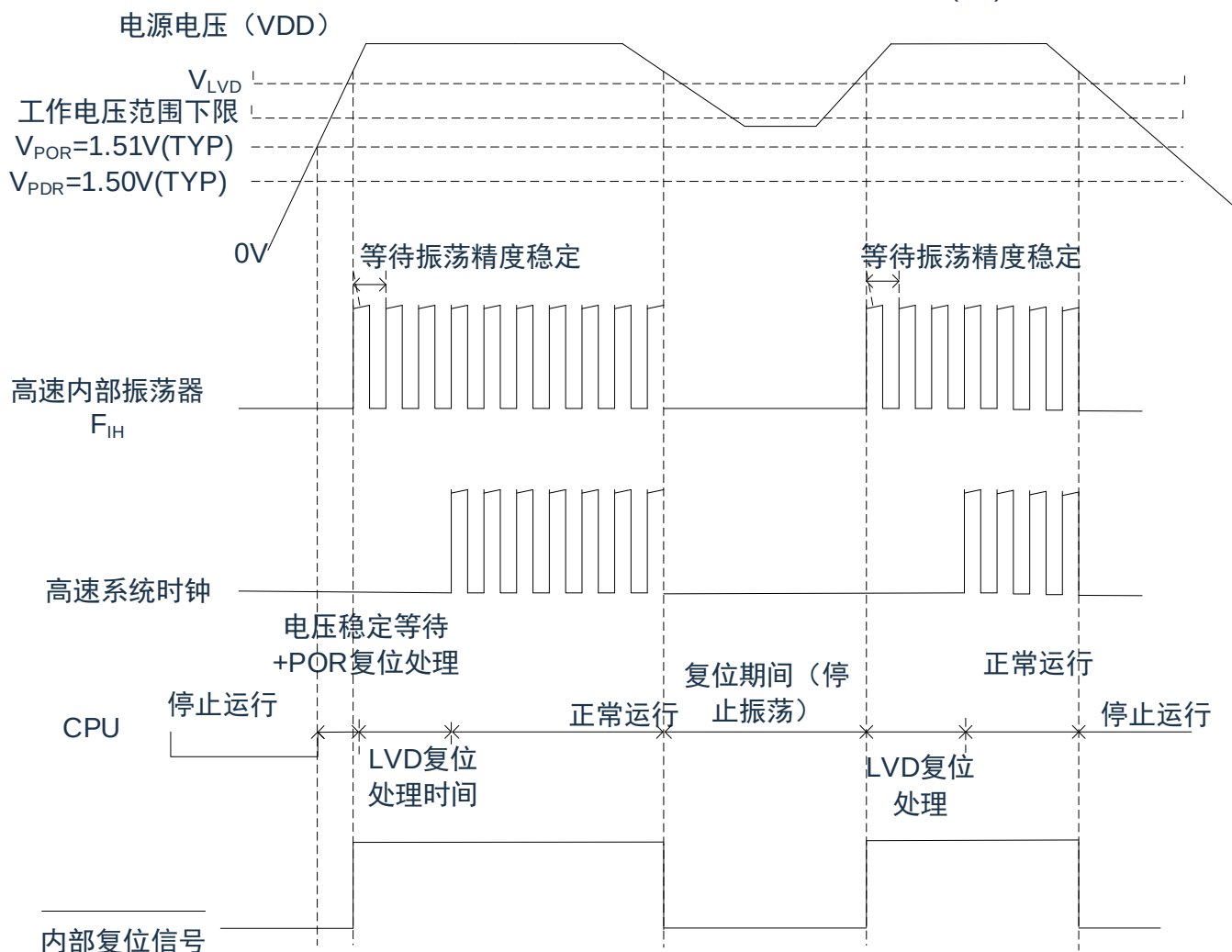
图23-2：位电路和电压检测电路的内部复位信号的产生时序(3/3)
