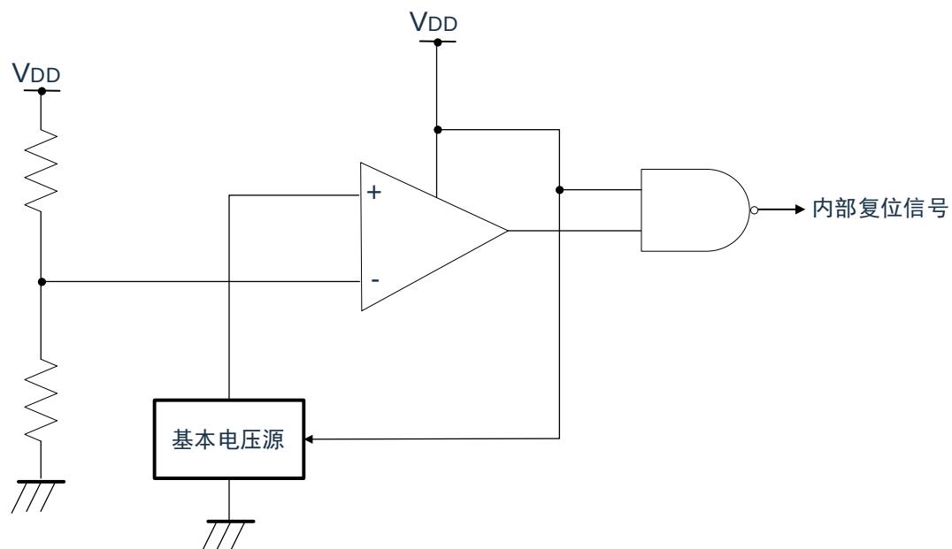
图23-1：上电复位电路的框图
