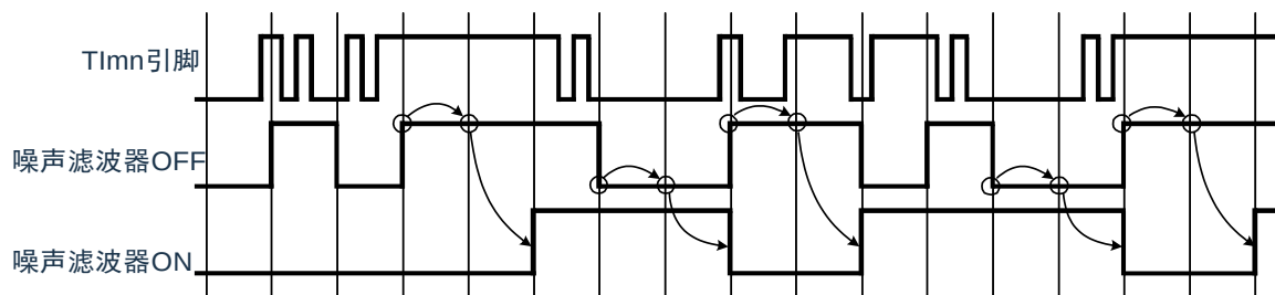
图6-18：Tlmn输入引脚在噪声滤波器ON或者OFF情况下的采样波形
