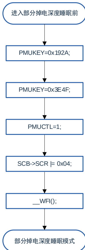
图 21-5：进入部分掉电的深度睡眠模式流程图
