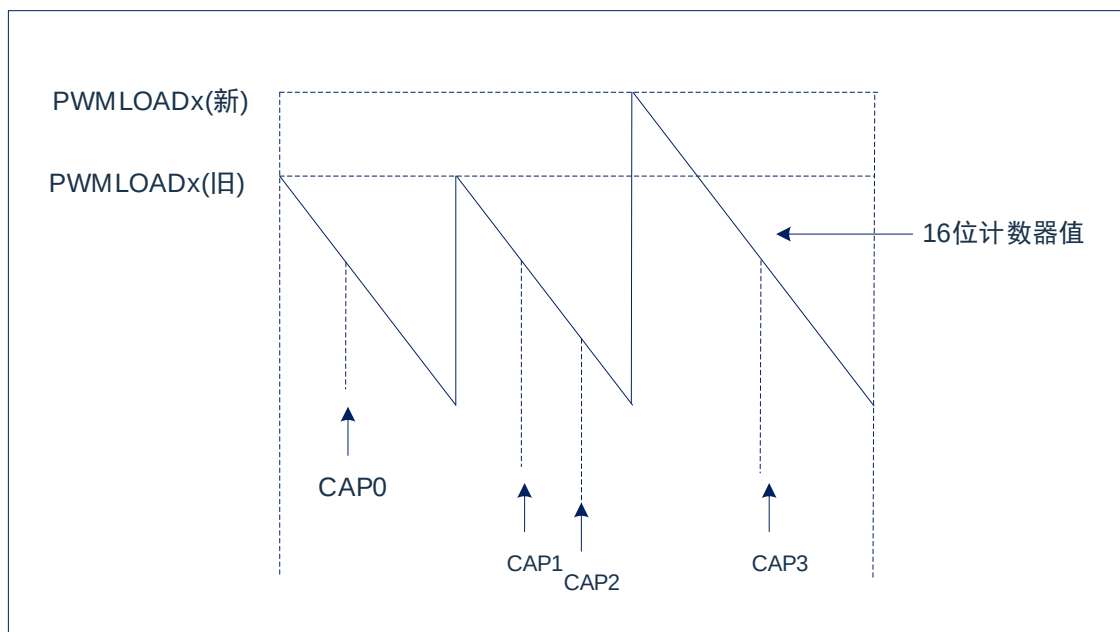
图 11-2：CAP0-CAP3 通道捕获操作
