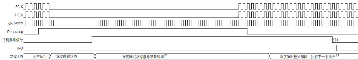
图21-6：通过中断请求解除深度睡眠模式
