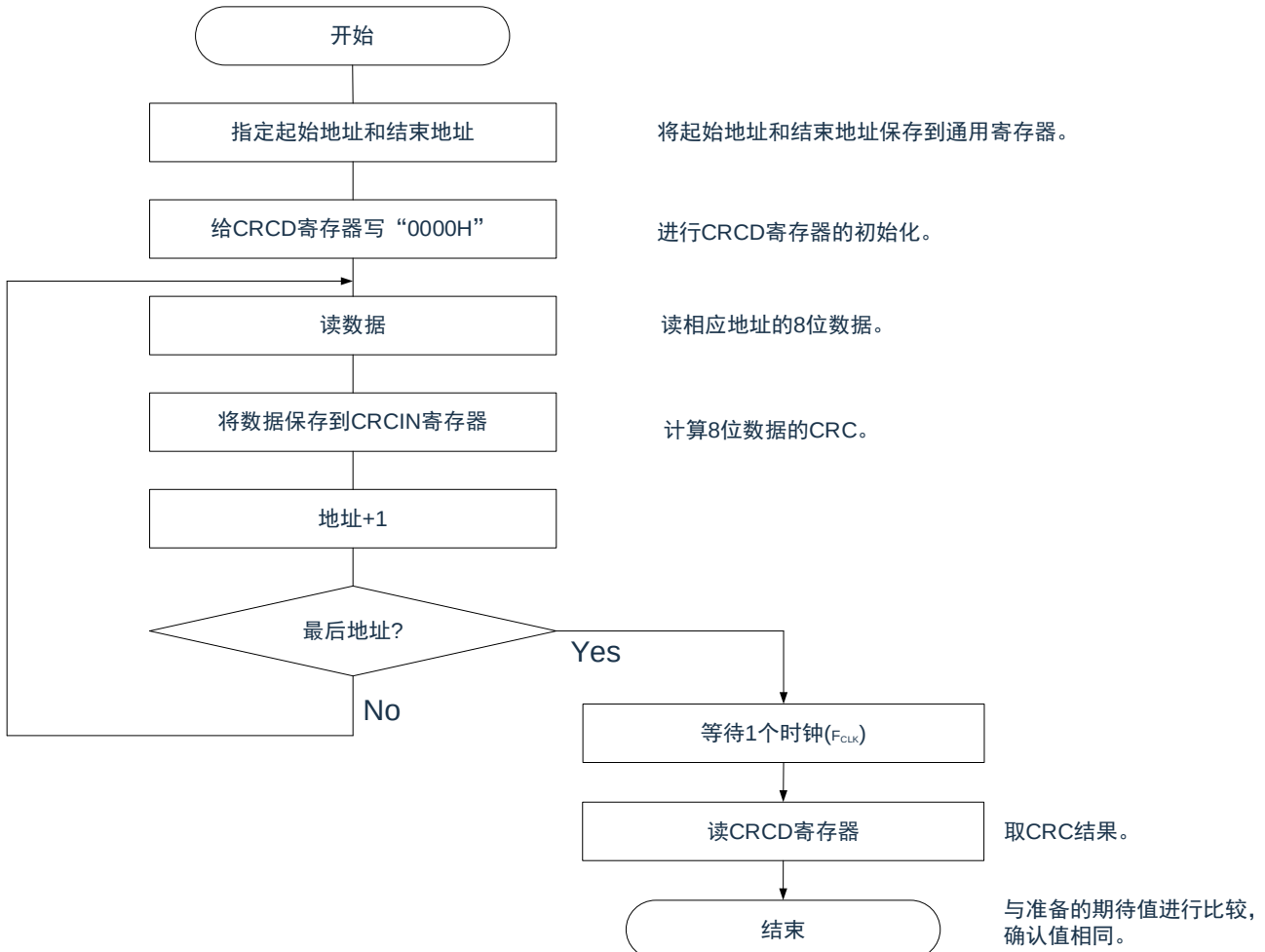
图25-2：CRC运算功能（通用CRC）的流程图
