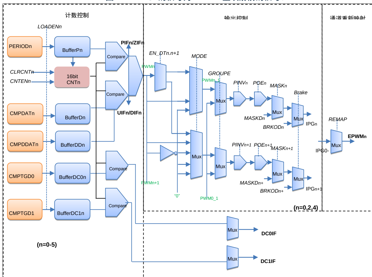
图12-1: IPGn的信号为EPWMn重映射前的信号。
