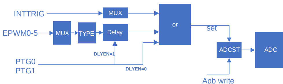
图16-1：ADC硬件触发启动
