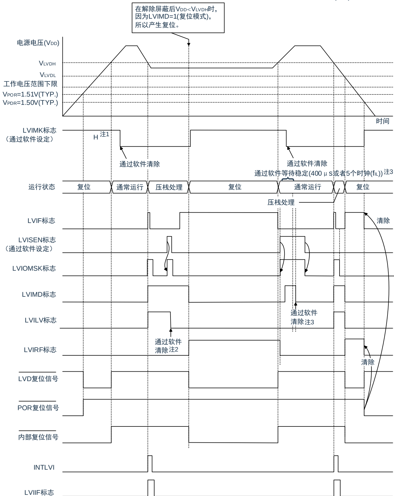
图 24-4：中断&复位信号的产生时序（选项字节的 LVIMDS1、LVIMDS0=1、0）(2/2)
