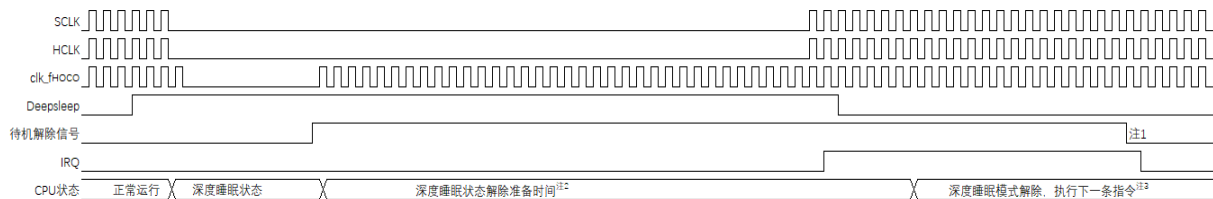
图21-3：通过中断请求解除深度睡眠模式
