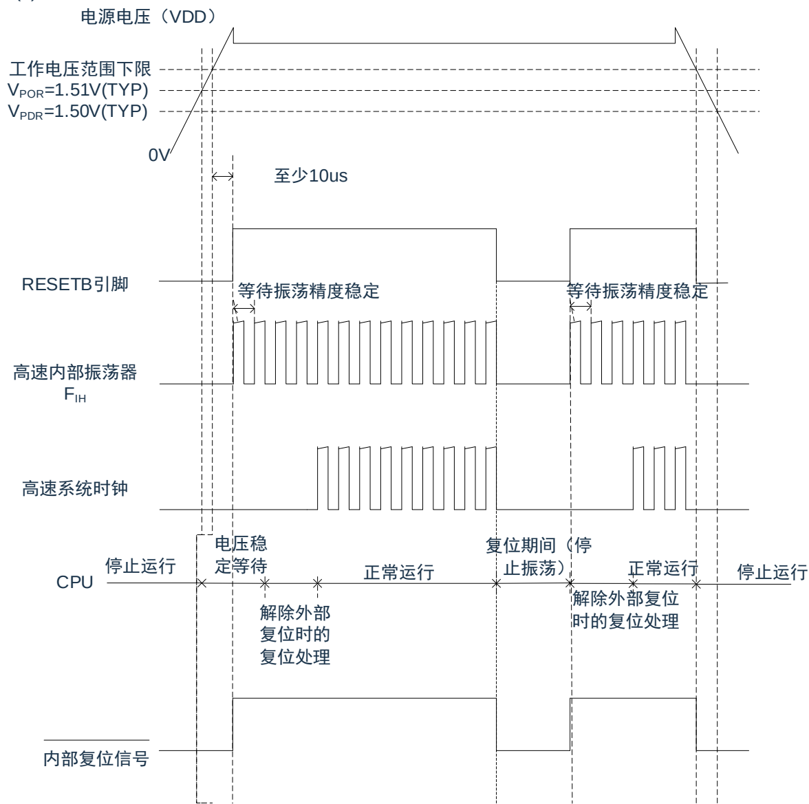
图 23-2：上电复位电路和电压检测电路的内部复位信号的产生时序(1/3)
