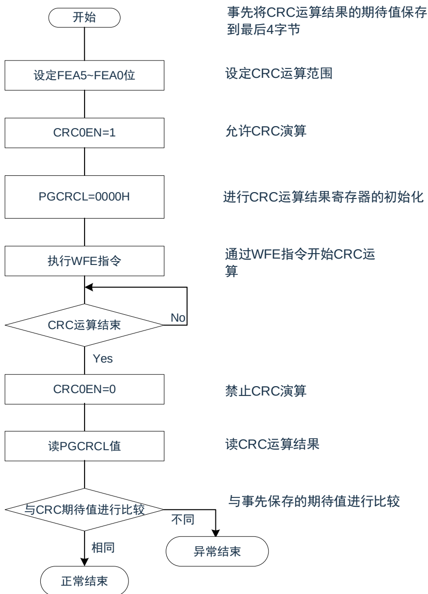
图25-1：闪存CRC运算功能（高速CRC）的流程图
