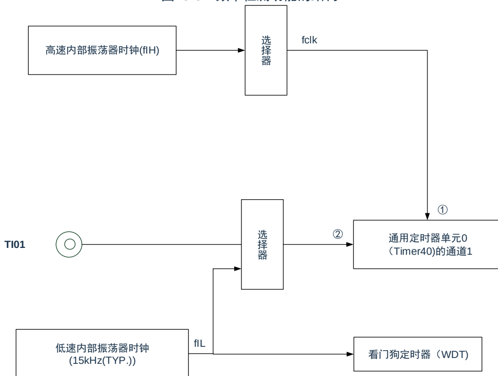
图25-3: 频率检测功能的结构
