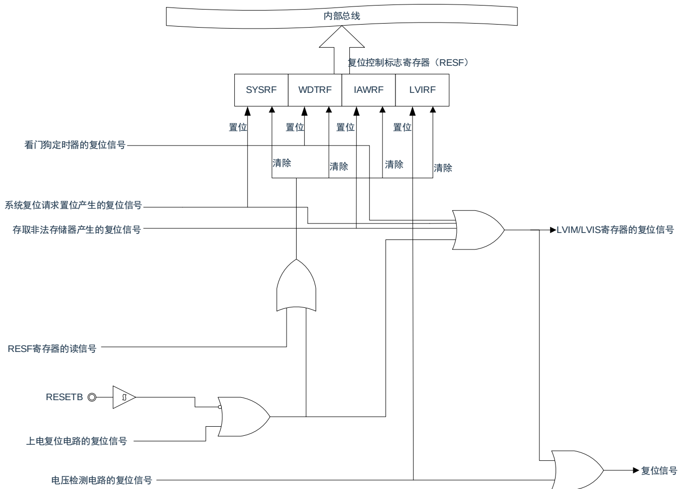
图22-1：复位功能的框图
