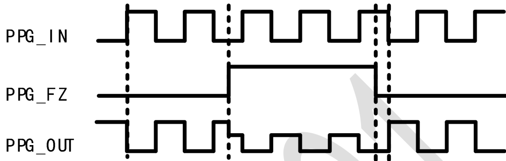
图 8- 1: CMS6401 上电启动时序图
