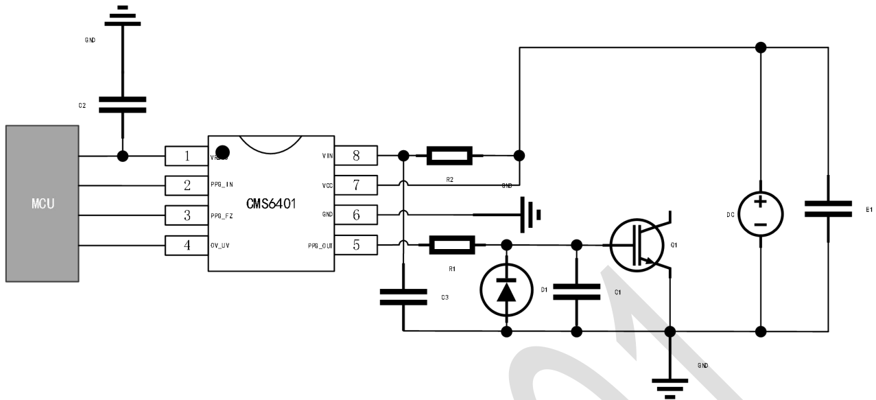
图 7- 1：CMS6401 典型应用电路
