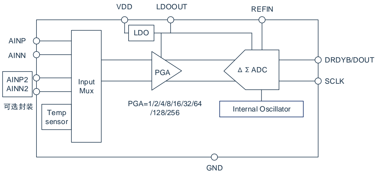
图 1-1: CMS1238 原理框图
