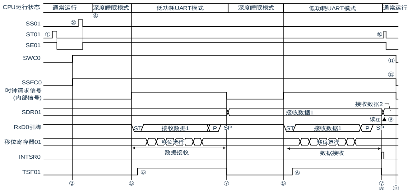
图 15-112: 低功耗 UART 模式运行 (SSECm=1) 的时序图
