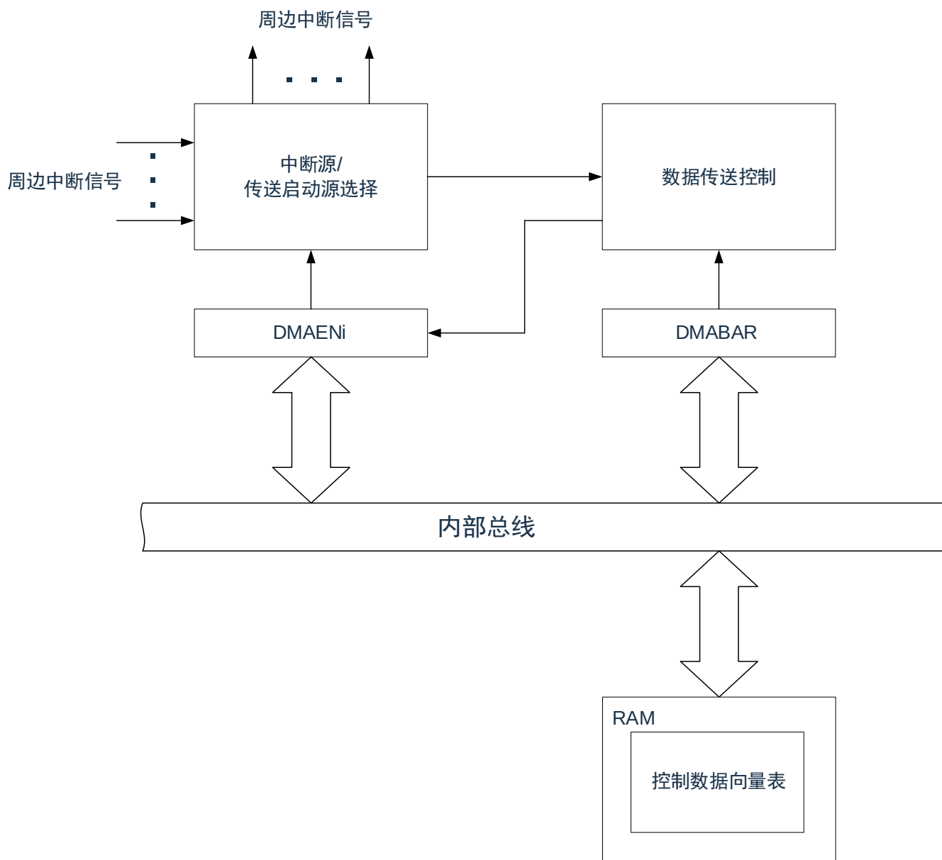
图 20-1: DMA 的框图
