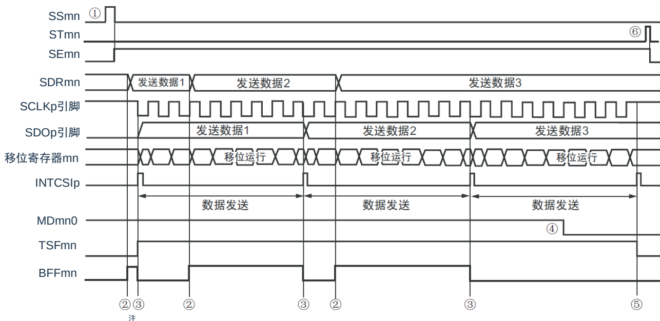
图 15-29：主控发送（连续发送模式）的时序图（类型 1：DAPmn=0、CKPmn=0）
