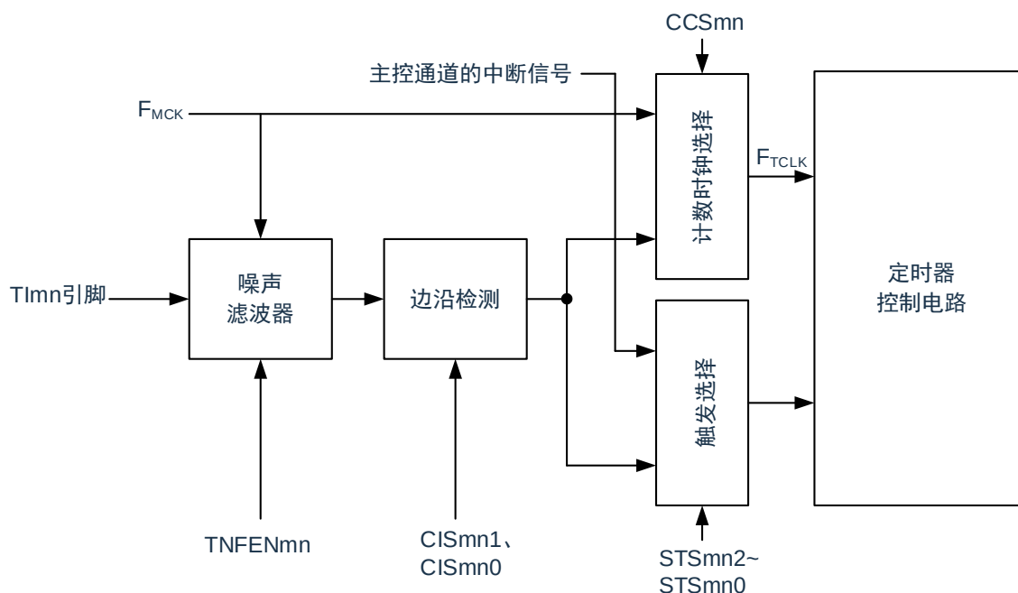
图 5-38：输入电路的结构
