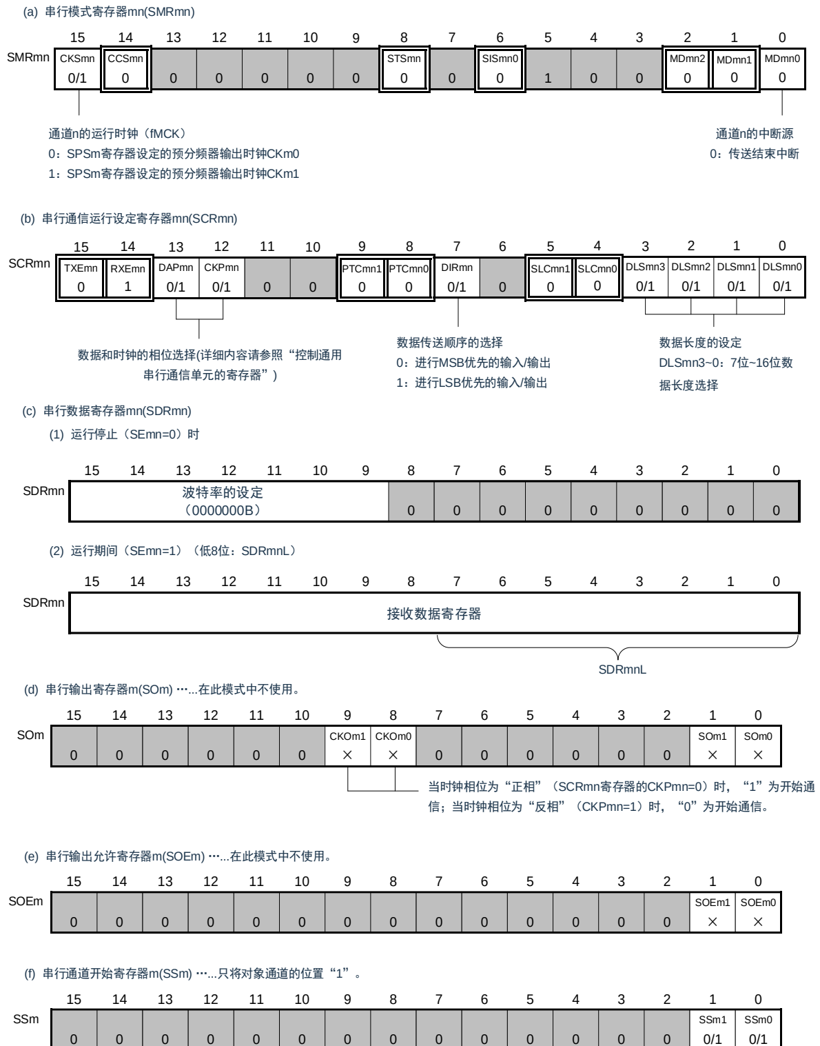
图 15-55: 3 线串行 I/O (SSPI00、SSPI01、SSPI10、SSPI11、SSPI20、SSPI21)
