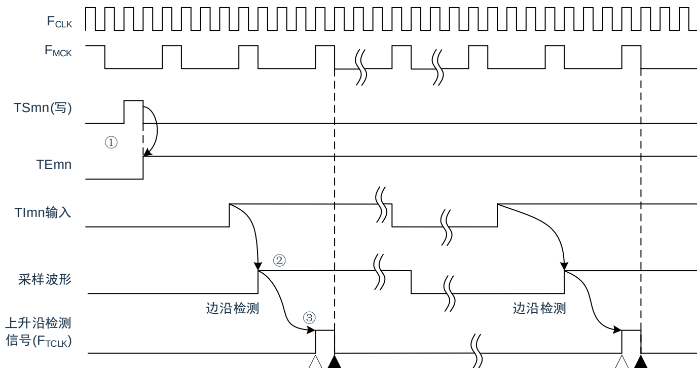
图 5-23: 计数时钟 ( F_{TCLK} ) 的时序 (CCSmn=1, 未使用噪声滤波器的情况)
