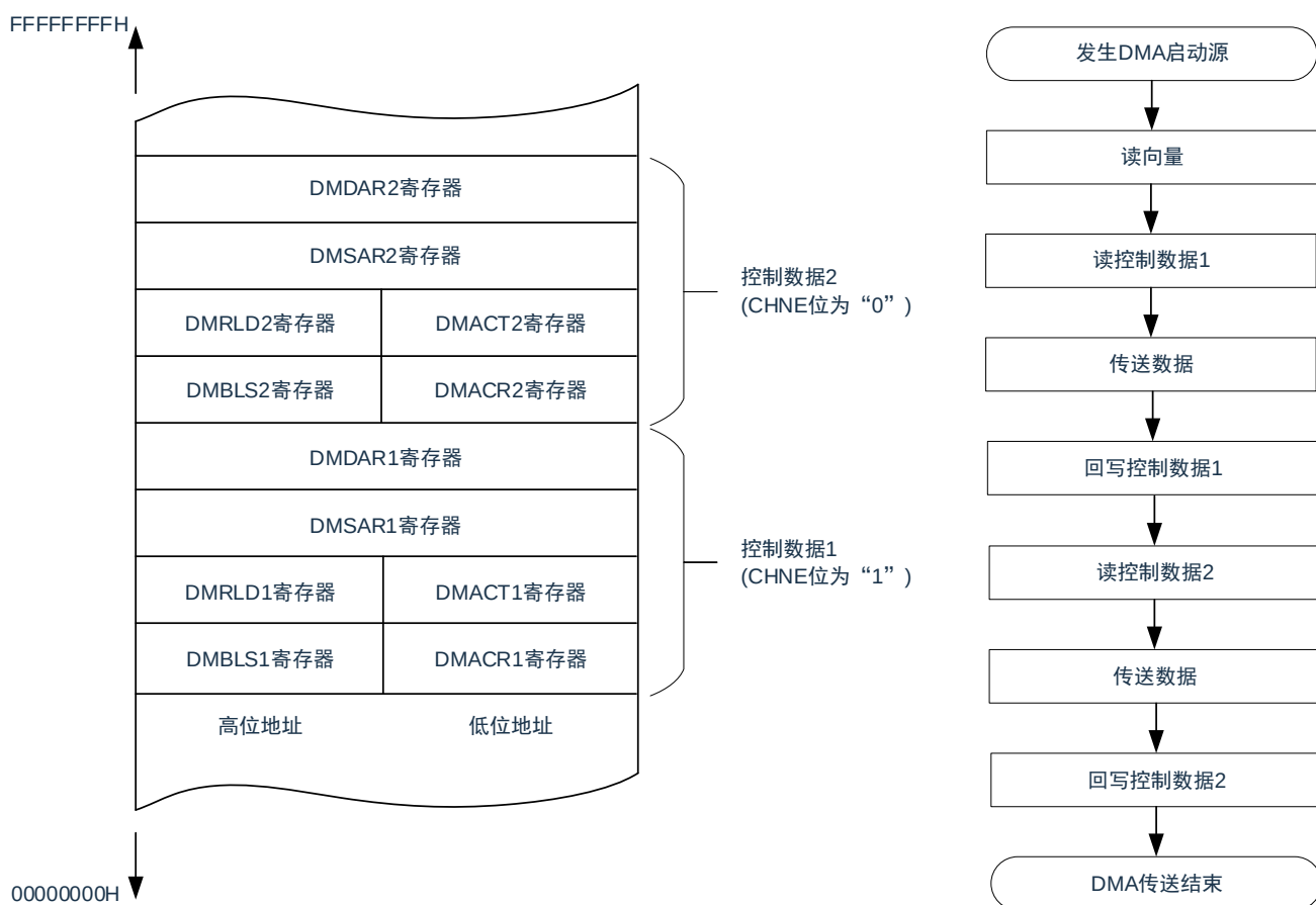
图 20-21：链传送的流程图
