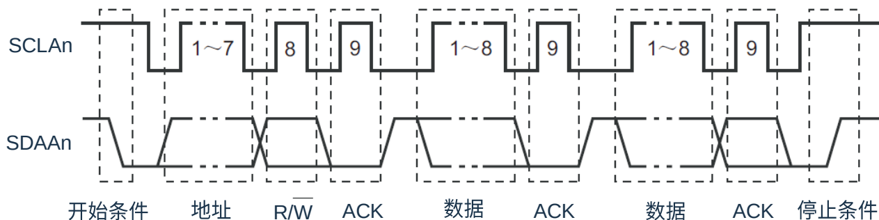
图 17-13: I 2 C 总线的串行数据传送时序
