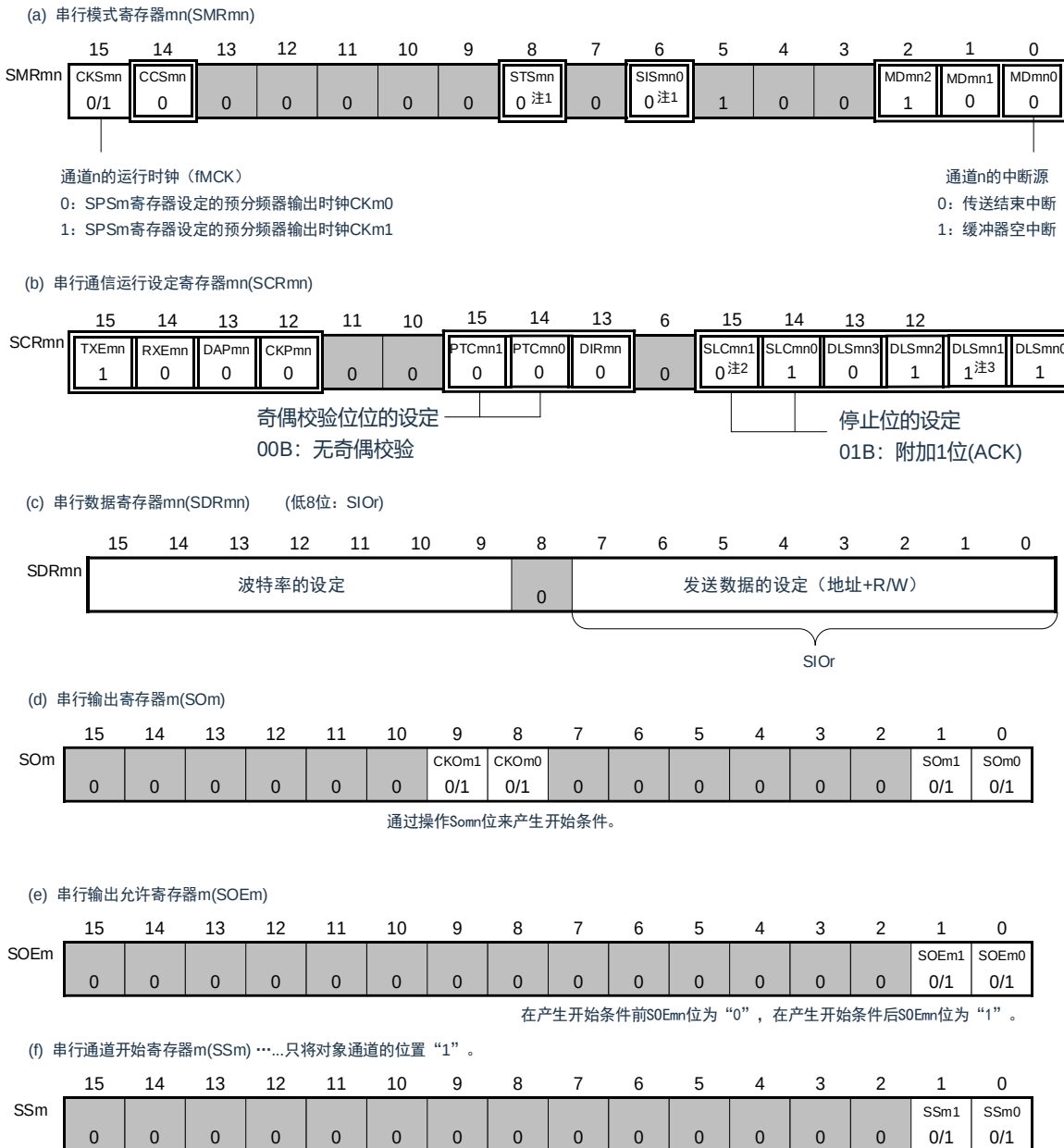
图 15-122：简易 I 2 C（IIC00、IIC01、IIC10、IIC11、IIC20、IIC21）地址段发送时的寄存器设定内容例子
