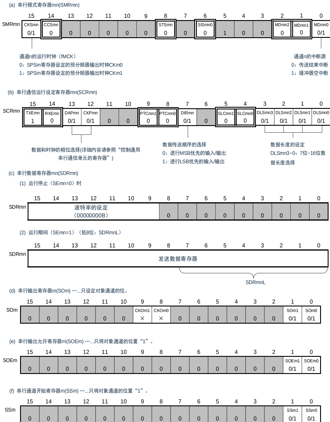
图 15-47：3 线串行 I/O（SSPI00、SSPI01、SSPI10、SSPI11、SSPI20、SSPI21）
