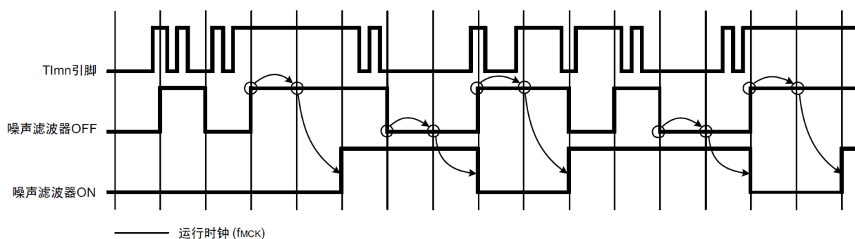
图 5-39：TImn 输入引脚在噪声滤波器 ON 或者 OFF 情况下的采样波形
