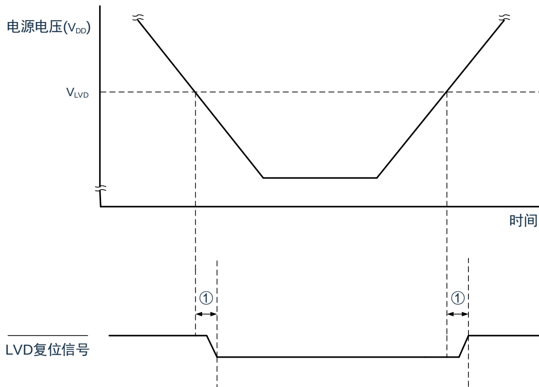
图 27-10：从产生 LVD 复位源到产生或者解除 LVD 复位的延迟
