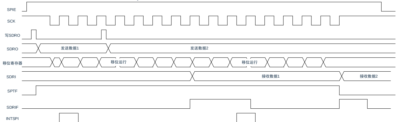
图 16-10: 发送/接收时序(连续发送模式)的时序图 (INTMD=1,CPHA=1、CPOL=1)
