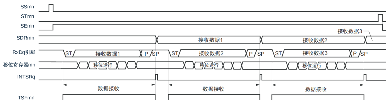
图 15-108: UART 接收的时序图
