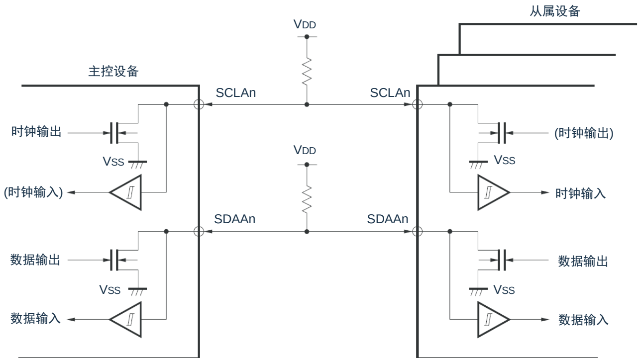
图 17-12: 引脚结构图
