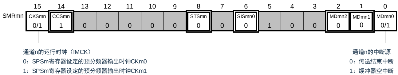
图 15-87：从属选择输入功能（SSPImn）从属发送和接收时的寄存器设定内容例子(1/2)
