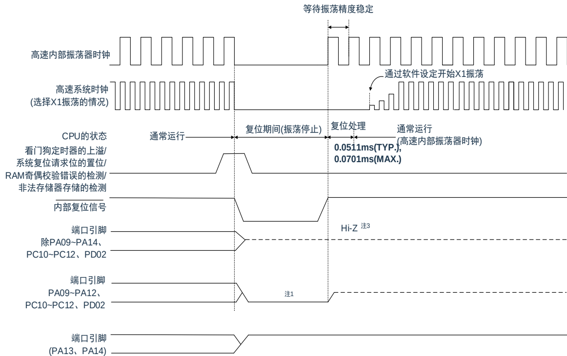
图 25-3: 因看门狗定时器的上溢、系统复位请求位的置位、RAM 奇偶校验错误的检测 或者非法存储器存取检测而产生的复位时序
