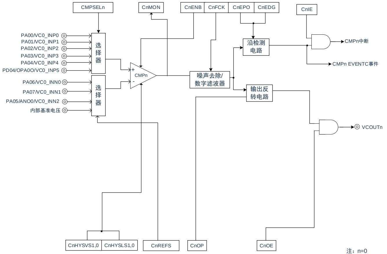
图 13-1：比较器 0 的框图
