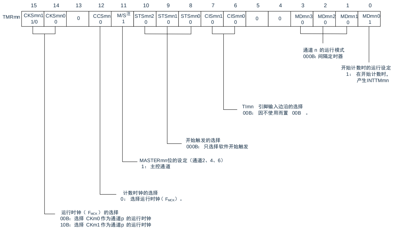
图 5-67: PWM 功能时（主控通道）的寄存器设定内容例子
