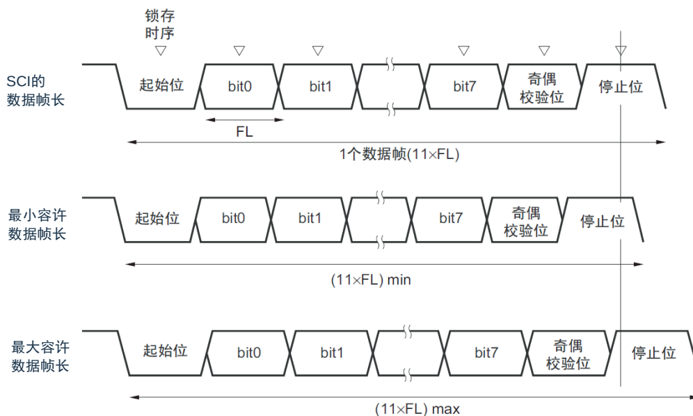
图 15-114: 接收时的波特率容许范围 (1 个数据的帧长=11 位的情况)
