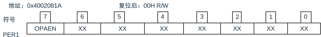
图 14-1: 外围允许寄存器 1 (PER1)
