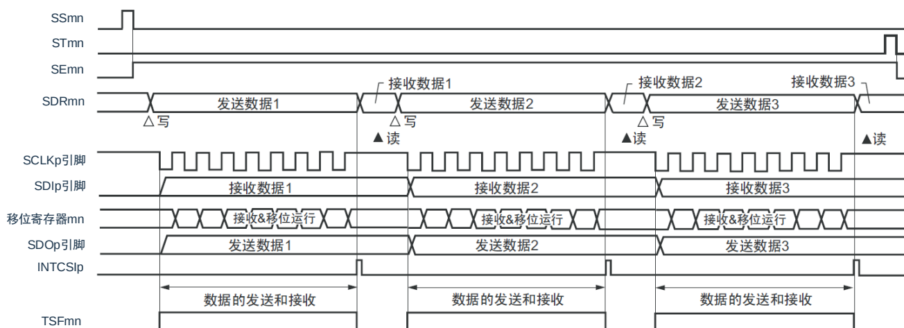
图 15-43：主控发送和接收（单次发送和接收模式）的时序图（类型 1：DAPmn=0、CKPmn=0）
