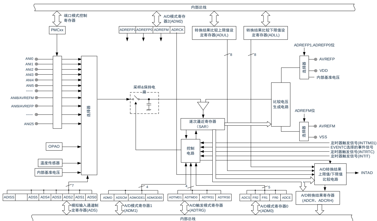
图 11-1: A/D 转换器的框图
