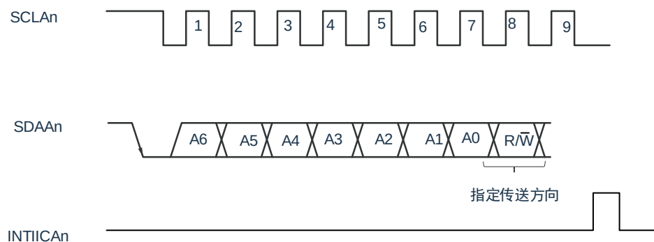
图 17-16: 传送方向的指定
