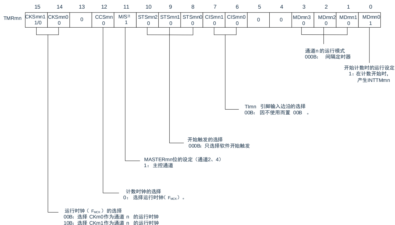
图 5-73：多重 PWM 输出功能时（主控通道）的寄存器设定内容例子
