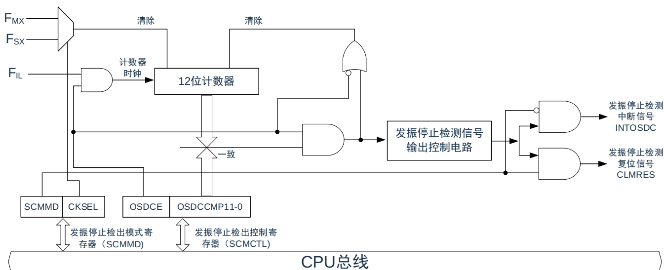
图 4-24：发振停止检测电路的框图（例）
