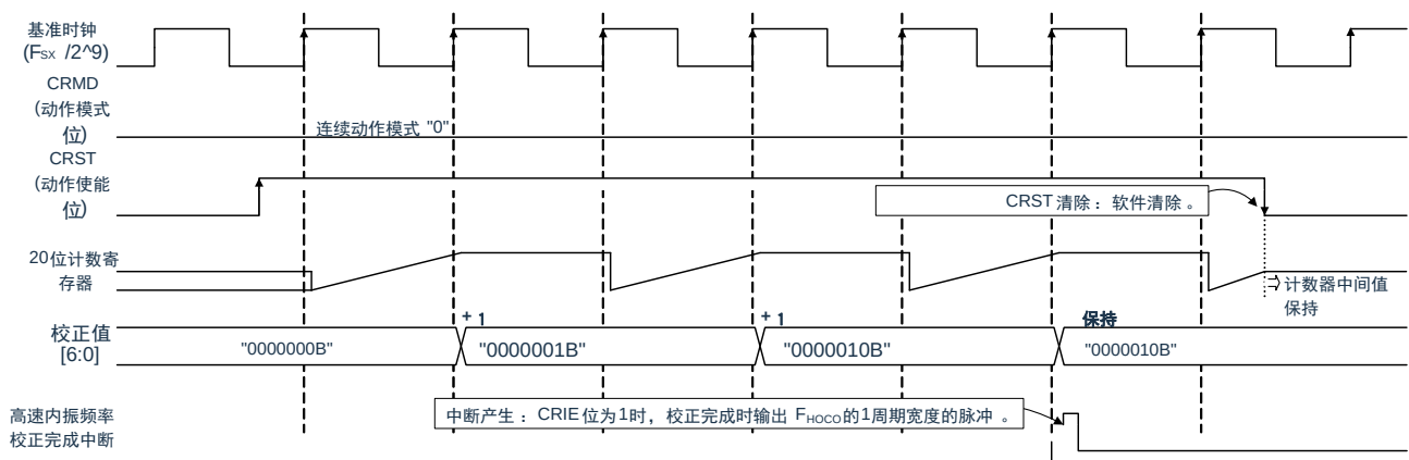
图 4-21：连续动作模式时序图
