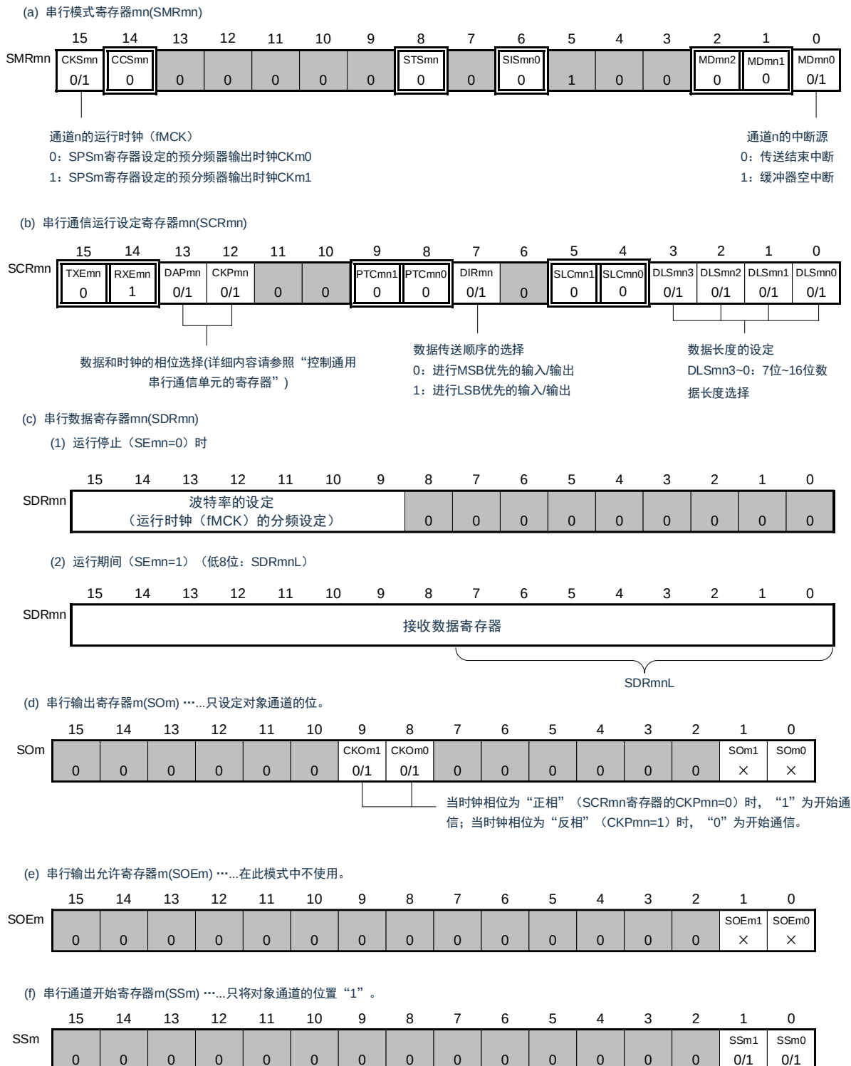
图 15-31: 3 线串行 I/O (SSPI00、SSPI01、SSPI10、SSPI11、SSPI20、SSPI21)
