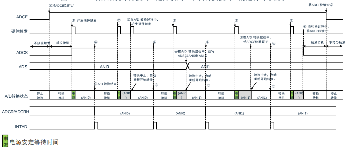
图 11-28：硬件触发等待模式（选择模式、单次转换模式）的运行时序例子
