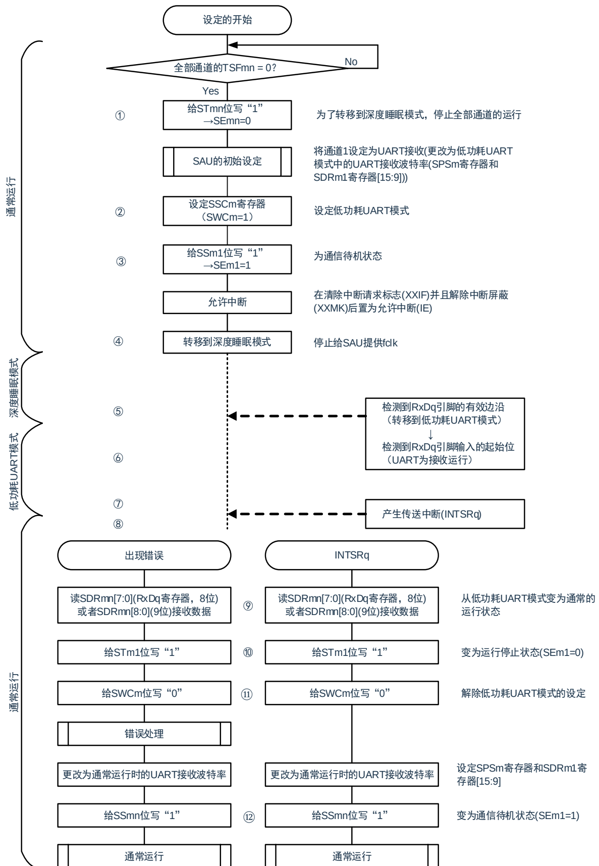
图 15-111: 低功耗 UART 模式运行 (SSECm=0/1) 的流程图
