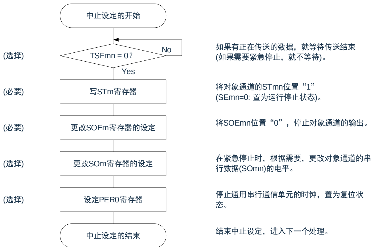
图 15-63：从属发送和接收的中止步骤
