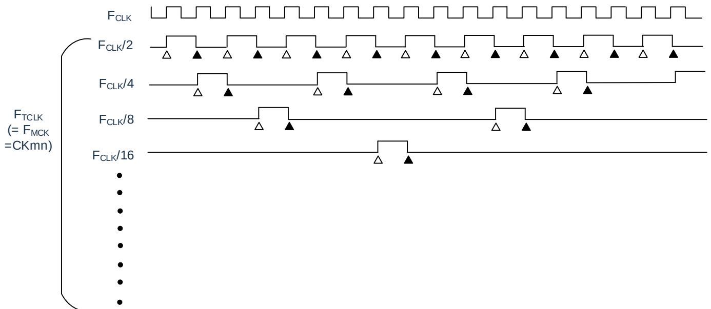
图 5-22: F_{CLK} 和计数时钟 ( F_{TCLK} ) 的时序 ( CCSmn=0 的情况)
