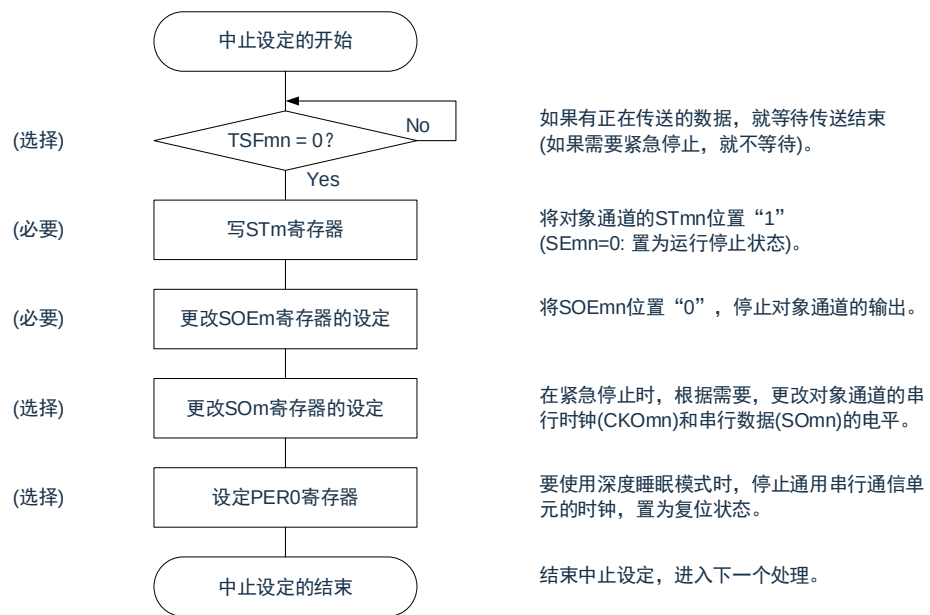
图 15-25: 主控发送的中止步骤
