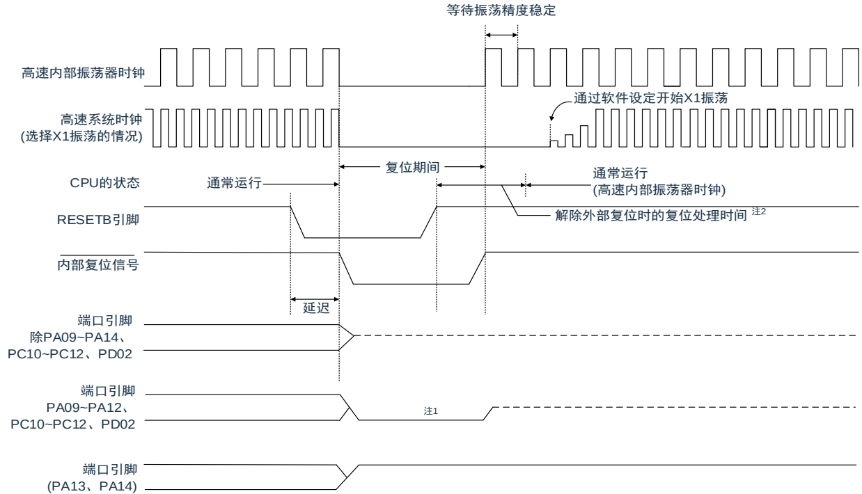
图 25-2: RESETB 输入的复位时序
