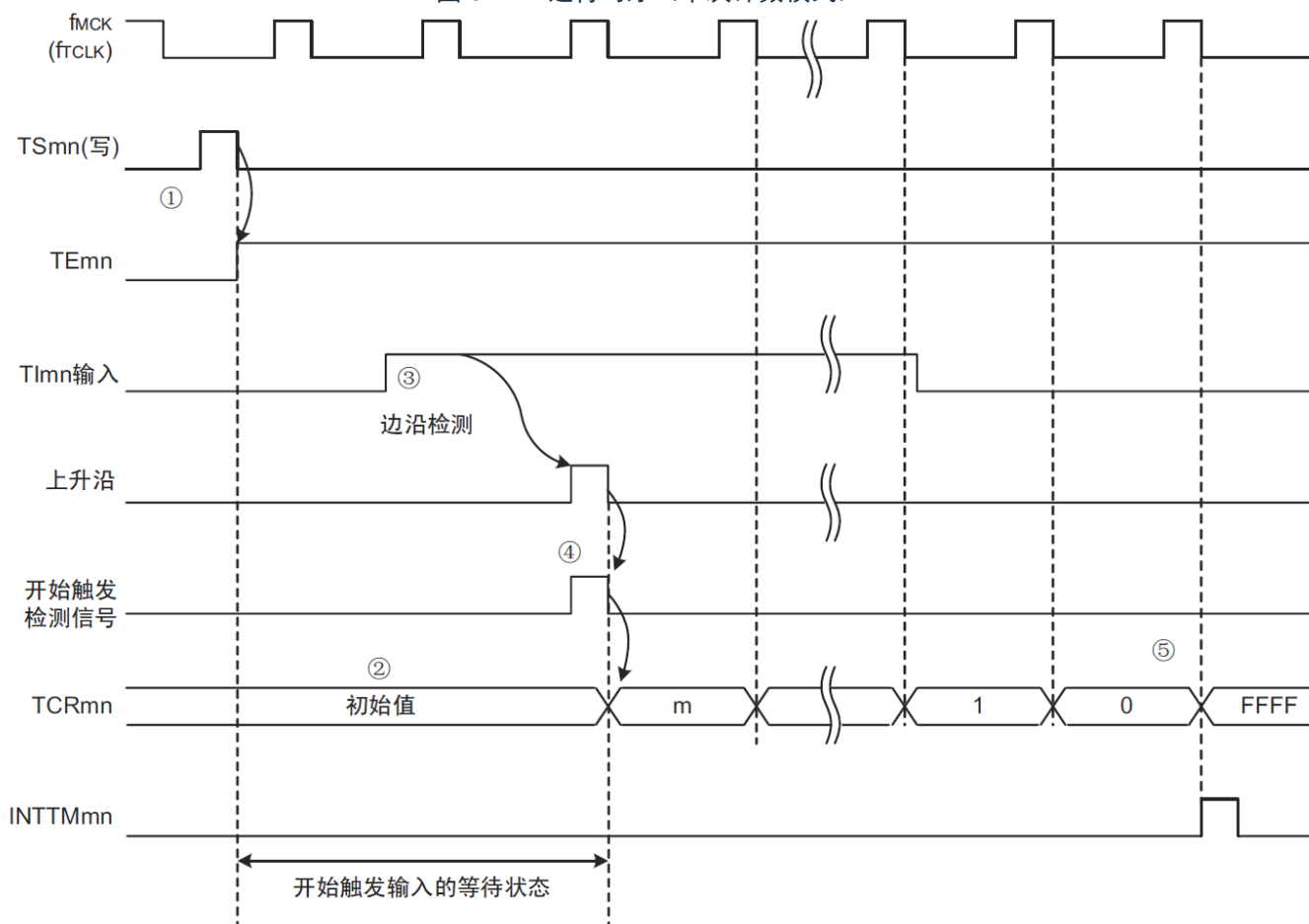
图 5-27：运行时序（单次计数模式）
