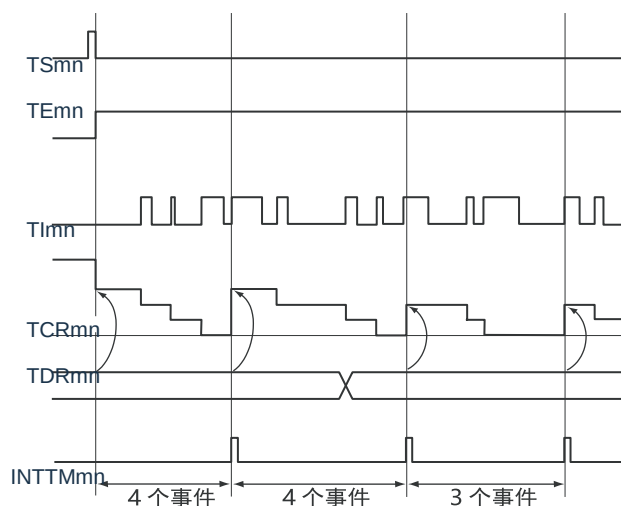
图 5-44：作为外部事件计数器运行的基本时序例子
