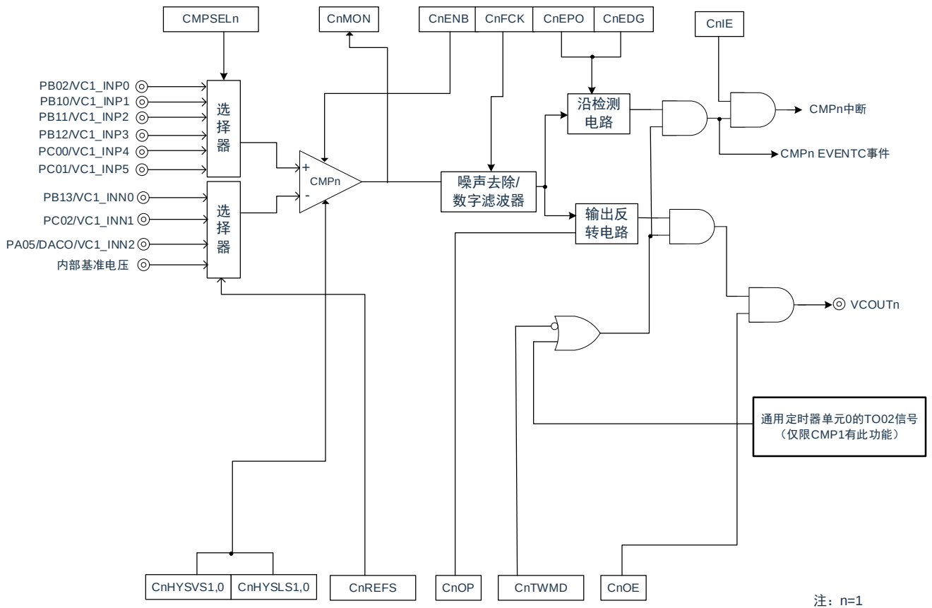
图 13-2：比较器 1 的框图
