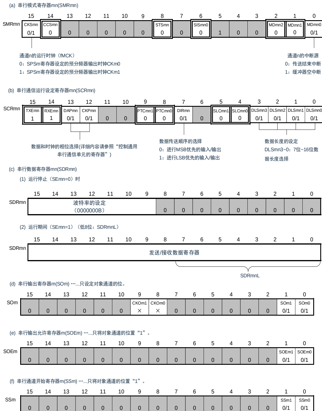
图 15-61: 3 线串行 I/O (SSPI00、SSPI01、SSPI10、SSPI11、SSPI20、SSPI21)
