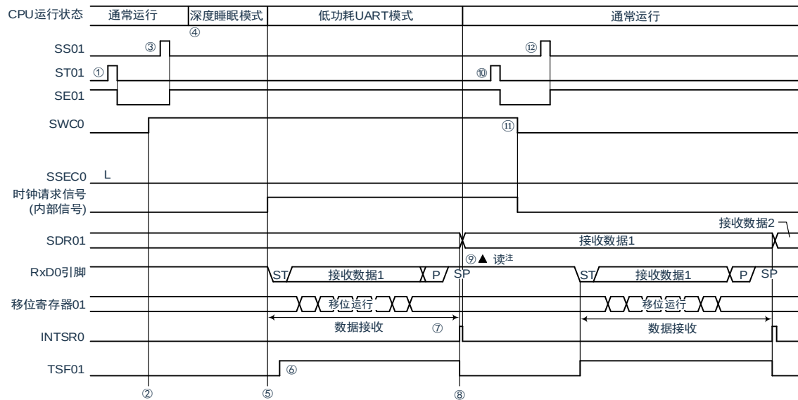
图 15-110: 低功耗 UART 模式运行 (SSECm=0/1) 时序图
