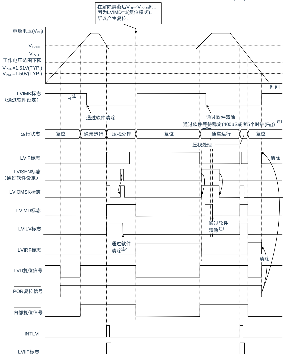
图 27-6：中断&复位信号的产生时序（选项字节的 LVIMDS1、LVIMDS0=1、0）(2/2)
