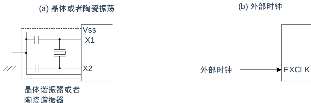
图 4-13：X1 振荡电路的外接电路例子
