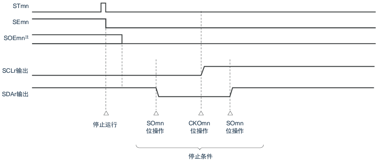
图 15-132：产生停止条件的时序图
