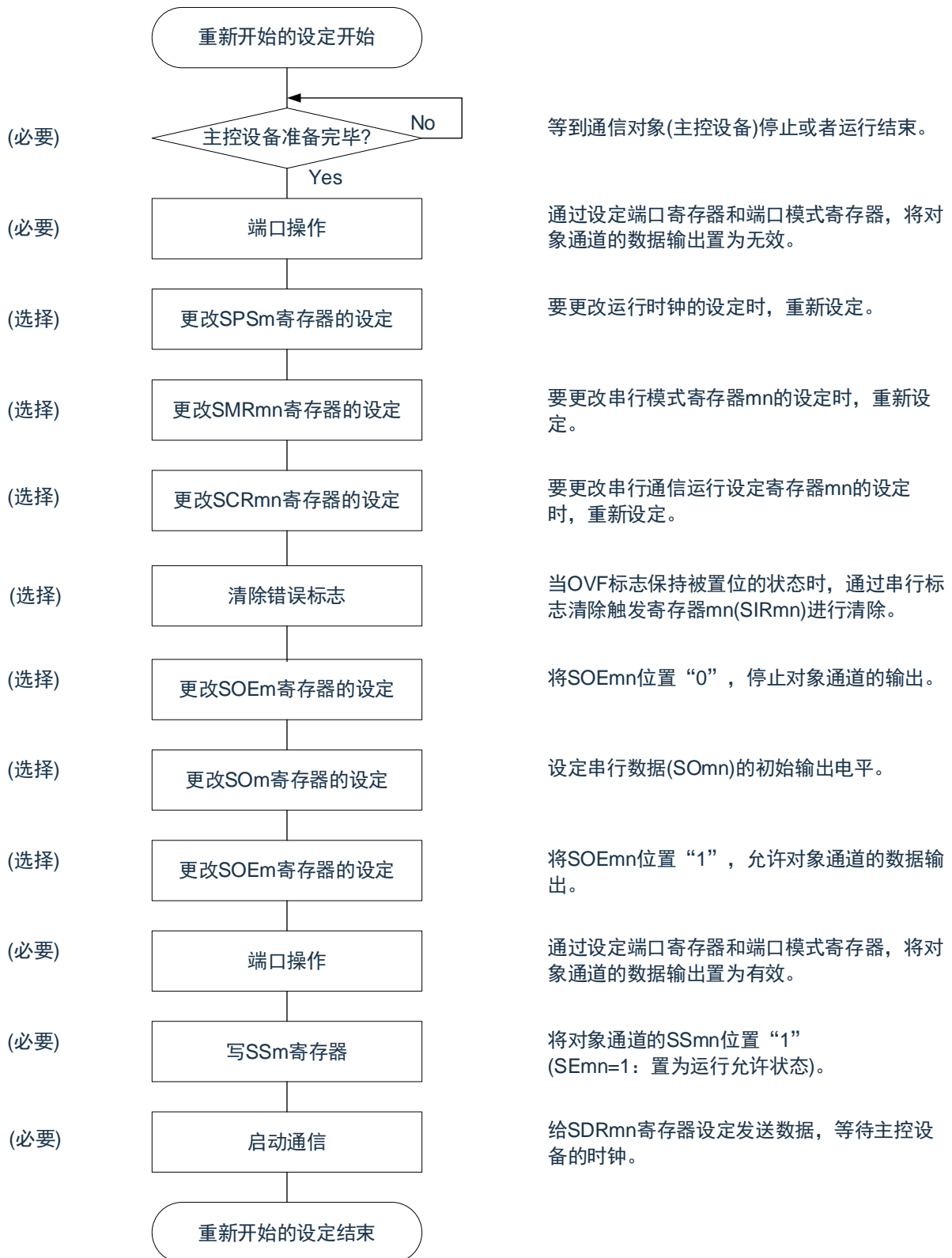
图 15-64: 重新开始从属发送和接收的设定步骤
