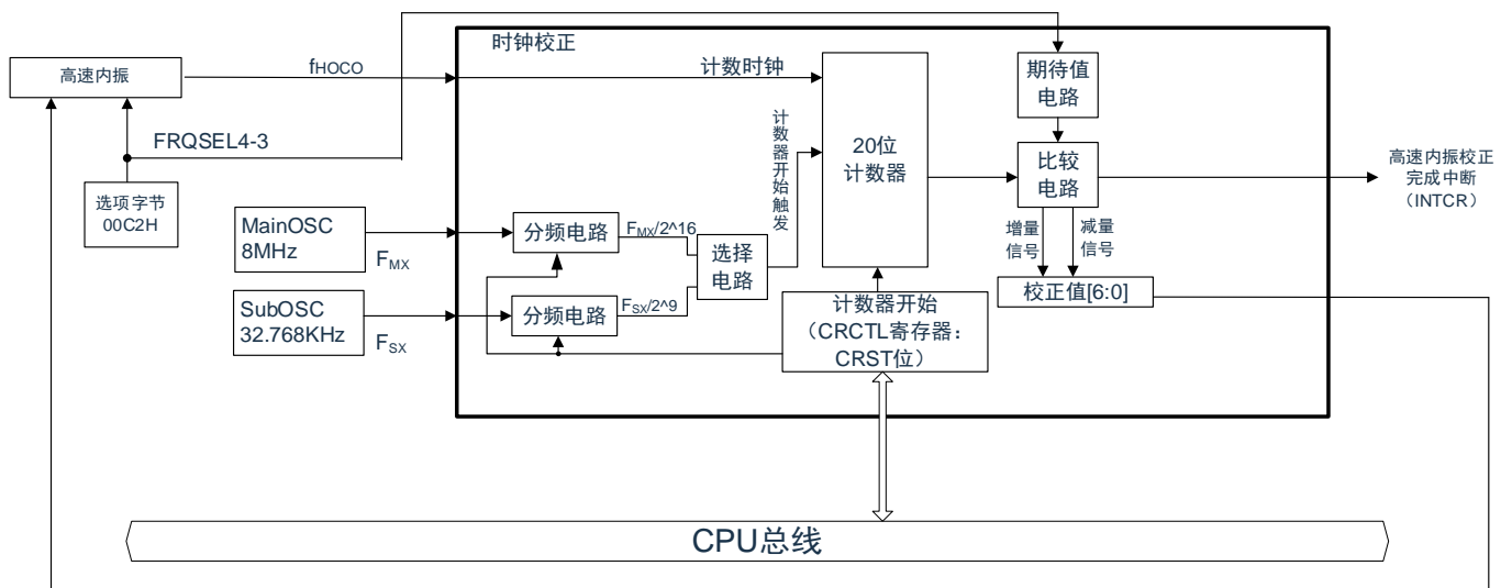
图 4-18：高速内振频率校正功能的动作框图
