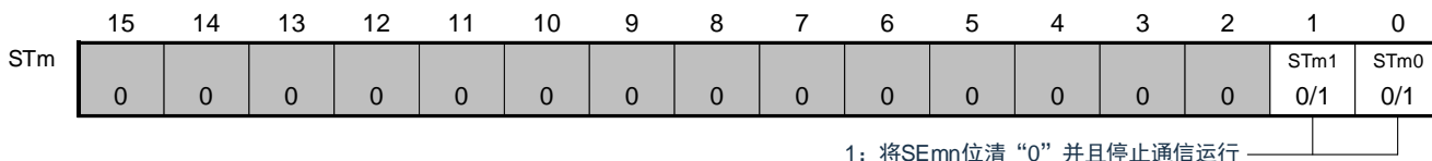
图 15-22: 按通道停止运行时的各寄存器的设定
