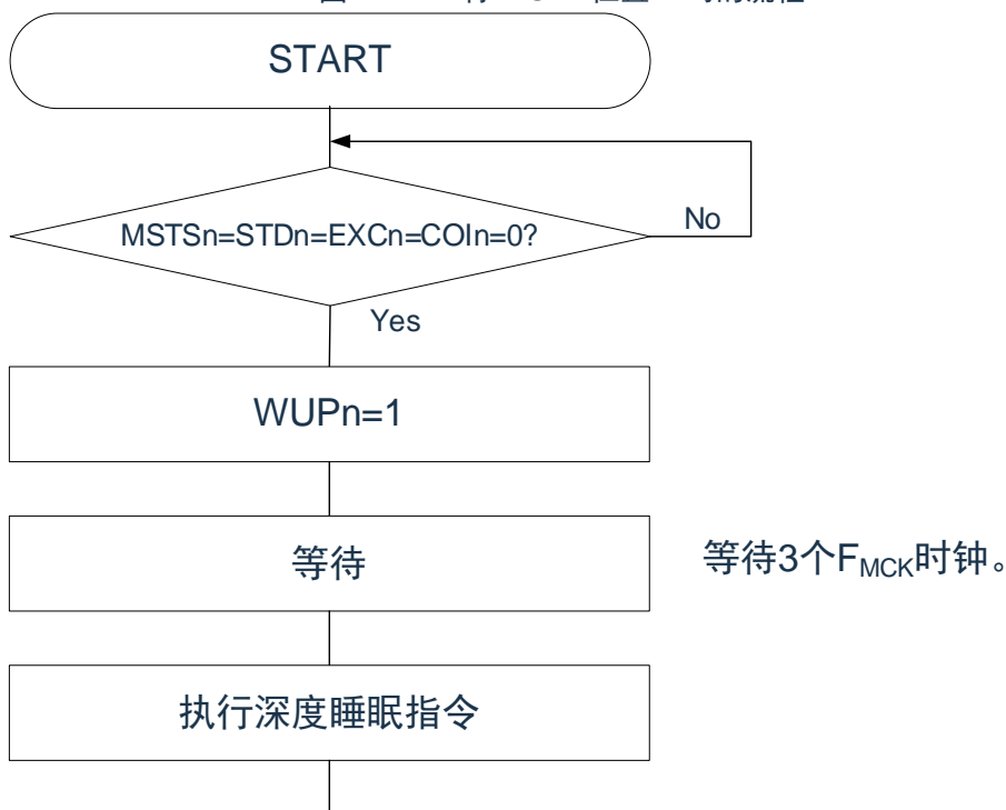
图 17-21：将 WUPn 位置“1”时的流程
