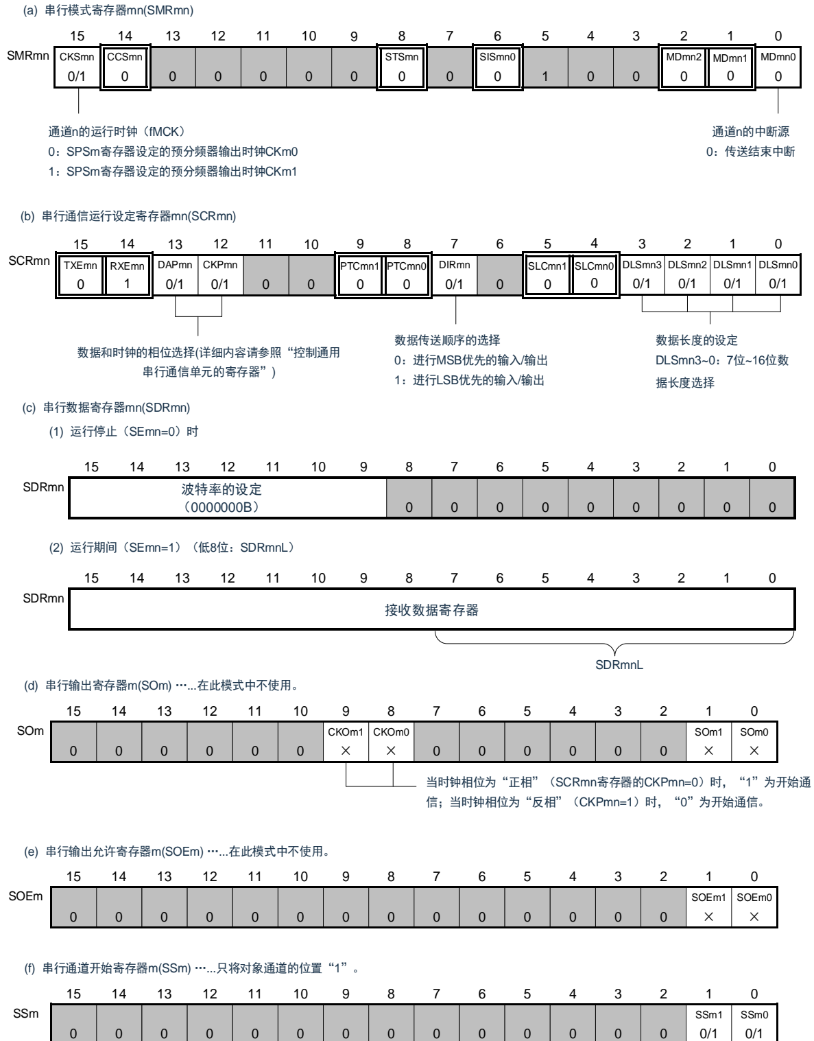
图 15-55: 3 线串行 I/O (SSPI00、SSPI01、SSPI10、SSPI11、SSPI20、SSPI21)
