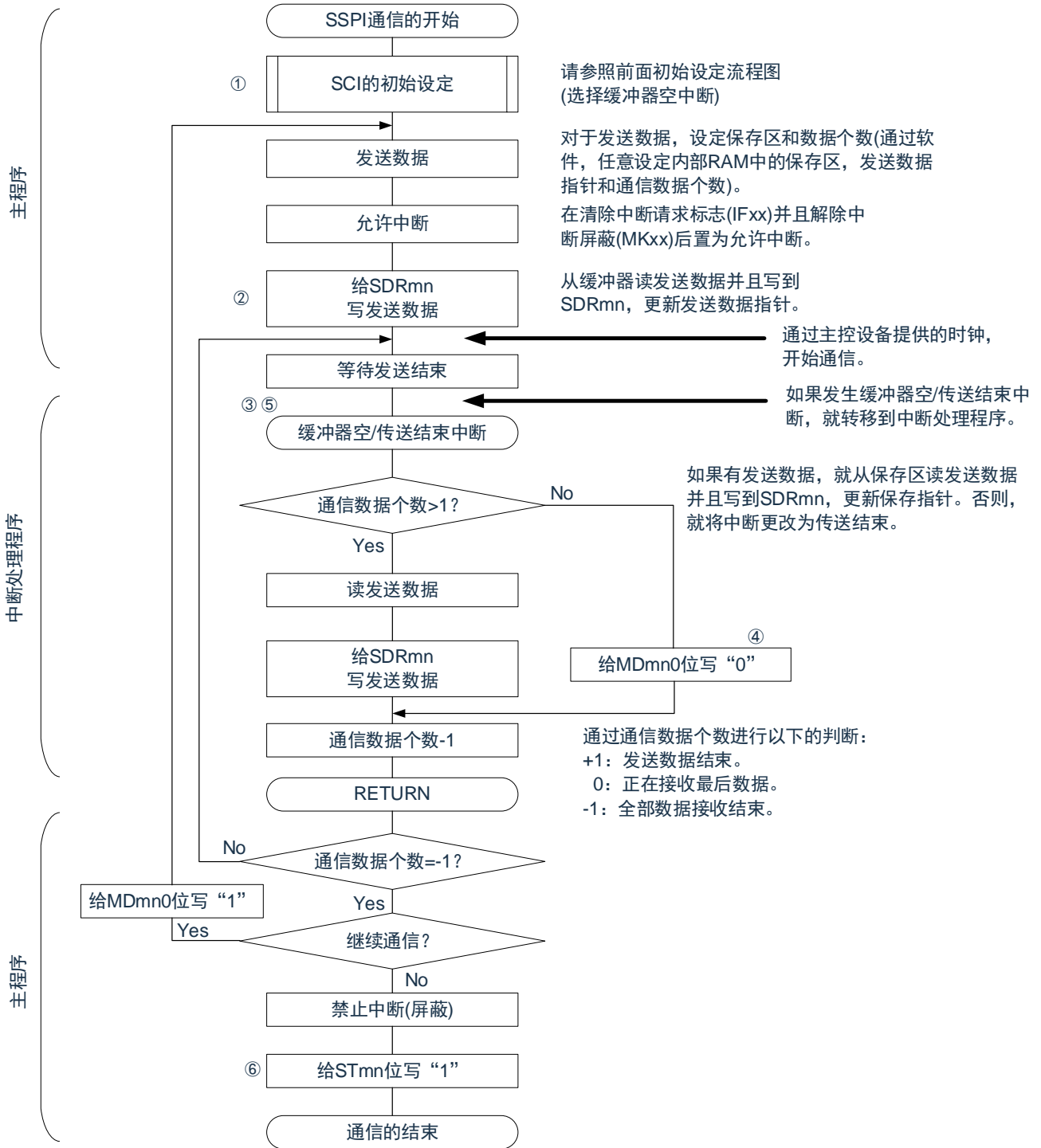
图 15-54: 从属发送（连续发送模式）的流程图
