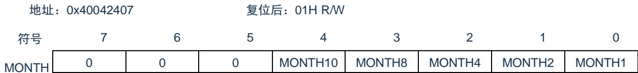
图 7-12: 月计数寄存器 (MONTH) 的格式
