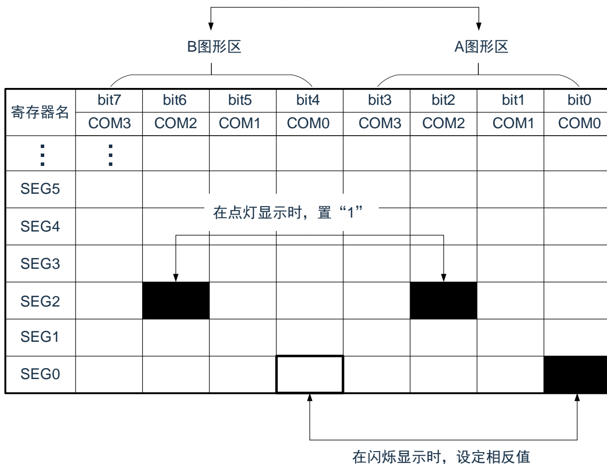
图 19-8：图形切换显示时的 LCD 显示寄存器的设定例子 在选择闪烁显示（BLCON=1）时， 交替显示A图形区和B图形区
