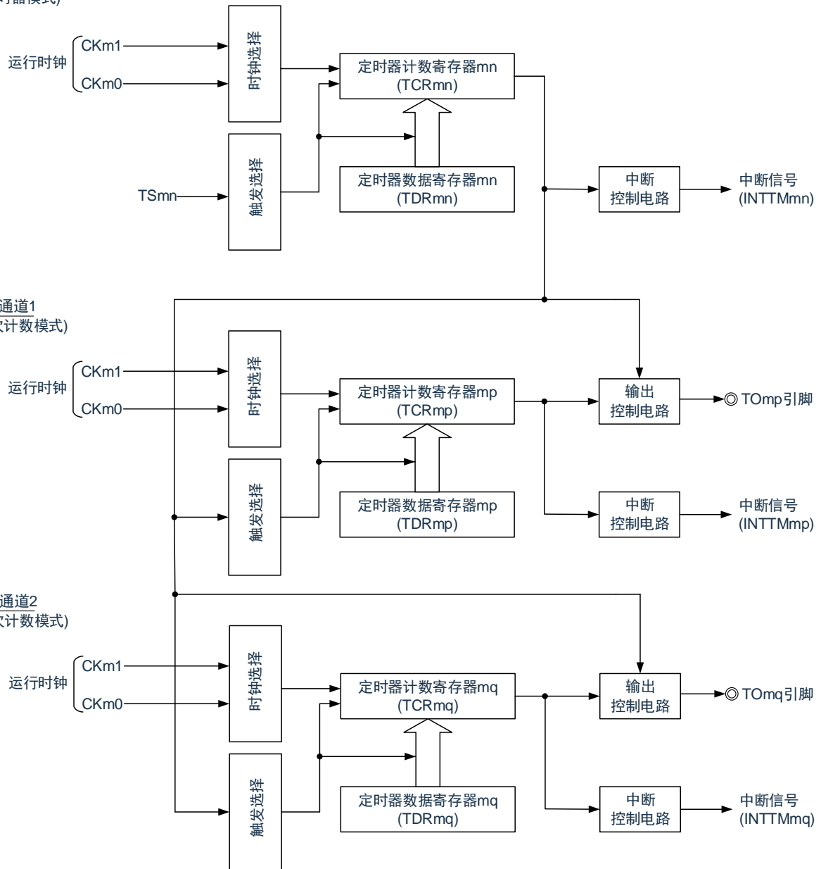
图 5-71: 作为多重 PWM 输出功能运行的框图 (输出 2 种 PWM 的情况)
