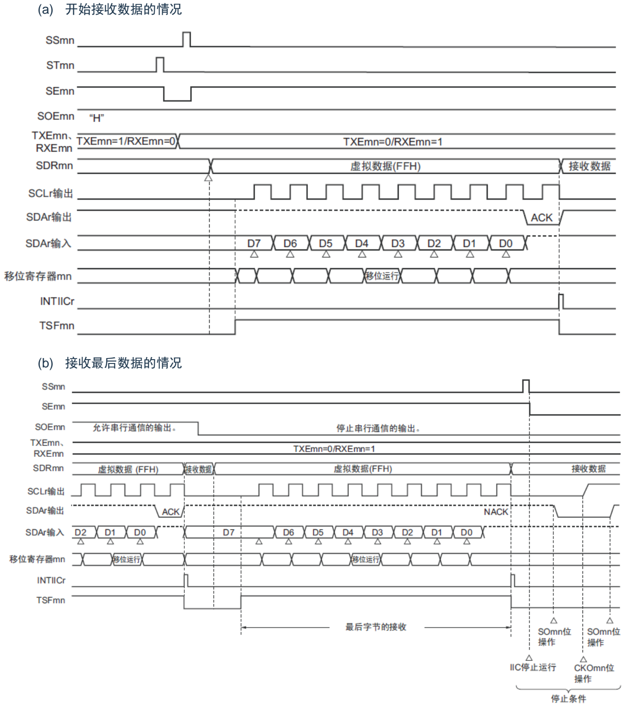
图 15-130: 数据接收的时序图
