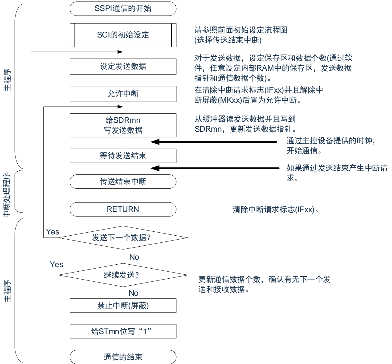
图 15-77: 从属发送（单次发送模式）的流程图
