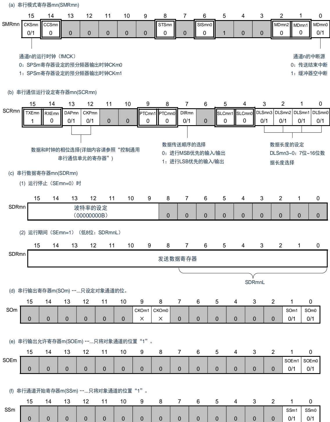
图 15-47: 3 线串行 I/O (SSPI00、SSPI01、SSPI10、SSPI11、SSPI20、SSPI21)
