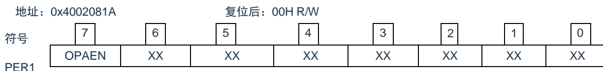
图 14-1: 外围允许寄存器 1 (PER1)
