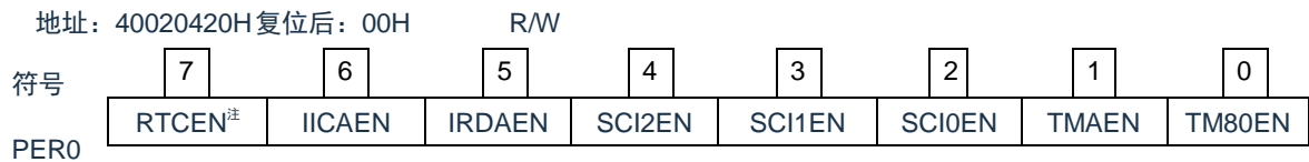
图 7-2: 外围允许寄存器 0 (PER0) 的格式
