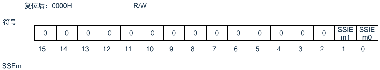
图 15-18: 从属选择功能启用寄存器 m (SSEm) 的格式
