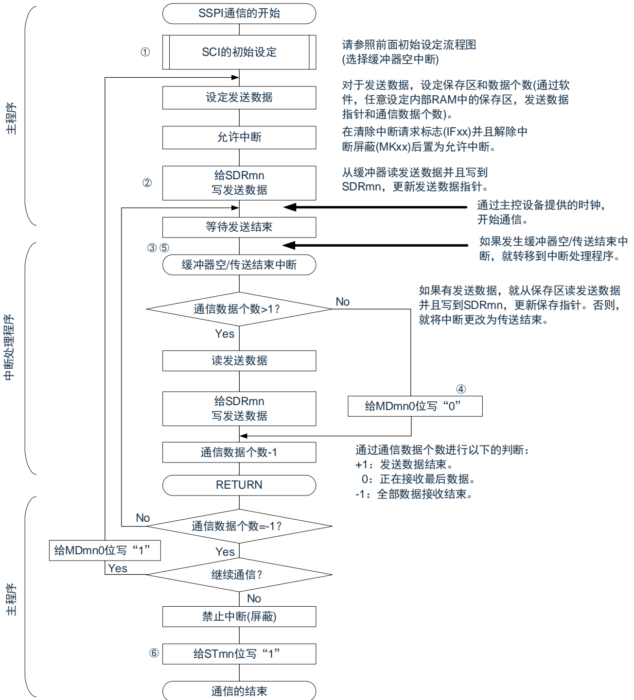
图 15-79: 从属发送（连续发送模式）的流程图
