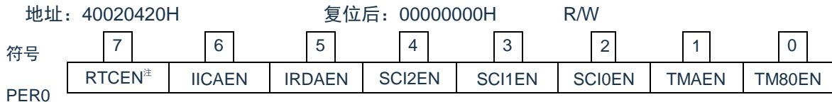
图 5-4: 外围允许寄存器 0 (PER0) 的表格
