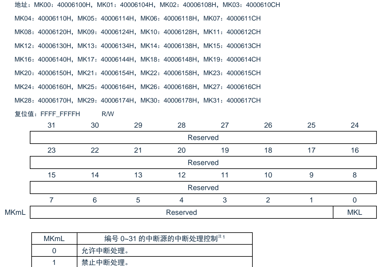
图 22-3: 中断请求屏蔽寄存器 (MKm) 的格式 (m=0~31)
