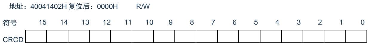
图 28-5: CRC 数据寄存器 (CRCD) 的格式
