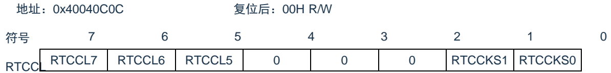
图 7-3: 实时时钟选择寄存器 (RTCCL) 的格式
