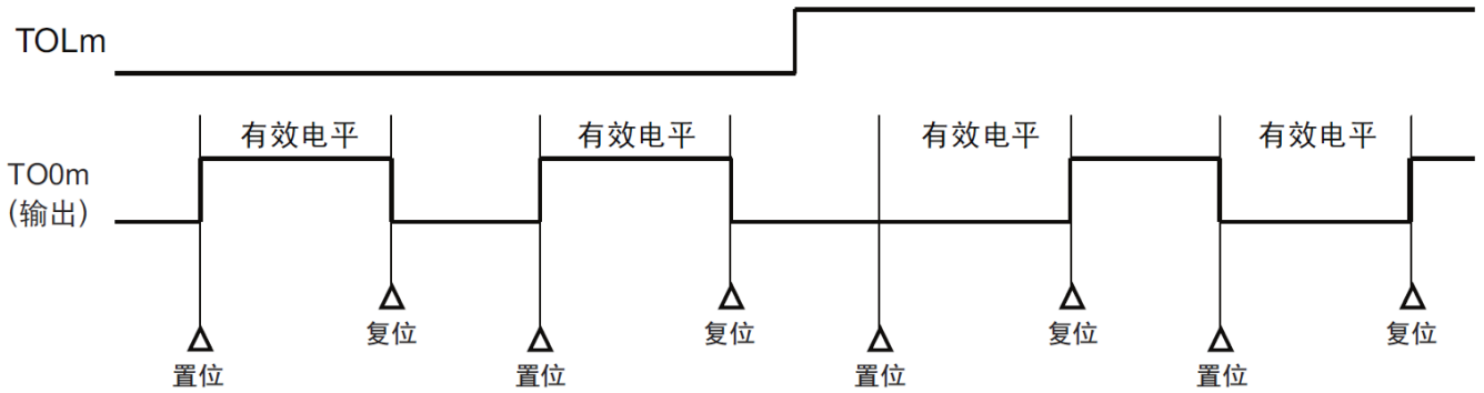
图 5-33: 在定时器运行中更改 TOLm 寄存器的内容时的运行
