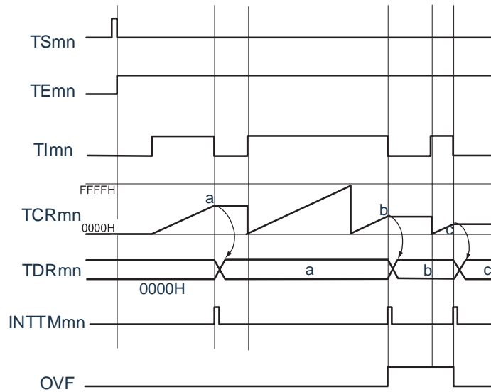
图 5-53: 作为输入信号高低电平宽度测量的运行基本时序例子
