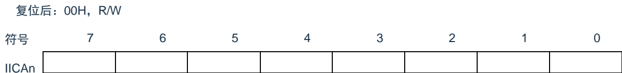
图 17-3: IICAn 移位寄存器 n (IICAn) 的格式
