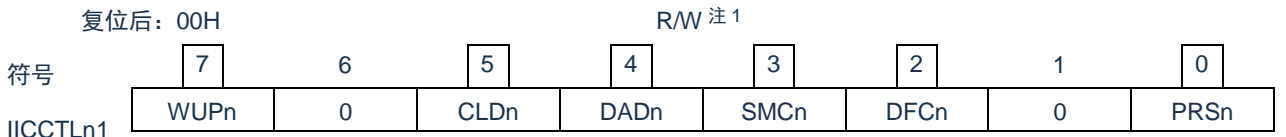
图 17-9: IICA 控制寄存器 n1 (IICCTLn1) 的格式(1/2)
