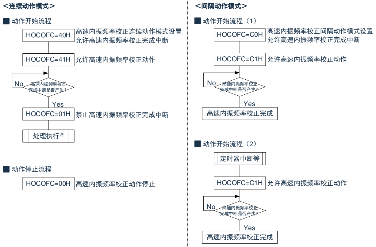
图 4-23: 动作模式设定流程 (例)
