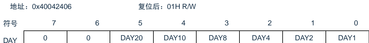
图 7-10: 日计数寄存器 (DAY) 的格式
