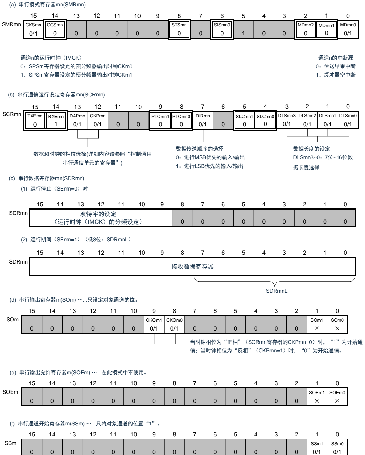
图 15-31: 3 线串行 I/O (SSPI00、SSPI01、SSPI10、SSPI11、SSPI20、SSPI21)
