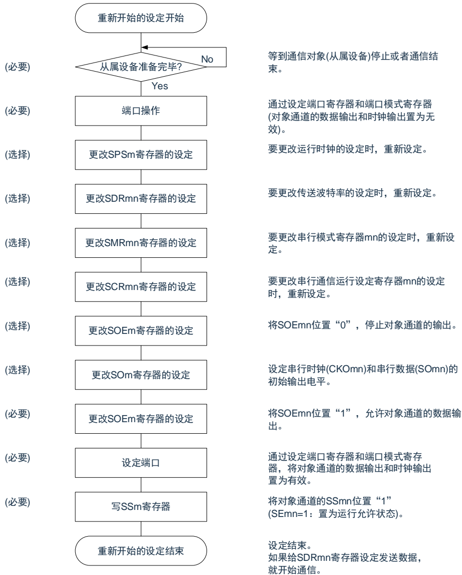
图 15-26: 重新开始主控发送的设定步骤
