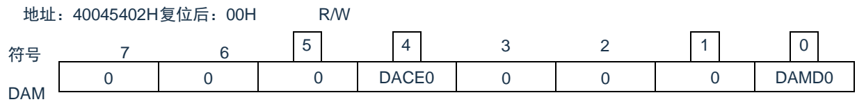
图 12-3: D/A 转换器的模式寄存器（DAM）的格式
