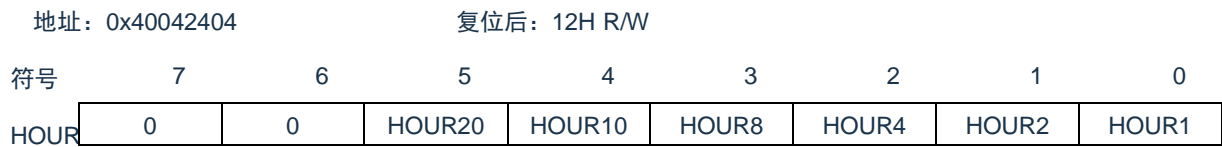
图 7-9: 小时计数寄存器 (HOUR) 的格式
