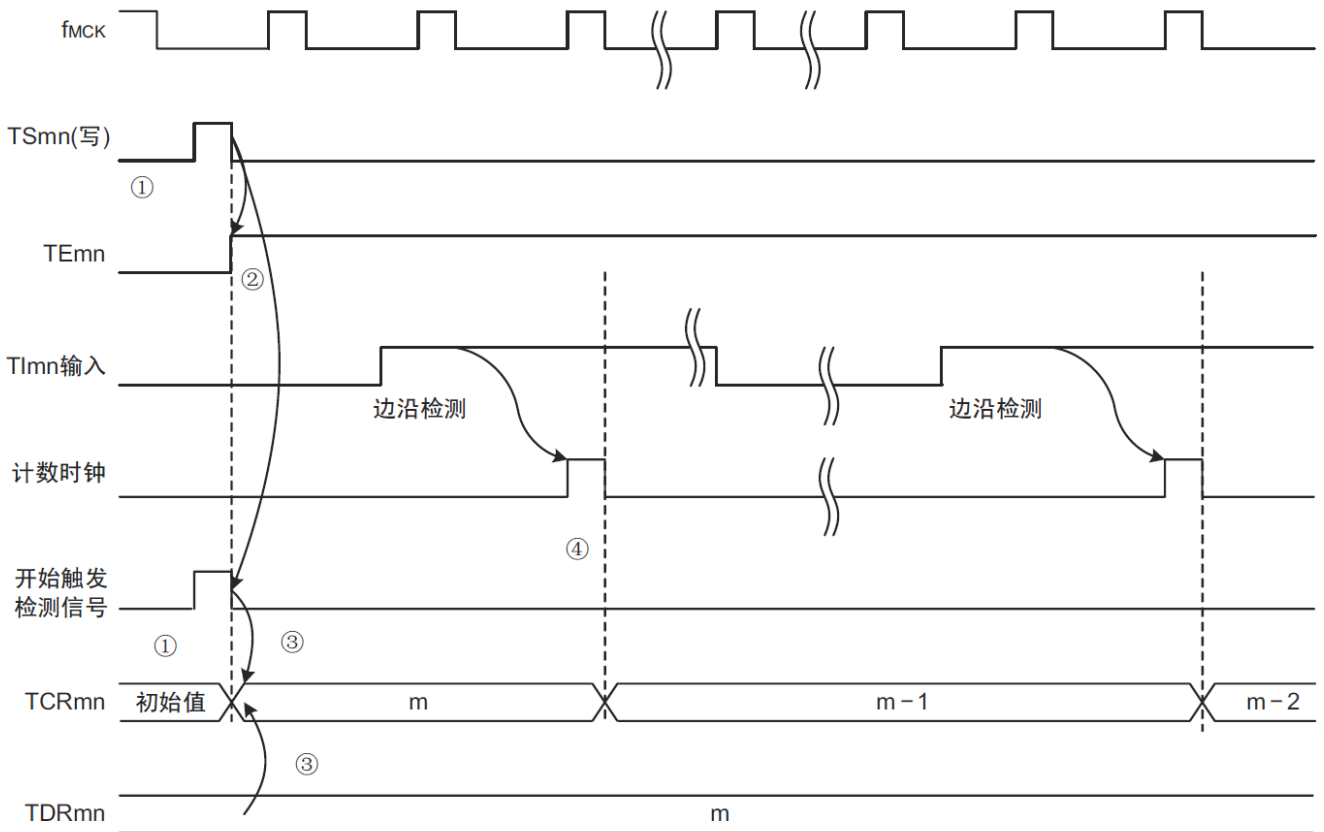
图 5-25: 运行时序 (事件计数器模式)
