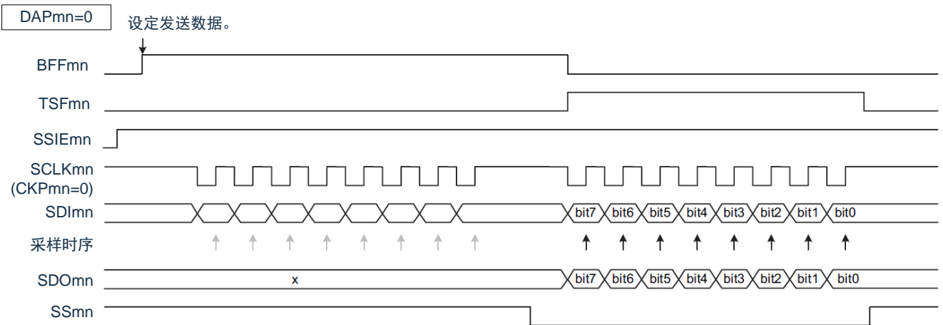
图 15-71：从属选择输入功能的时序图
