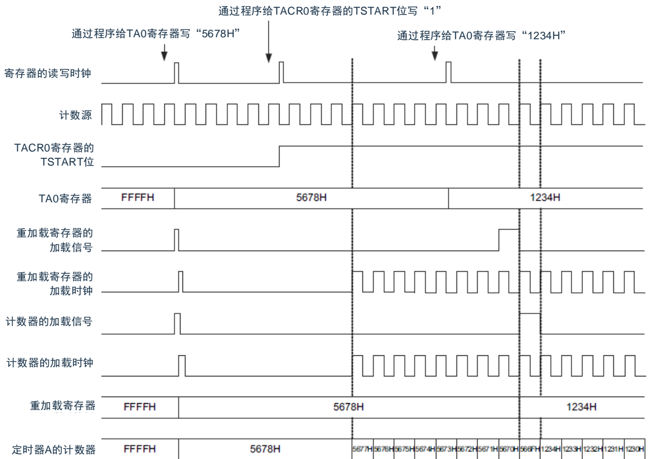
图 6-9：由 TSTART 位的值决定的改写时序图
