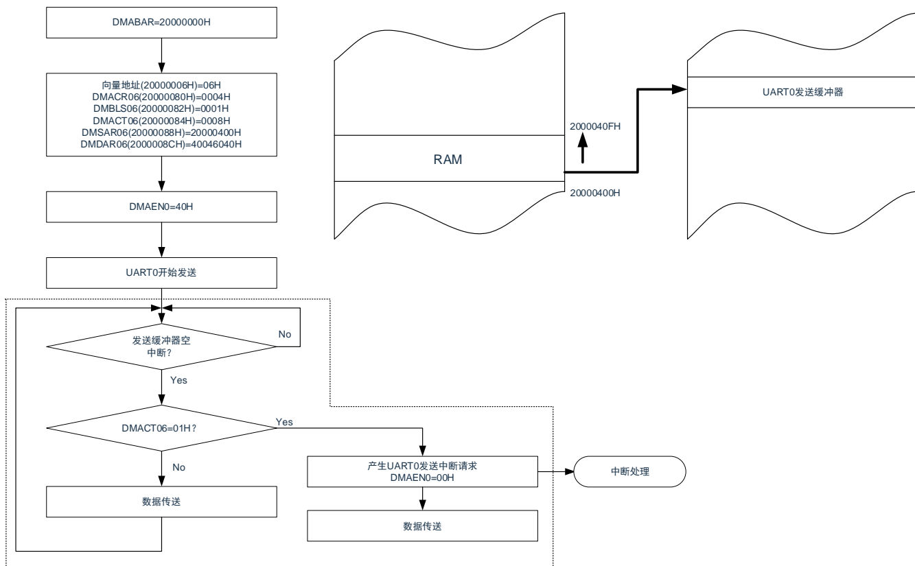
图 20-18: 正常模式的使用例子 2: UART0 连续发送
