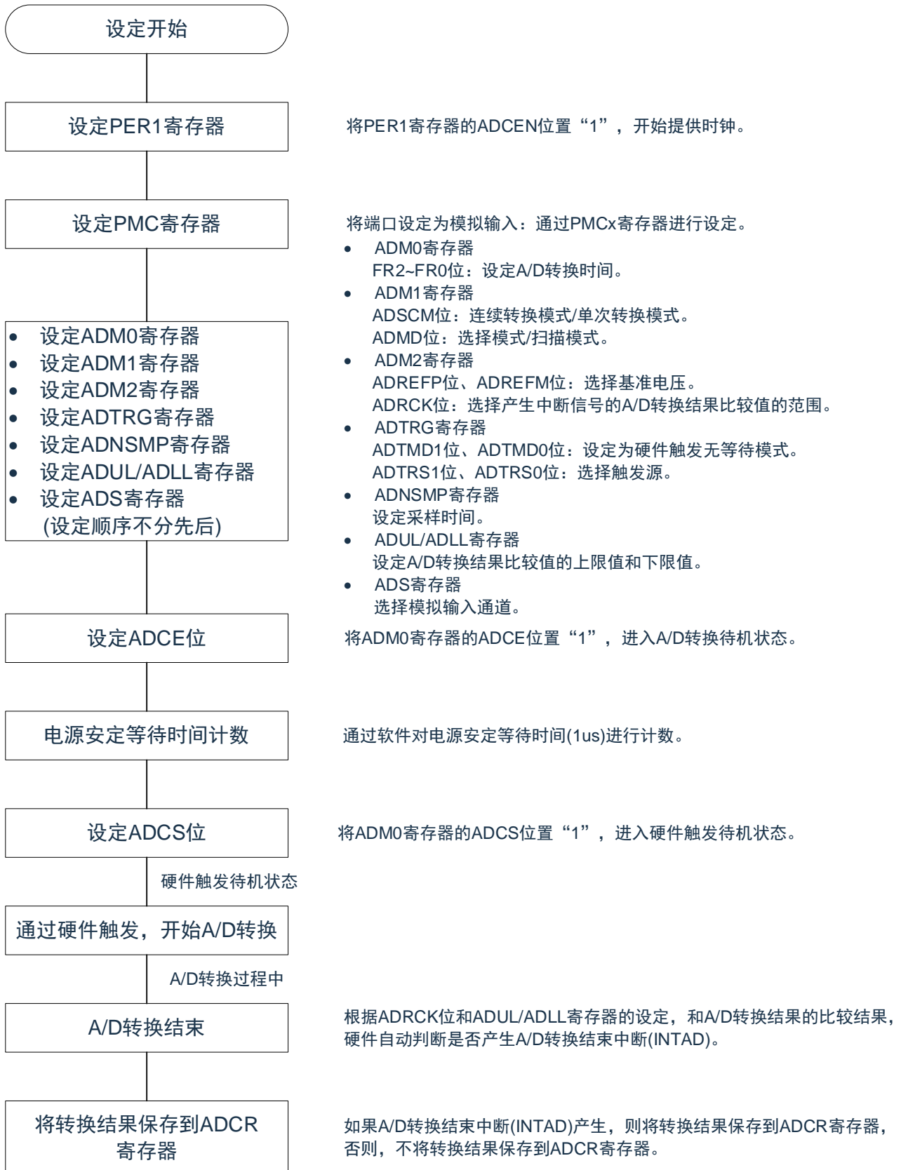
图 11-32：硬件触发无等待模式的设定
