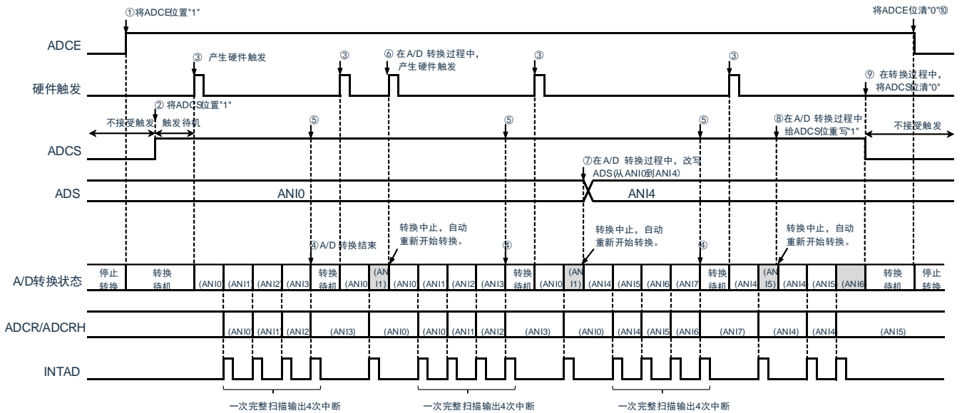
图 11-26: 硬件触发无等待模式（扫描模式、单次转换模式）的运行时序例子
