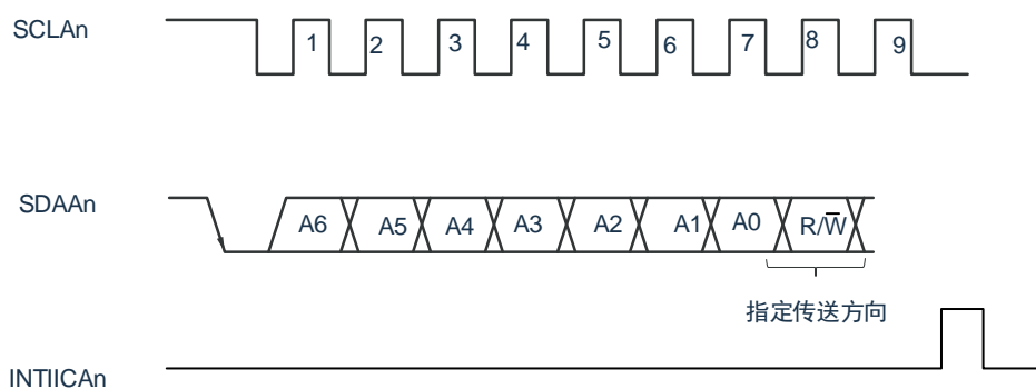
图 17-16: 传送方向的指定
