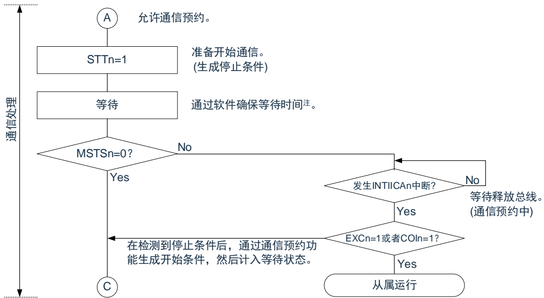
图 17-28: 多主控系统的主控运行(2/3)
