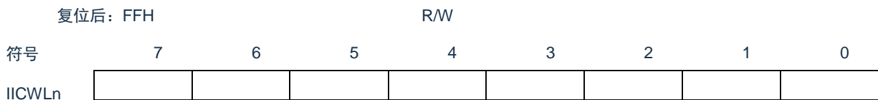
图 17-10: IICA 低电平宽度设定寄存器 n (IICWLn) 的格式
