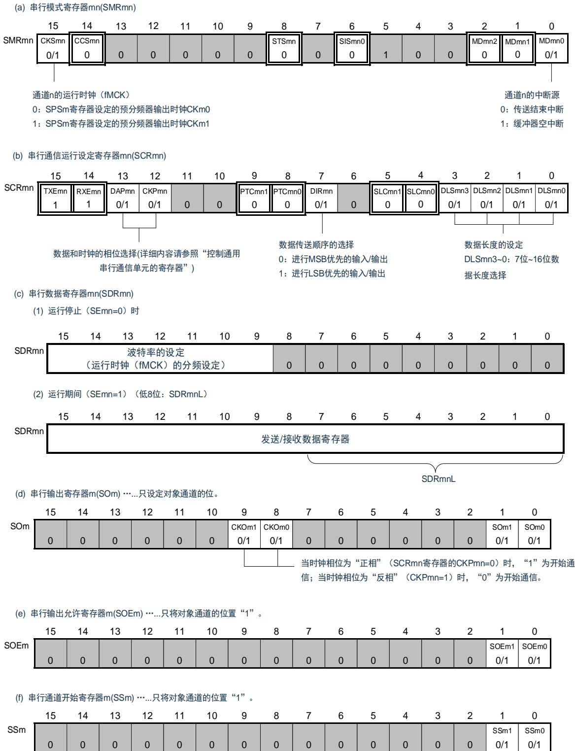
图 15-39: 3 线串行 I/O (SSPI00、SSPI01、SSPI10、SSPI11、SSPI20、SSPI21)
