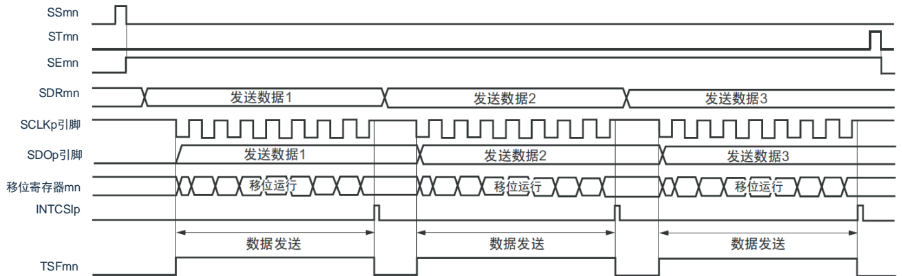
图 15-51：从属发送（单次发送模式）的时序图（类型 1：DAPmn=0、CKPmn=0）
