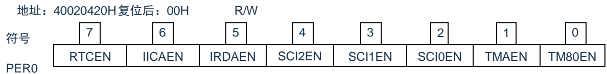
图 18-2: 外围允许寄存器 0 (PER0) 的格式
