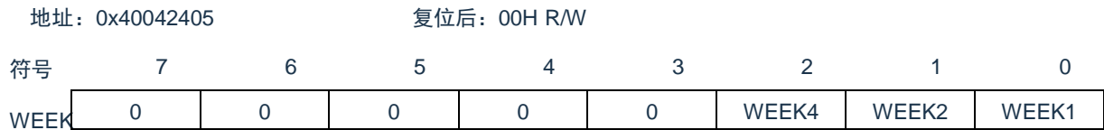
图 7-11：星期计数寄存器 (WEEK) 的格式
