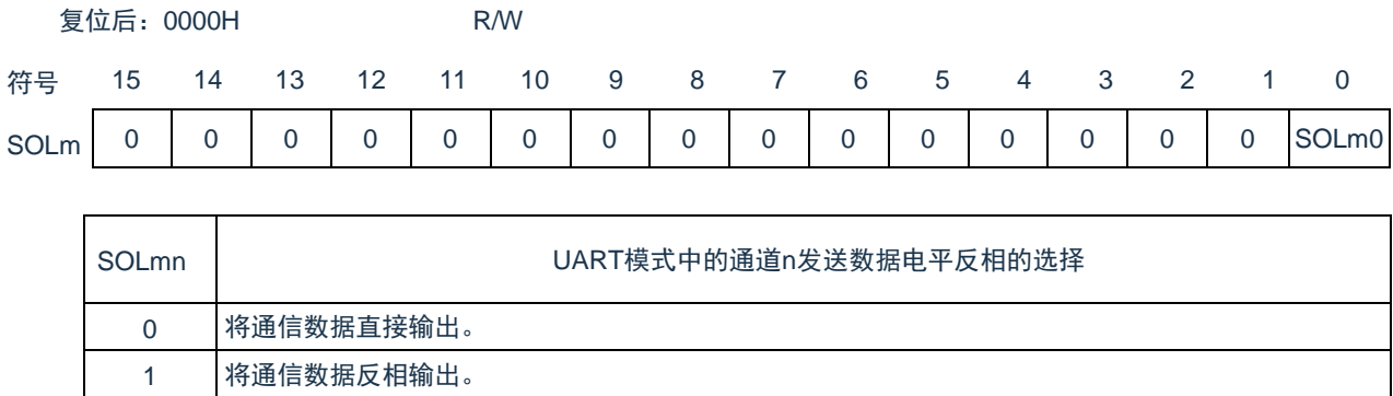
图 15-15: 串行输出电平寄存器 m (SOLm) 的格式
