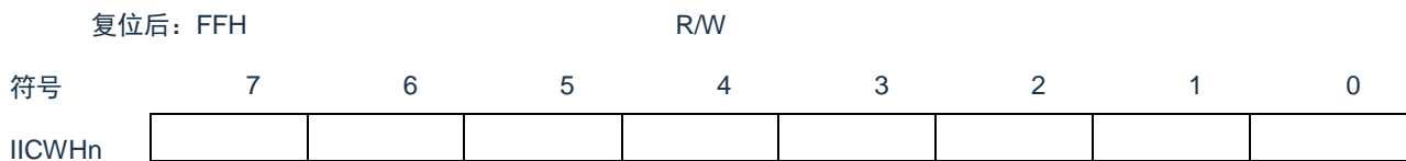
图 17-11: IICA 高电平宽度设定寄存器 n (IICWHn) 的格式
