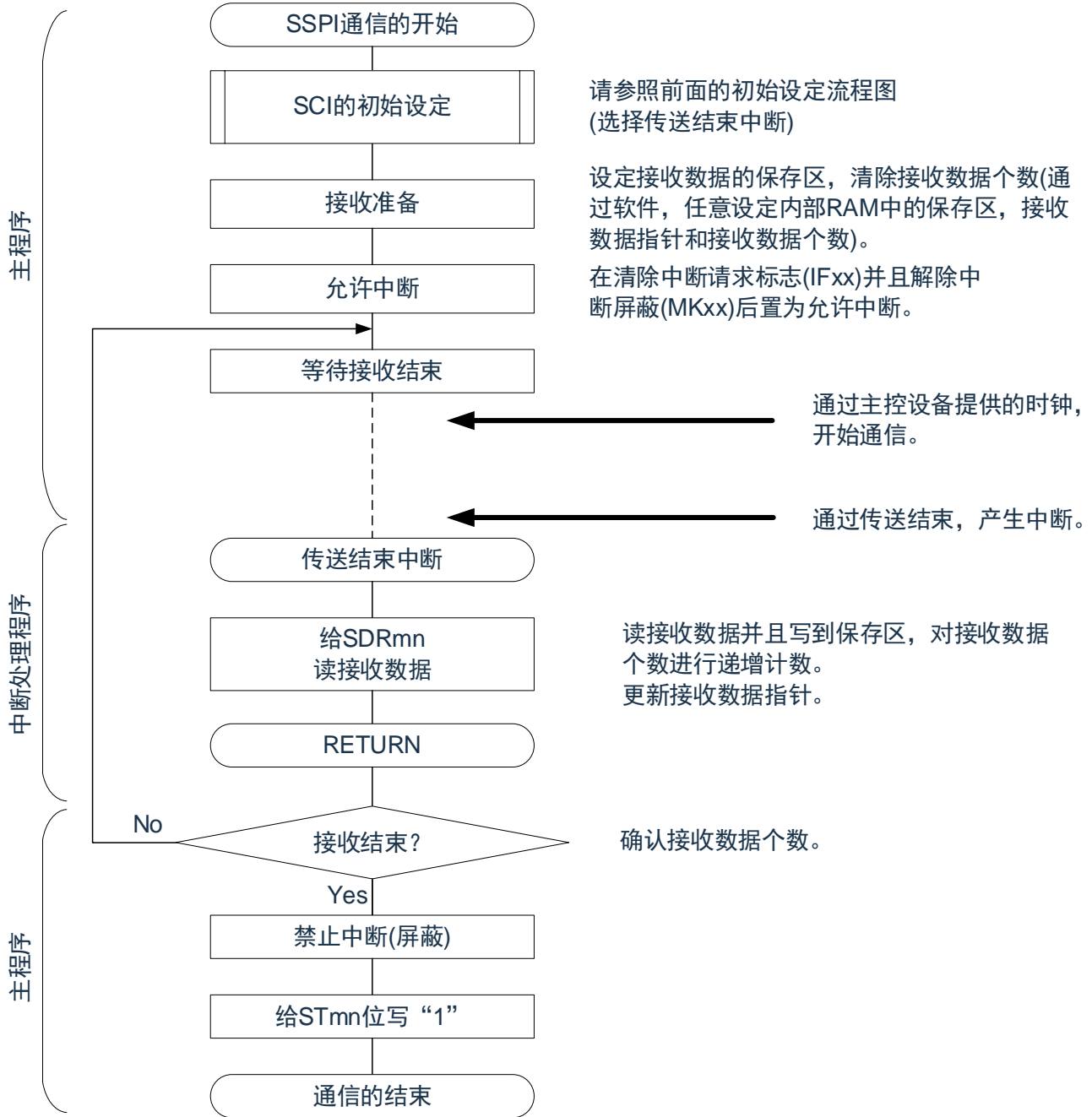
图 15-60: 从属接收 (单次接收模式) 的流程图
