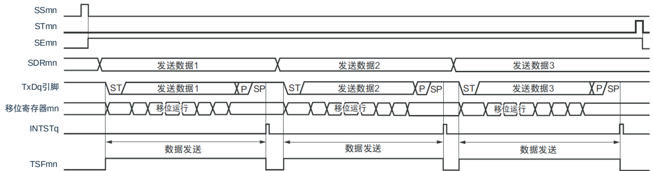
图 15-100: UART 发送（单次发送模式）的时序图
