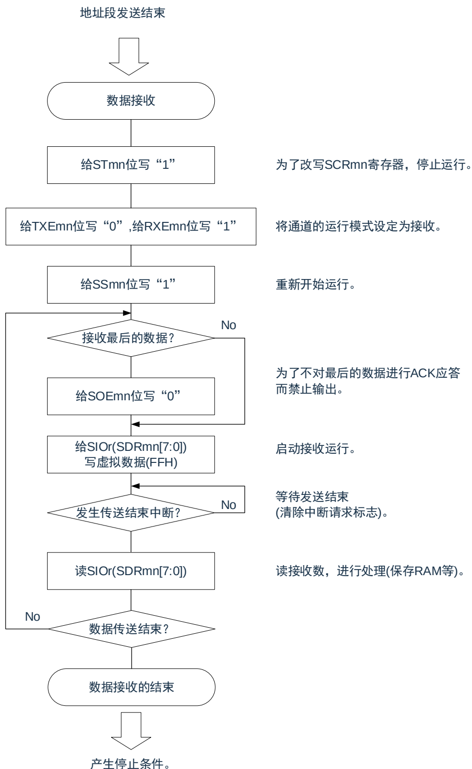
图 15-131：数据接收的流程图
