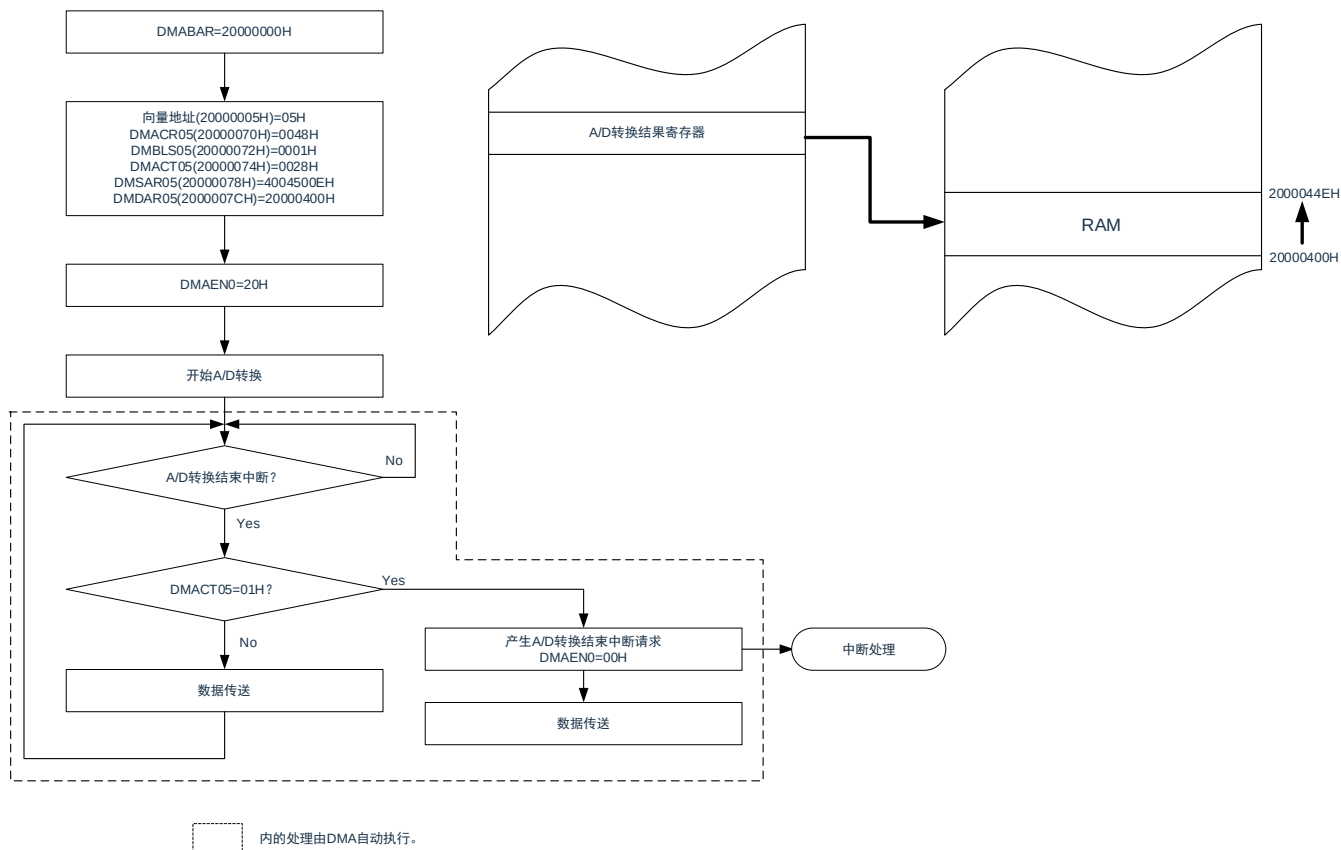
图 20-17：正常模式的使用例子 1：连续取 A/D 转换结果
