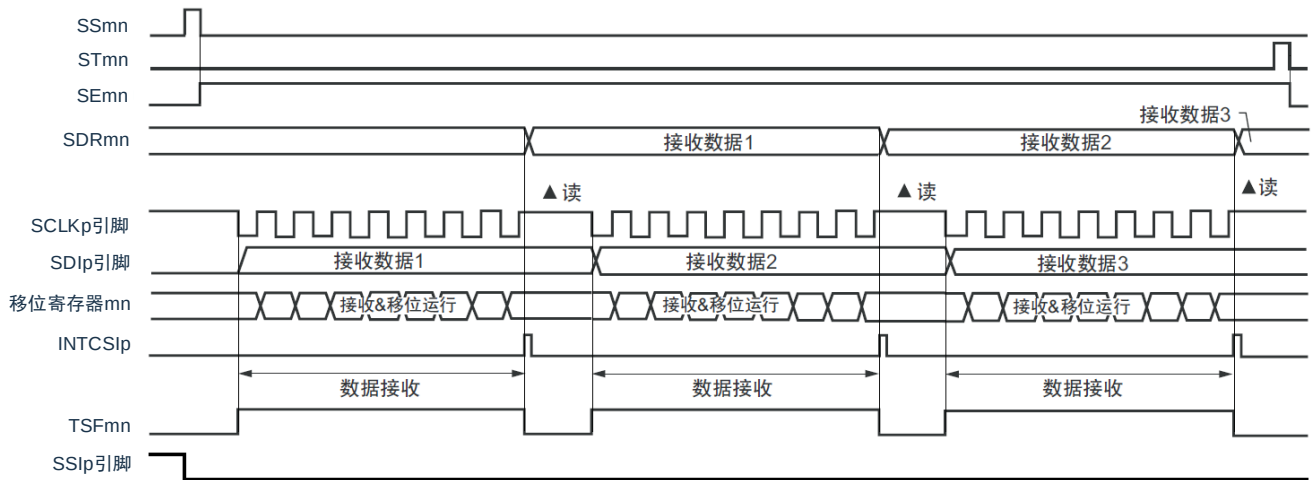
图 15-85：从属接收（单次接收模式）的时序图（类型 1：DAPmn=0、CKPmn=0）
