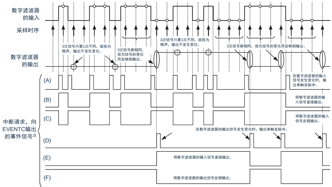
图 13-13: 数字滤波器、中断请求和向 EVENTC 输出事件信号的运行
