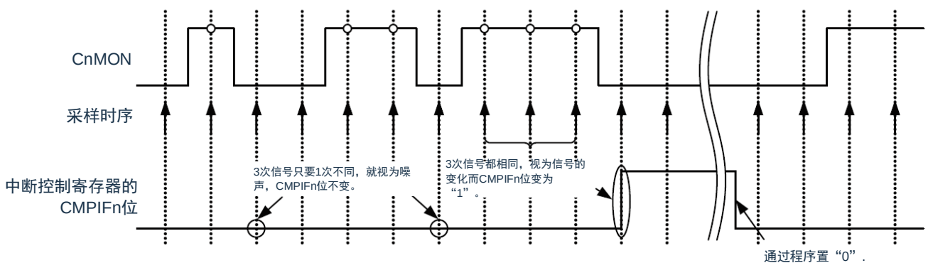
图 13-12: 比较器 n (n=0、1) 的数字滤波器和中断运行例子
