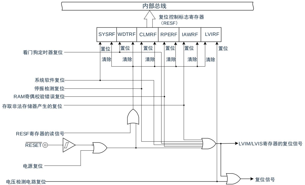
图 25-1: 复位功能的框图
