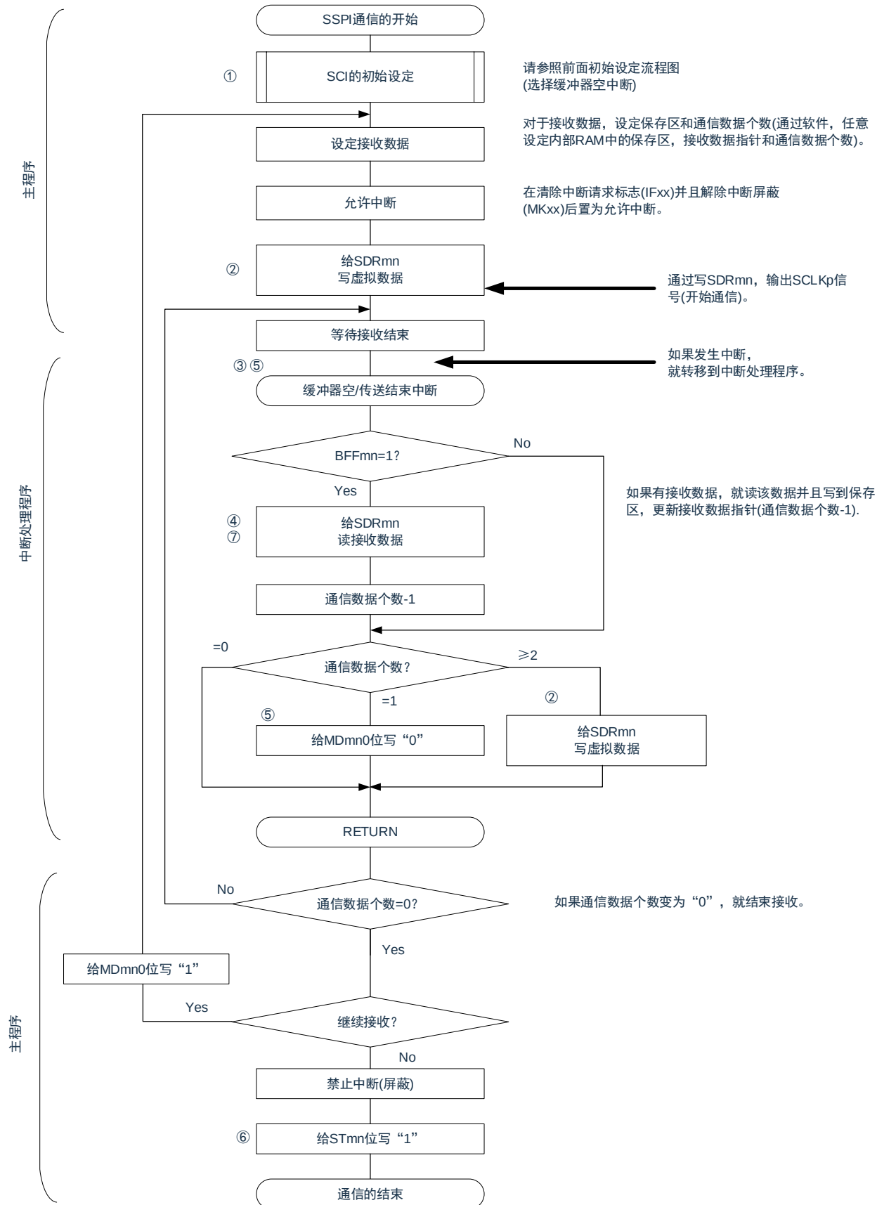
图 15-38: 主控接收（连续接收模式）的流程图
