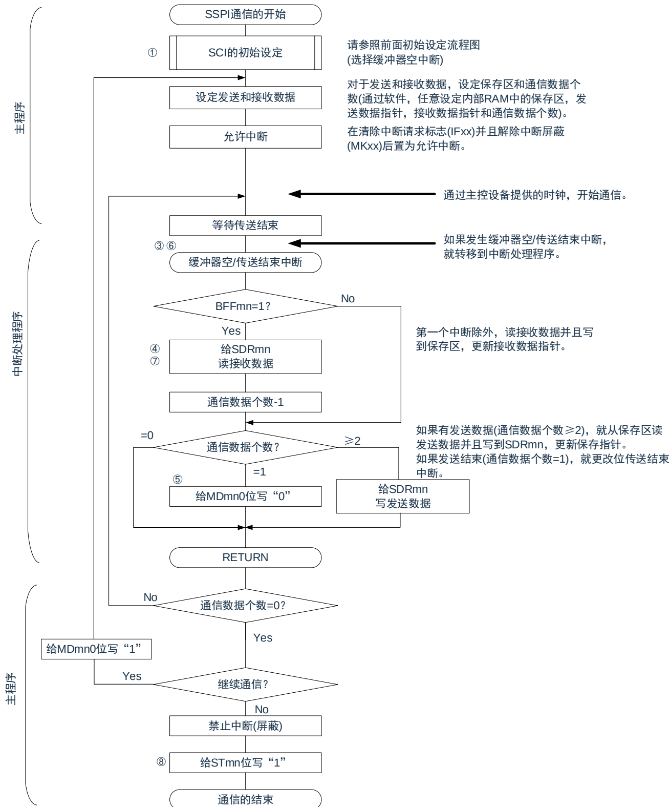
图 15-94: 从属发送和接收（连续发送和接收模式）的流程图
