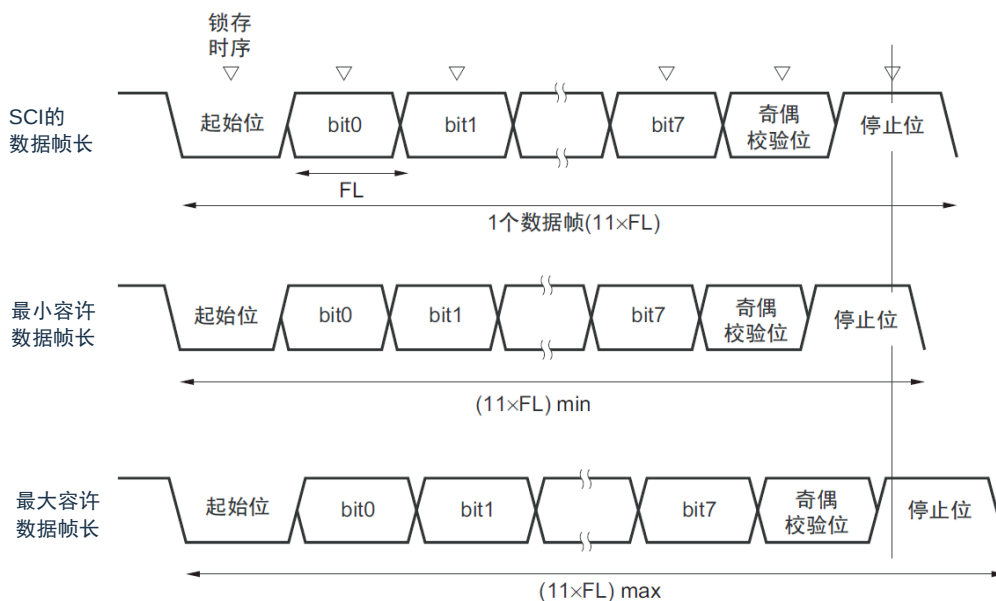
图 15-114: 接收时的波特率容许范围 (1 个数据帧的帧长=11 位的情况)
