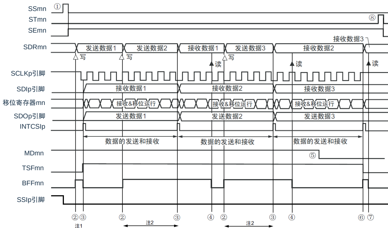
图 15-93：从属发送和接收（连续发送和接收模式）的时序图（类型 1：DAPmn=0、CKPmn=0）
