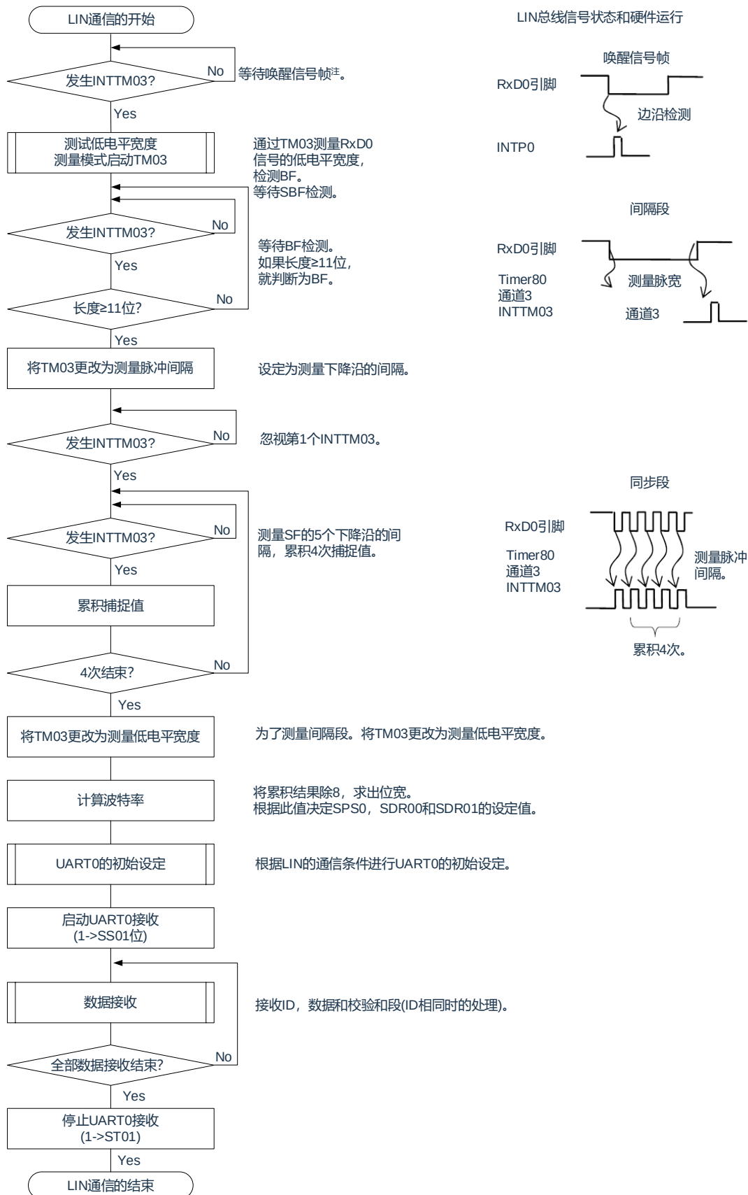
图 15-120: LIN 接收的流程图
