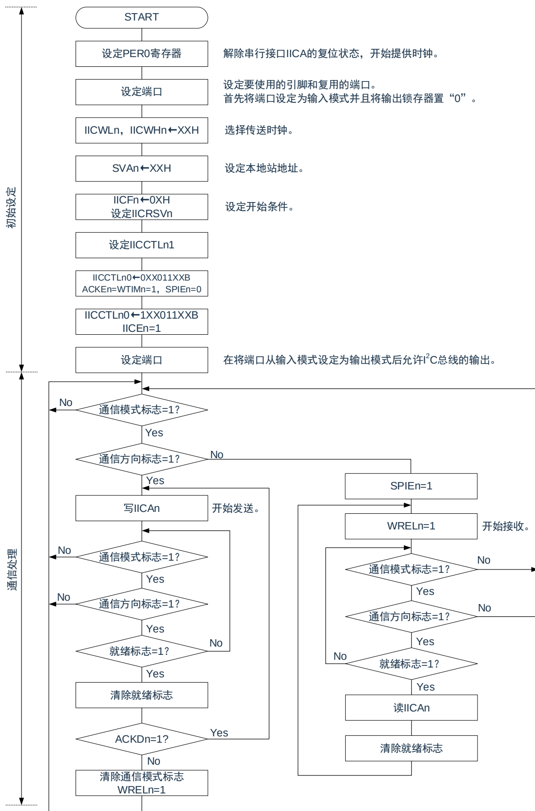
图 17-29：从属运行步骤(1)
