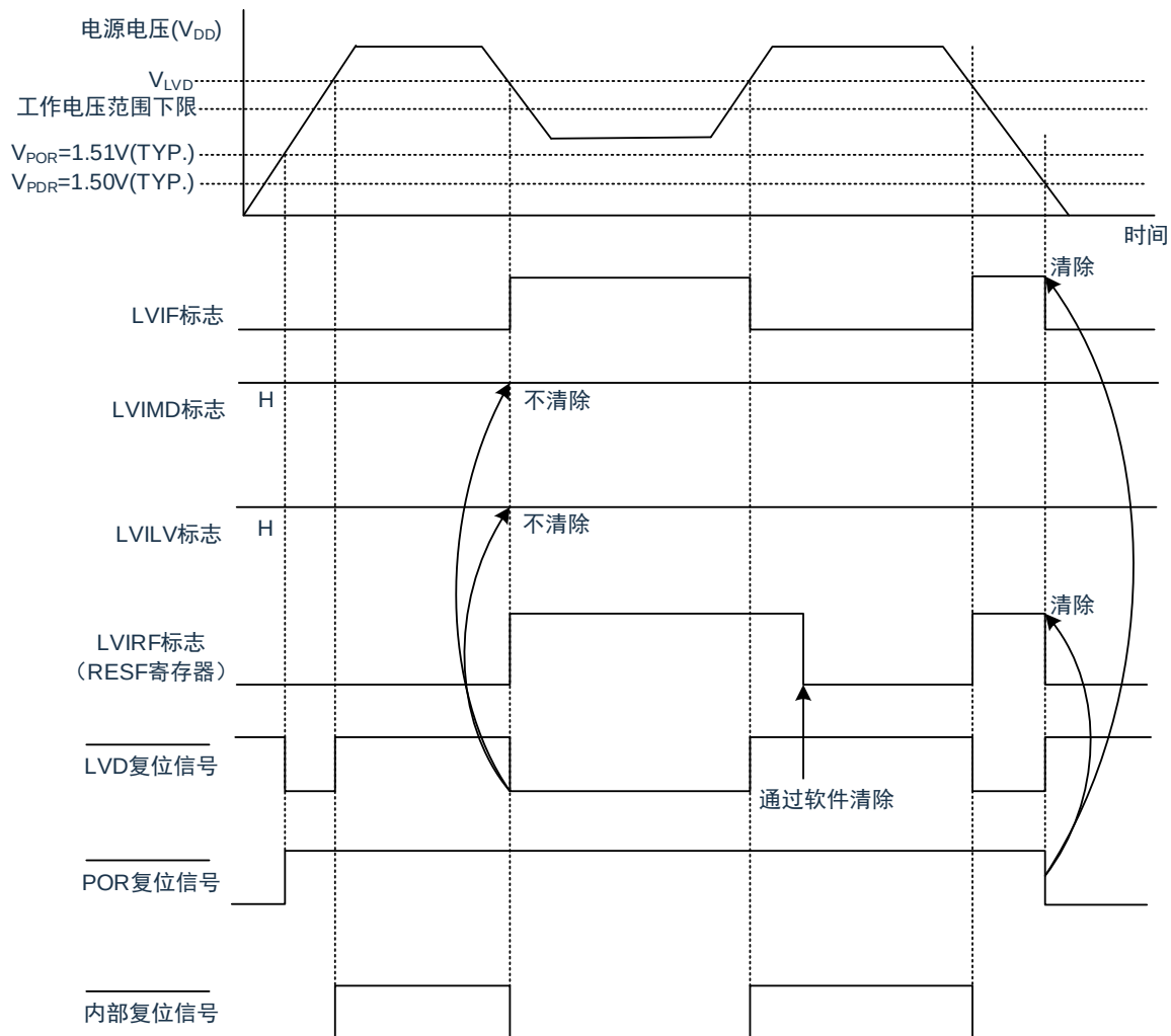
图 27-4：内部复位信号的产生时序（选项字节的 LVIMDS1、LVIMDS0=1、1）
