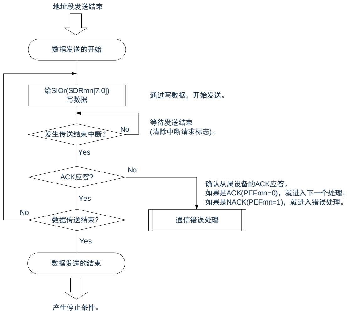
图 15-128: 数据发送的流程图
