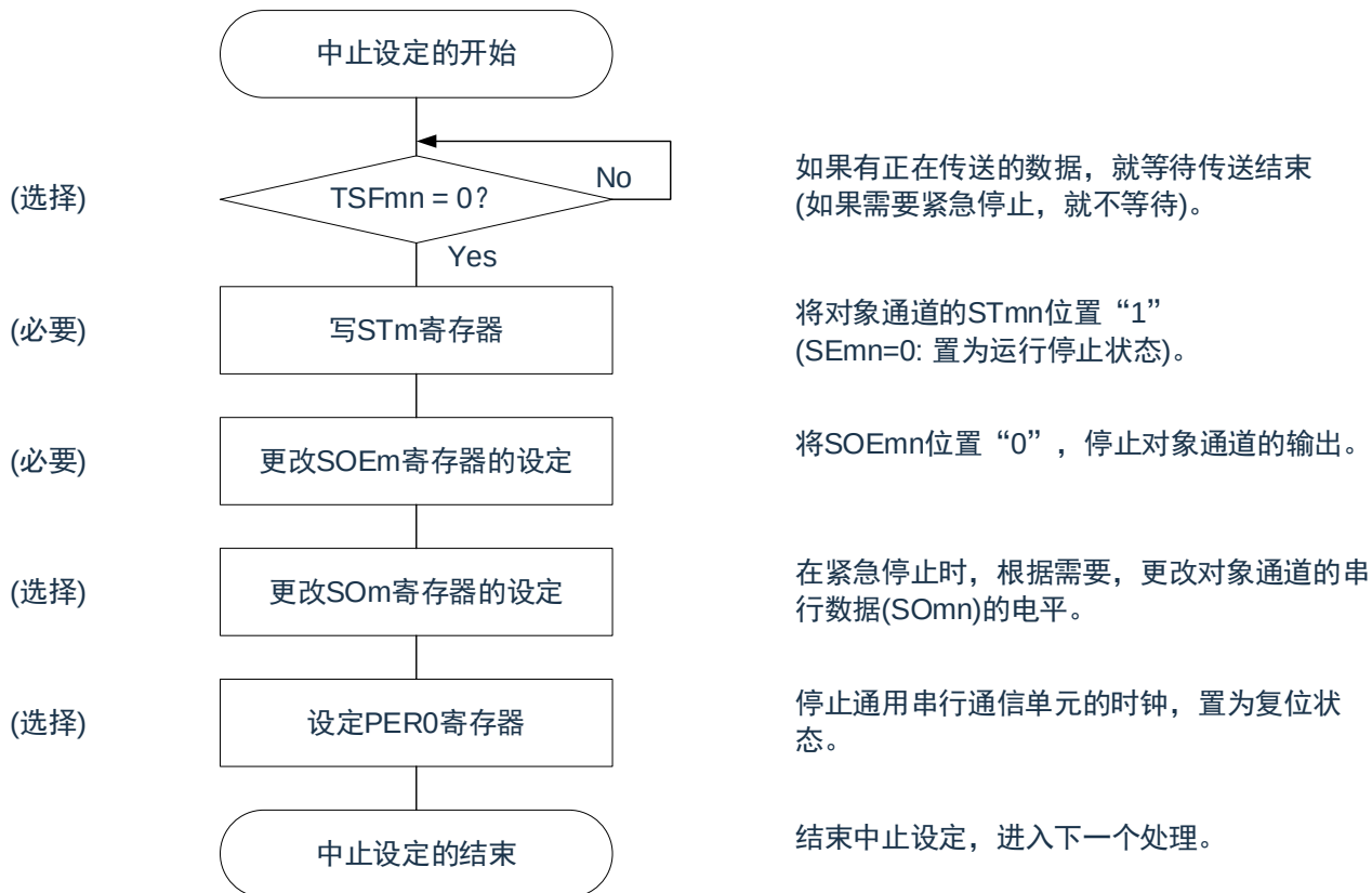
图 15-89：从属发送和接收的中止步骤
