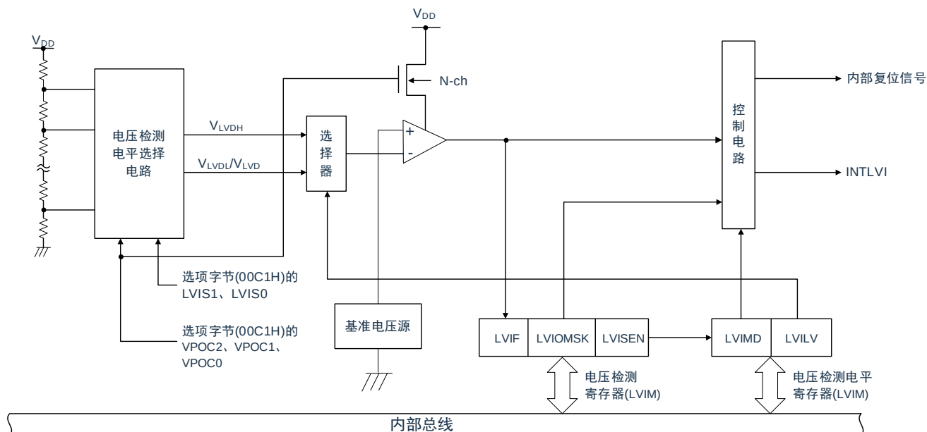
图 27-1：电压检测电路的框图
