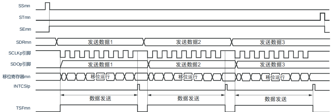
图 15-27：主控发送（单次发送模式）的时序图（类型 1：DAPmn=0、CKPmn=0）
