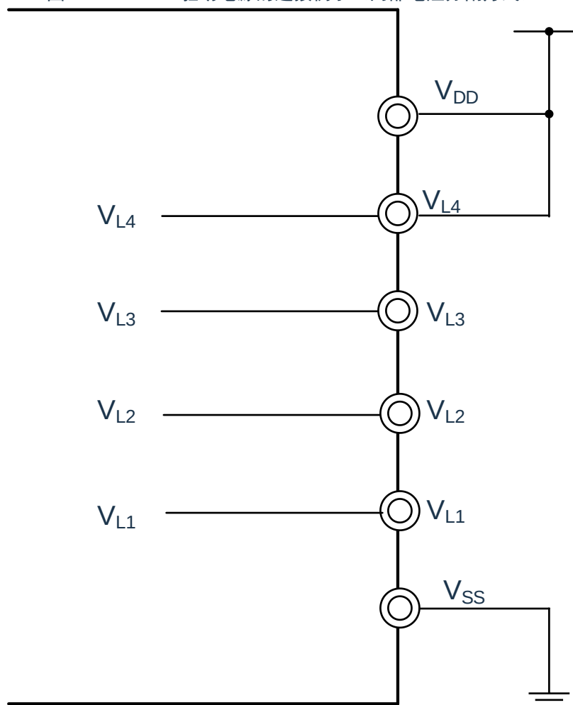
图 19-11: LCD 驱动电源的连接例子（内部电阻分割方式）
