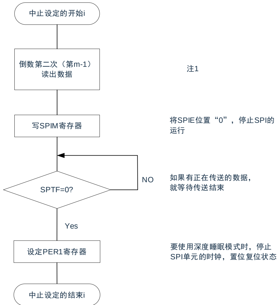
图 16-12：主控接收的中止步骤
