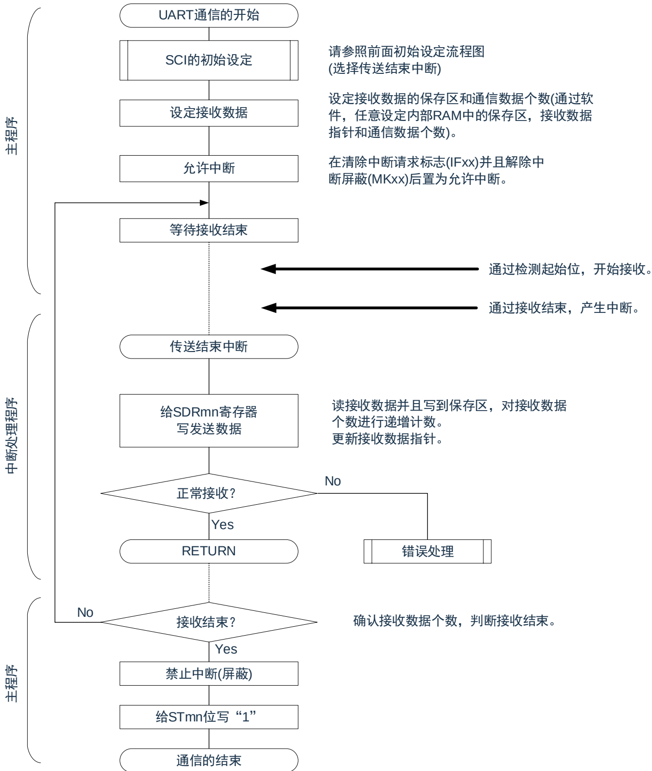
图 15-109: UART 接收的流程图
