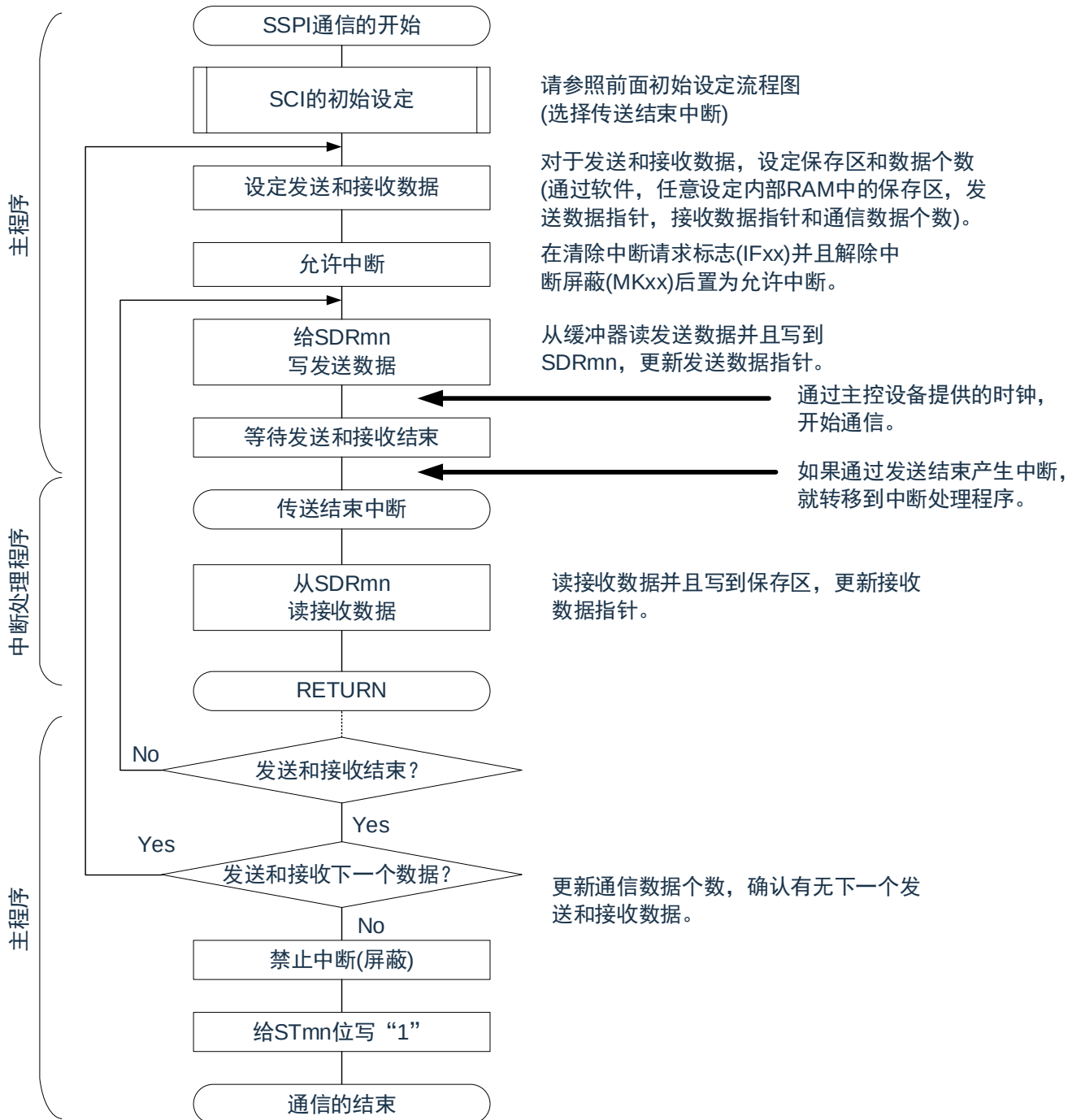
图 15-92: 从属发送和接收（单次发送和接收模式）的流程图
