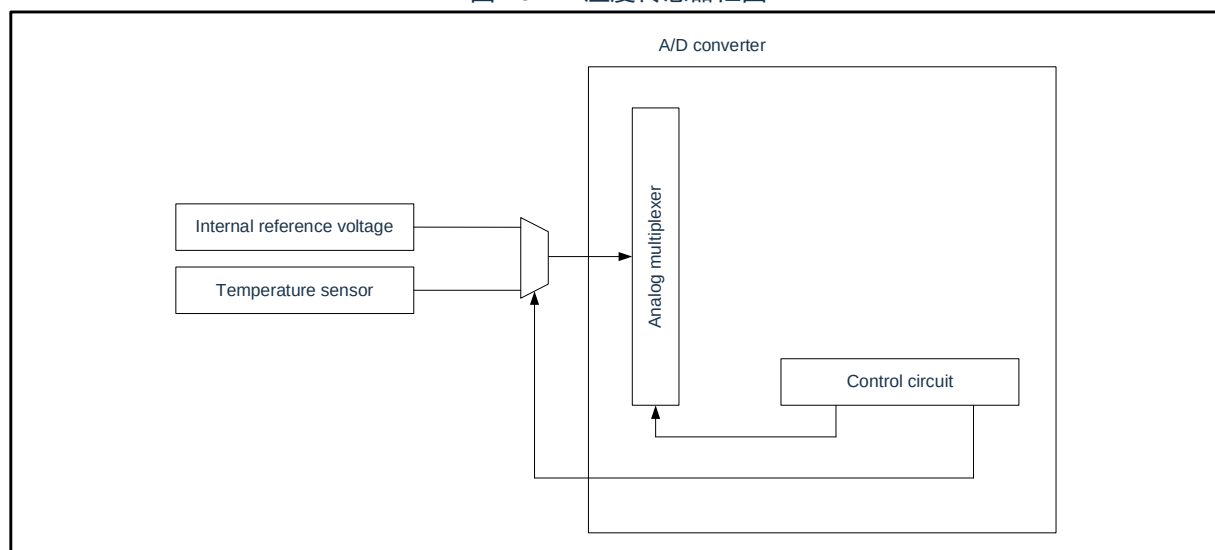
图 29-1：温度传感器框图
