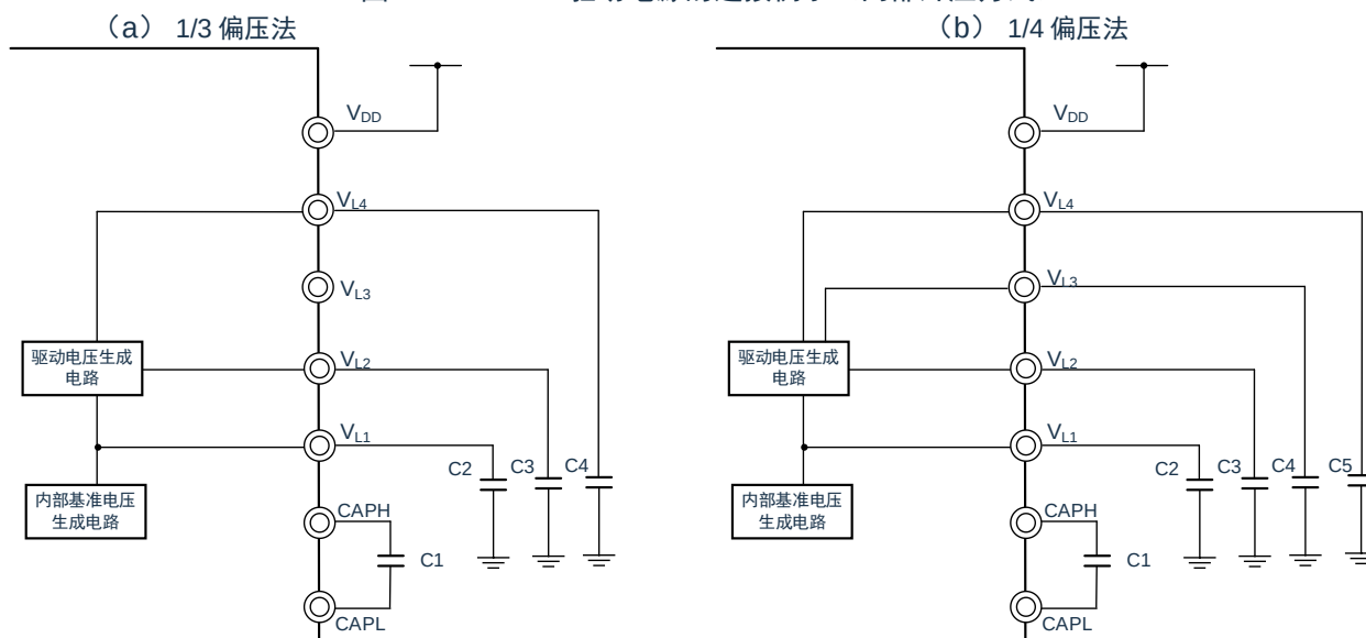
图 19-13: LCD 驱动电源的连接例子（内部升压方式）
