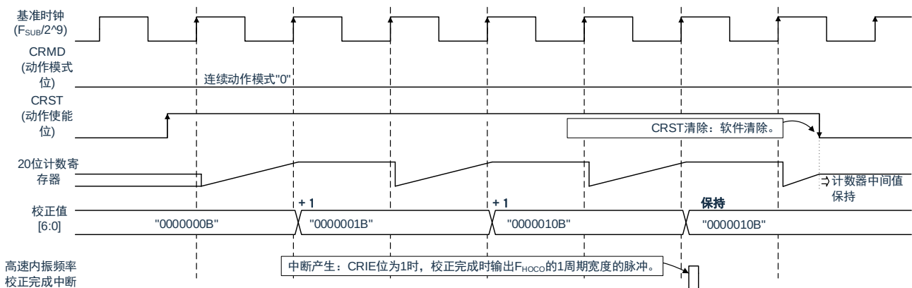
图 4-21：连续动作模式时序图
