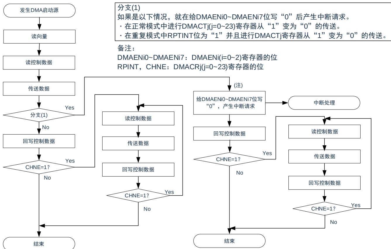
图 20-15: DMA 的内部运行流程图
