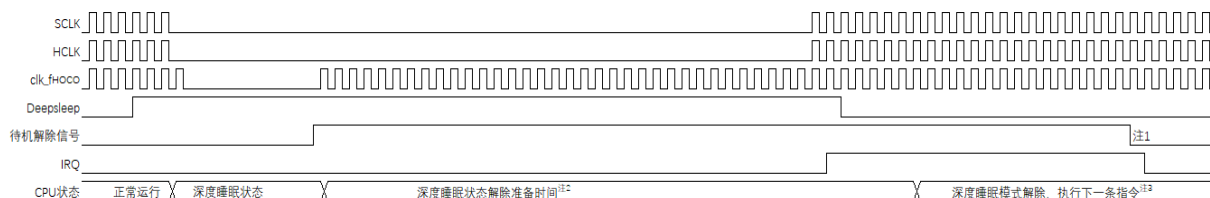
图 24-3：通过中断请求解除深度睡眠模式
