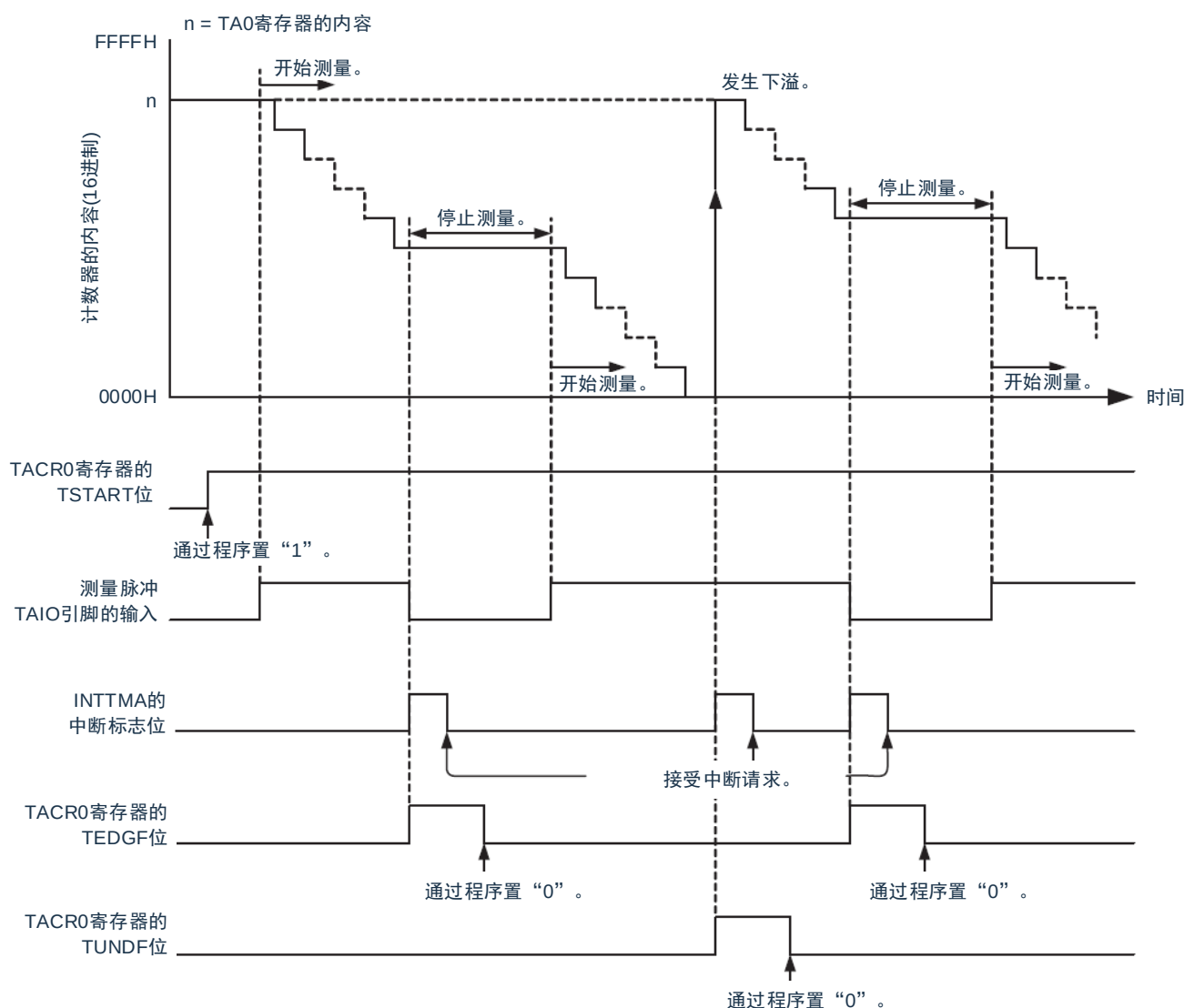
图 6-14：脉冲测量模式的运行例子
