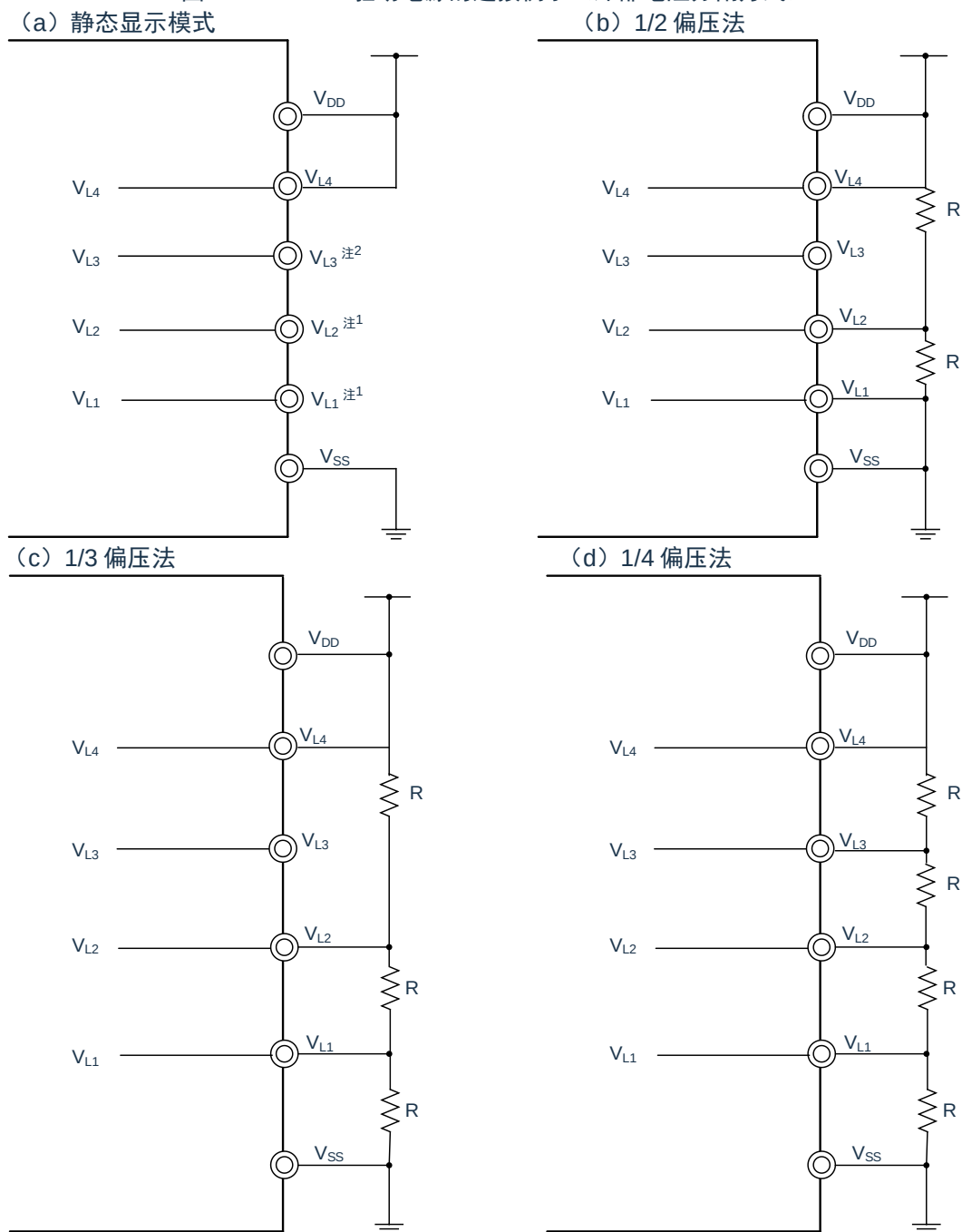
图 19-12: LCD 驱动电源的连接例子（外部电阻分割方式）
