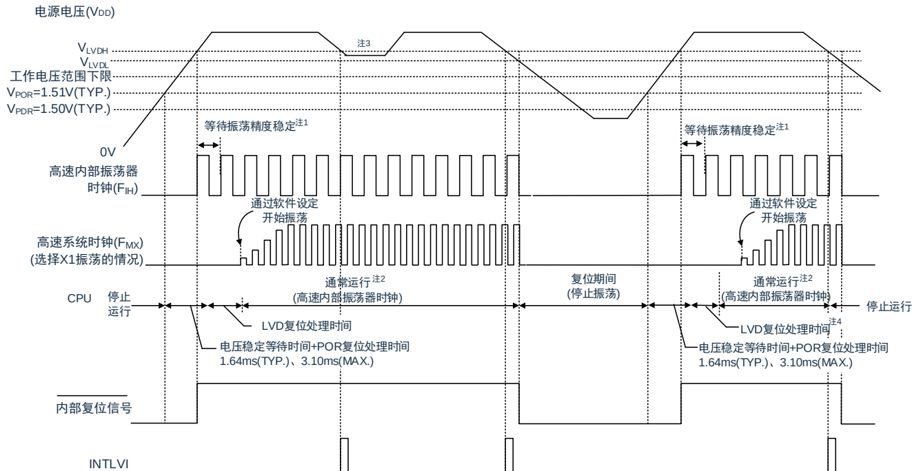
图 26-3：上电复位电路和电压检测电路的内部复位信号的产生时序(2/3)
