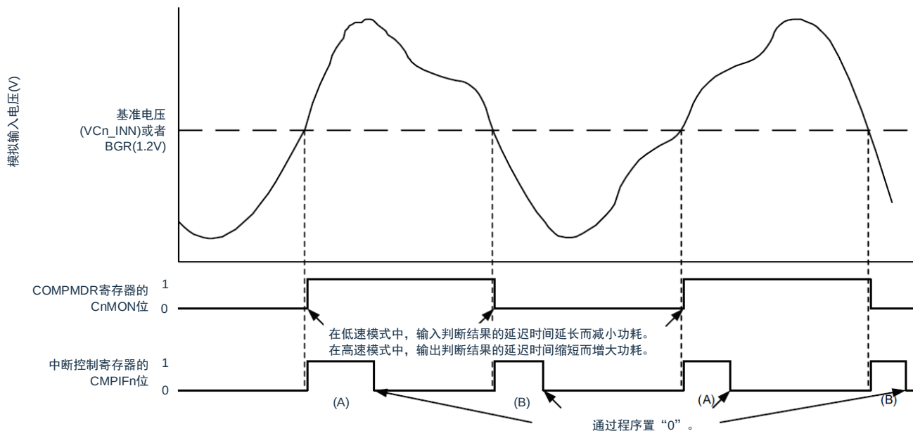
图 13-10：比较器 n ( n=0, 1 ) 的运行例子（基本模式）
