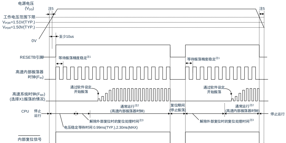
图 26-2：上电复位电路和电压检测电路的内部复位信号的产生时序(1/3)
