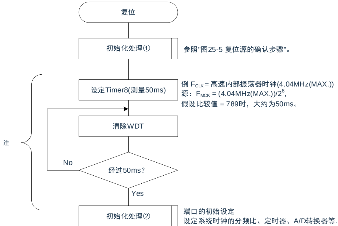
图 27-9: LVD 检测电压附近的电源电压波动不超过 50ms 时的软件处理例子
