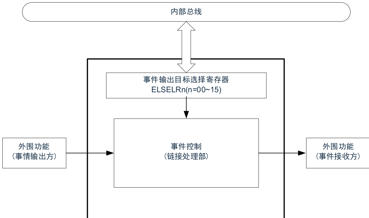
图 21-1: EVENTC 的框图
