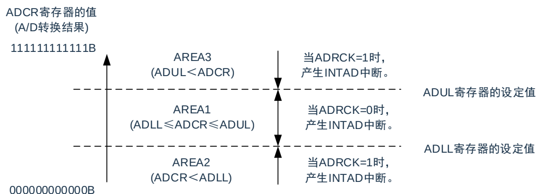
图 11-6: ADRCK 位的中断信号产生范围
