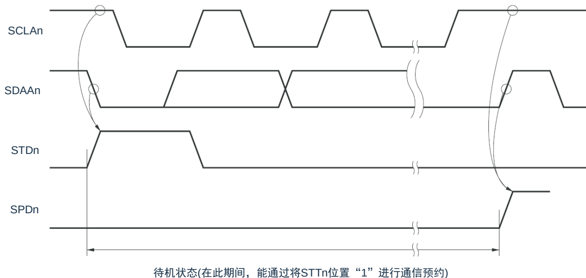
图 17-25：通信预约的接受时序
