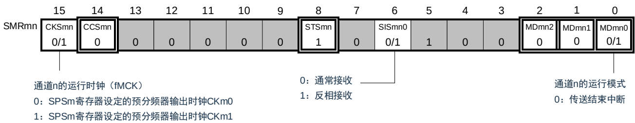
图 15-104: UART (UART0~UART2) 的 UART 接收时的寄存器设定内容例子(1/2)
