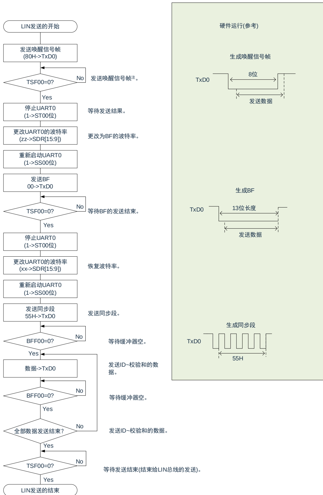
图 15-118: LIN 发送的流程图
