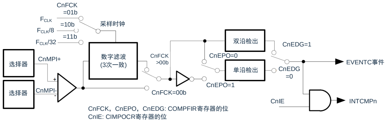
图 13-11: 比较器 n (n=0、1) 的数字滤波器和沿检出结构
