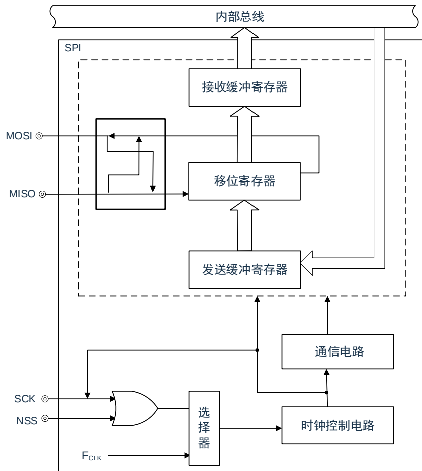
图 16-1：串行接口 SPI 的框图
