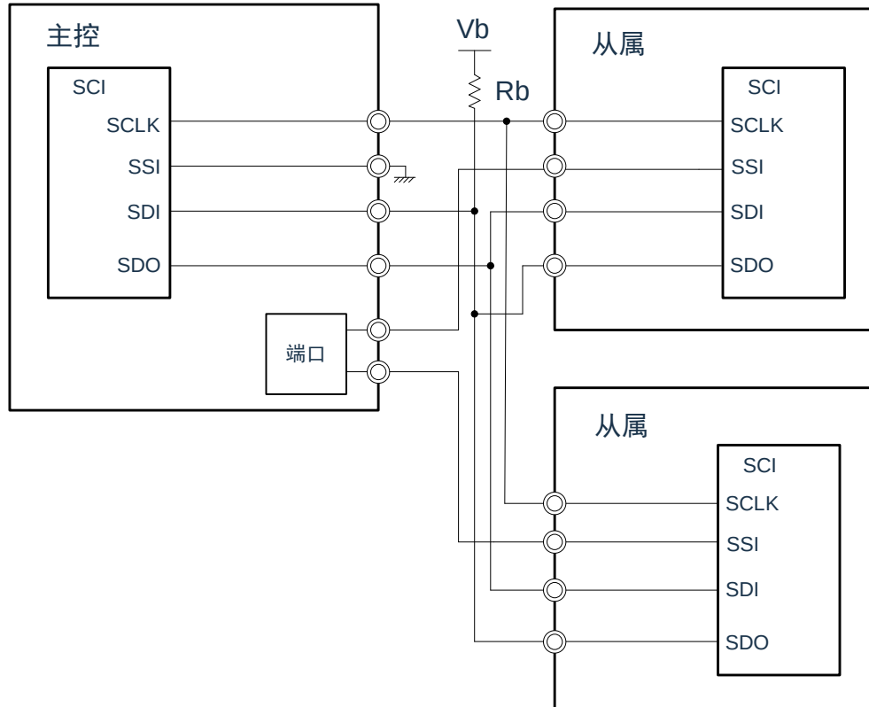
图 15-70：从属选择输入功能的结构例子
