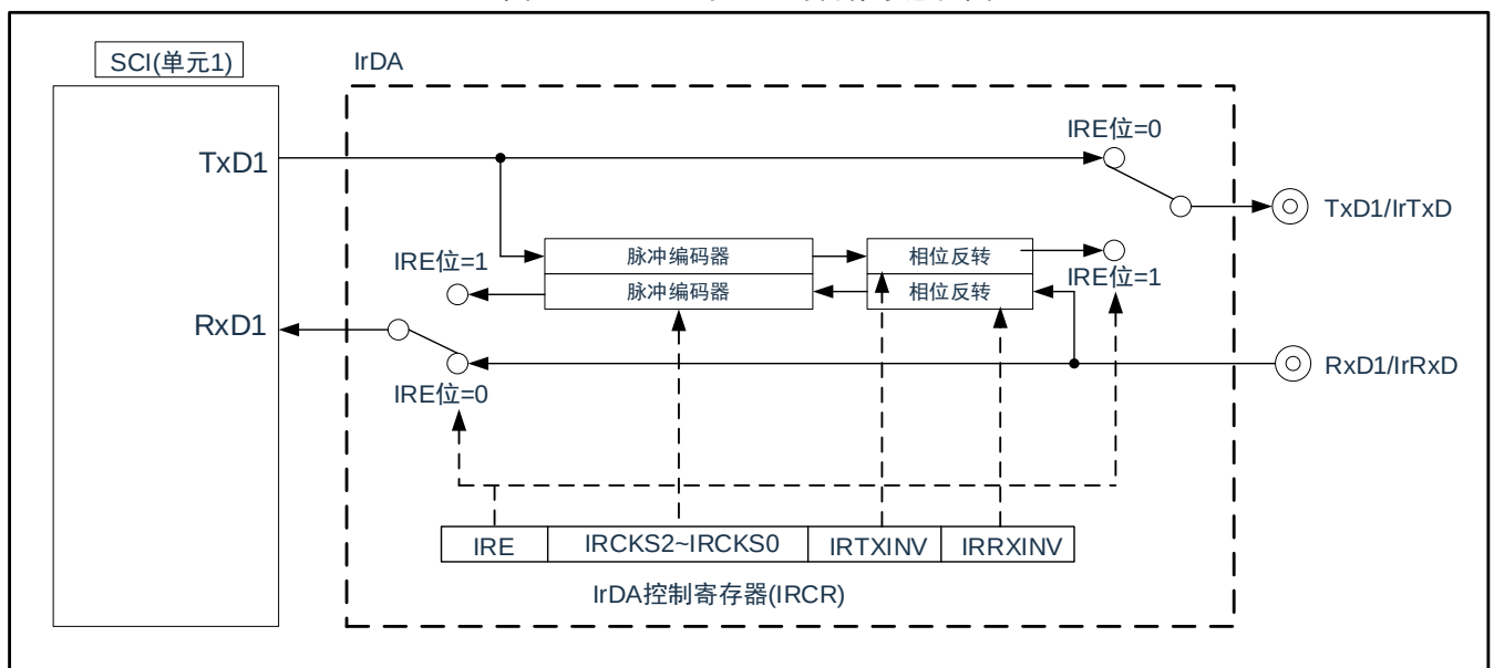
图 18-1：IrDA 与 SCI 的合作示意框图
