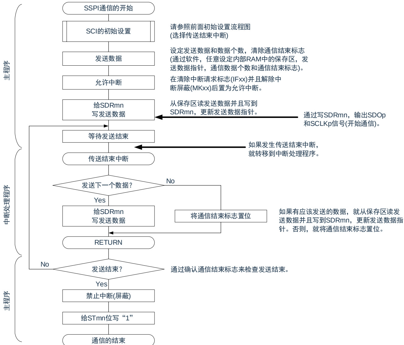
图 15-28: 主控发送（单次发送模式）的流程图
