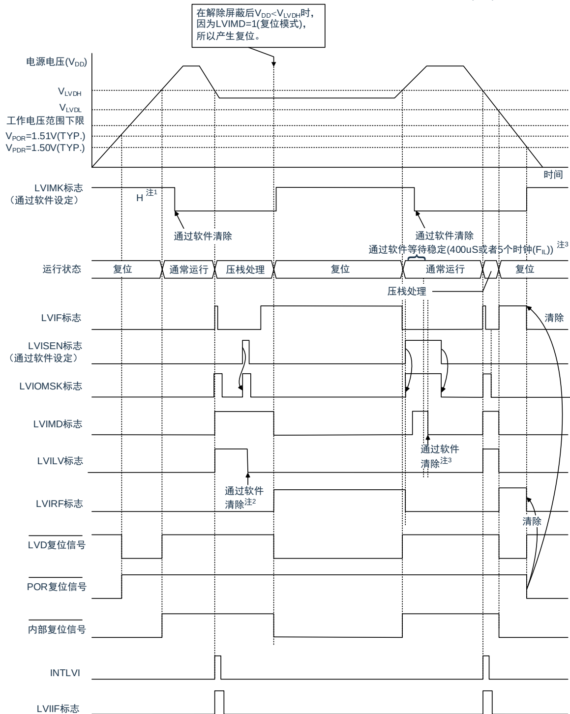
图 27-6：中断&复位信号的产生时序（选项字节的 LVIMDS1、LVIMDS0=1、0）(2/2)
