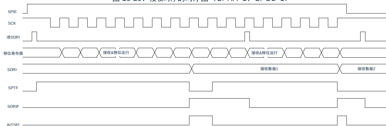
图 16-20: 接收时序的时序图 (CPHA=1、CPOL=1)
