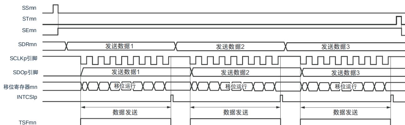
图 15-51：从属发送（单次发送模式）的时序图（类型 1：DAPmn=0、CKPmn=0）
