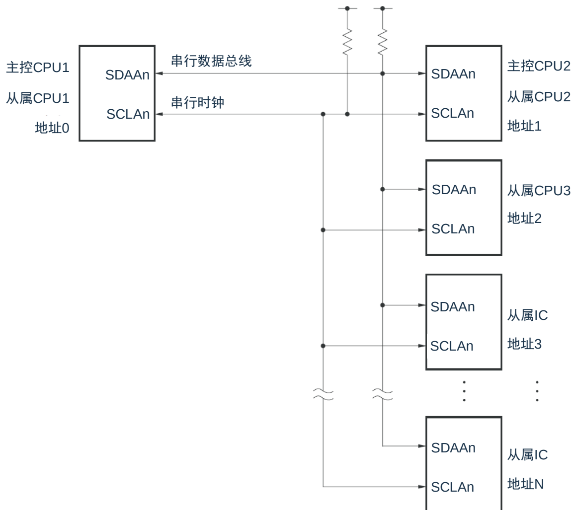
图 17-2: I 2 C 总线的串行总线结构例子
