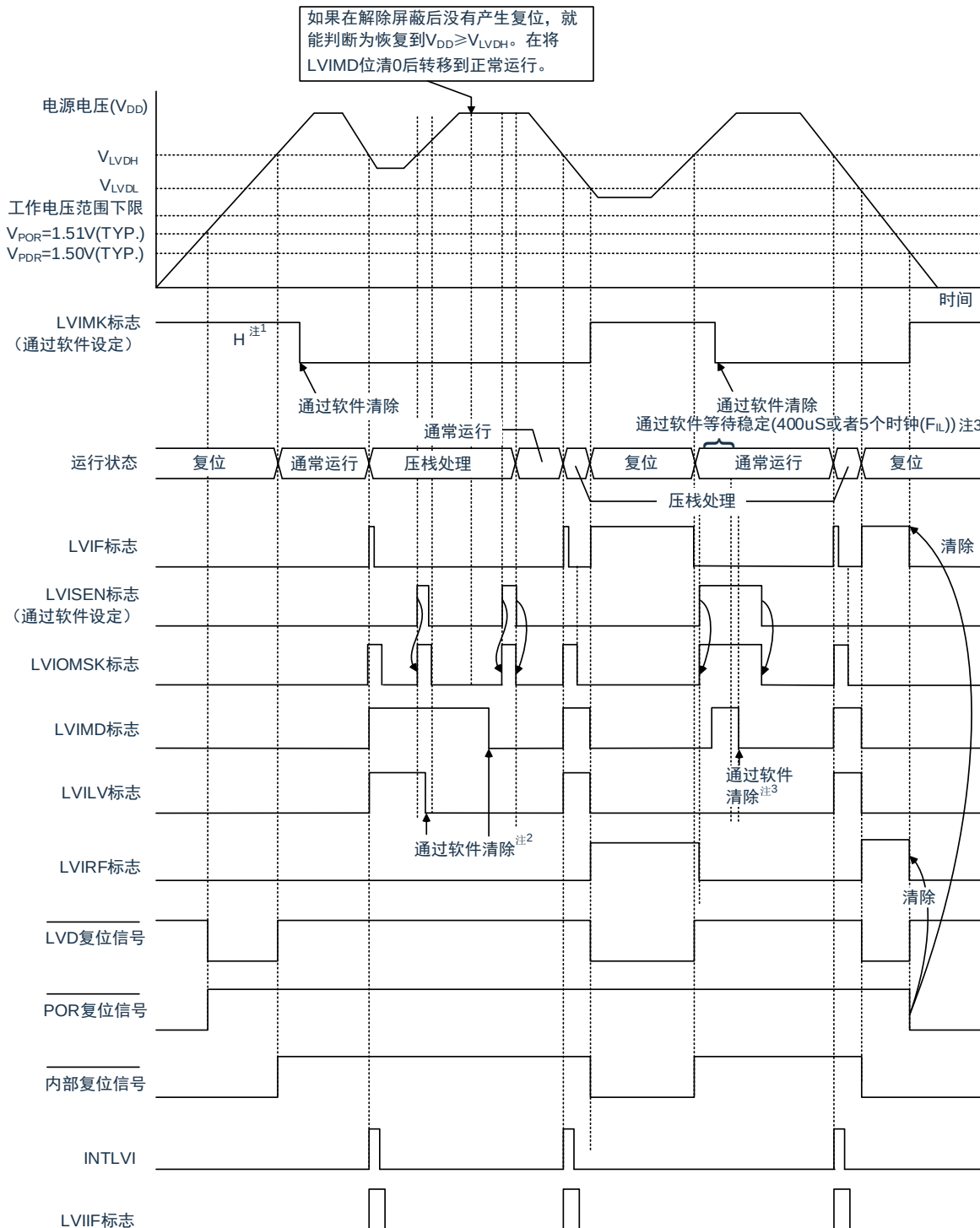
图 27-6：复位&中断信号的产生时序（选项字节的 LVIMDS1、LVIMDS0=1、0）(1/2)
