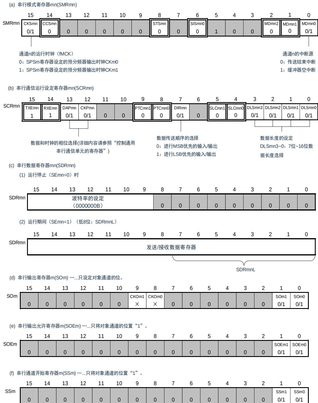
图 15-61: 3 线串行 I/O (SSPI00、SSPI01、SSPI10、SSPI11、SSPI20、SSPI21) 从属发送和接收时的寄存器设定内容例子
