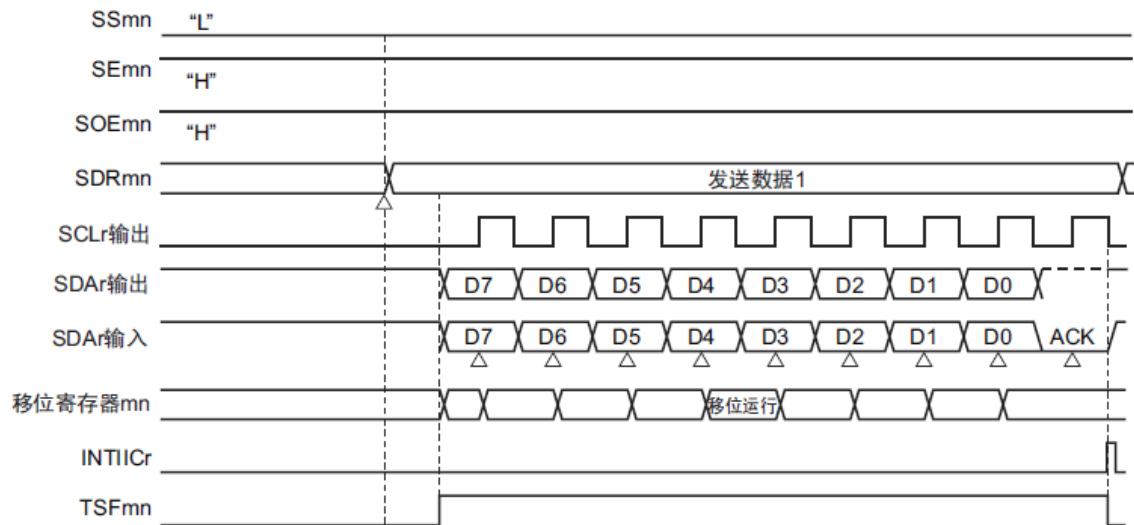
图 15-127: 数据发送的时序图
