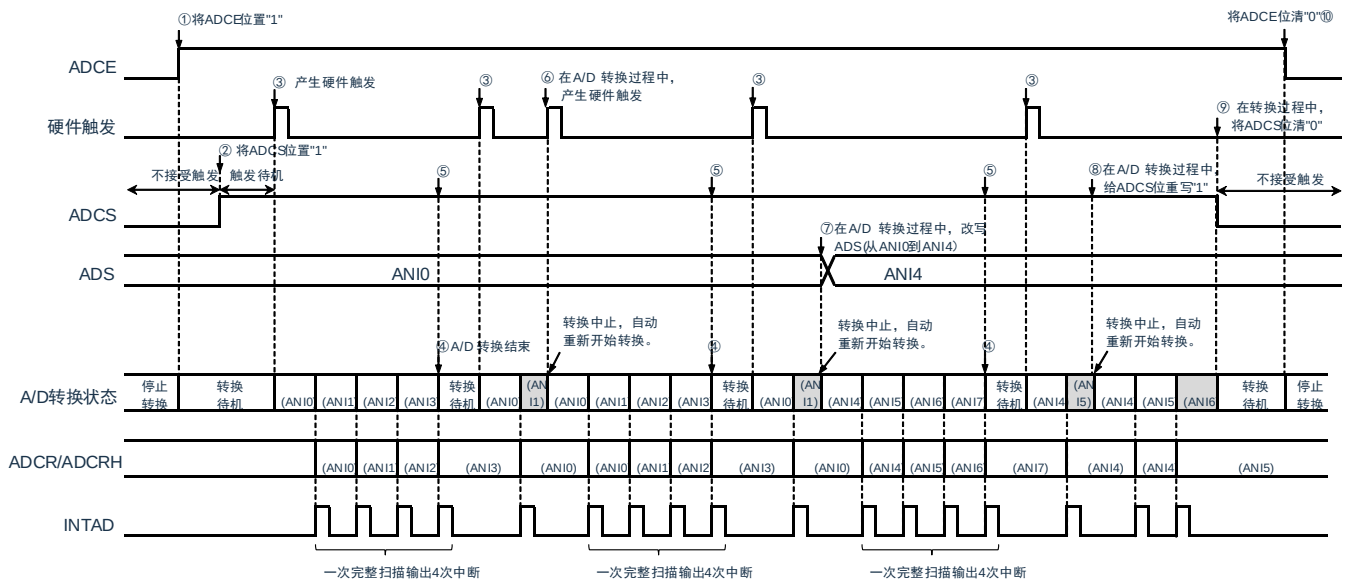
图 11-25: 硬件触发无等待模式（扫描模式、单次转换模式）的运行时序例子
