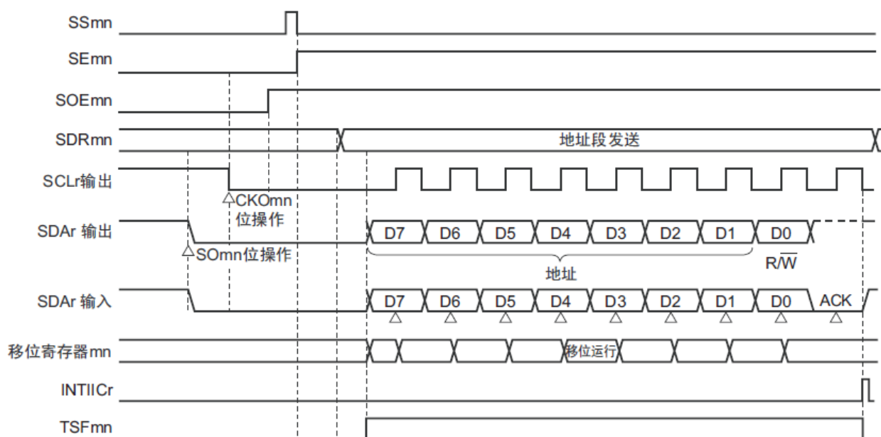
图 15-124: 地址段发送的时序图
