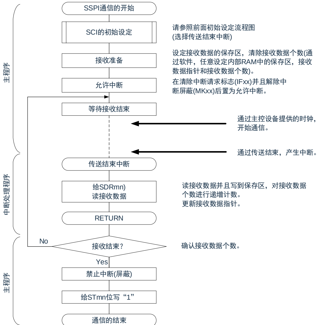
图 15-86: 从属接收（单次接收模式）的流程图
