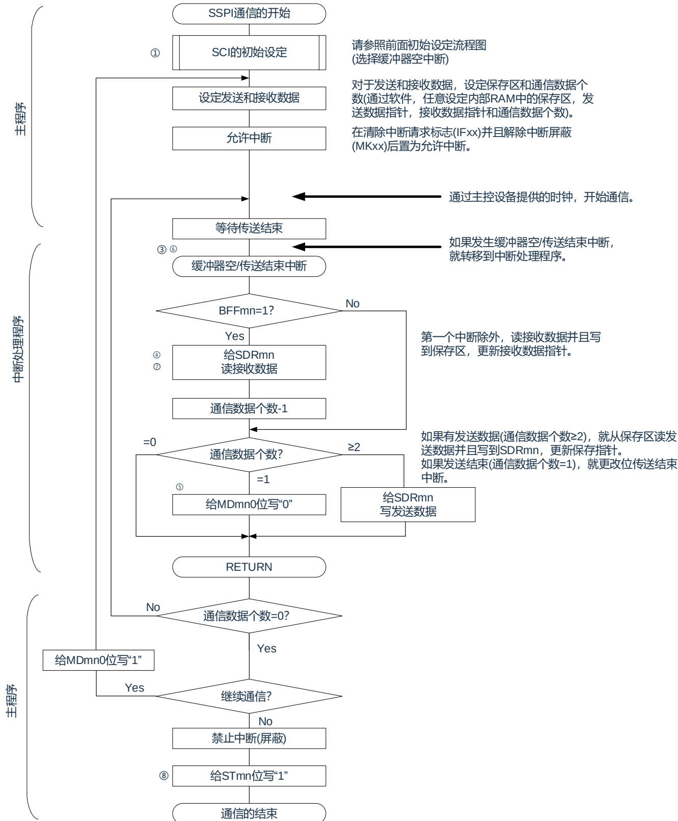
图 15-68: 从属发送和接收（连续发送和接收模式）的流程图
