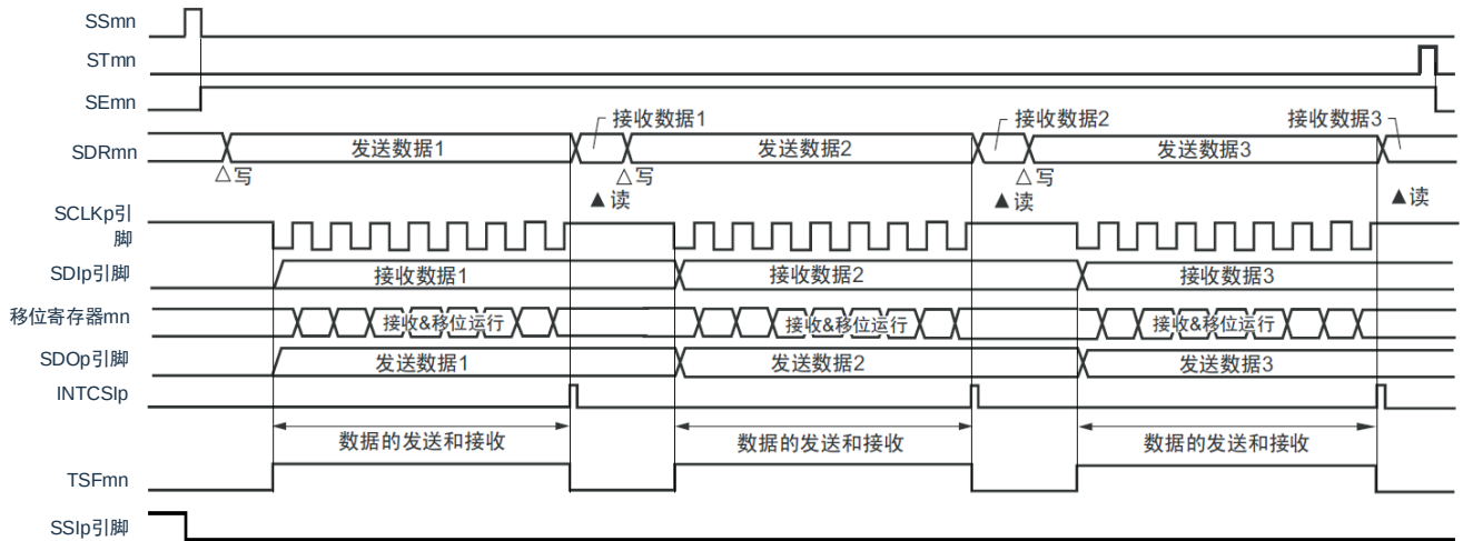
图 15-91：从属发送和接收（单次发送和接收模式）的时序图（类型 1：DAPmn=0、CKPmn=0）
