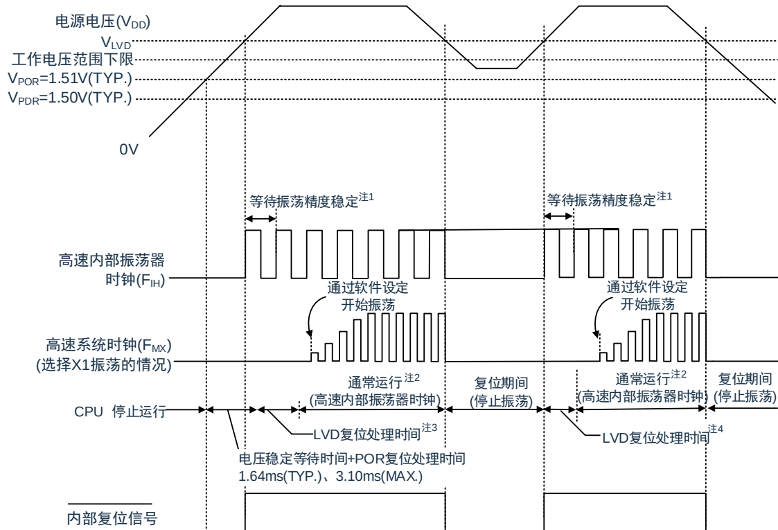
图 26-4：上电复位电路和电压检测电路的内部复位信号的产生时序(3/3)
