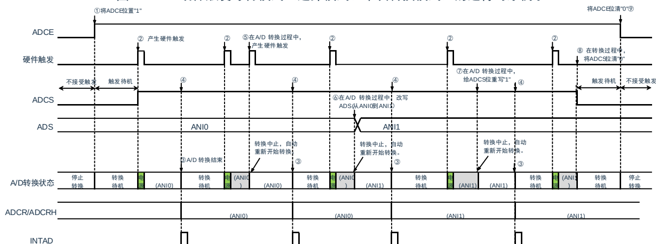
图 11-27：硬件触发等待模式（选择模式、单次转换模式）的运行时序例子
