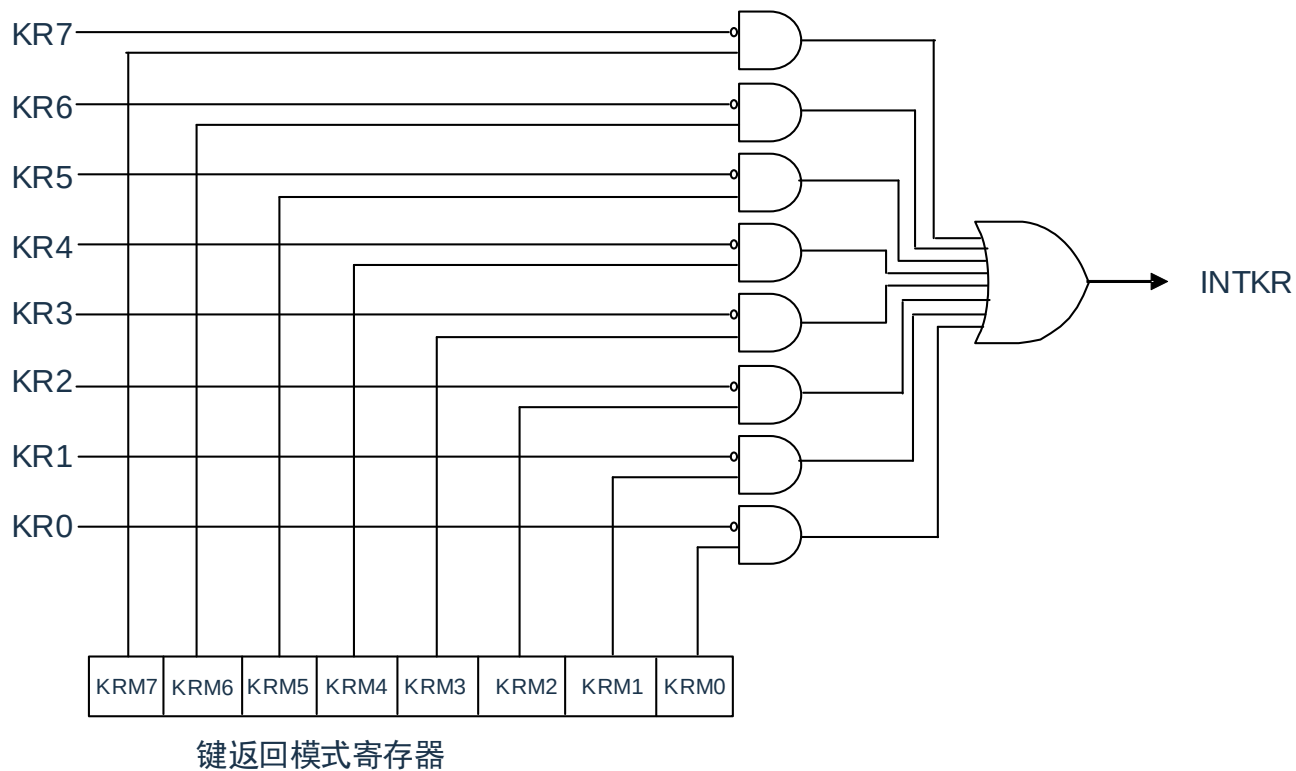
图 23-1: 键中断的框图
