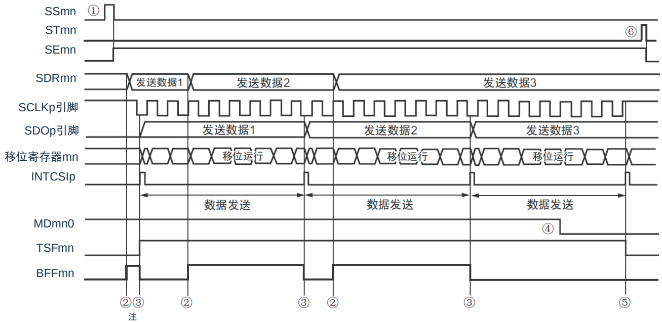
图 15-53：从属发送（连续发送模式）的时序图（类型 1：DAPmn=0、CKPmn=0）
