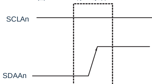
图 17-18: 停止条件
