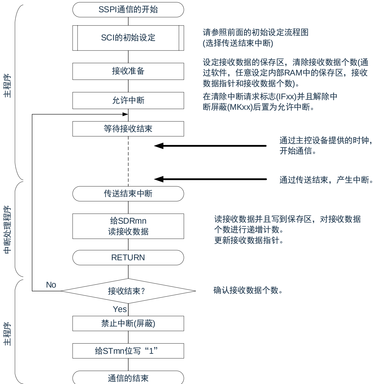
图 15-60: 从属接收（单次接收模式）的流程图
