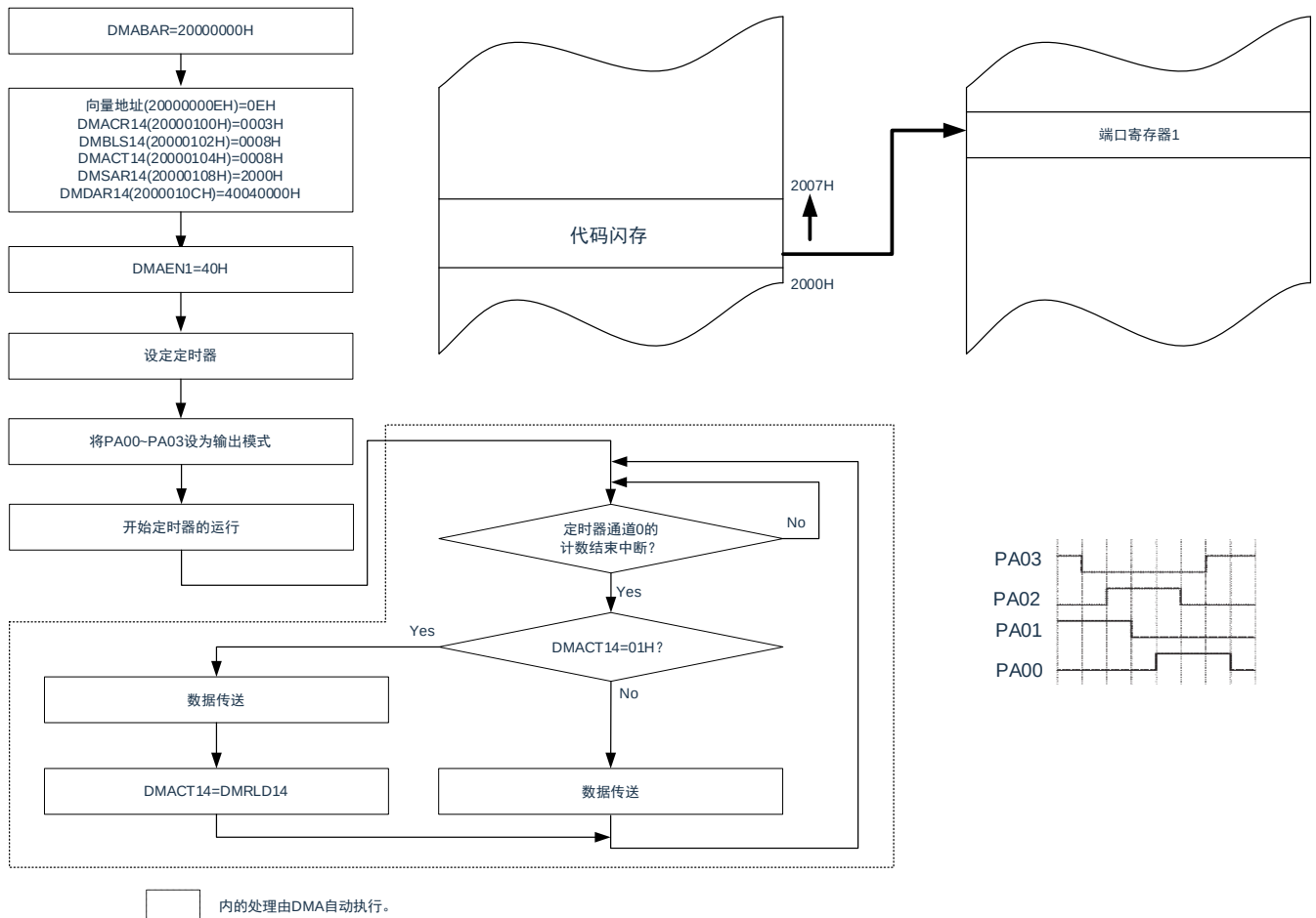
图 20-20：重复模式的使用例子 1：使用端口的步进马达控制脉冲输出
