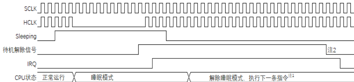
图 24-1：通过中断请求解除睡眠模式
