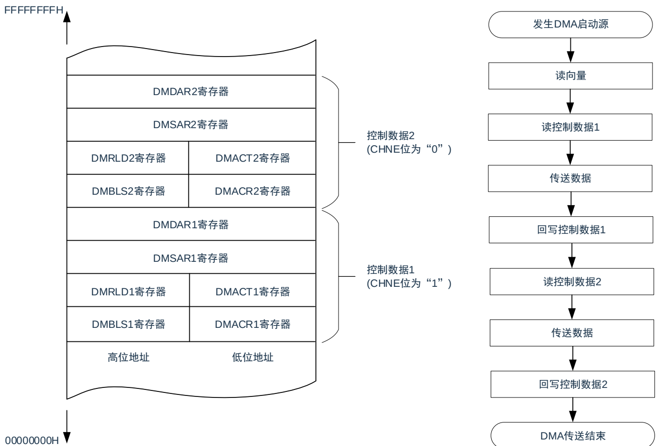
图 20-21：链传送的流程图
