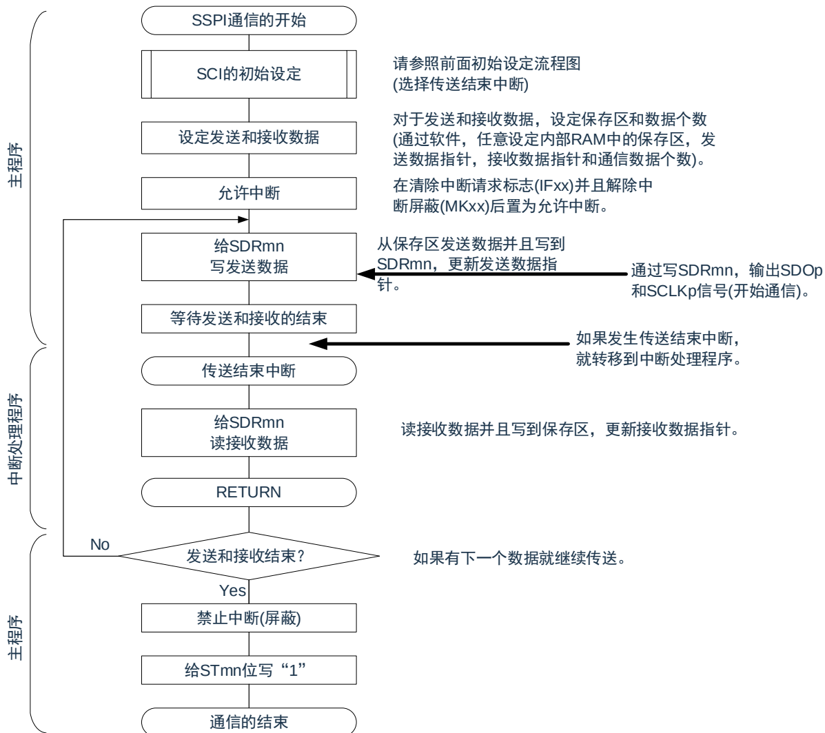
图 15-44: 主控发送和接收（单次发送和接收模式）的流程图
