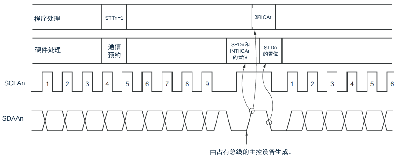
图 17-24：通信预约的时序
