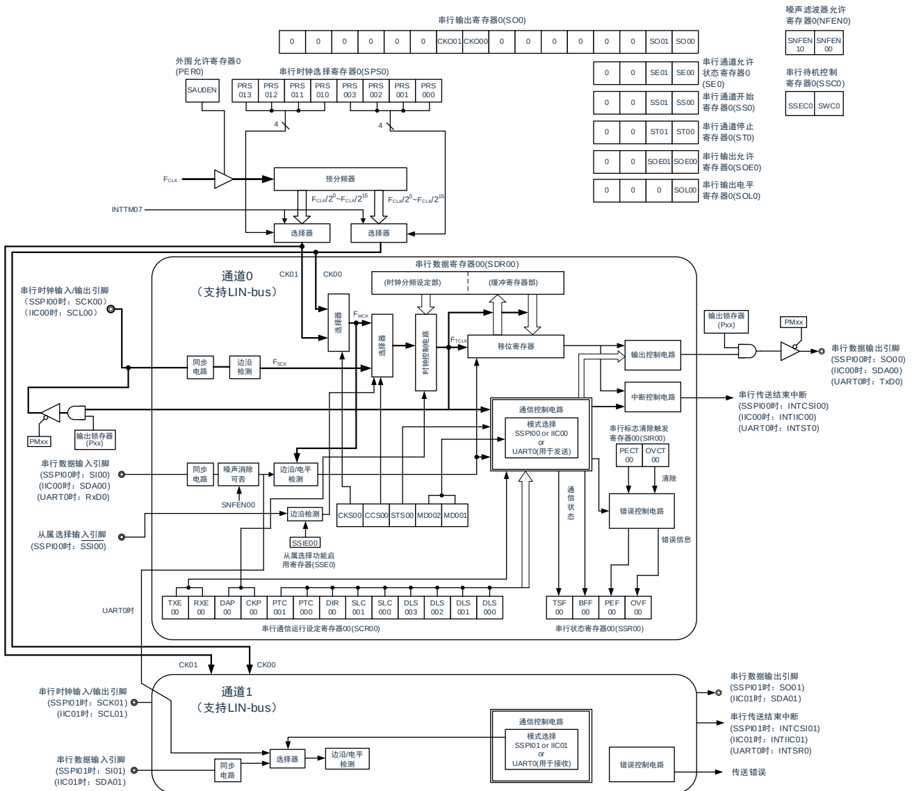
图 15-1：通用串行通信单元 0 的框图
