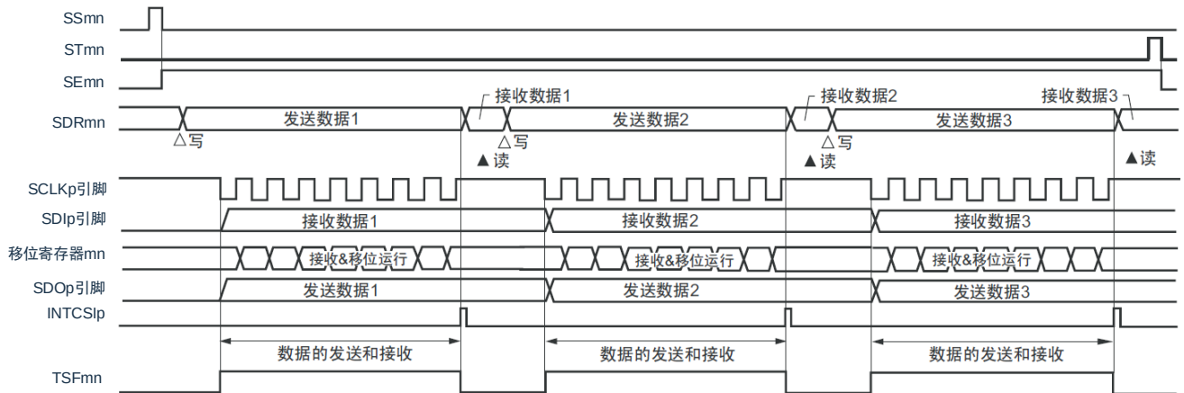
图 15-65：从属发送和接收（单次发送和接收模式）的时序图（类型 1：DAPmn=0、CKPmn=0）
