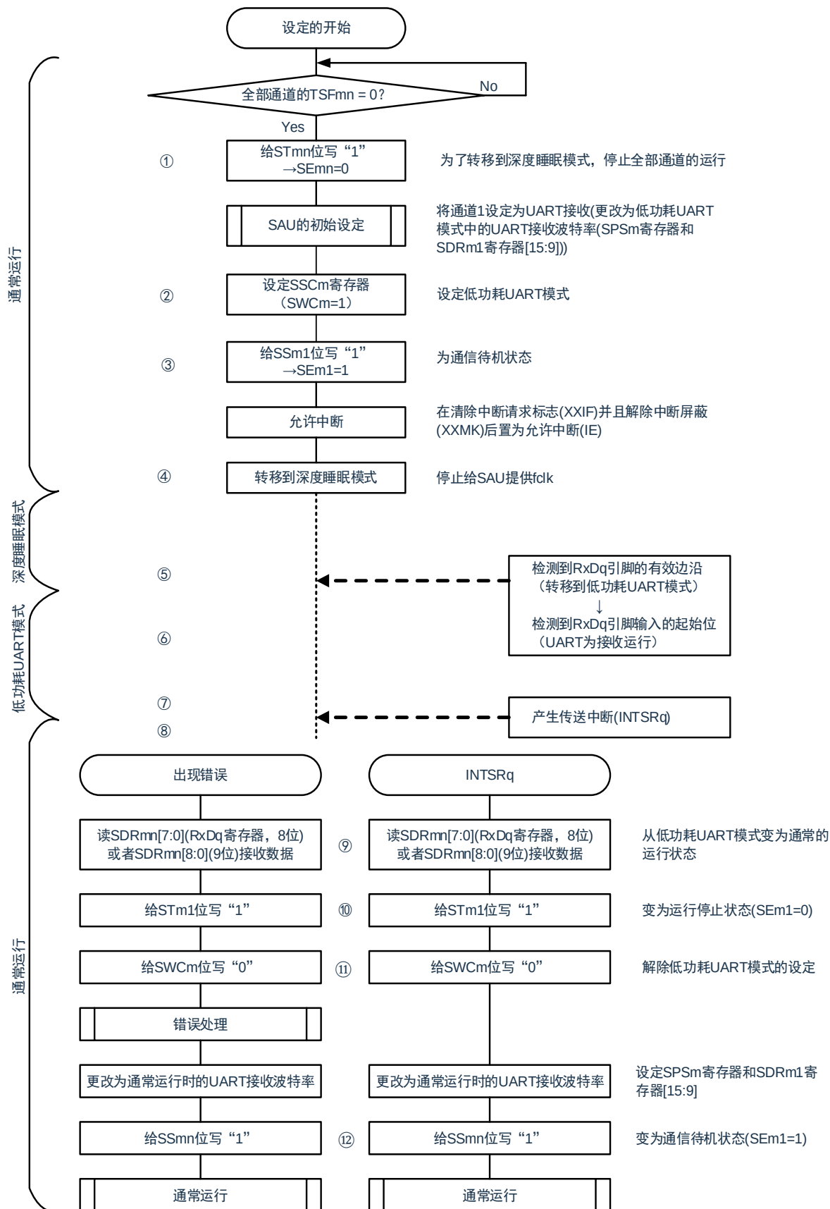
图 15-111: 低功耗 UART 模式运行 (EOCm1=0、SSECm=0/1) 的流程图
