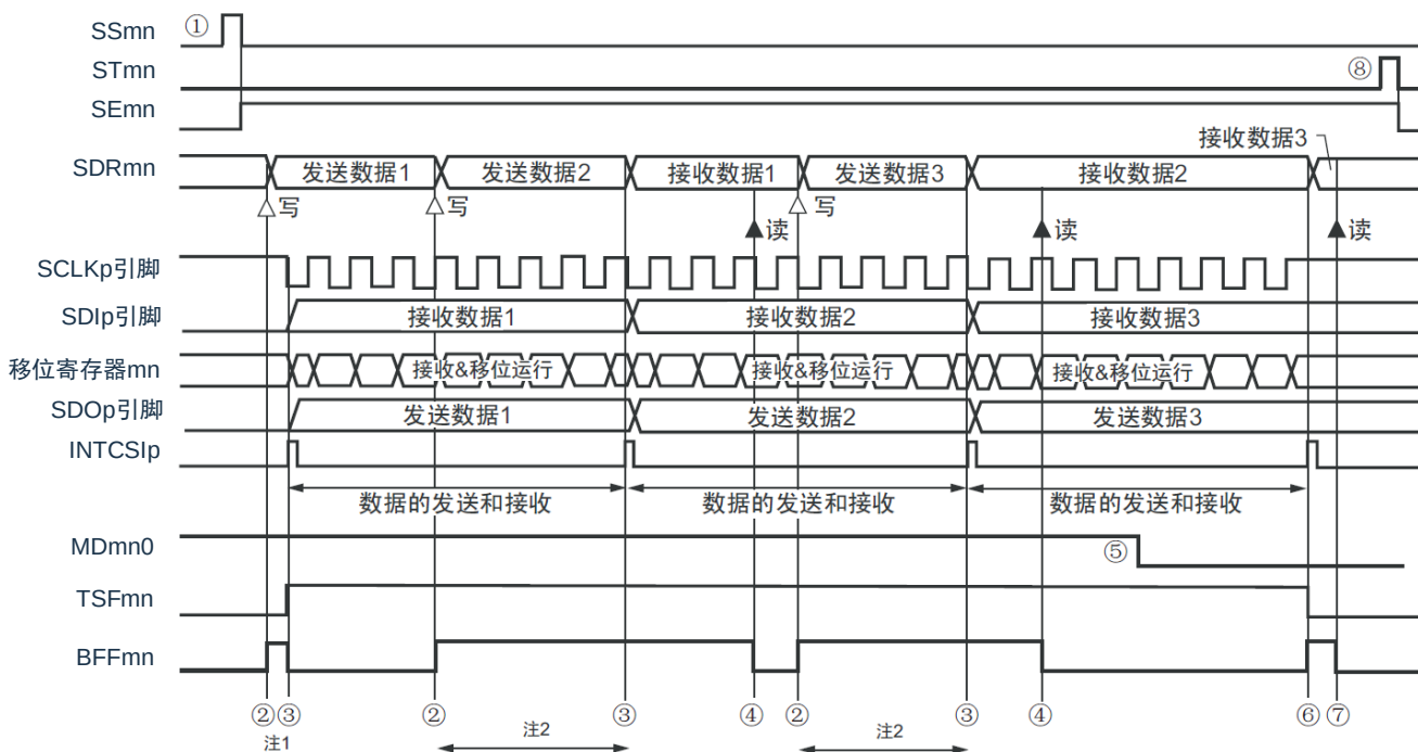
图 15-45：主控发送和接收（连续发送和接收模式）的时序图（类型 1：DAPmn=0、CKPmn=0）
