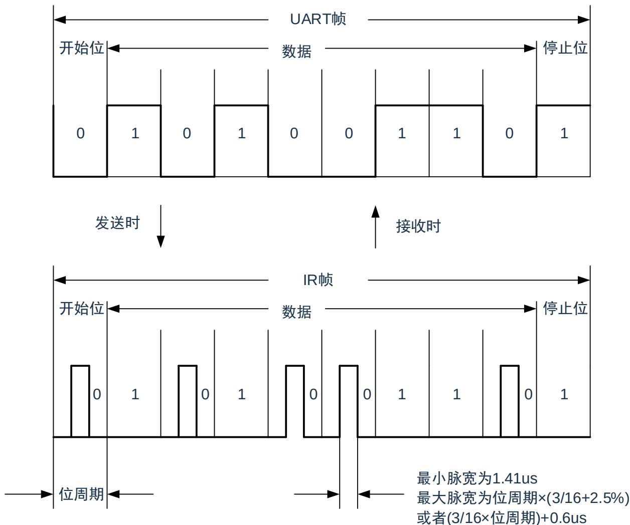
图 18-4：IrDA 的发送/接收运行图
