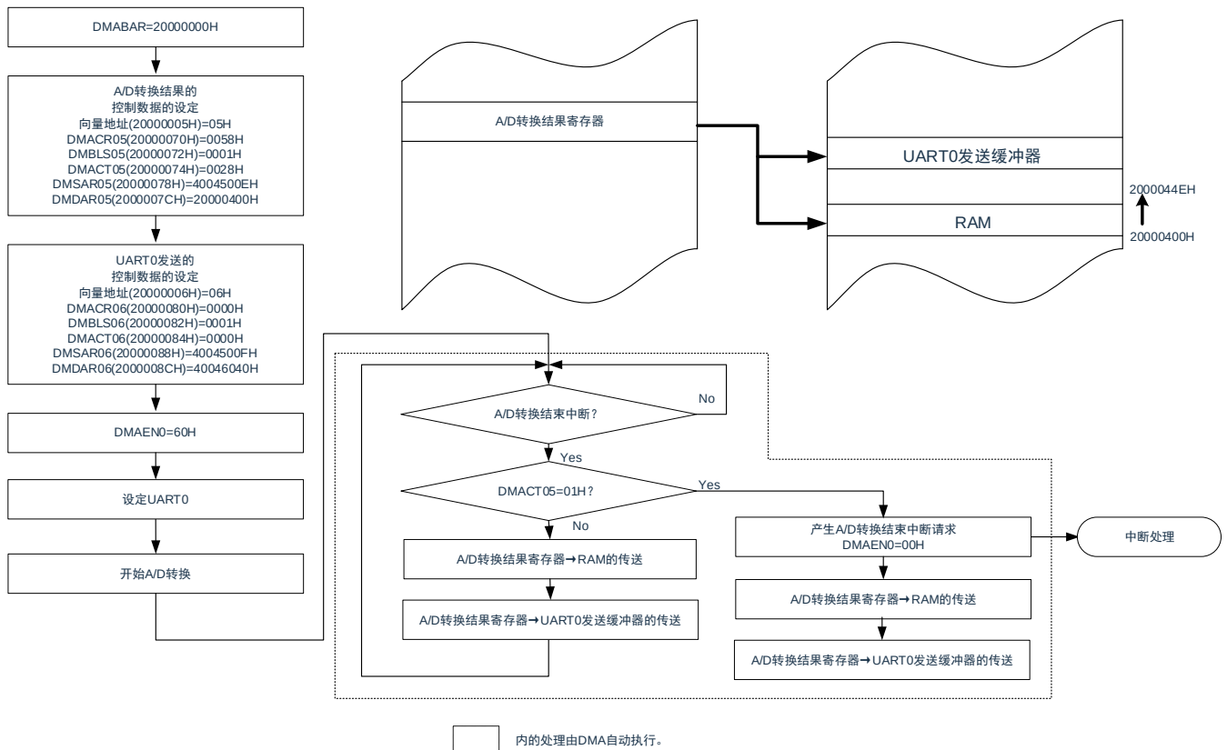
图 20-22：链传送的使用例子：连续取 A/D 转换结果进行 UART0 发送
