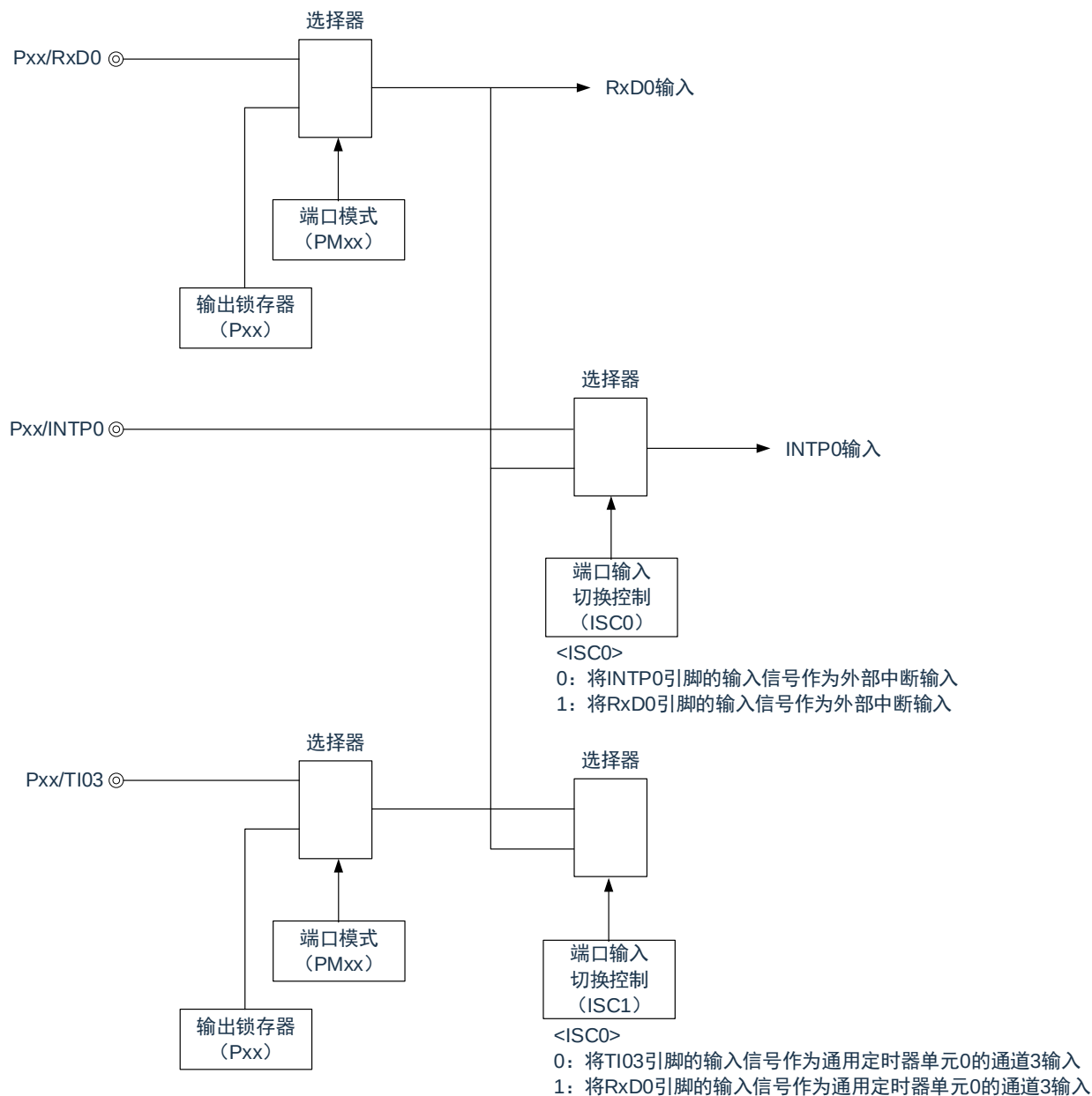
图 15-121：用于 LIN 接收操作的端口结构图
