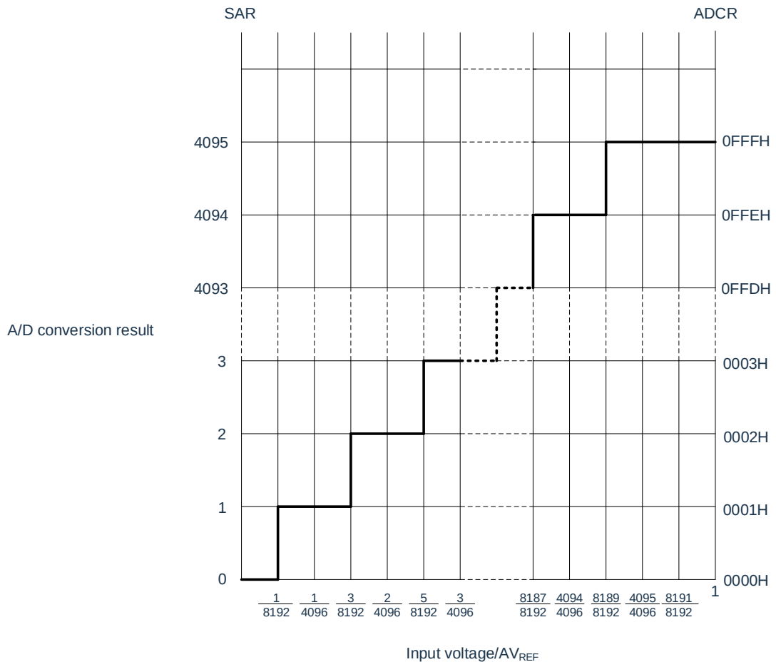
图 11-17: 模拟输入电压和 A/D 转换结果的关系
