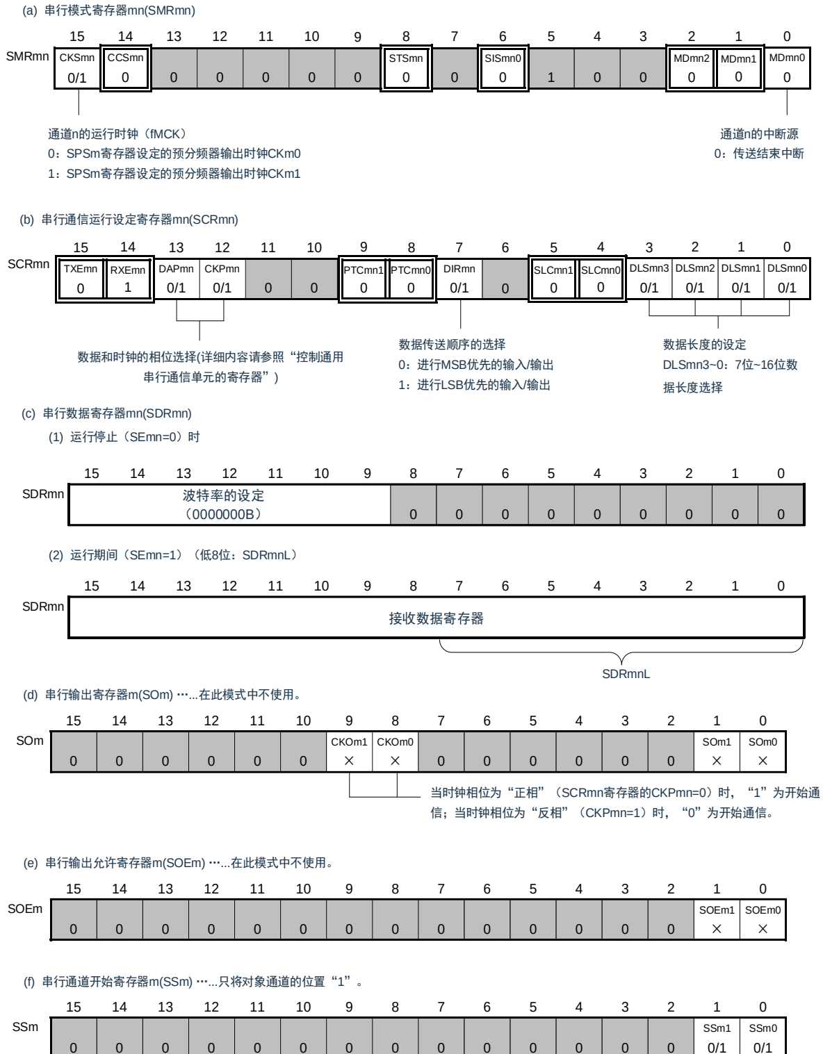
图 15-55: 3 线串行 I/O (SSPI00、SSPI01、SSPI10、SSPI11、SSPI20、SSPI21) 从属接收时的寄存器设定内容例子
