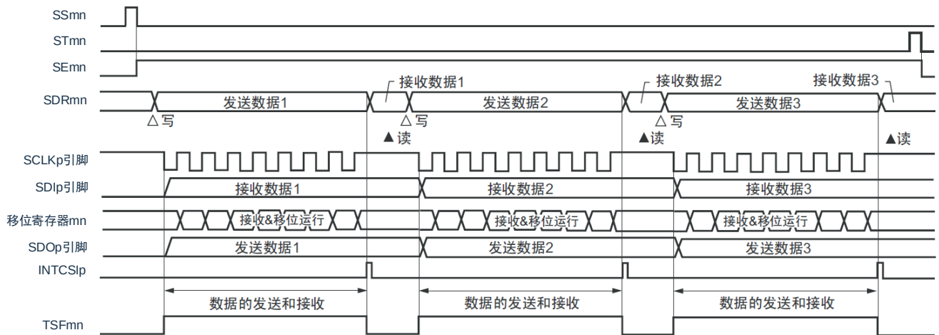
图 15-43：主控发送和接收（单次发送和接收模式）的时序图（类型 1：DAPmn=0、CKPmn=0）
