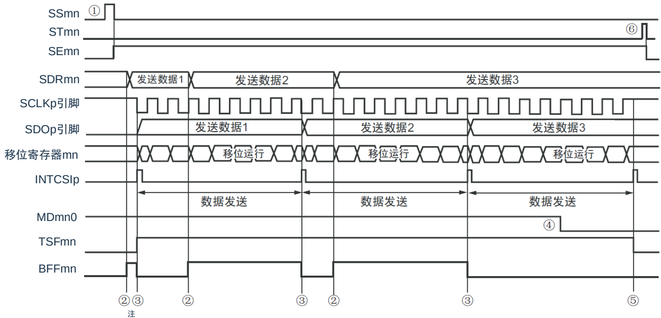
图 15-29：主控发送（连续发送模式）的时序图（类型 1：DAPmn=0、CKPmn=0）
