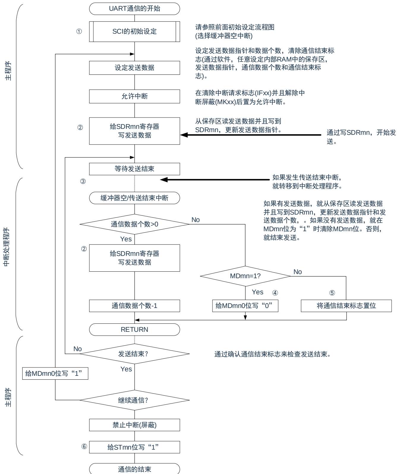
图 15-103: UART 发送（连续发送模式）的流程图
