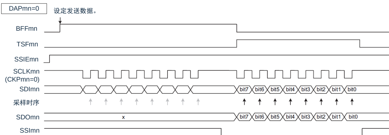
图 15-71：从属选择输入功能的时序图
