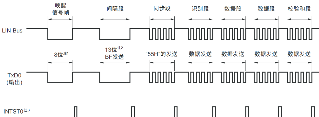
图 15-117: LIN 的发送操作
