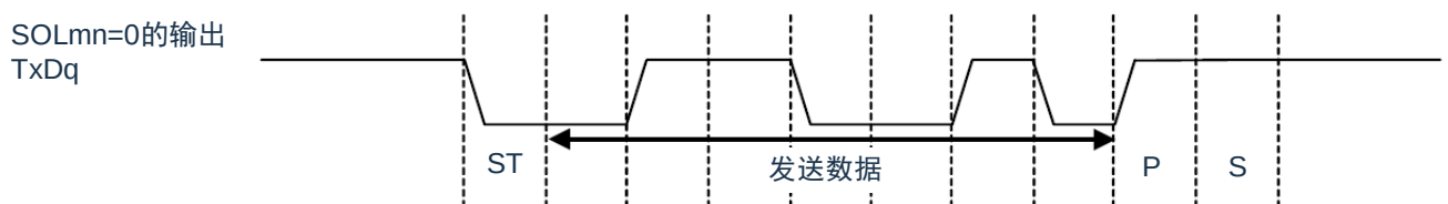
图 15-16: 发送数据的电平反相例子
