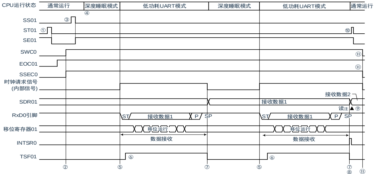
图 15-112：低功耗 UART 模式运行 (EOCm1=1、SSECm=1) 的时序图
