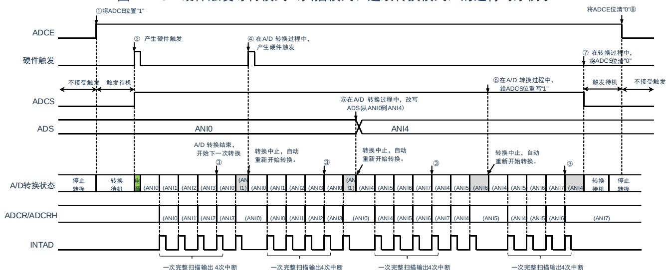
图 11-28：硬件触发等待模式（扫描模式、连续转换模式）的运行时序例子
