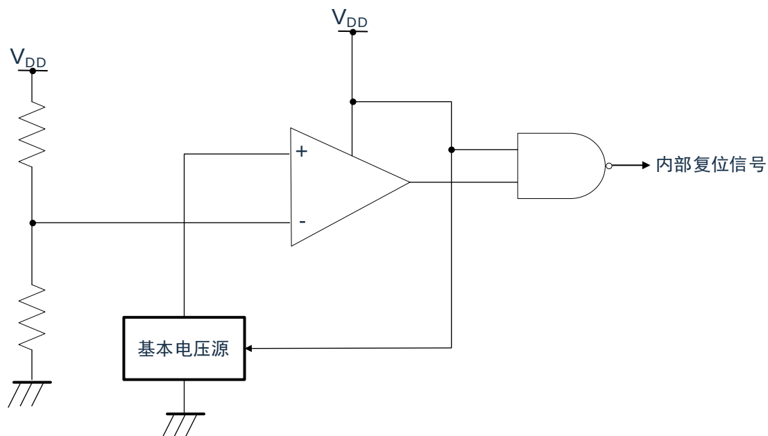
图 26-1：上电复位电路的框图
