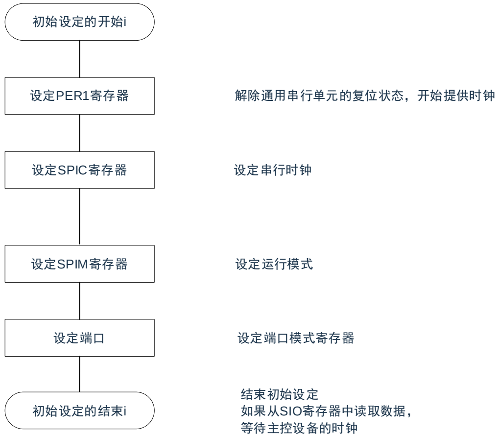
图 16-18：从属接收的初始设置步骤
