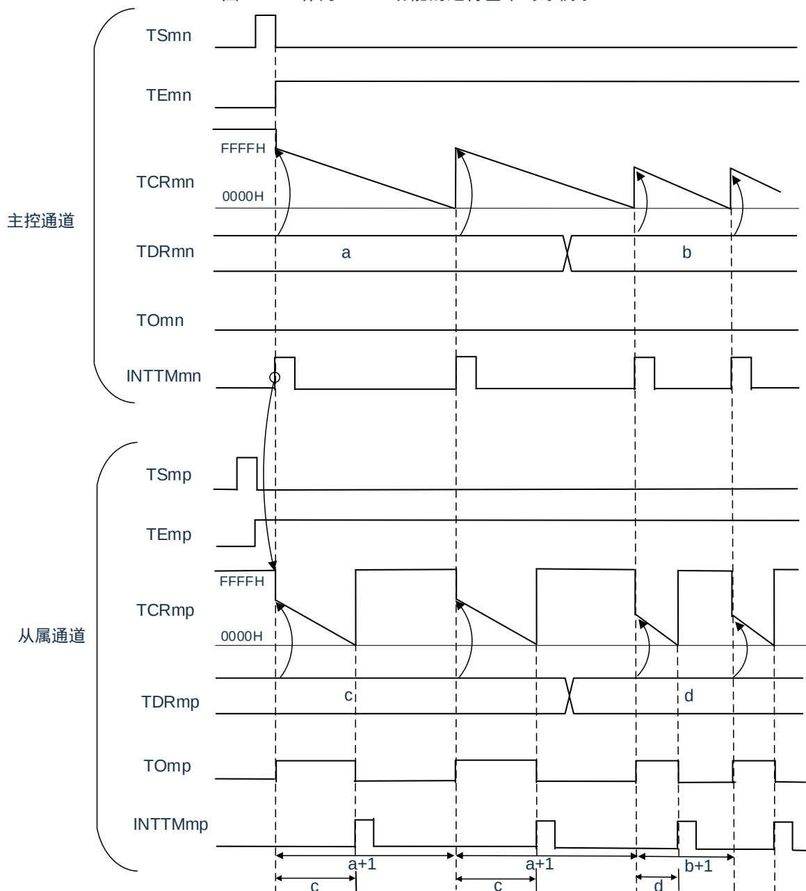
图 5-67: 作为 PWM 功能的运行基本时序例子
