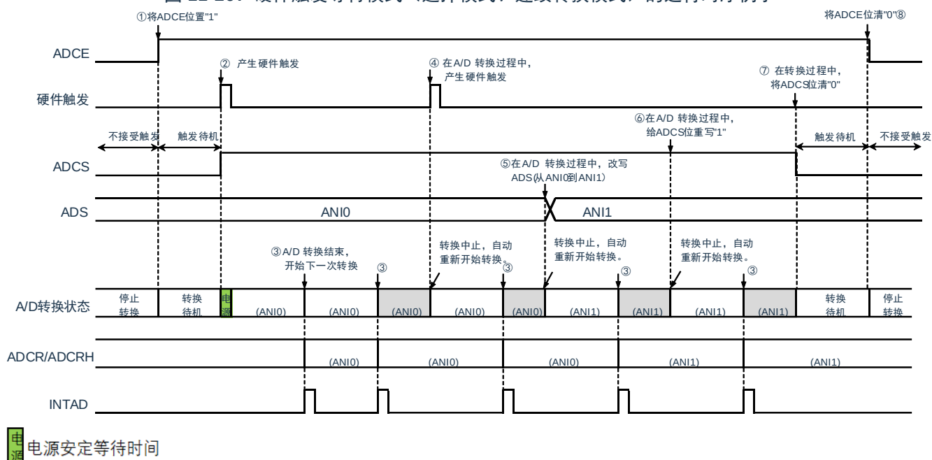
图 11-26：硬件触发等待模式（选择模式、连续转换模式）的运行时序例子
