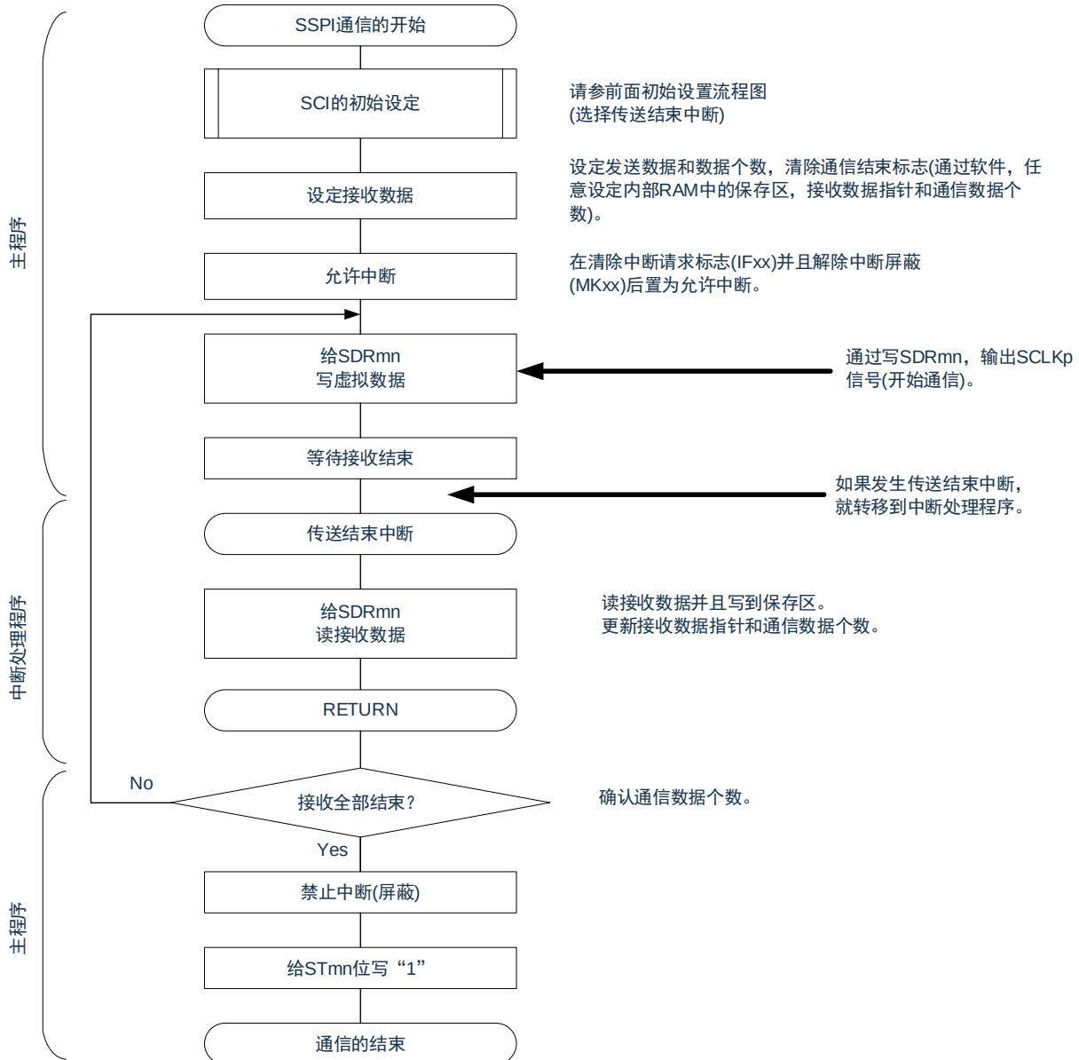
图 15-36: 主控接收（单次接收模式）的流程图
