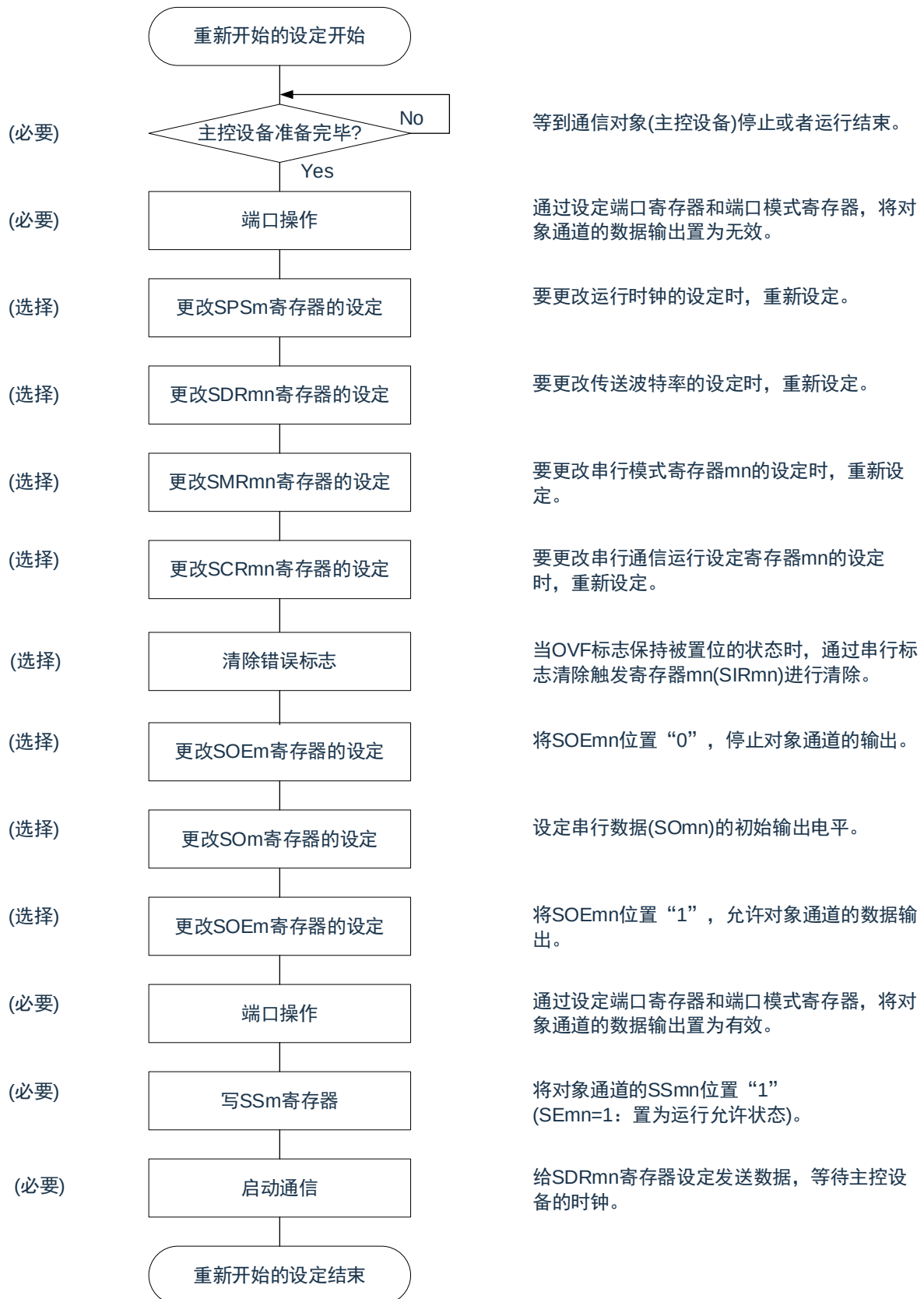
图 15-50：重新开始从属发送的设定步骤
