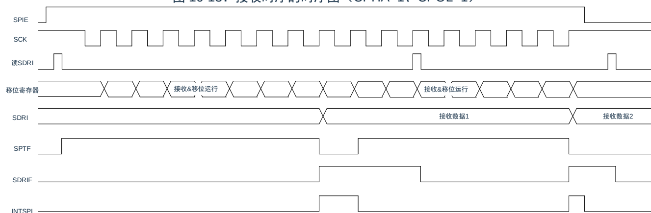
图 16-13: 接收时序的时序图 (CPHA=1、CPOL=1)
