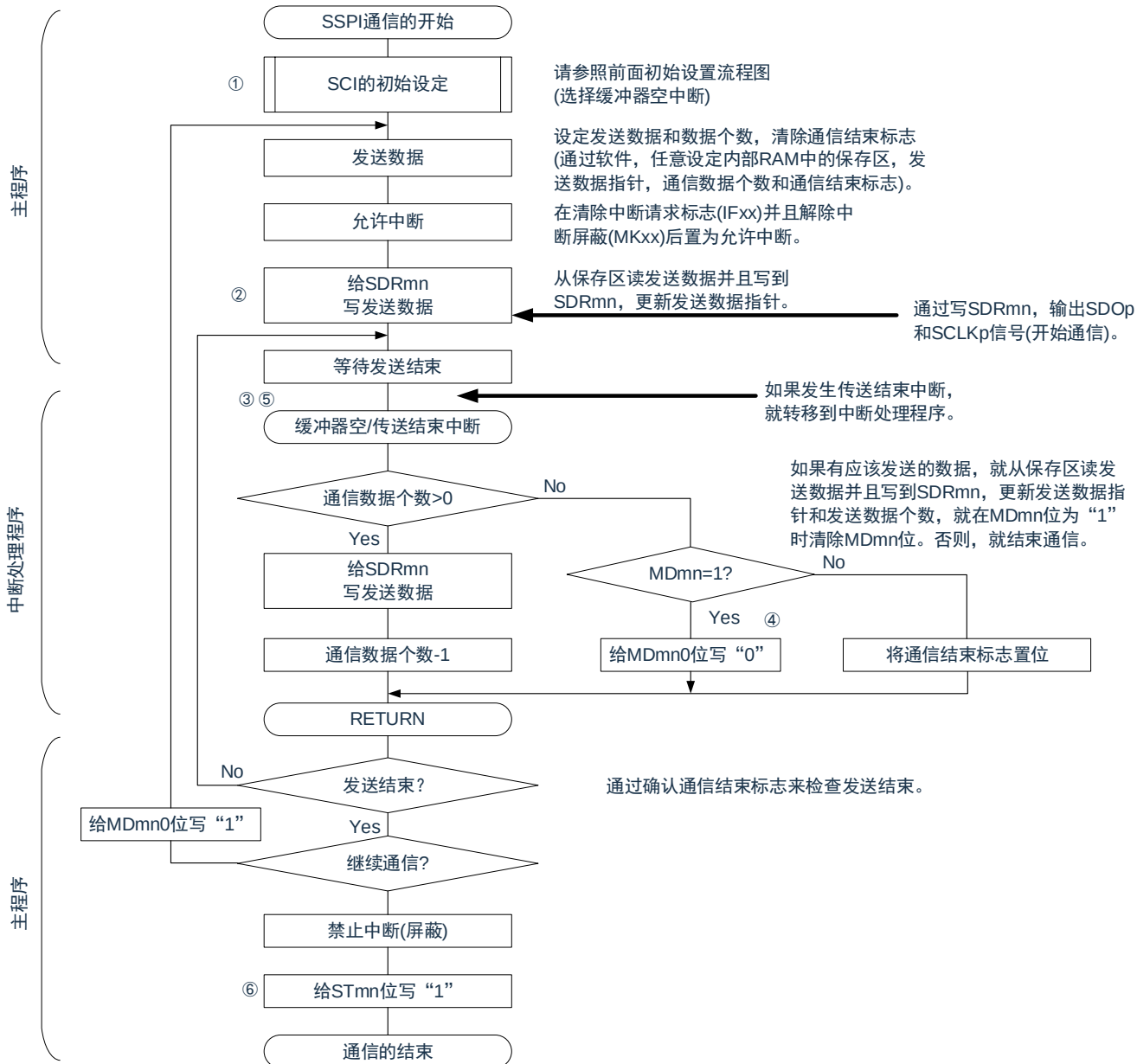
图 15-30: 主控发送（连续发送模式）的流程图
