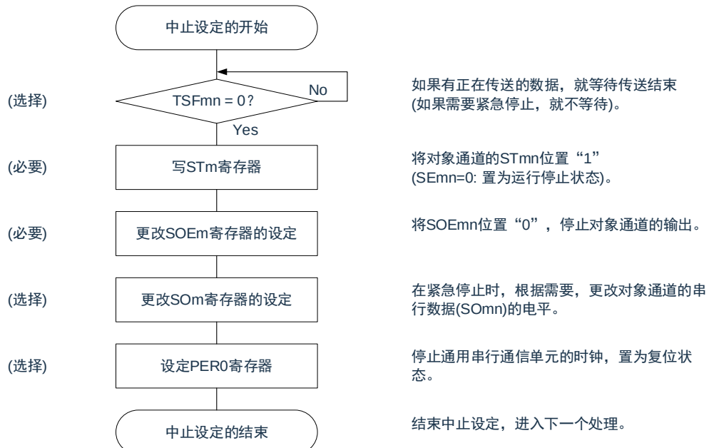
图 15-49：从属发送的中止步骤
