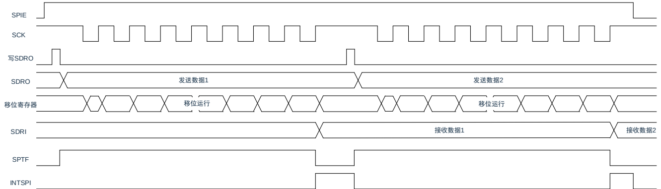
图 16-10: 发送/接收时序(连续发送模式)的时序图 (INTMD=1,CPHA=1、CPOL=1)
