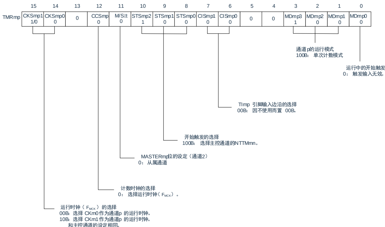
图 5-63: 单触发脉冲输出功能时（从属通道）的寄存器设定内容例子
