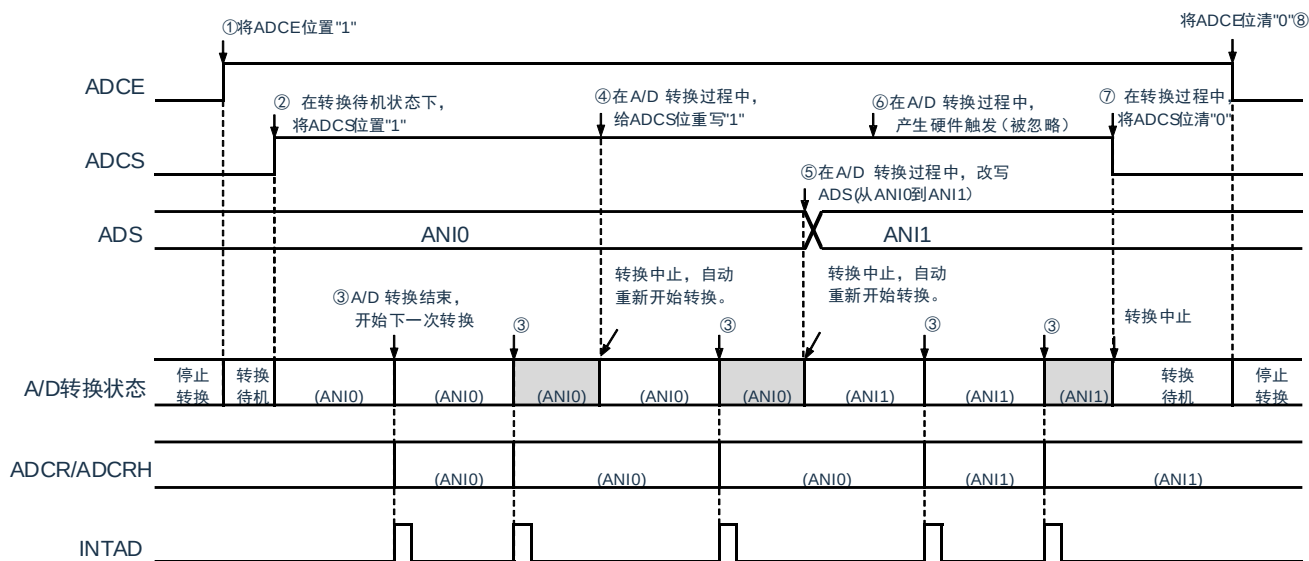
图 11-18：软件触发模式（选择模式、连续转换模式）的运行时序例子
