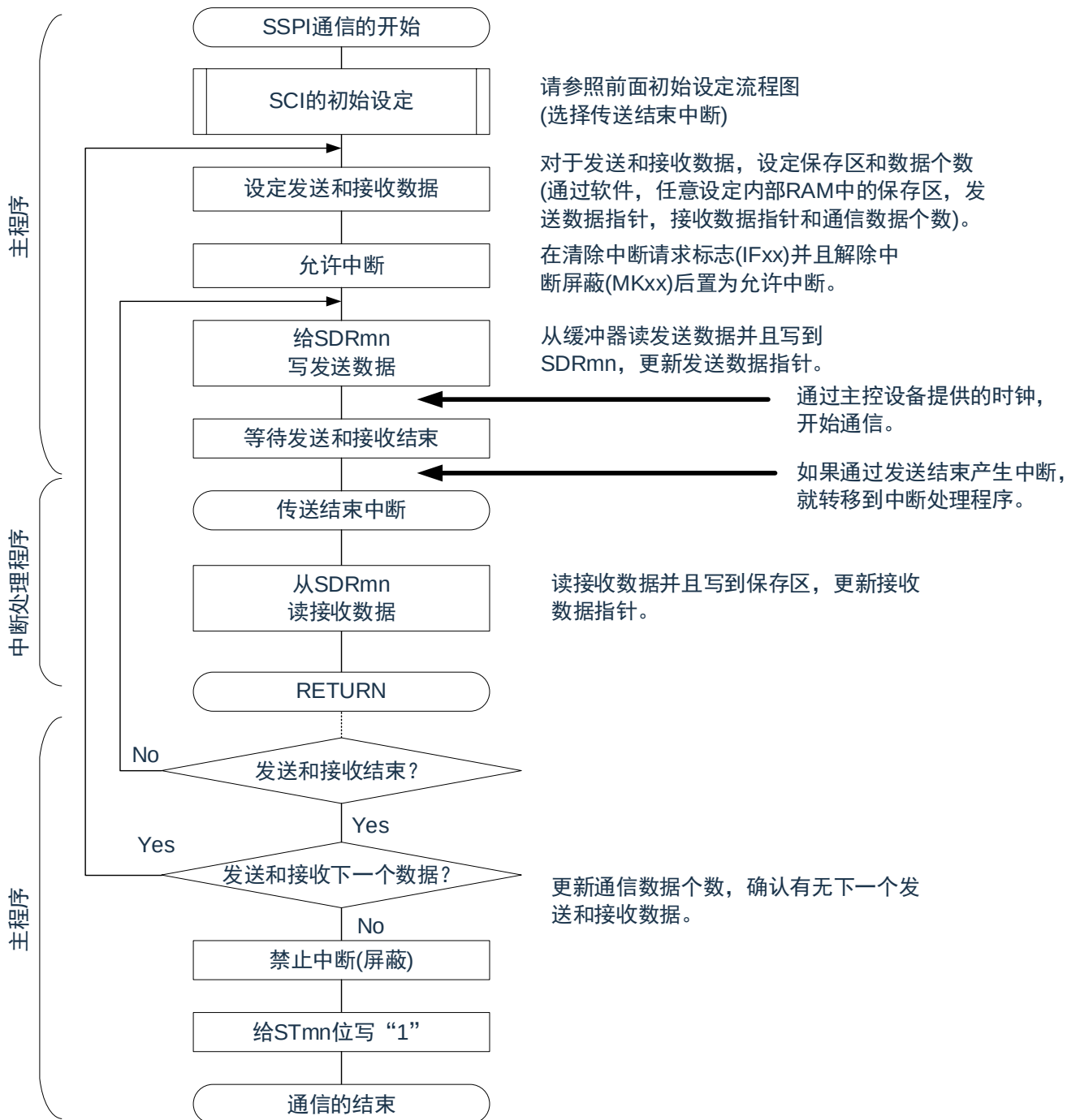
图 15-66: 从属发送和接收（单次发送和接收模式）的流程图
