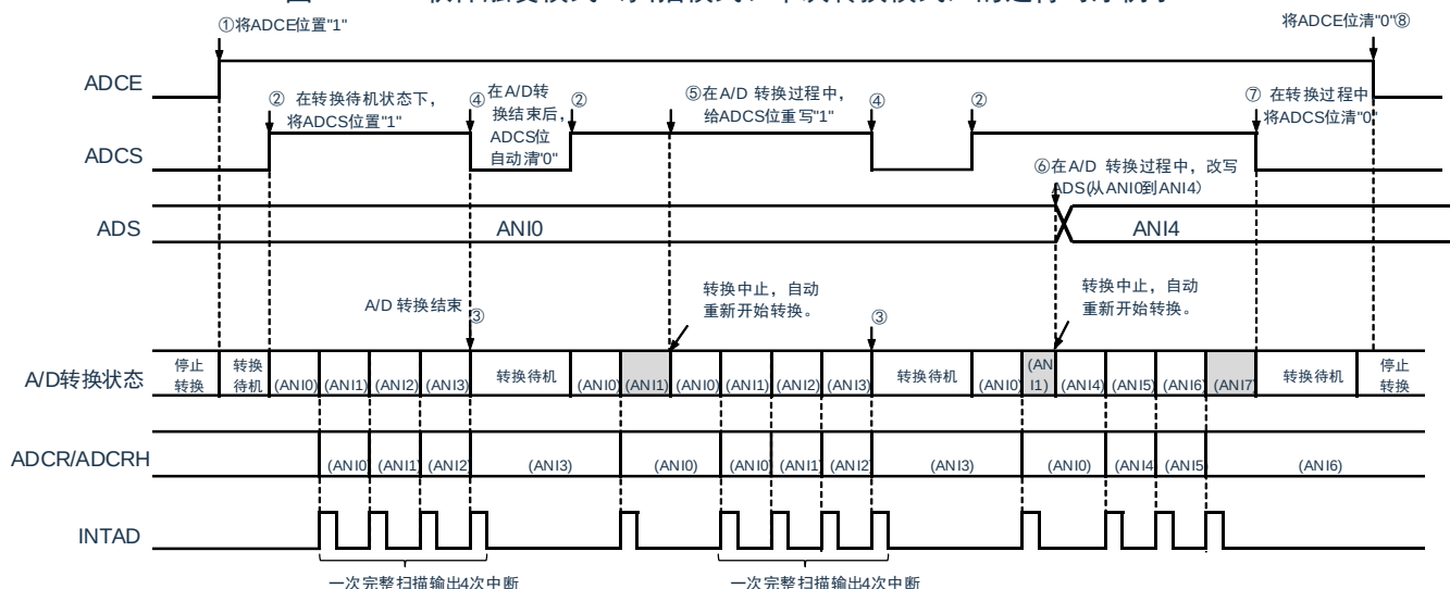
图 11-21：软件触发模式（扫描模式、单次转换模式）的运行时序例子
