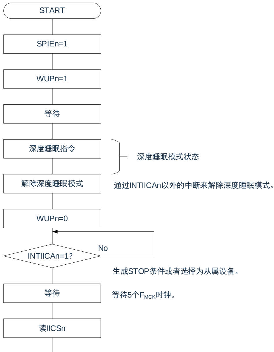
图 17-23: 在通过 INTIICAn 以外的中断来解除深度睡眠模式后作为主控设备运行的情况
