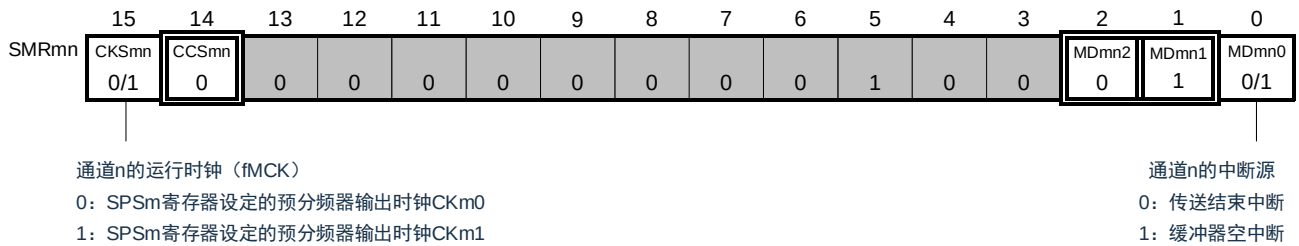
图 15-96: UART (UART0~UART2) 的 UART 发送时的寄存器设定内容例子(1/2)
