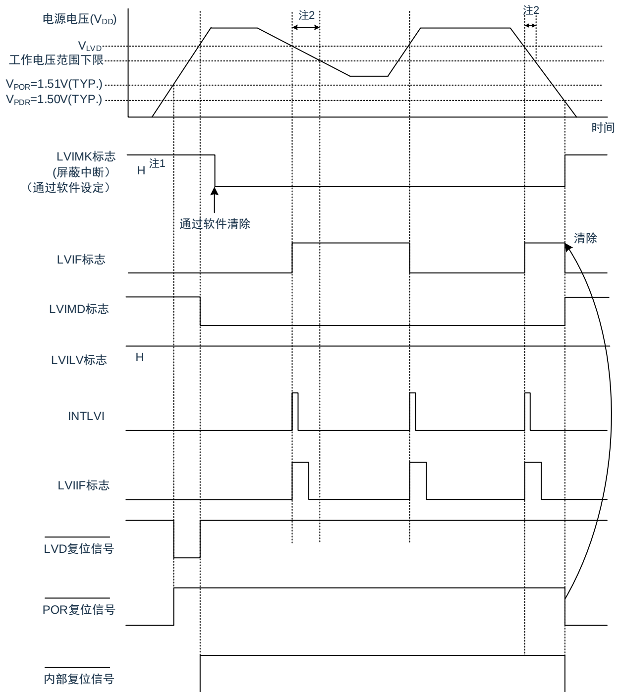
图 27-5：中断信号的产生时序（选项字节的 LVIMDS1、LVIMDS0=0、1）
