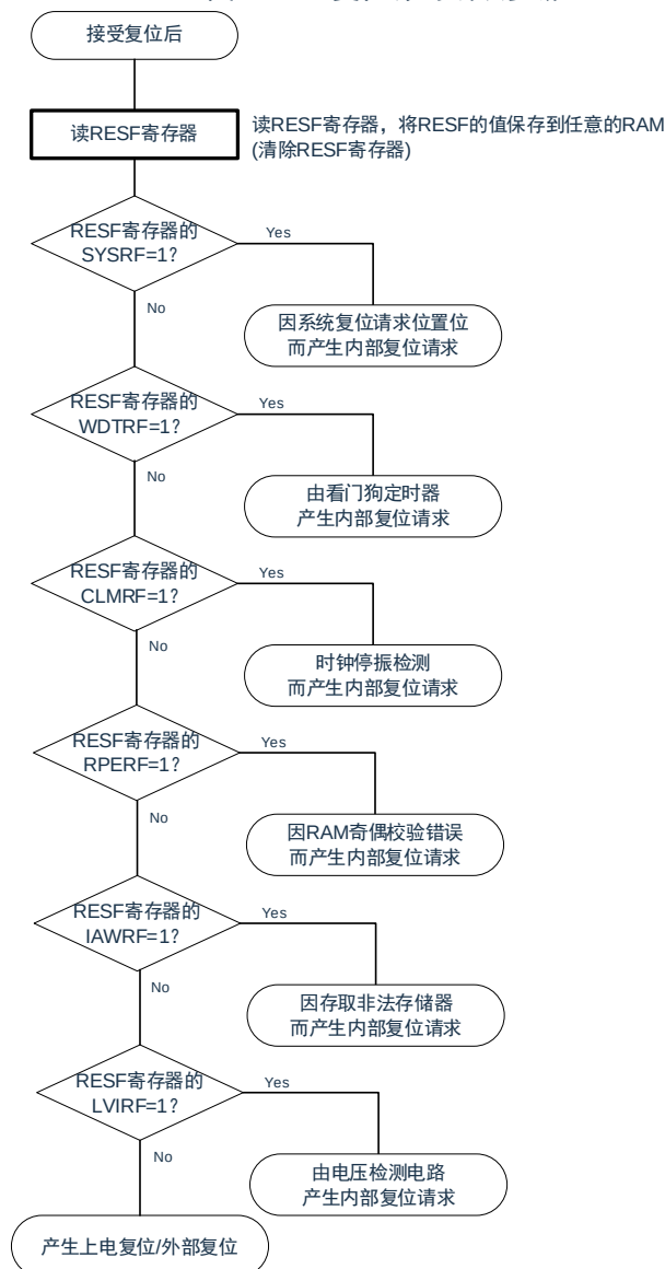
图 25-5：复位源的确认步骤
