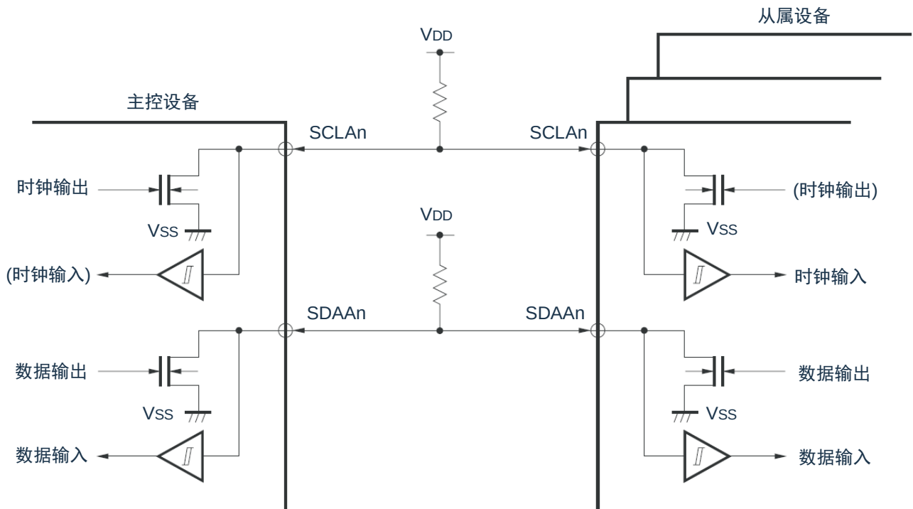
图 17-12: 引脚结构图
