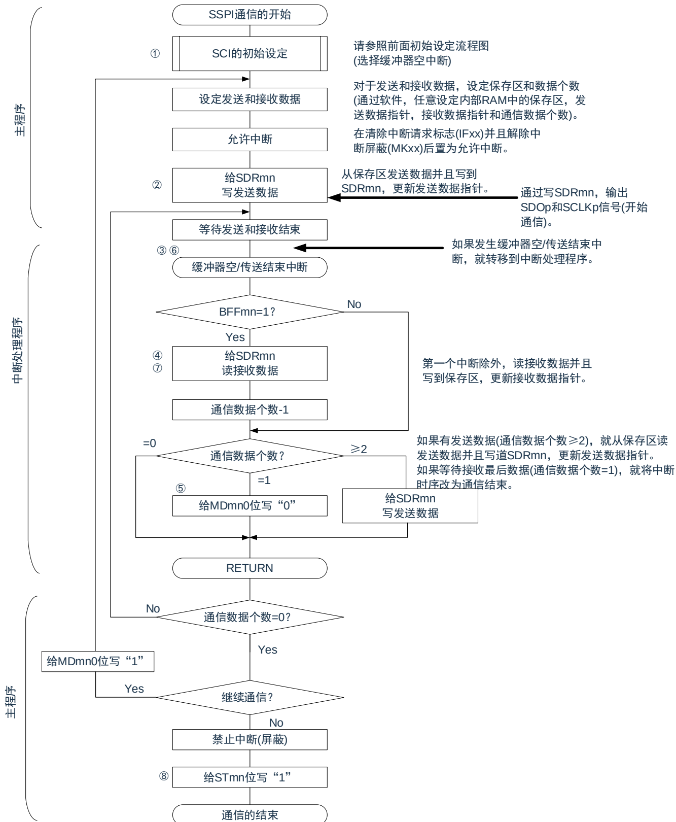
图 15-46: 主控发送和接收（连续发送和接收模式）的流程图
