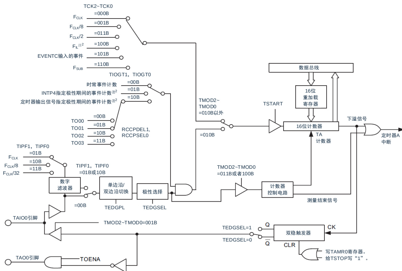
图 6-1: 定时器 A 的框图
