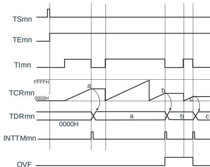
图 5-54: 作为输入信号高低电平宽度测量的运行基本时序例子
