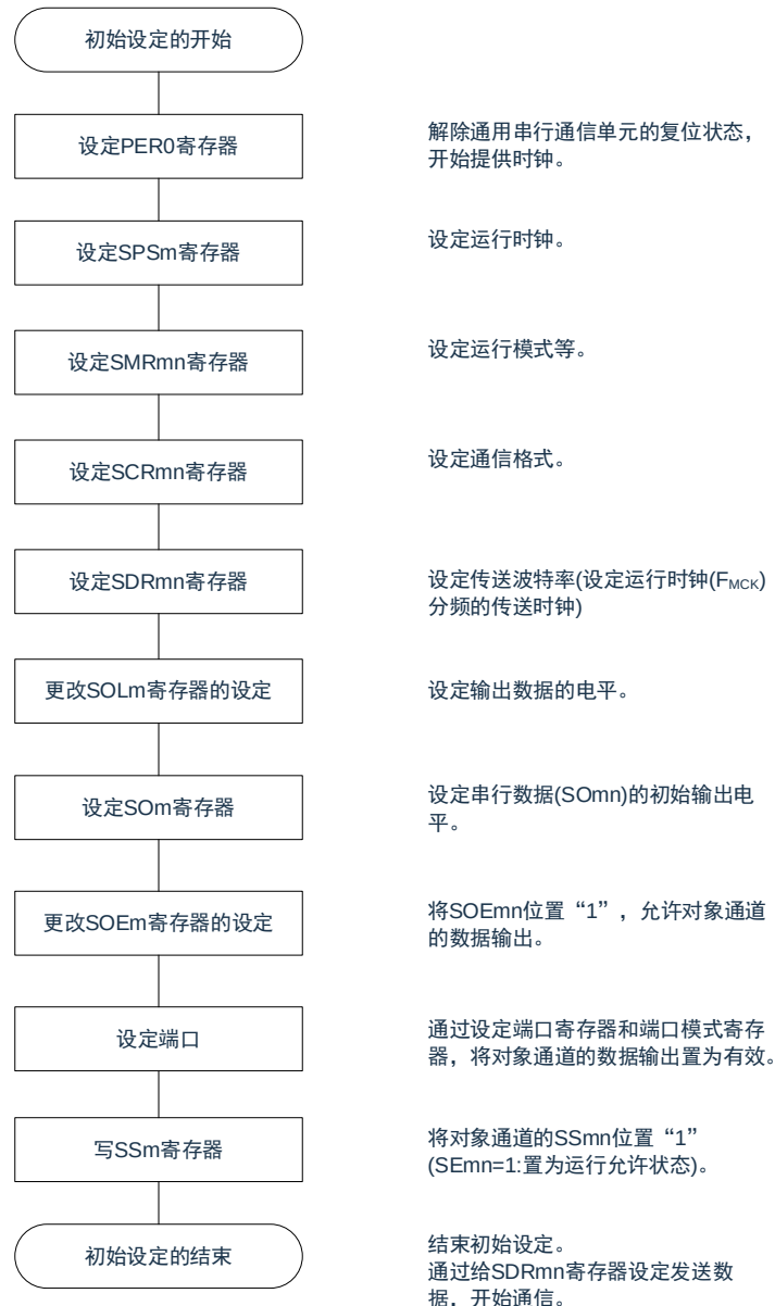
图 15-97: UART 发送的初始设定步骤
