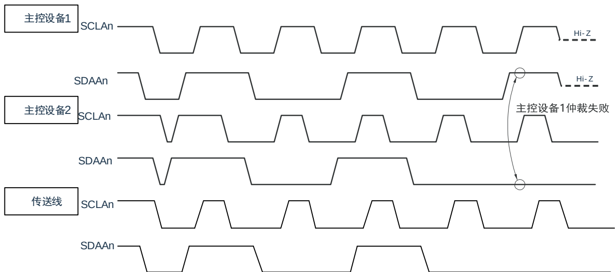
图 17-20：仲裁时序例子
