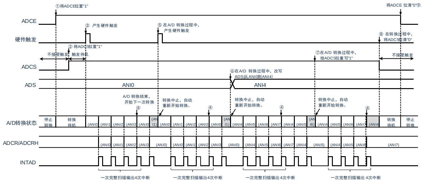
图 11-24：硬件触发无等待模式（扫描模式、连续转换模式）的运行时序例子
