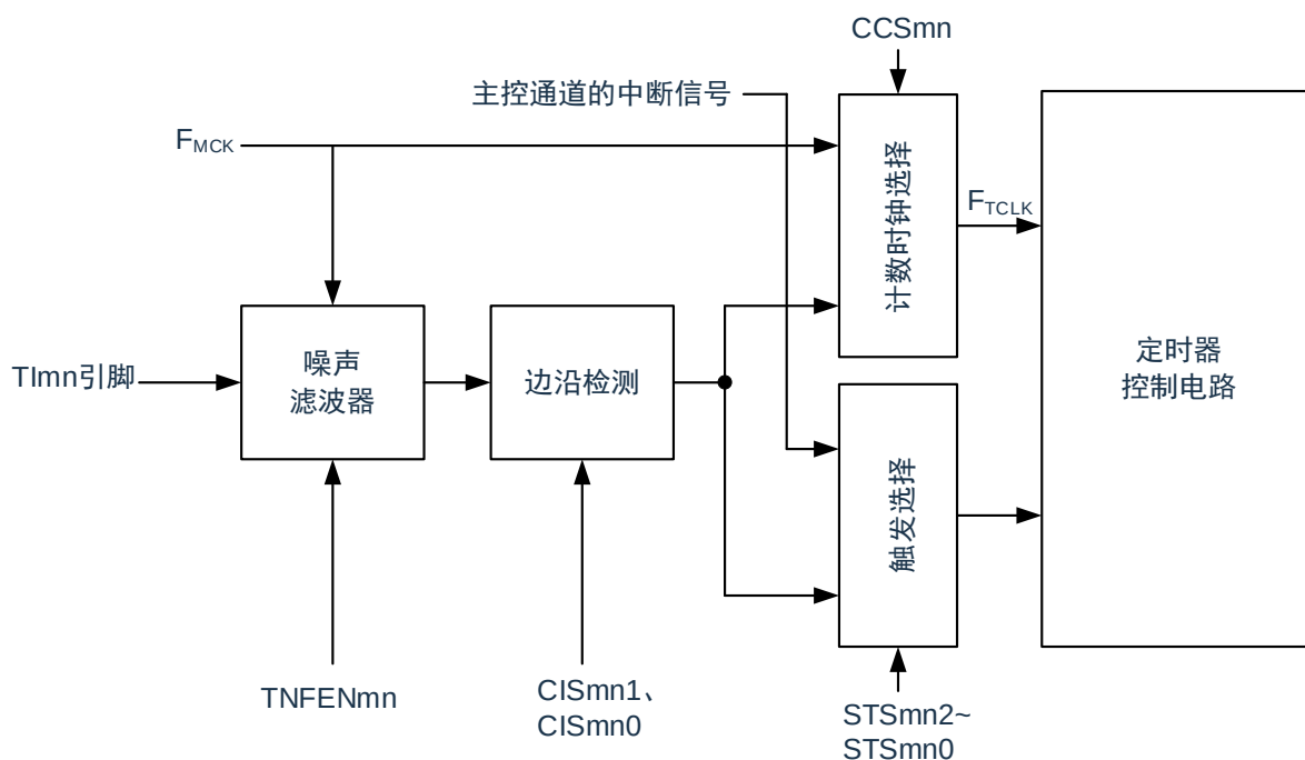
图 5-39：输入电路的结构
