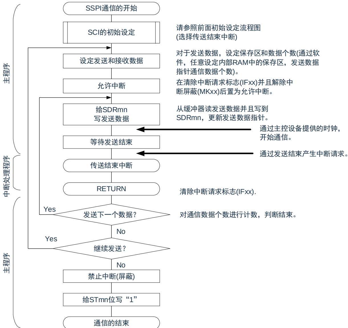
图 15-52: 从属发送（单次发送模式）的流程图
