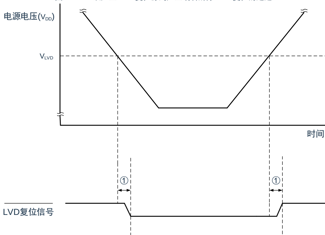
图 27-10：从产生 LVD 复位源到产生或者解除 LVD 复位的延迟
