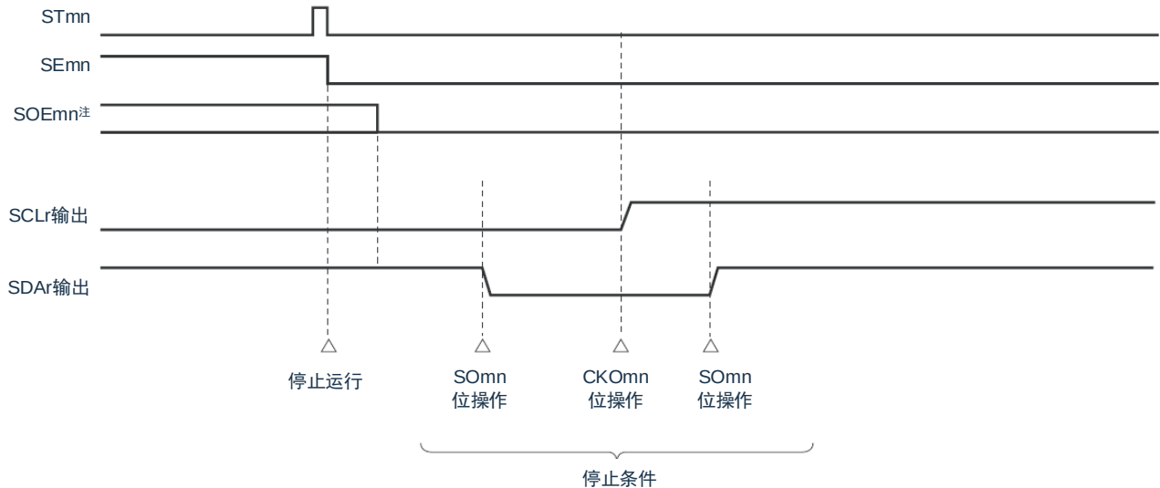
图 15-132：产生停止条件的时序图
