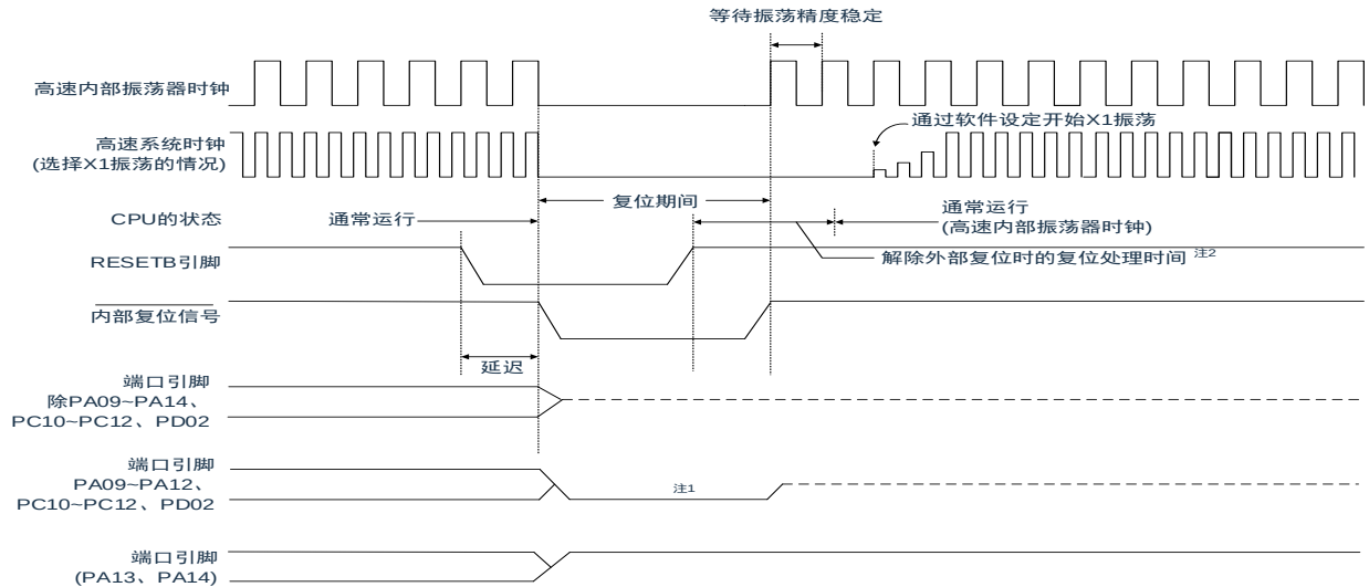
图 25-2: RESETB 输入的复位时序
