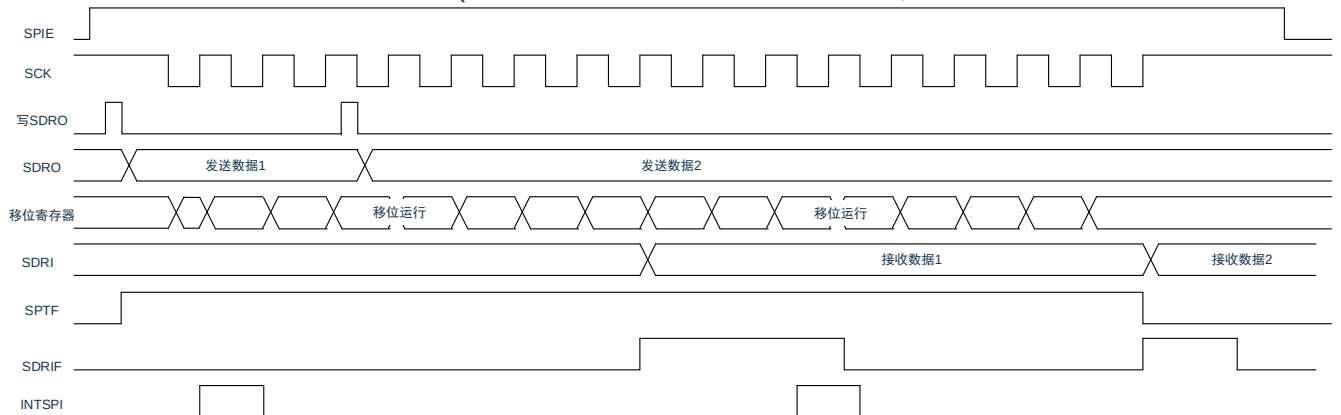
图 16-10: 发送/接收时序(连续发送模式)的时序图 (INTMD=1,CPHA=1、CPOL=1)
