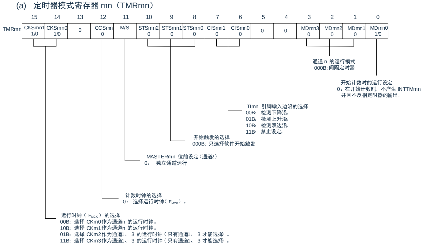
图 5-46：外部事件计数器模式时的寄存器设定内容例子
