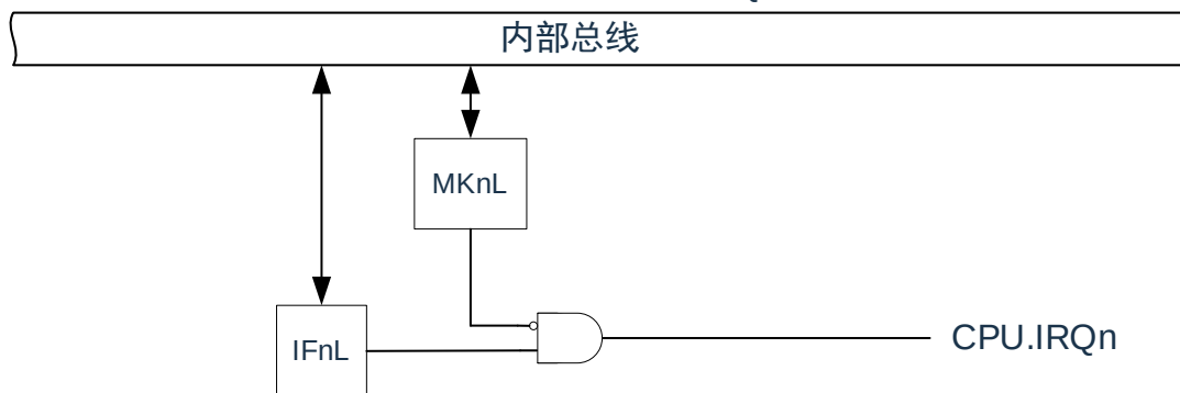
图 22-4：各标志寄存器与 CPU.IRQ 的关系
