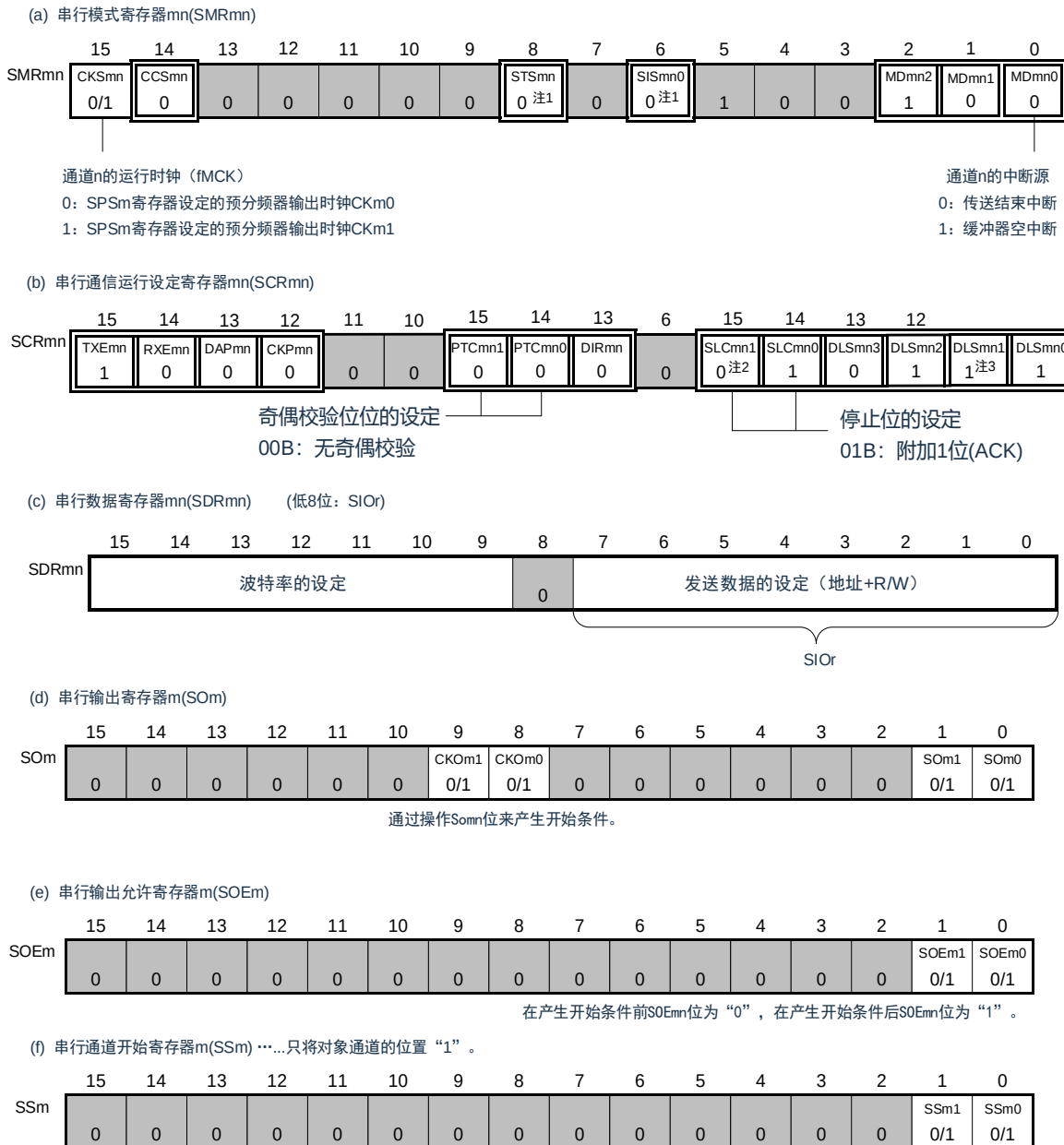
图 15-122: 简易 I 2 C (IIC00、IIC01、IIC10、IIC11、IIC20、IIC21) 地址段发送时的寄存器设定内容例子
