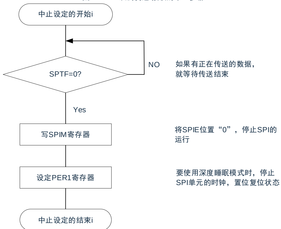
图 16-15：从属发送/接收的中止步骤
