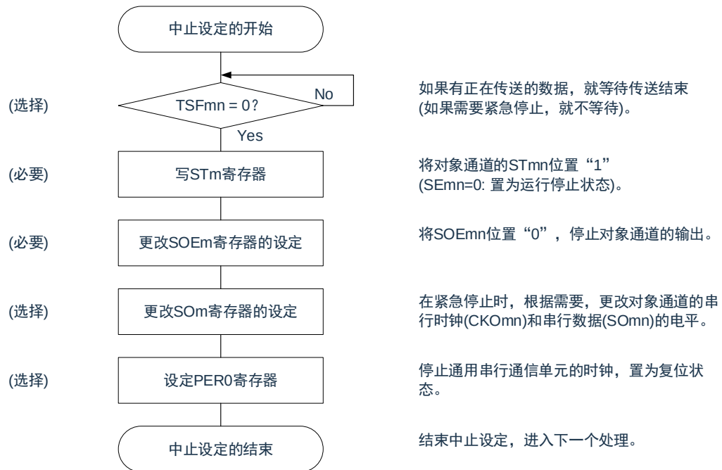
图 15-33: 主控接收的中止步骤
