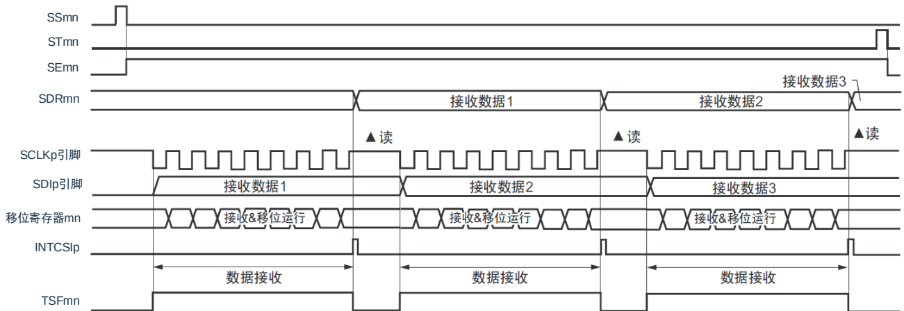
图 15-59：从属接收（单次接收模式）的时序图（类型 1：DAPmn=0、CKPmn=0）
