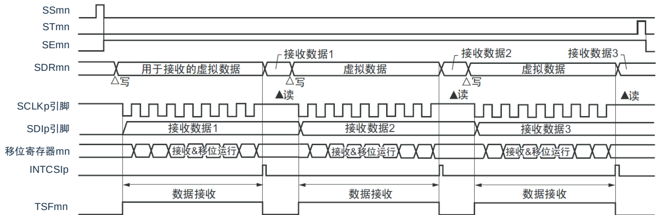
图 15-35：主控接收（单次接收模式）的时序图（类型 1：DAPmn=0、CKPmn=0）
