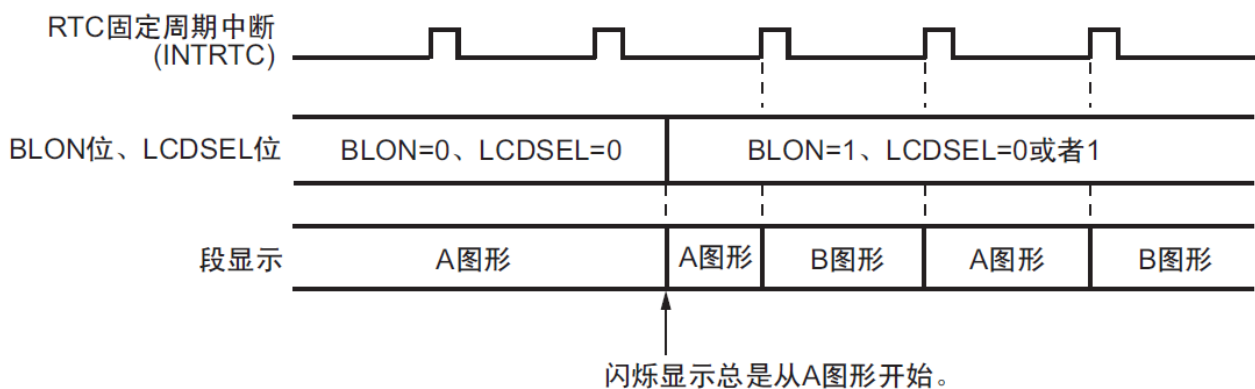
图 19-9：从 A 图形显示到闪烁显示的切换运行
