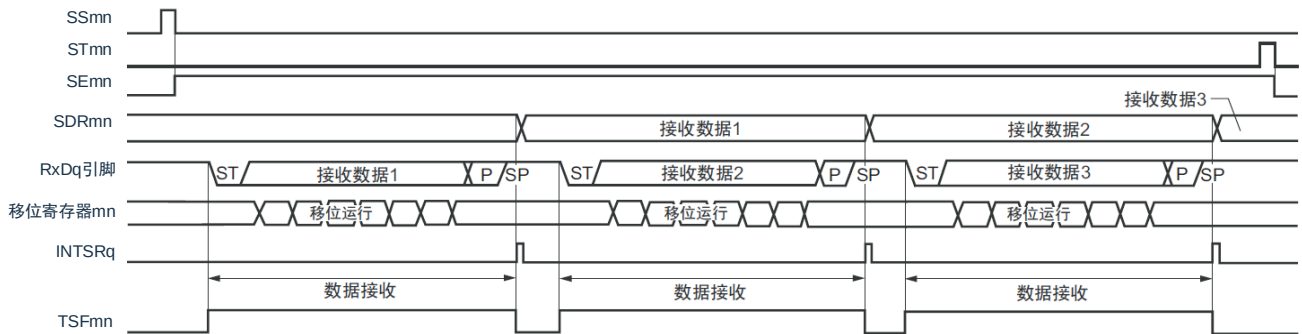
图 15-108: UART 接收的时序图
