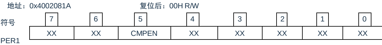
图 13-3：外围允许寄存器 1（PER1）的格式
