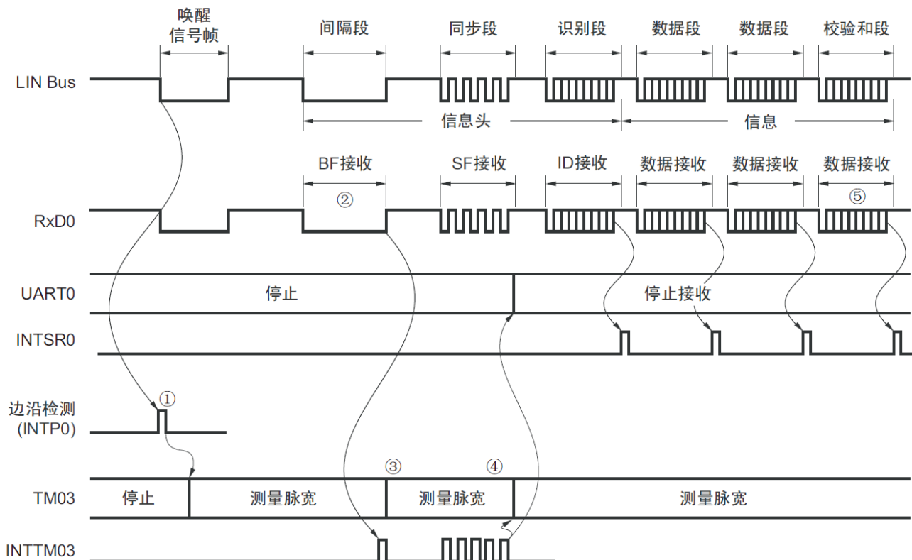
图 15-119: LIN 的接收操作
