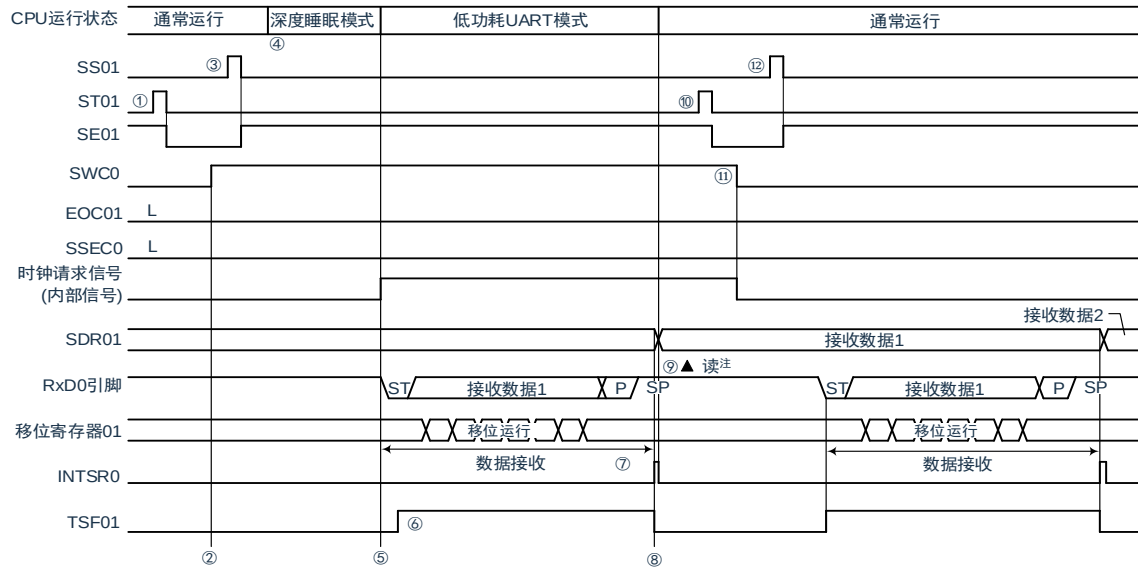
图 15-110：低功耗 UART 模式运行 (EOCm1=0、SSECm=0/1) 时序图
