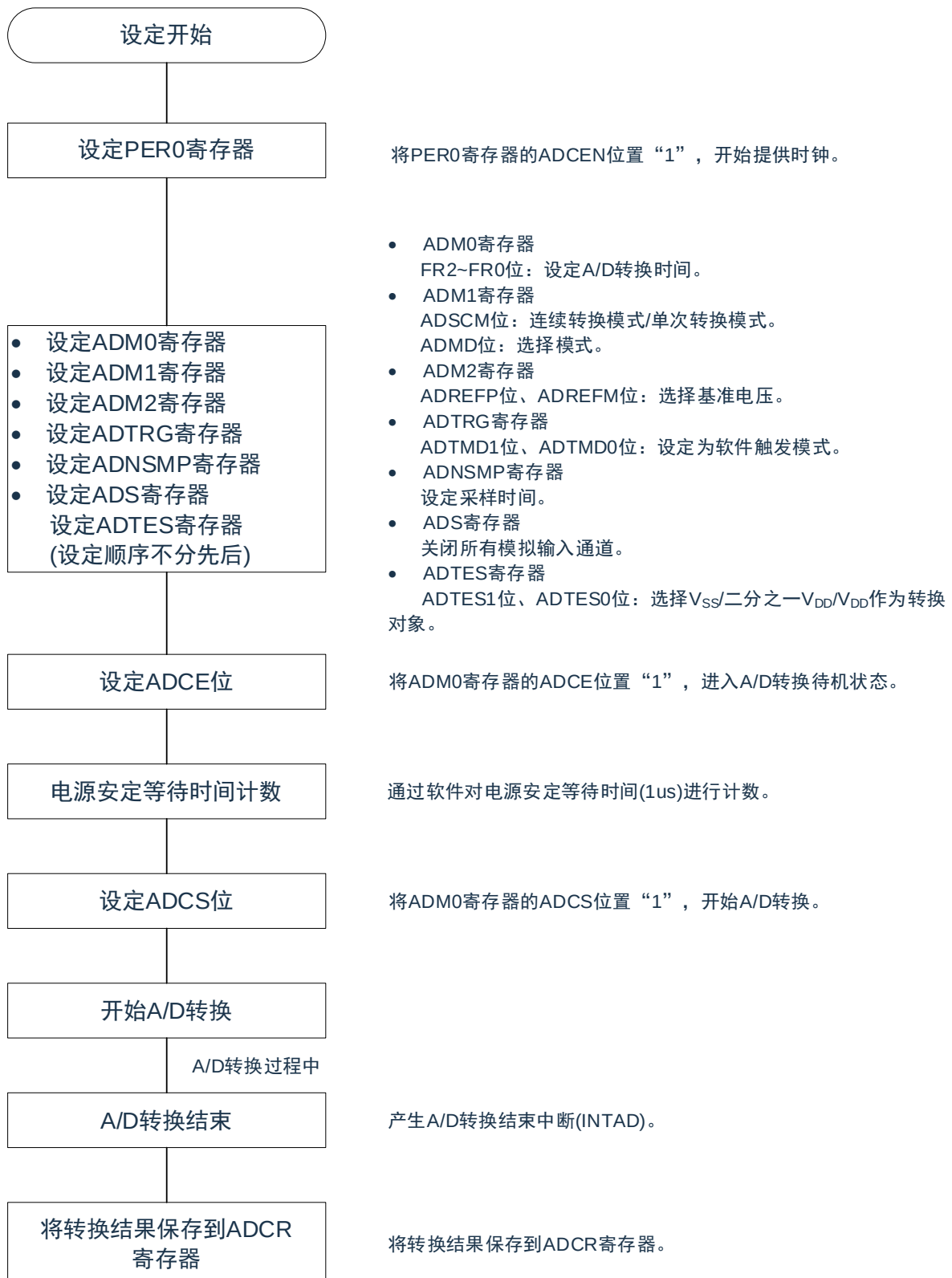
图 11-34：测试模式的设定( V_{SS}/half\_V_{DD}/V_{DD} 作为转换对象)
