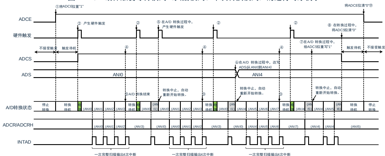
图 11-29：硬件触发等待模式（扫描模式、单次转换模式）的运行时序例子
