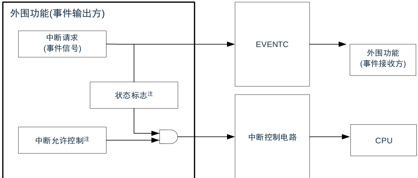
图 21-3：中断处理和 EVENTC 的关系
