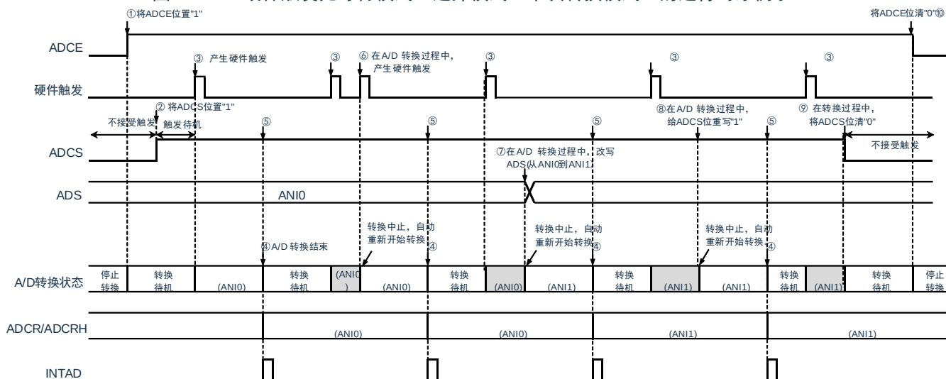
图 11-23：硬件触发无等待模式（选择模式、单次转换模式）的运行时序例子
