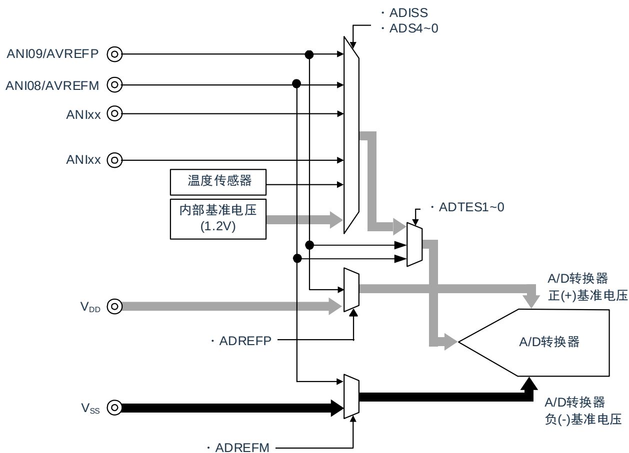
图 28-11: A/D 测试功能的结构
