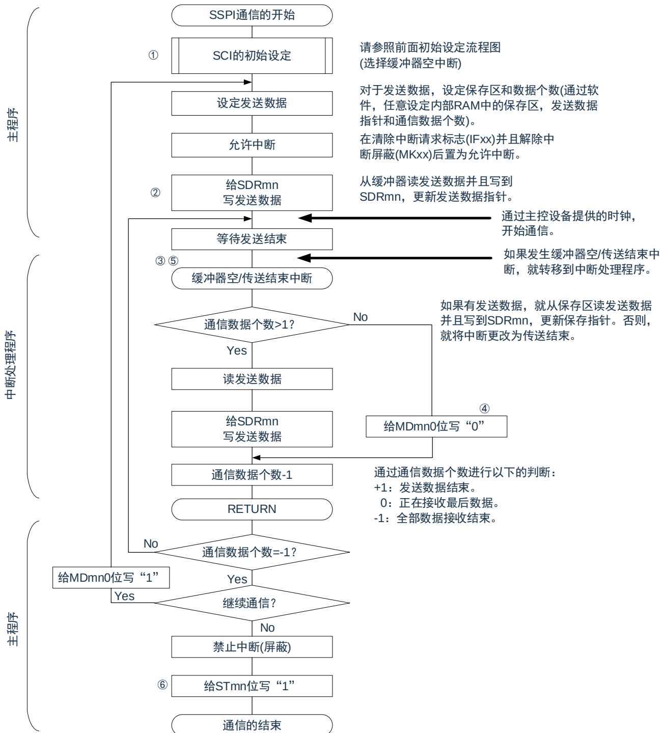
图 15-79: 从属发送（连续发送模式）的流程图
