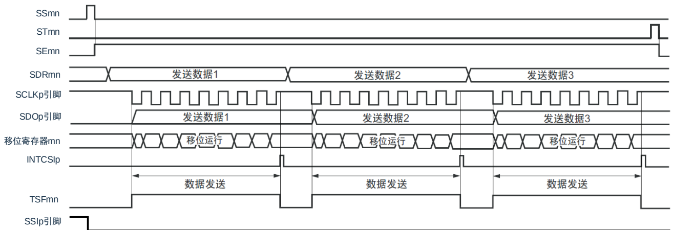
图 15-76：从属发送（单次发送模式）的时序图（类型 1：DAPmn=0、CKPmn=0）
