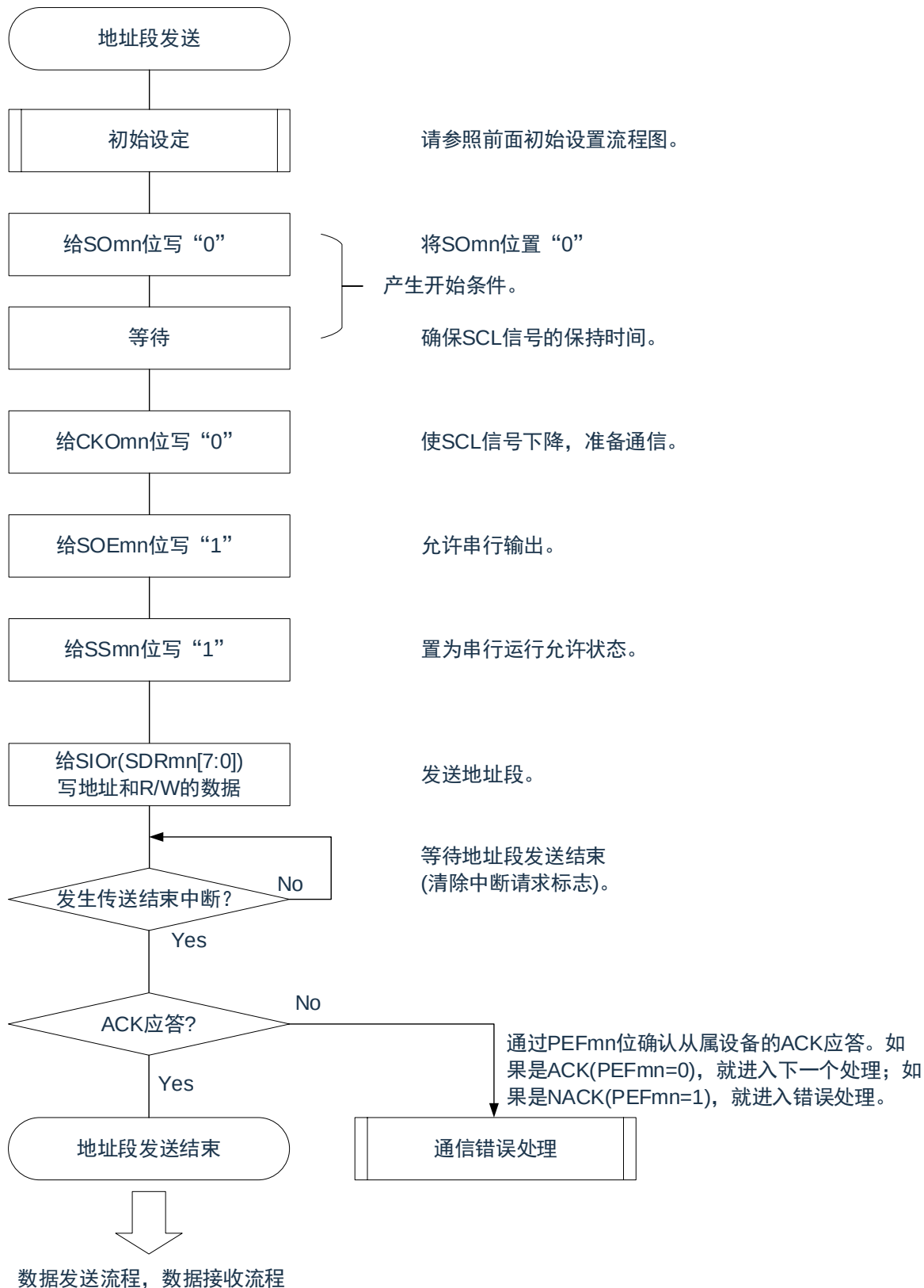
图 15-125：地址段发送的流程图
