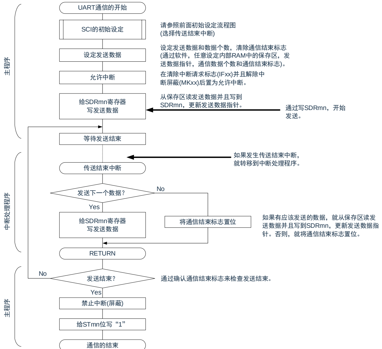
图 15-101: UART 发送（单次发送模式）的流程图
