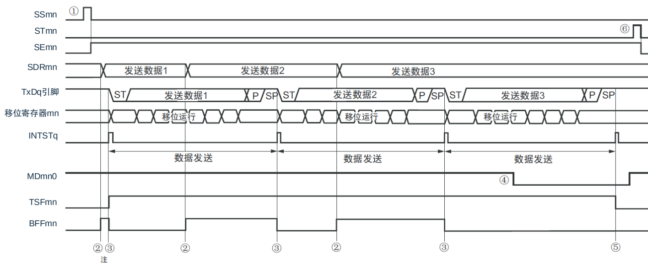
图 15-102: UART 发送（连续发送模式）的时序图
