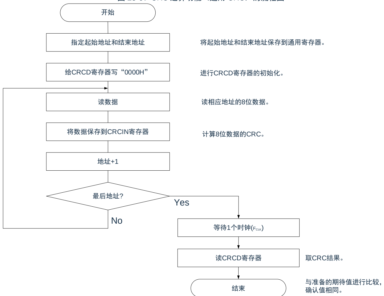
图 28-6: CRC 运算功能（通用 CRC）的流程图
