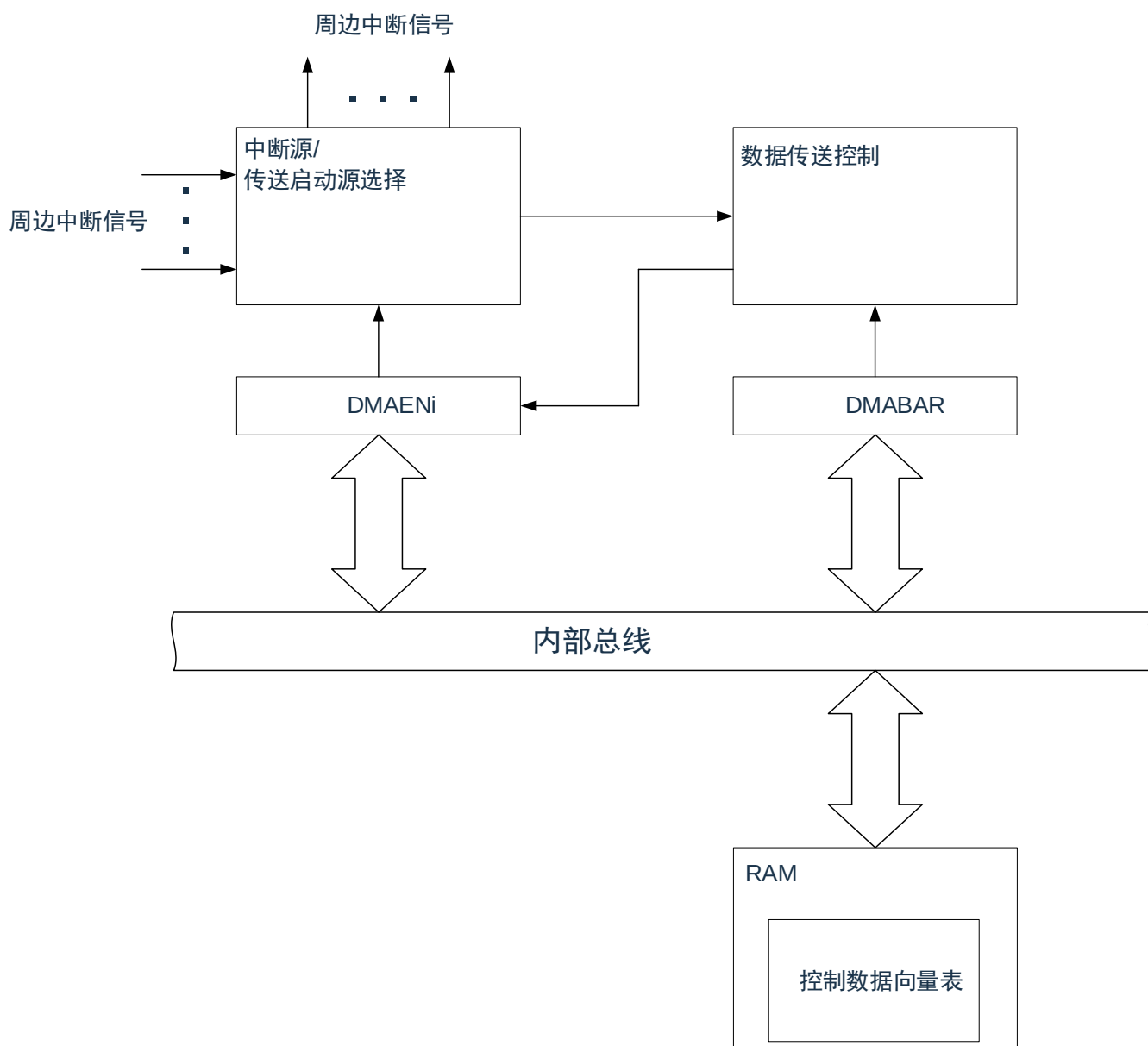
图 20-1：DMA 的框图
