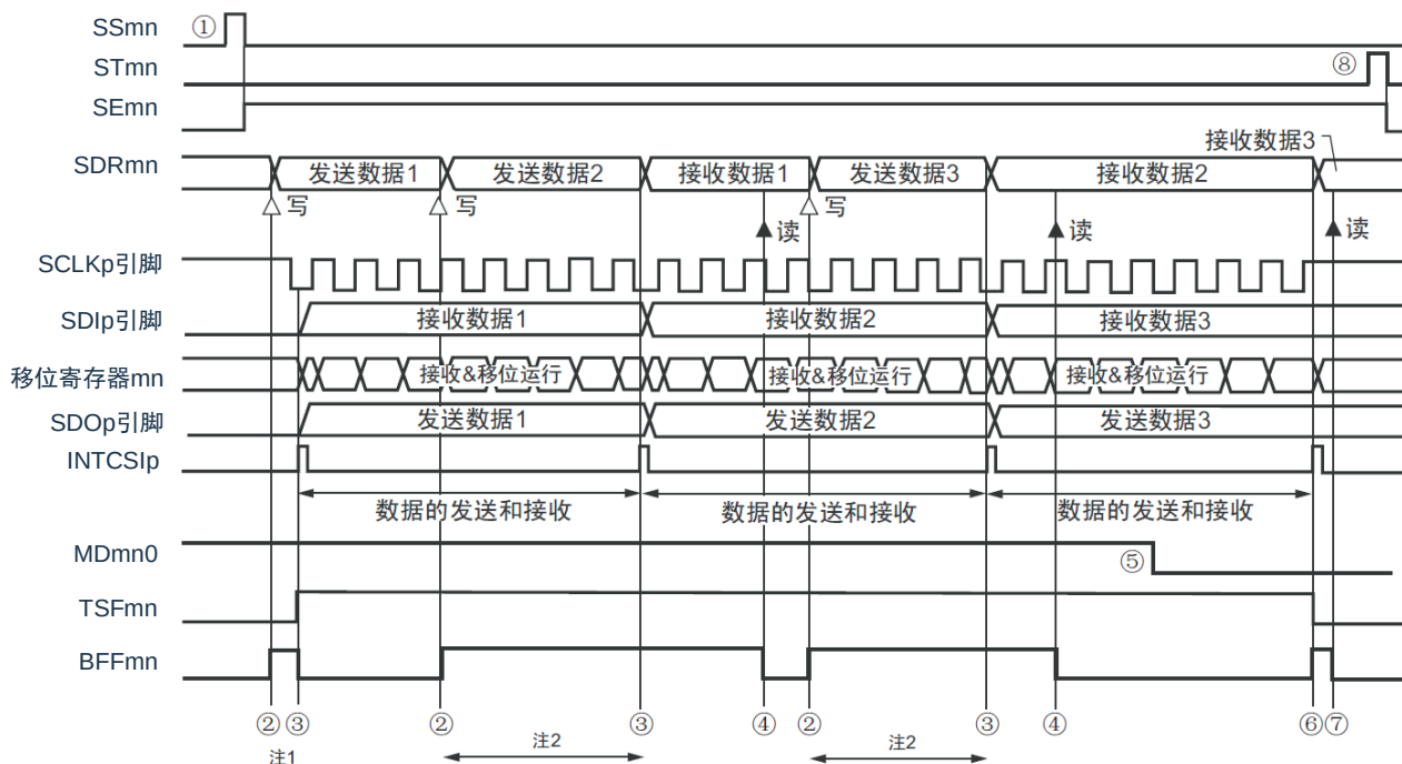
图 15-67：从属发送和接收（连续发送和接收模式）的时序图（类型 1：DAPmn=0、CKPmn=0）
