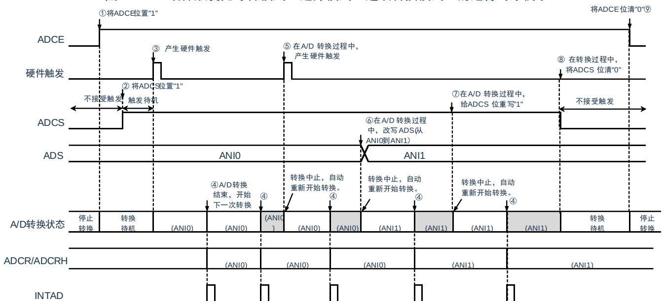
图 11-22：硬件触发无等待模式（选择模式、连续转换模式）的运行时序例子
