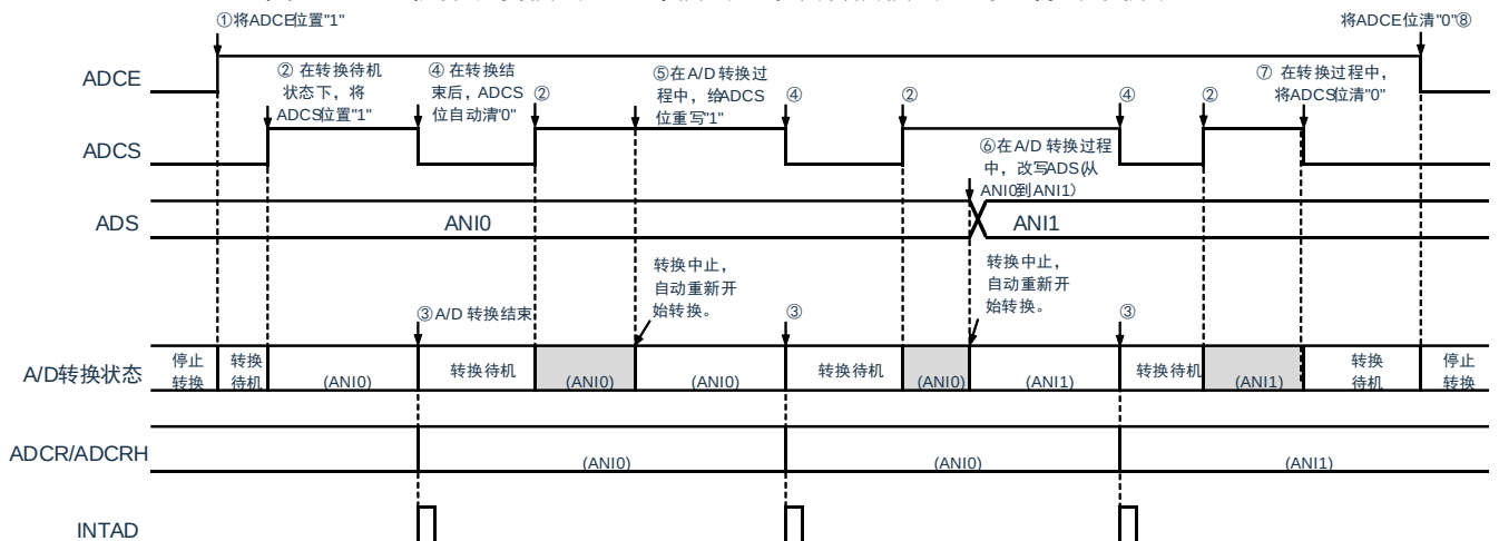
图 11-19：软件触发模式（选择模式、单次转换模式）的运行时序例子
