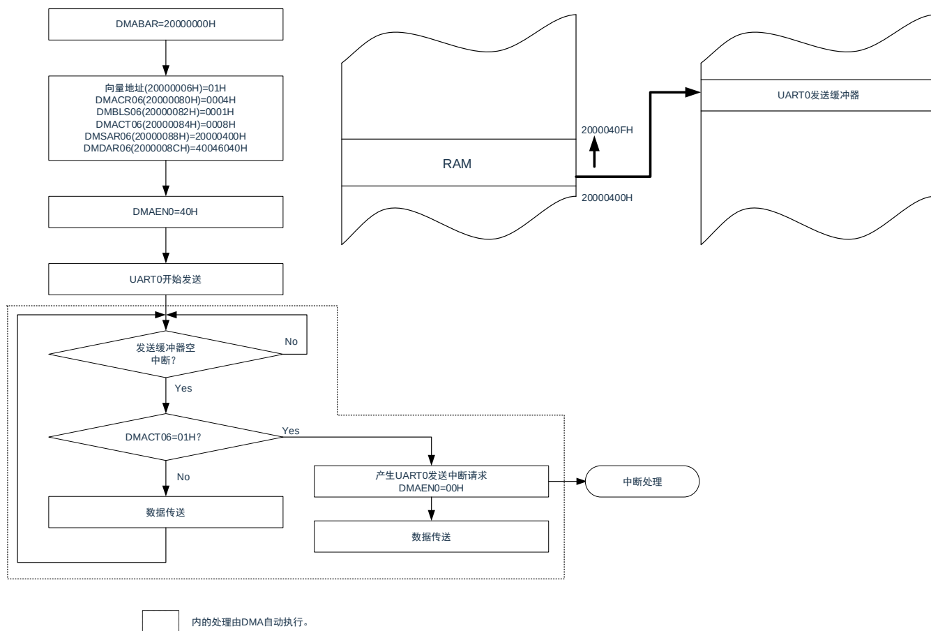
图 20-18: 正常模式的使用例子 2: UART0 连续发送
