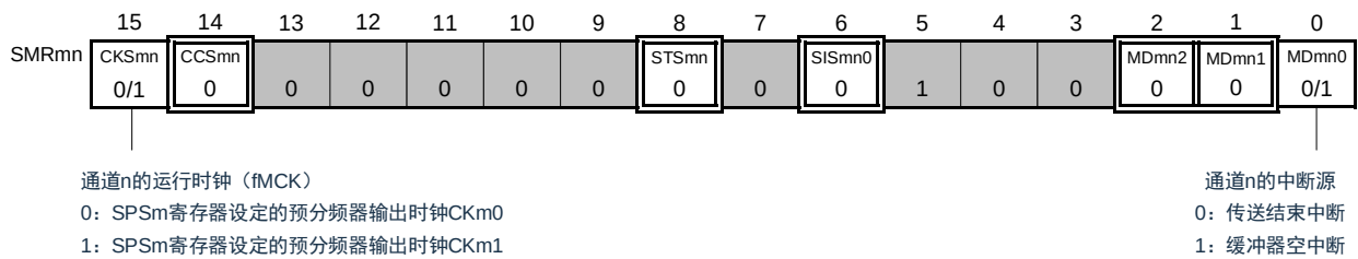
图 15-23: 3 线串行 I/O (SSPI00、SSPI01、SSPI10、SSPI11、SSPI20、SSPI21) 主控发送时的寄存器设定内容例子
