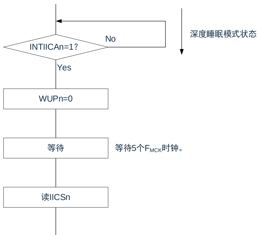
图 17-22：通过地址匹配将 WUPn 位置“0”时的流程（包括接收扩展码）
