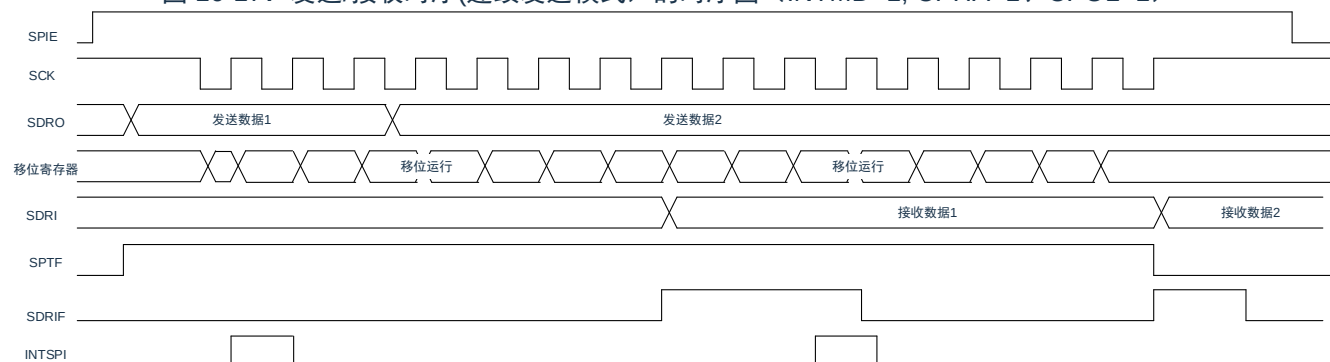
图 16-17: 发送/接收时序(连续发送模式)的时序图 (INTMD=1, CPHA=1、CPOL=1)
