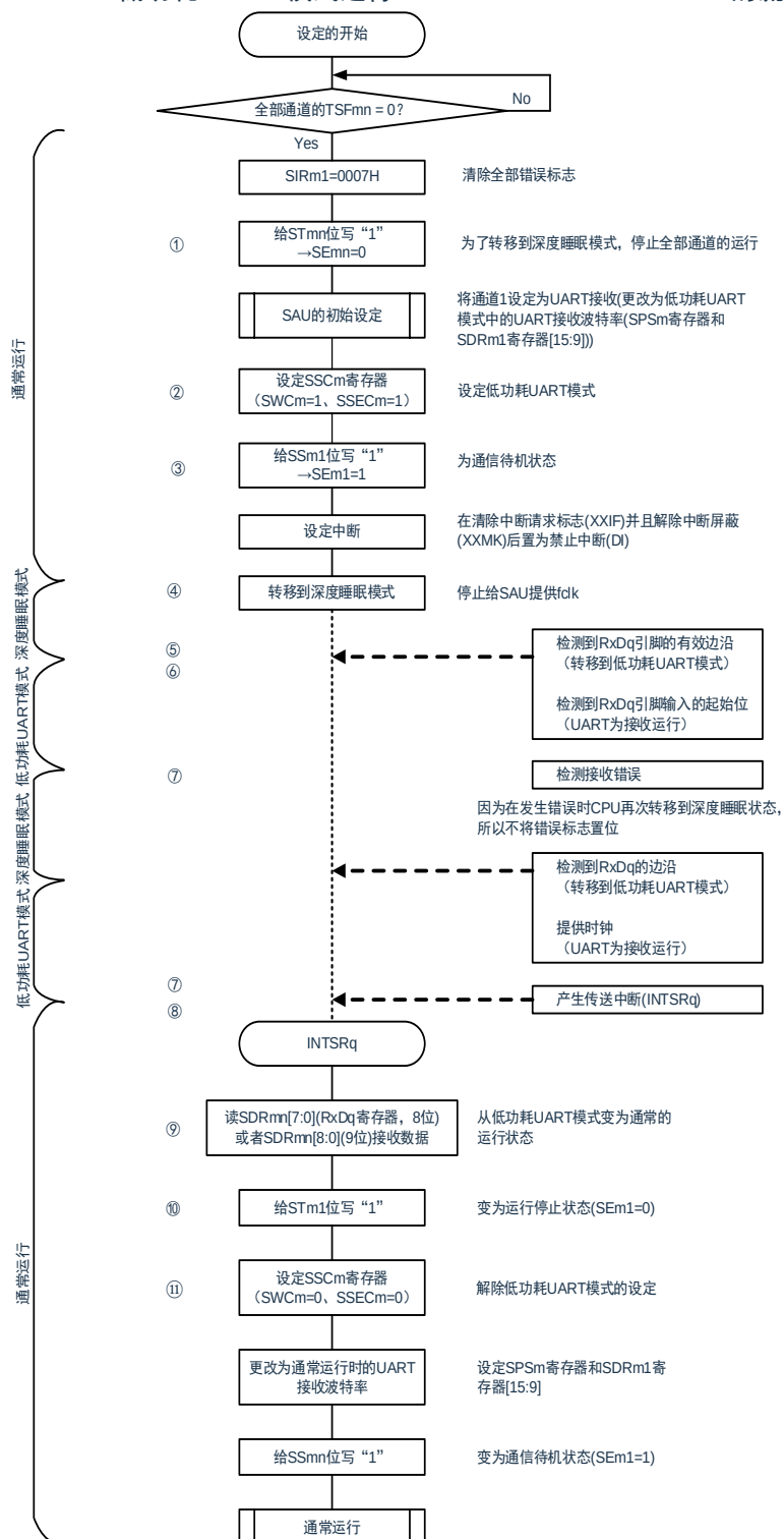
图 15-113: 低功耗 UART 模式运行 (EOCm1=1、SSECm=1) 的流程图
