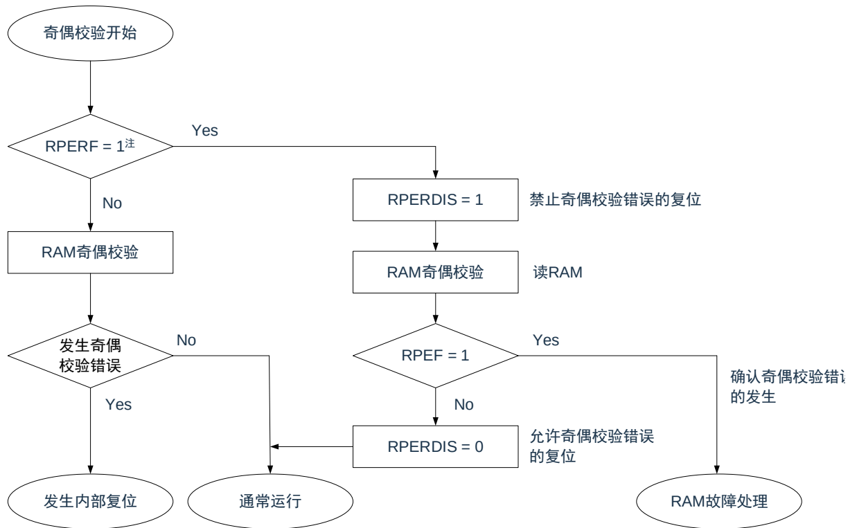
图 28-8：RAM 奇偶校验的流程
