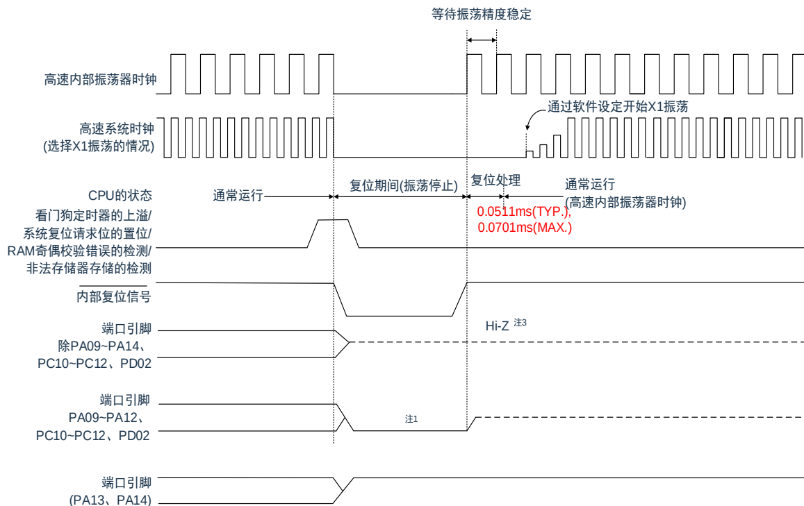
图 25-3: 因看门狗定时器的上溢、系统复位请求位的置位、RAM 奇偶校验错误的检测 或者非法存储器存取的检测而产生的复位时序
