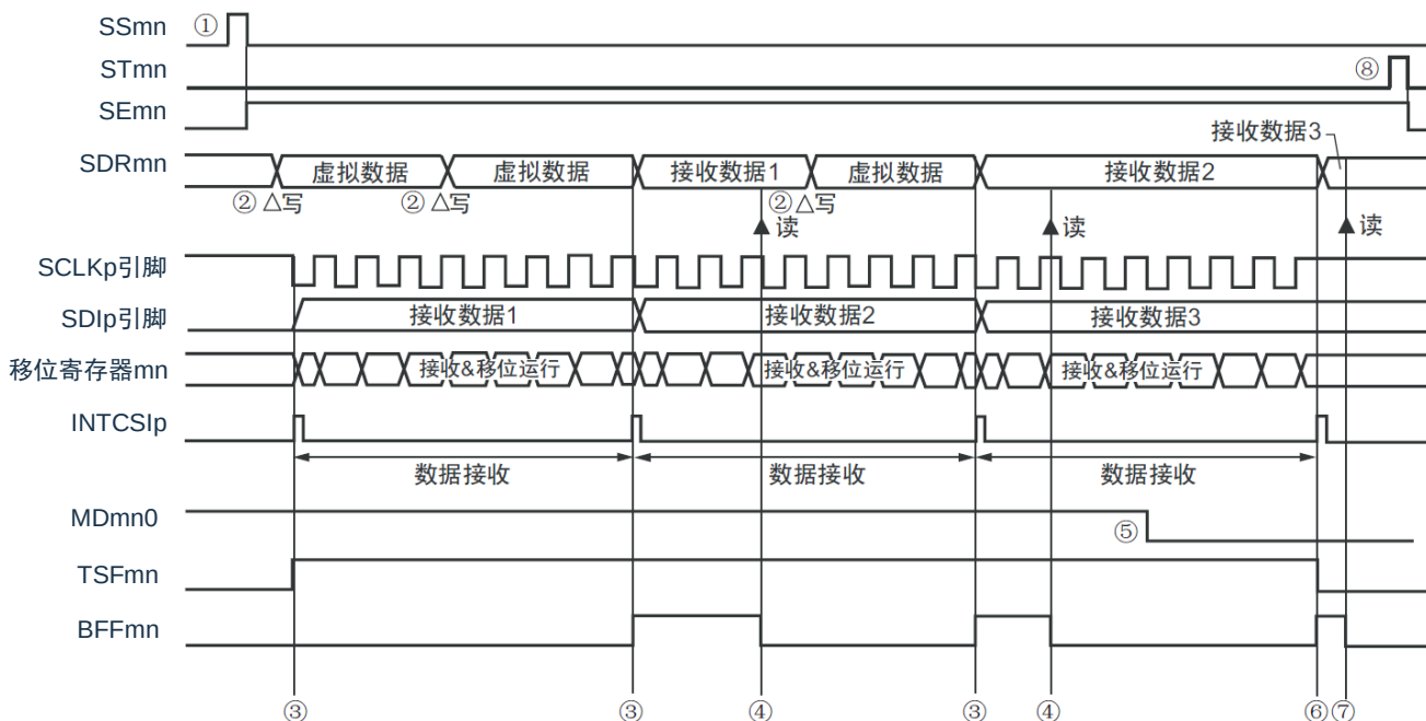
图 15-37：主控接收（连续接收模式）的时序图（类型 1：DAPmn=0、CKPmn=0）
