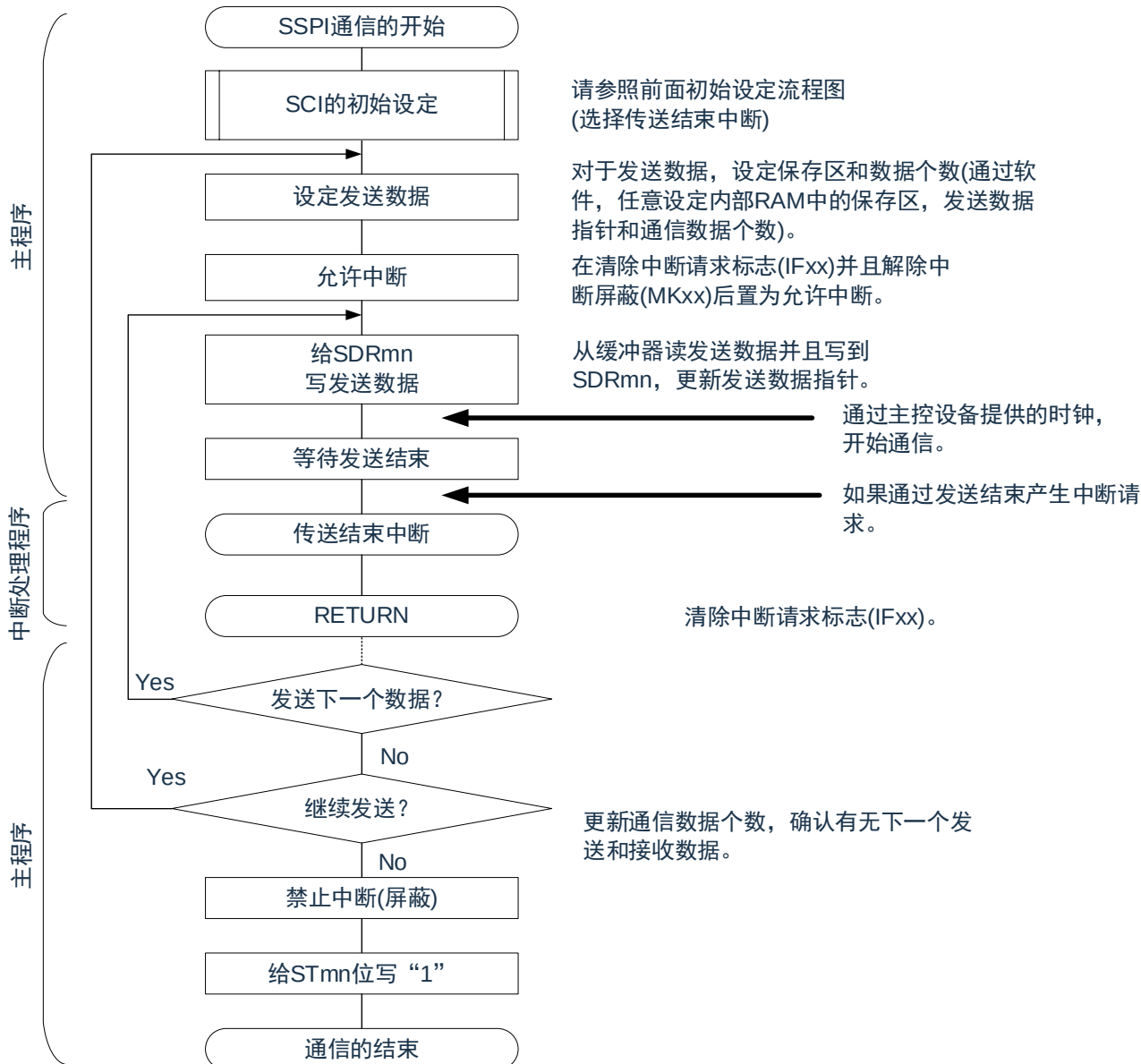
图 15-77: 从属发送（单次发送模式）的流程图
