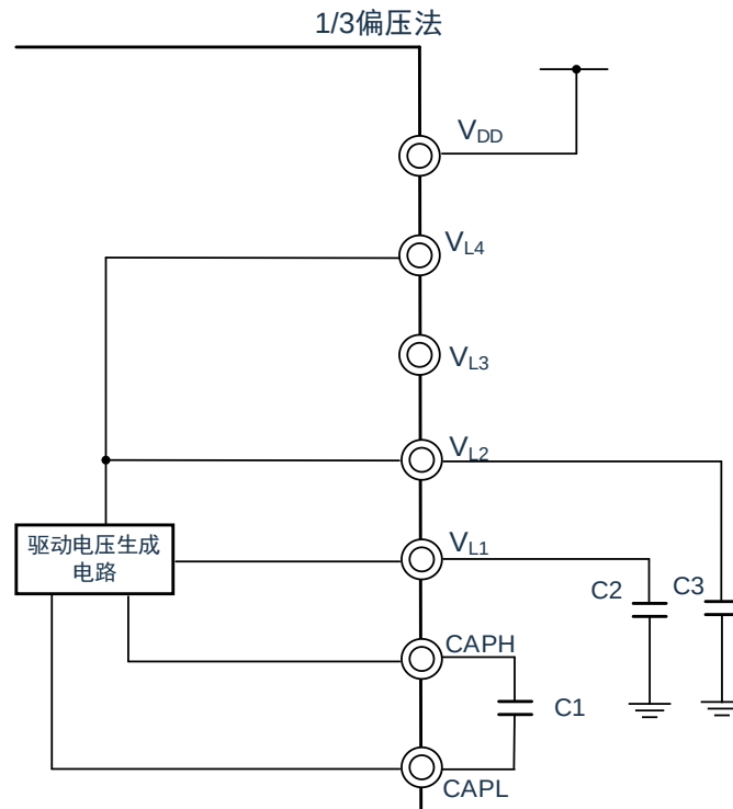
图 19-14：LCD 驱动电源的连接例子（电容分割方式）
