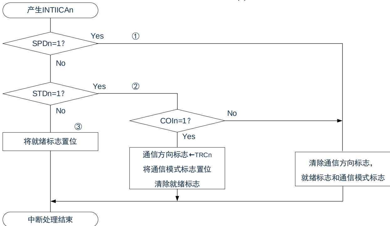
图 17-30：从属运行步骤(2)
