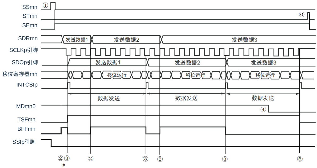
图 15-78：从属发送（连续发送模式）的时序图（类型 1：DAPmn=0、CKPmn=0）
