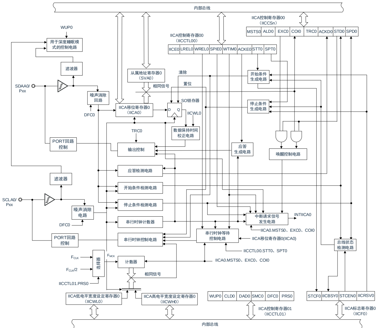
图 17-1: 串行接口 IICA 的框图
