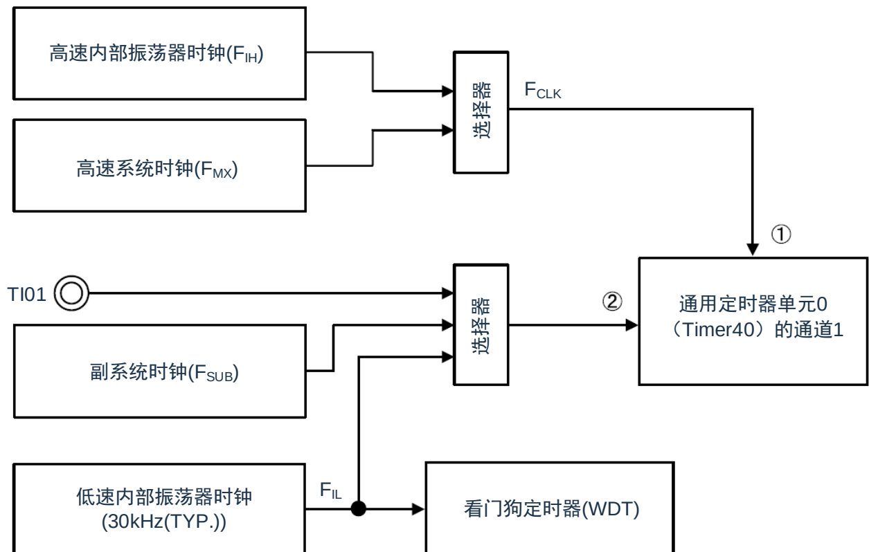
图 28-10：频率检测功能的结构
