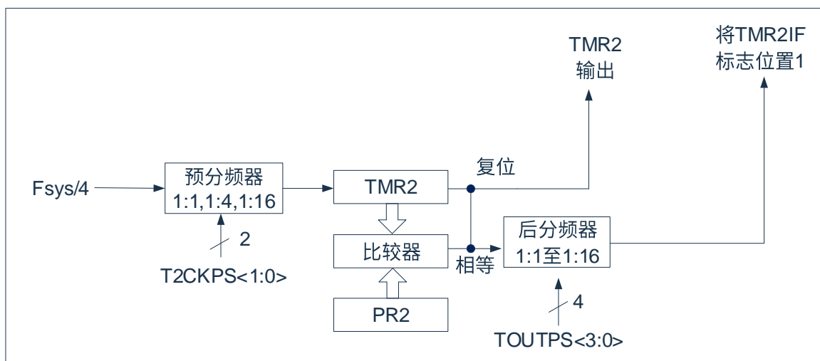
图 9-1: TIMER2 框图
