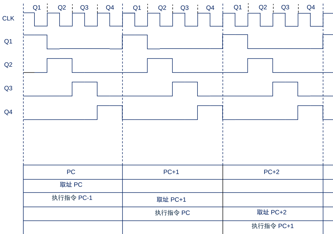
图 3-1：时钟与指令周期时序图
